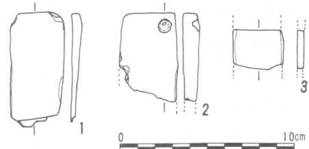
第14図 砥石
