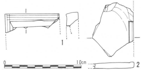
第13図 硯
