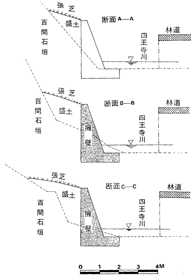
断面計画図
