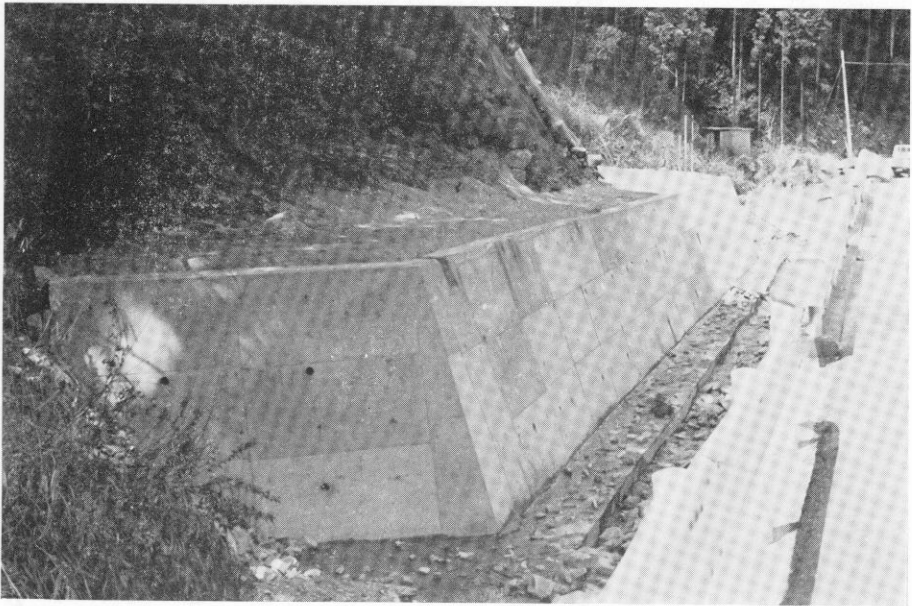
図版13 百間石垣保全工事
