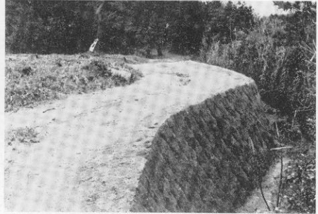
図版40 主城原礎石建物跡基壇保全工事
