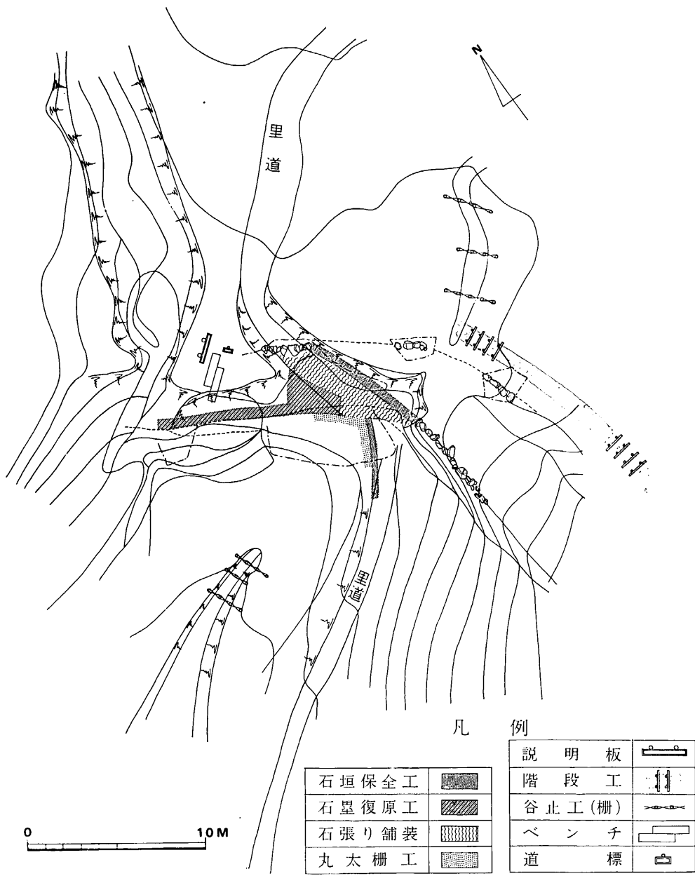
第4図 大石垣遺構復原保全工事
