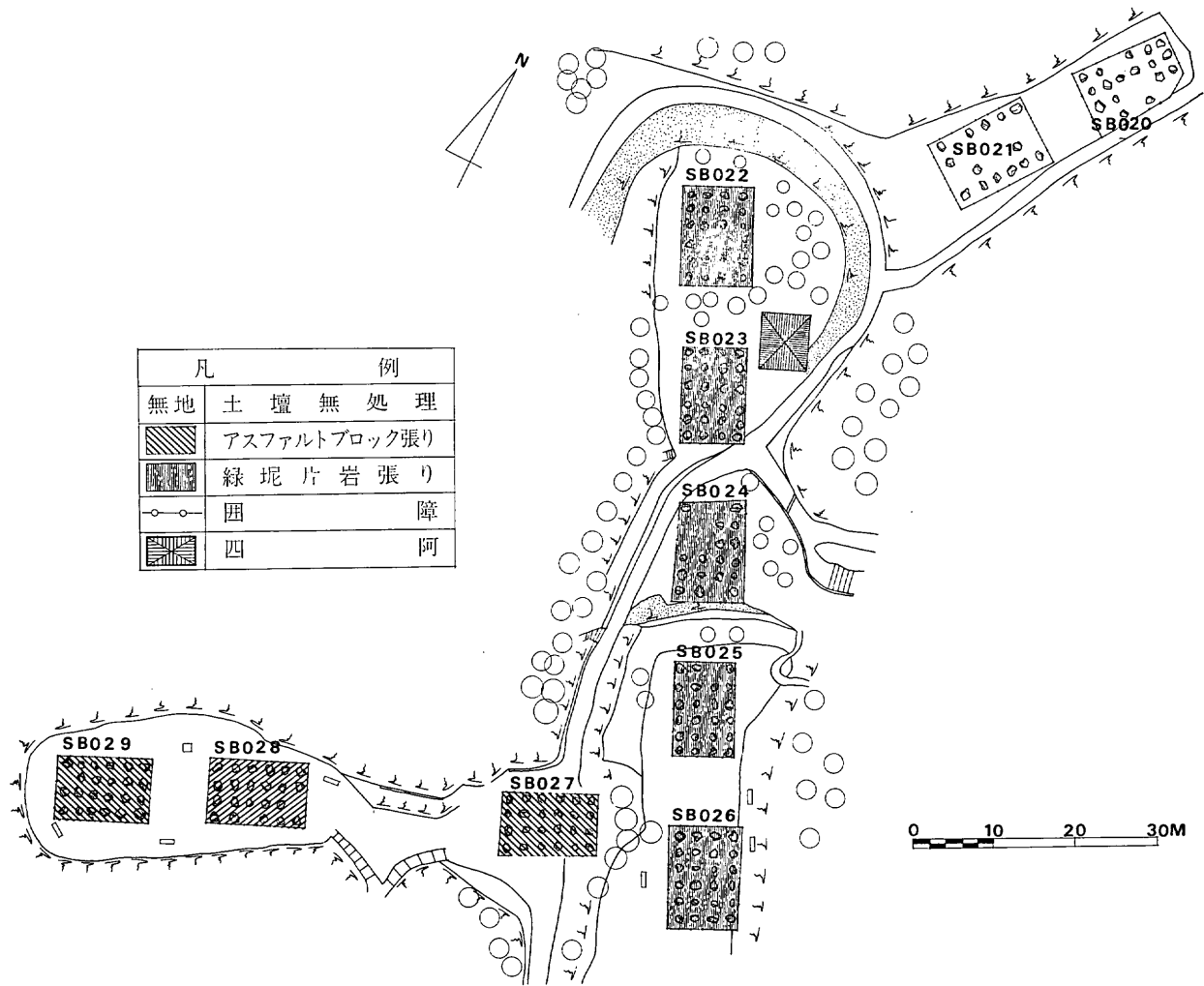
第5図 尾花礎石建物跡群整備工事
