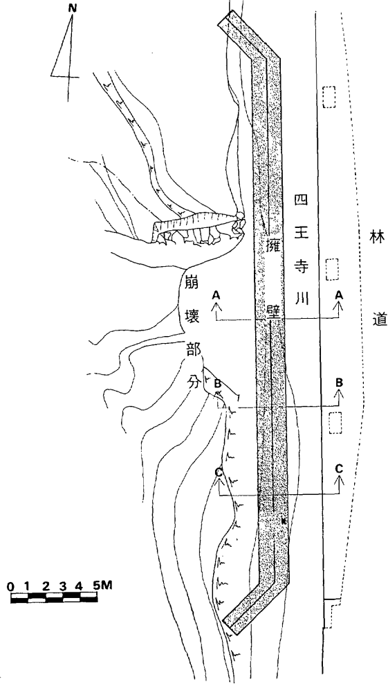
平面計画図
