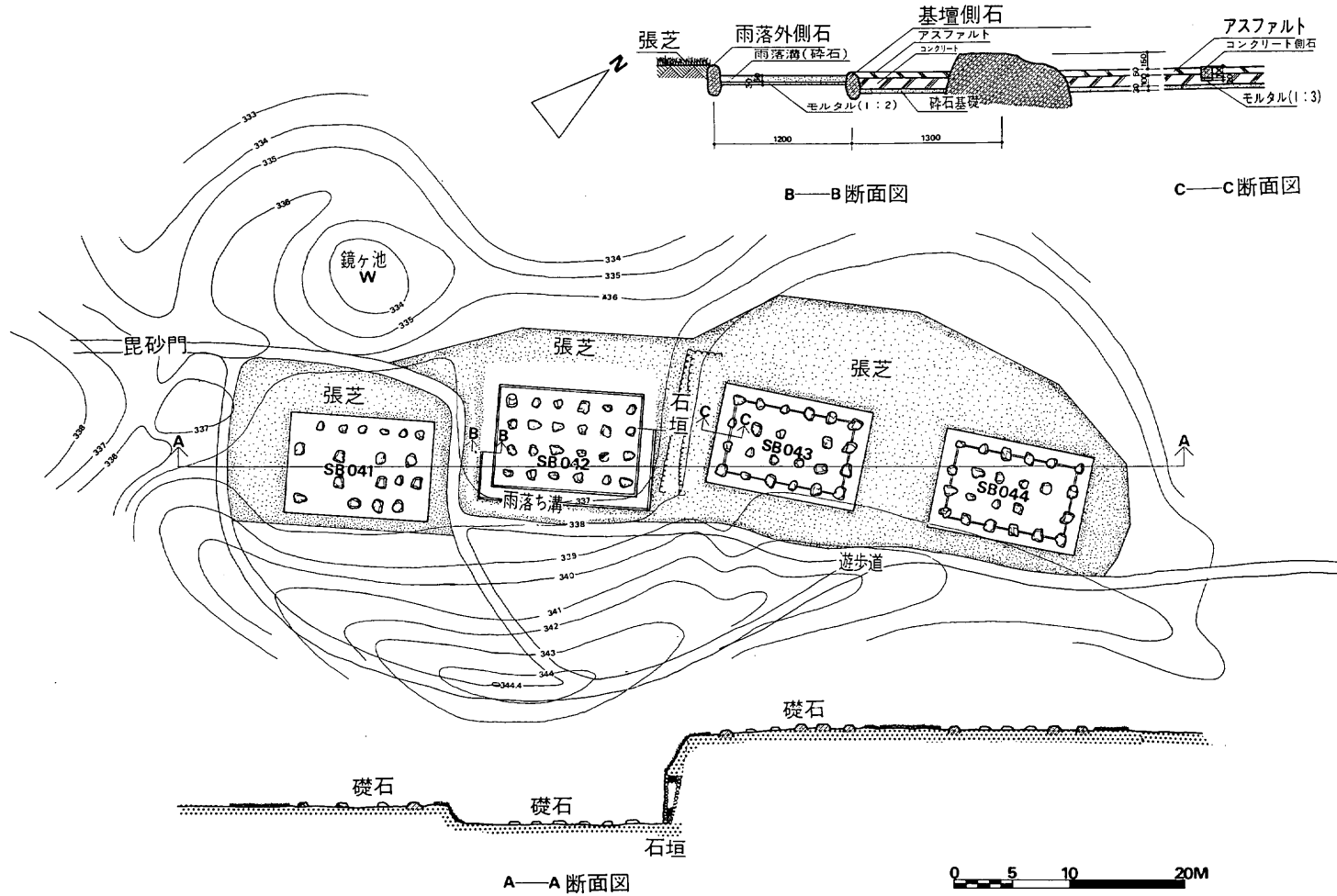
第6図 増長天礎石建物跡群整備工事
