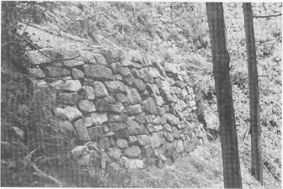
図版15 石積復原工事
