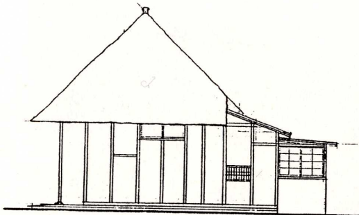
東面立面図
