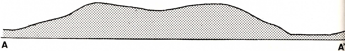
中二子古墳 墳丘断面図
