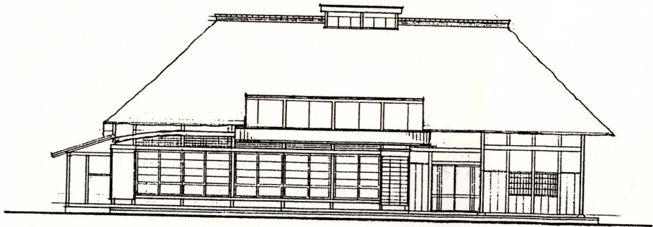
南面立面図
