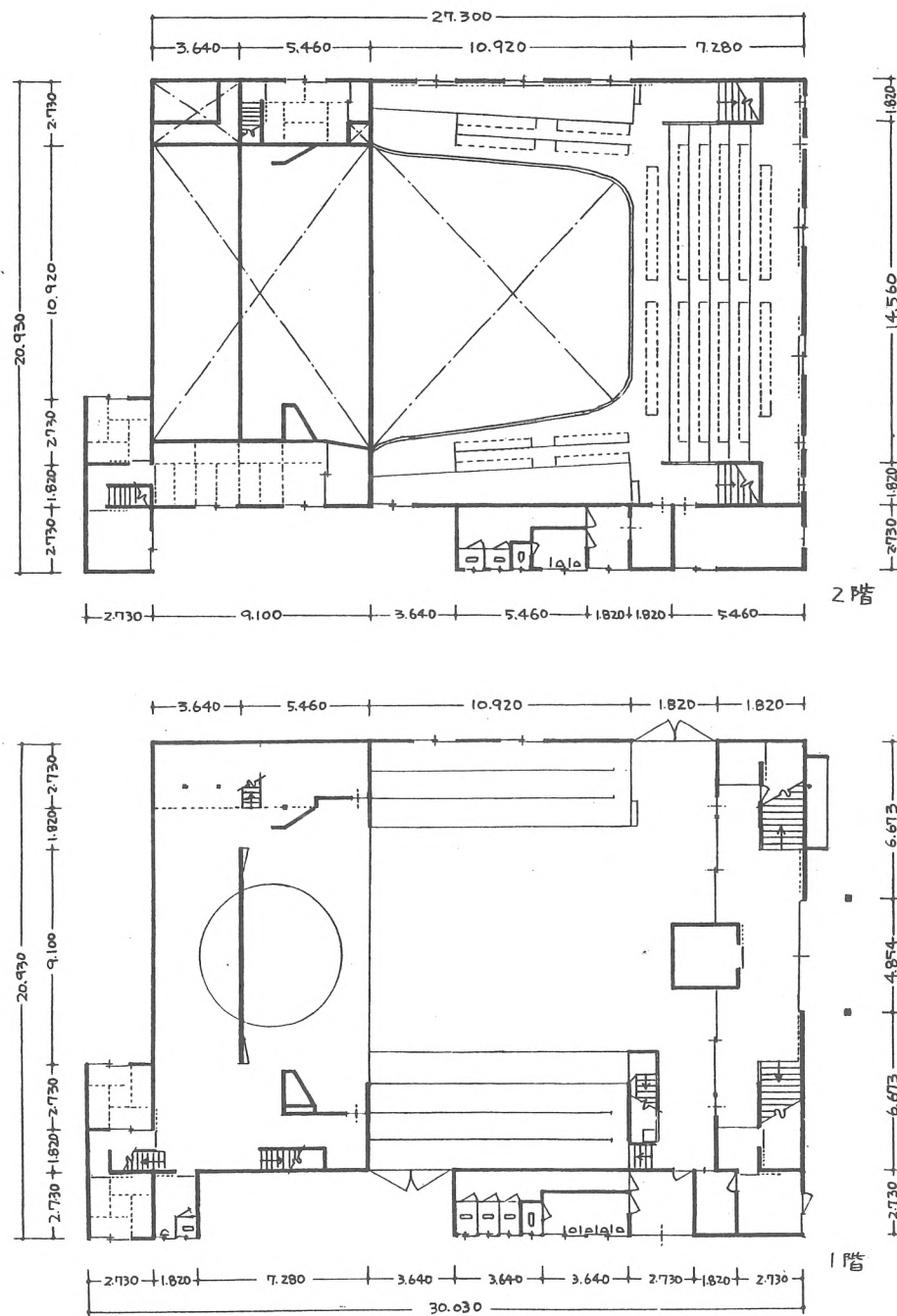
実測平面図 - 図 85
