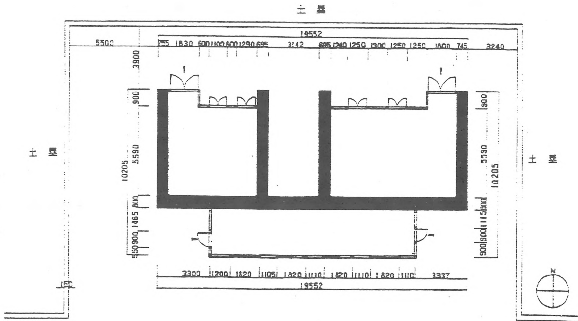
黒色火薬製造工場実測平面図 - 図89
