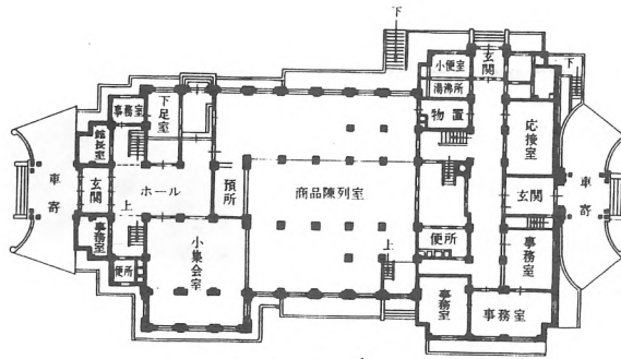
1階平面図 \frac{1}{400}
