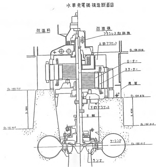
改造工事前後水車発電機断面図 - 図61
