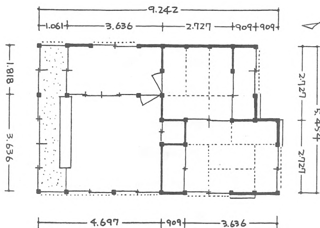
創業事務所実測平面図-図66
