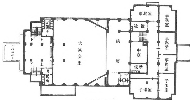
2階平面図 \frac{1}{400}
