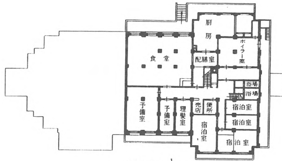
地階平面図 \frac{1}{400} (当初の部屋配置、以下同様)
