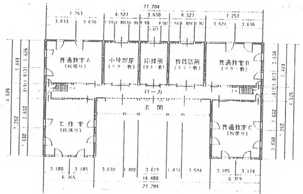
1階平面図 - 図74
