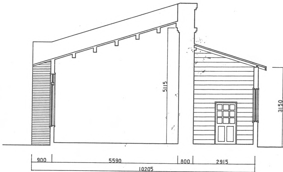
黒色火薬製造工場実測断面図 - 図90
