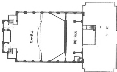
4階平面図 \frac{1}{400}
