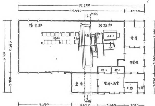
野口水車実測平面図 - 図 79
