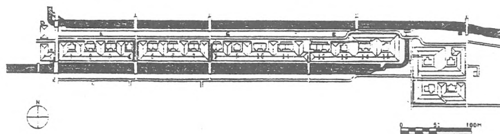
黒色火薬地帯工場配置図（日本化薬(株)岩鼻作業所時代、昭和33年）- 図88
