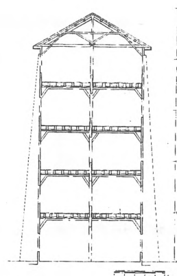
工場断面図-図67
