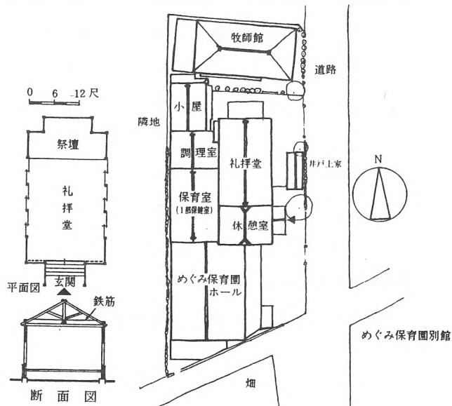
平面図・配置図-図84
