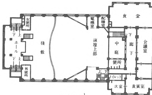
3階平面図 \frac{1}{400}
