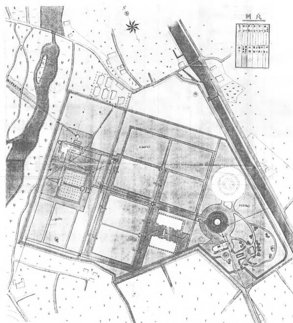
浄水場配置図 - 写真133
