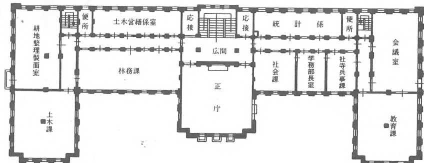
3階平面図
