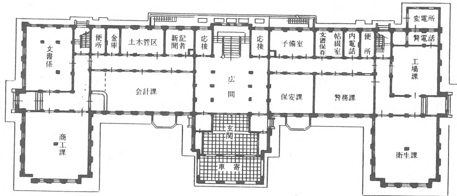
1階平面図
