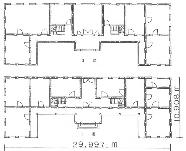
平面図-図72
