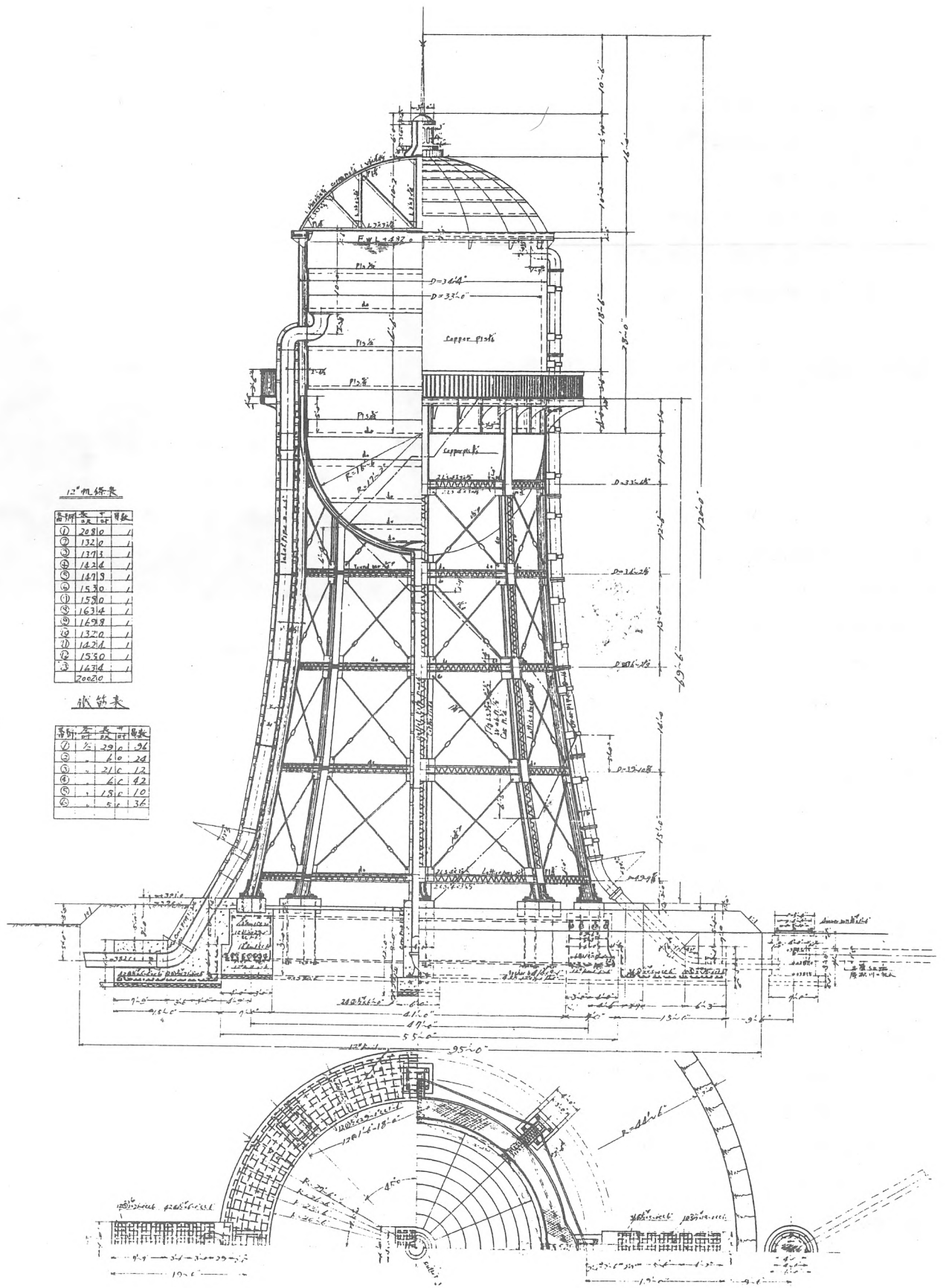
配水塔設計圖 - 圖80
