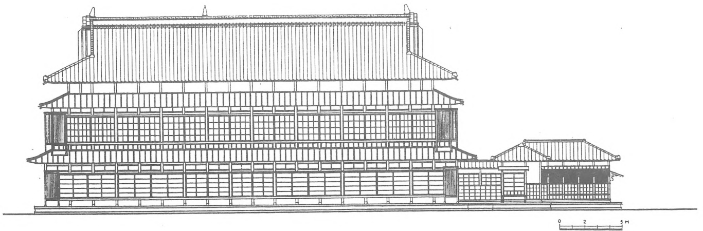
別館復元図（側面） - 図70
