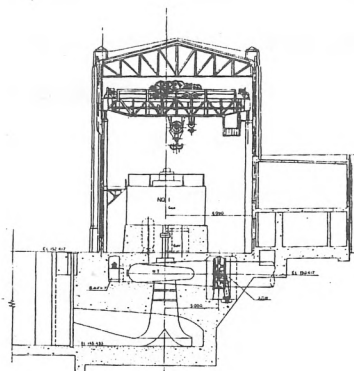
本屋建屋断面図-図60
