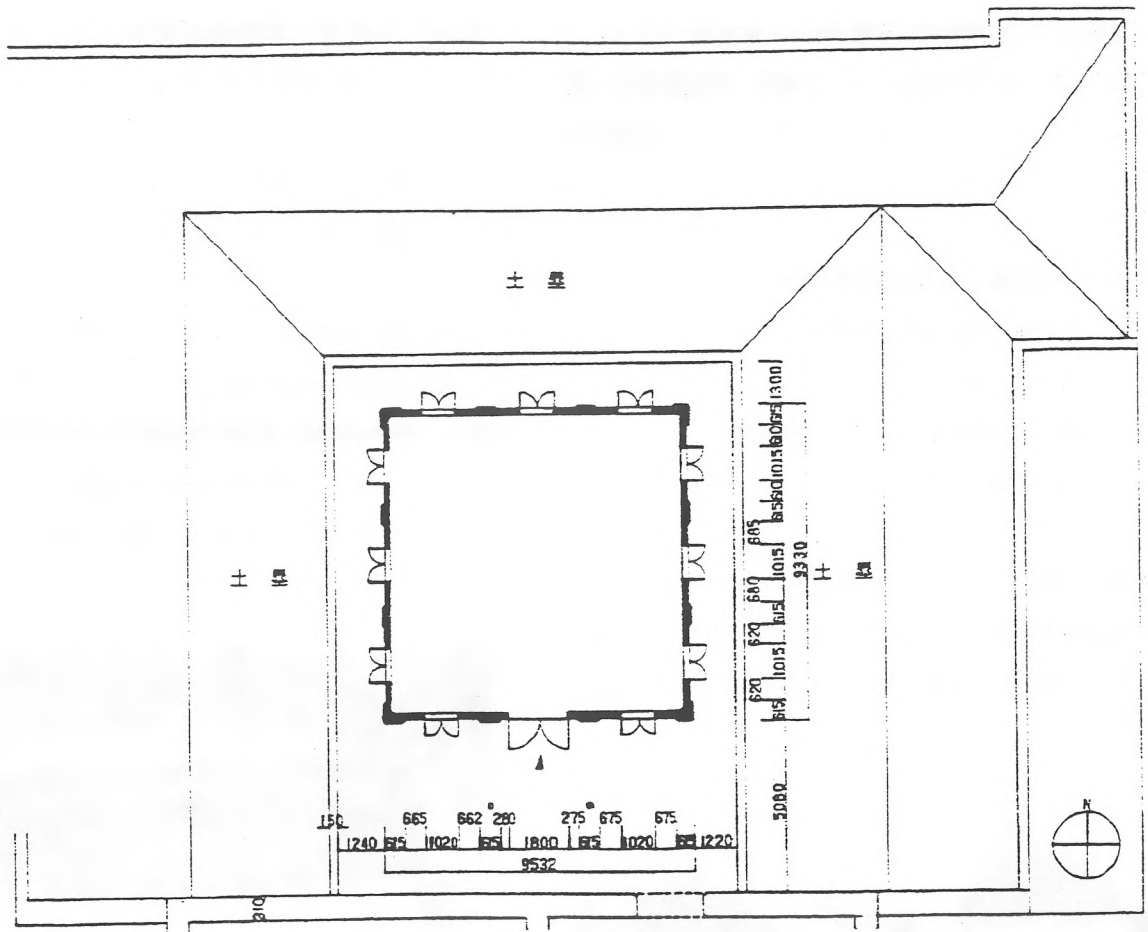
火薬一時置場実測平面図-図91
