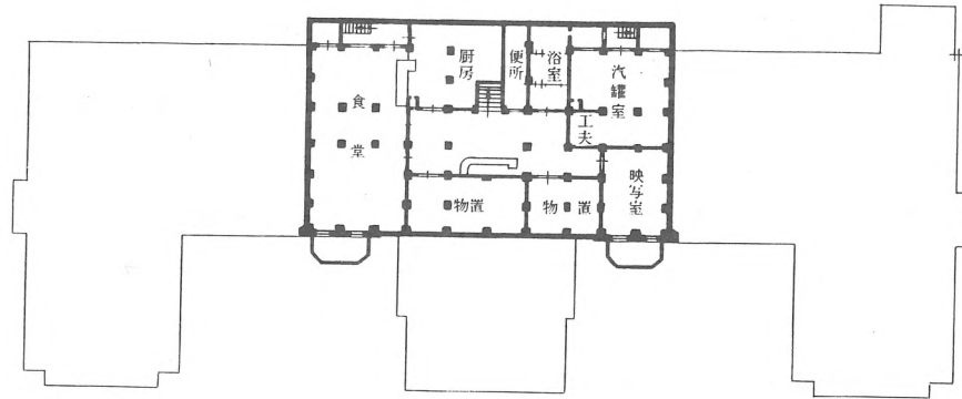
地階平面図 (当初の部屋配置、以下同様)
