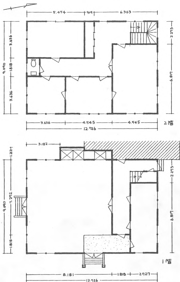
記念館実測平面図-図65
