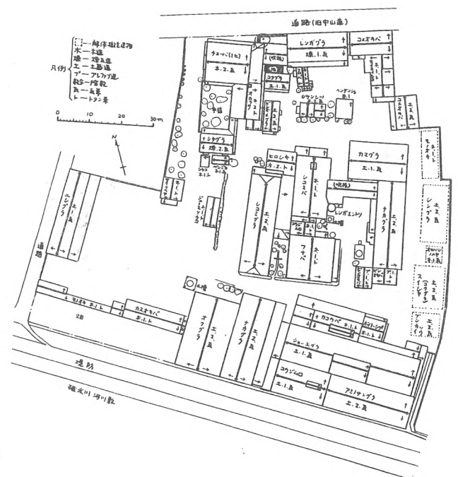
配置図 - 図64
