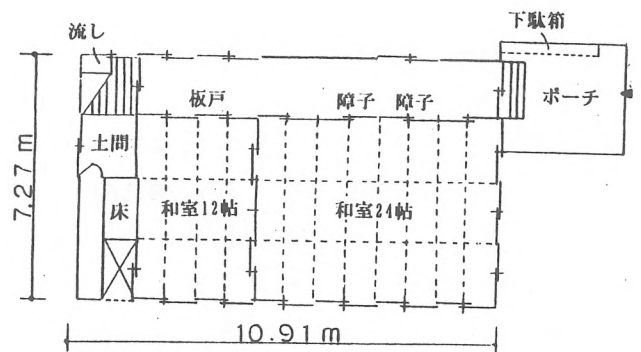
旧大岩分校実測平面図 - 図73
