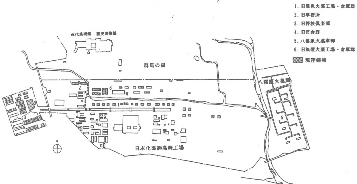
旧岩鼻火薬製造所配置図(現状) - 図87
