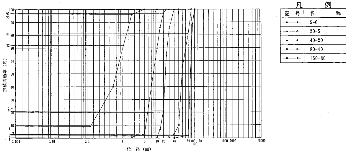
第307図 原石山骨材の粒度分布
