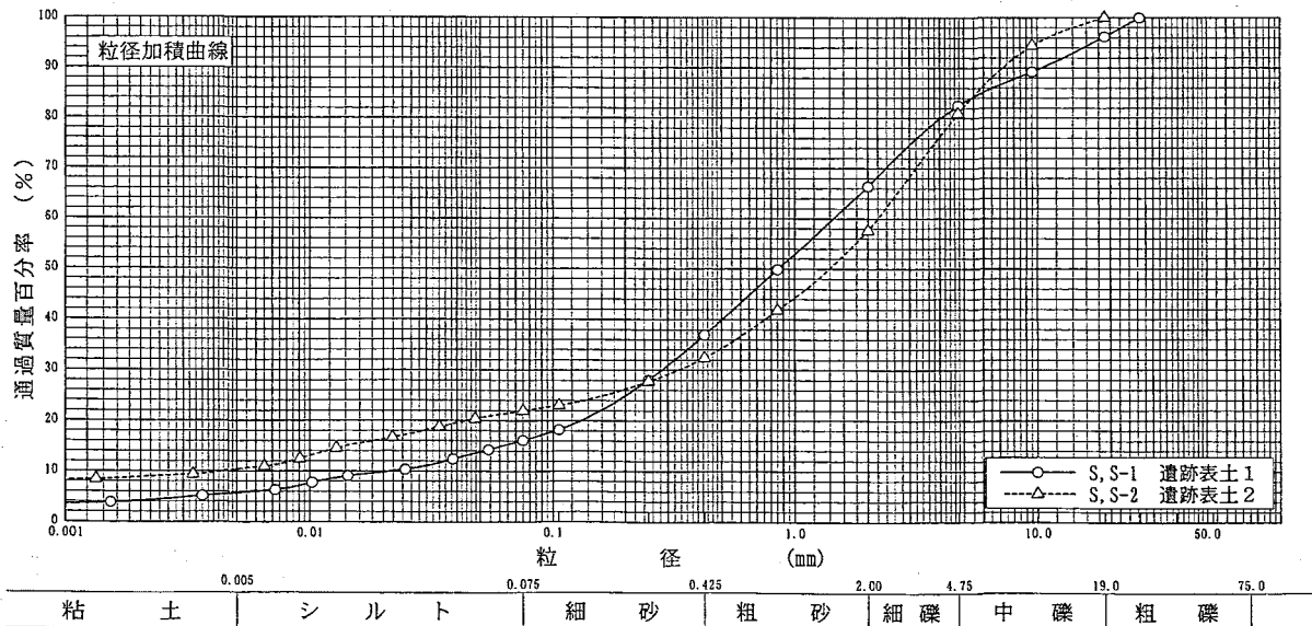
第299図 粒径加積曲線
