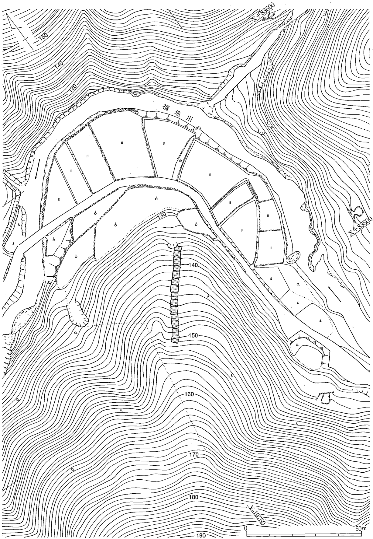
第17図 内ヶ磯窯跡周辺地形測量図 (1/1,000)
