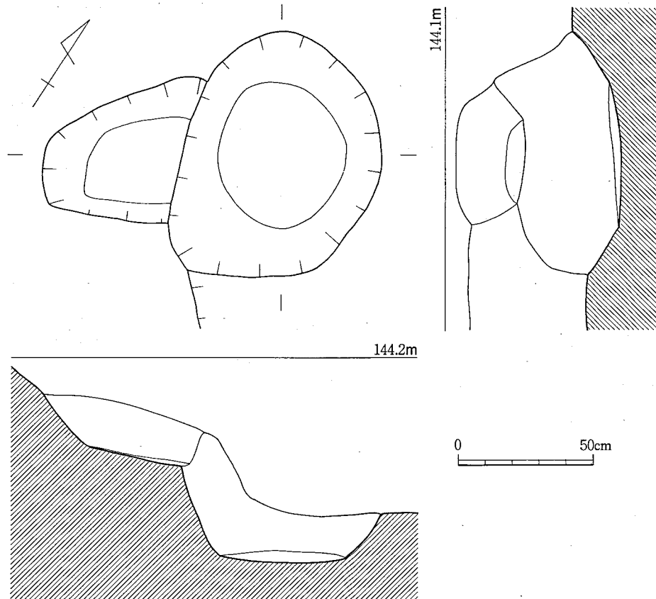
第100図 東物原土壌27実測図 (1/20)
