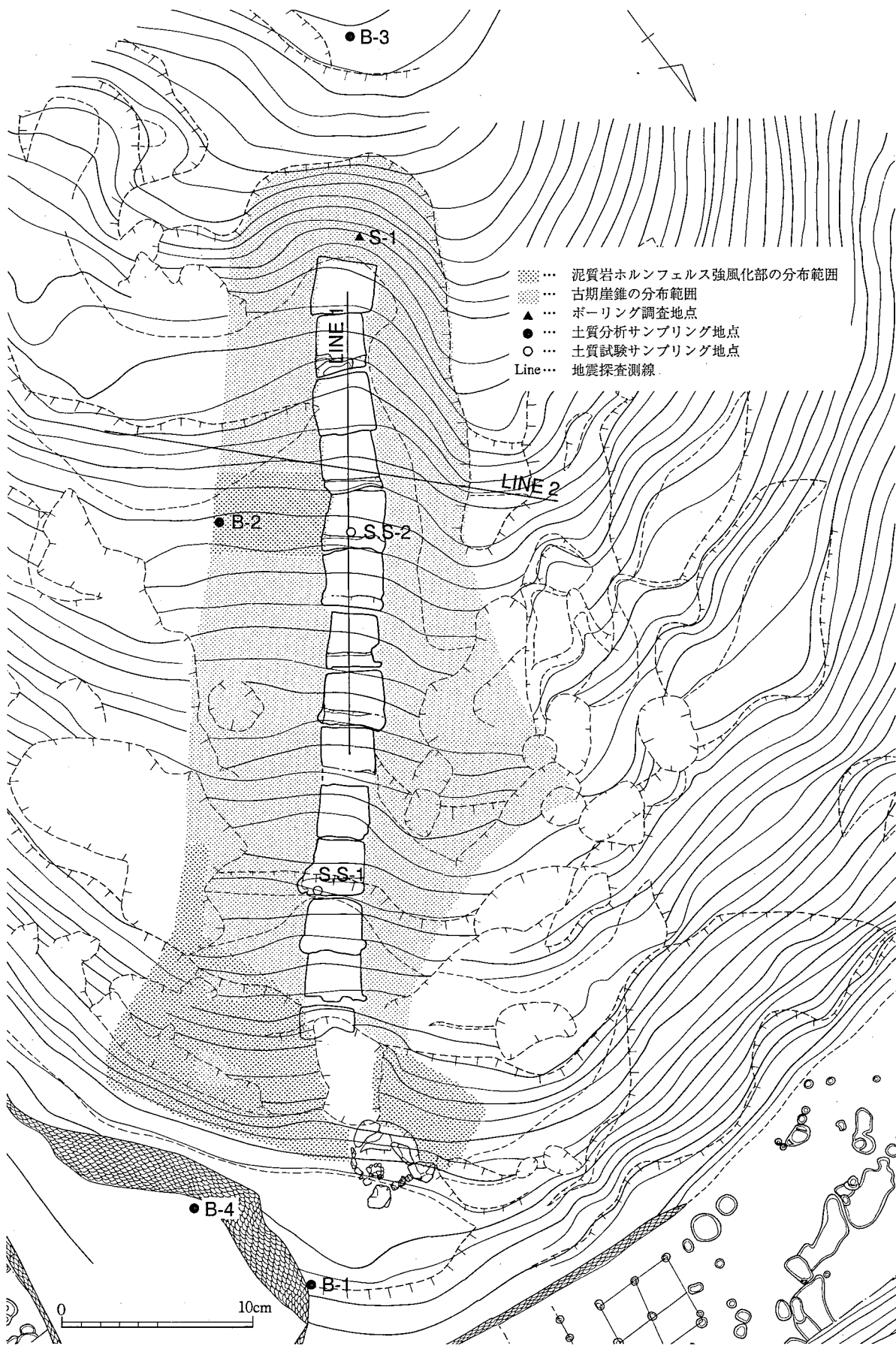
第301図 表層地質図
