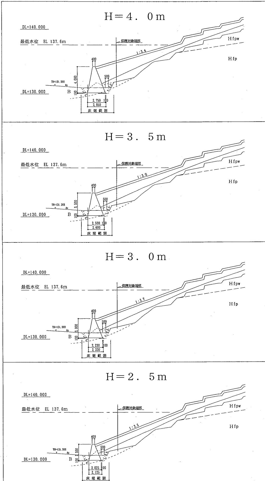
第312図 擁壁高と法面勾配の検討図
