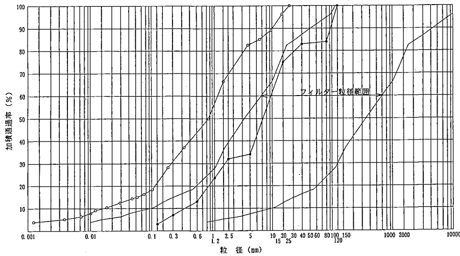
第308図 窯跡フィルター（原石山骨材）
