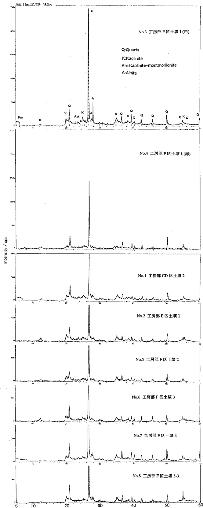
第320図 粘土のX線解析パターン
