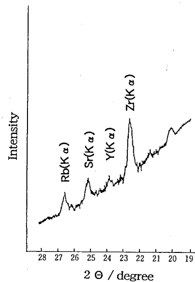
第315図 指標重元素部の蛍光X線スペクトル
