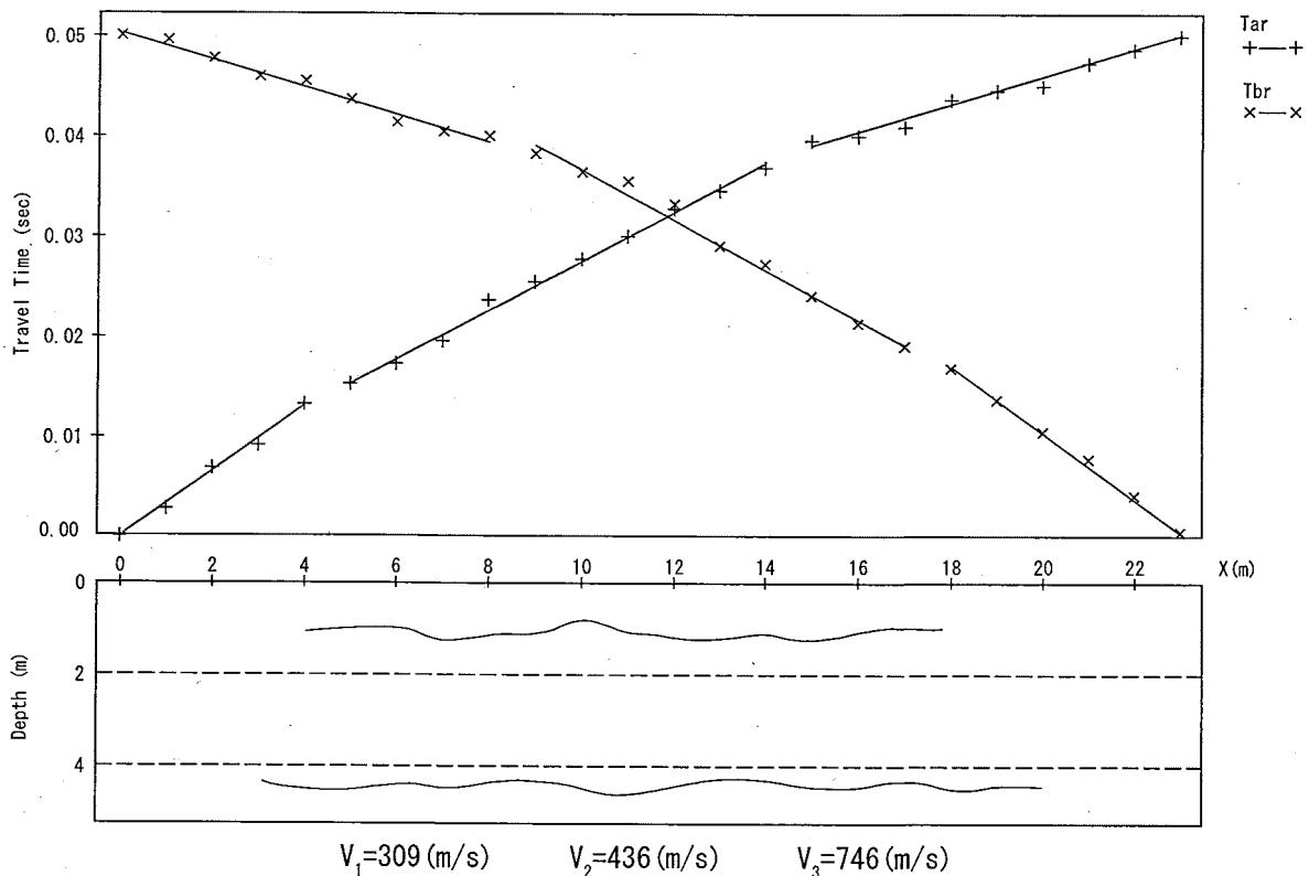
第303図 窯跡の主軸方向の弾性波探査の走時曲線および解析断面図
