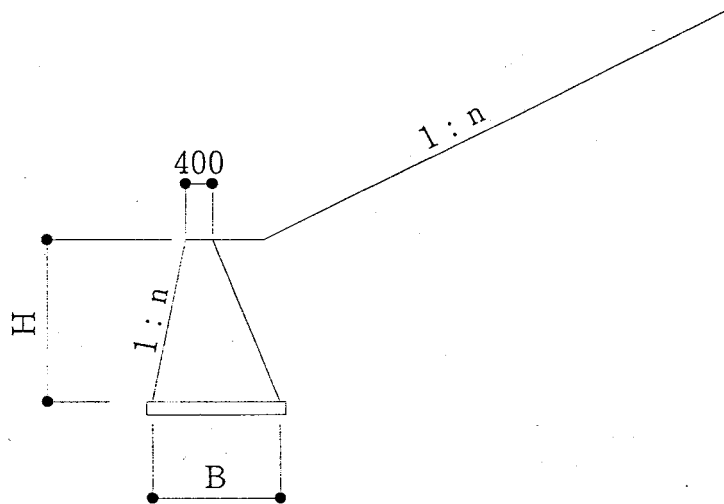
第311図 安定検討の基本的断面形状図
