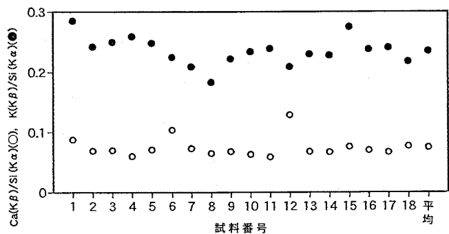
第319図 Ca(K\beta)/Si(K\alpha) , K(K\beta)/Si(K\alpha)
