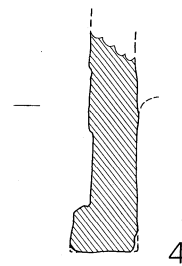
第8图 出土瓦実測图(1)
