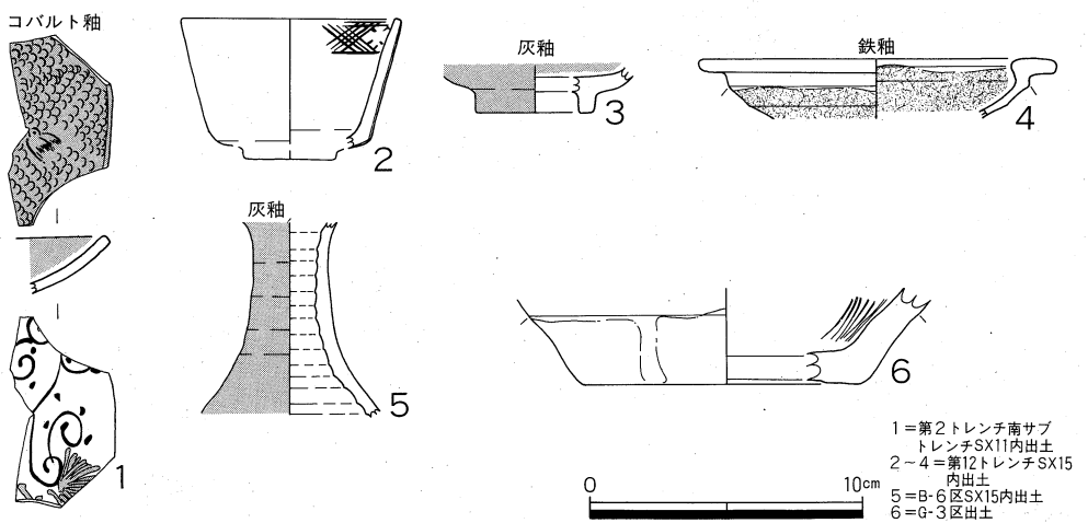
第22図 出土陶磁器実測図(1)
