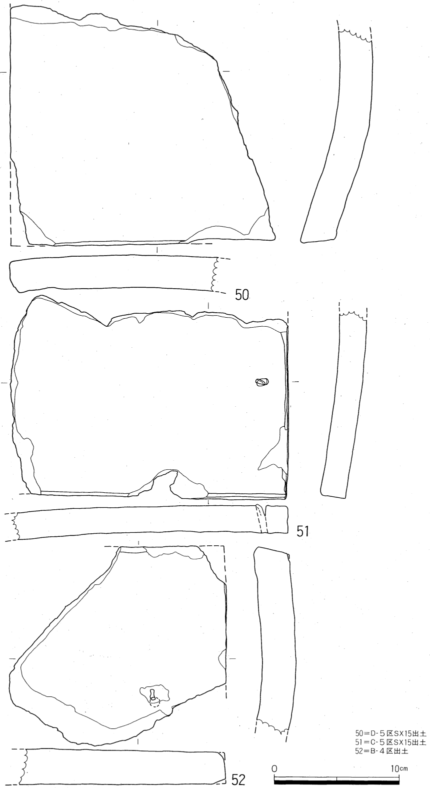
第15图 出土瓦実測图(8)
