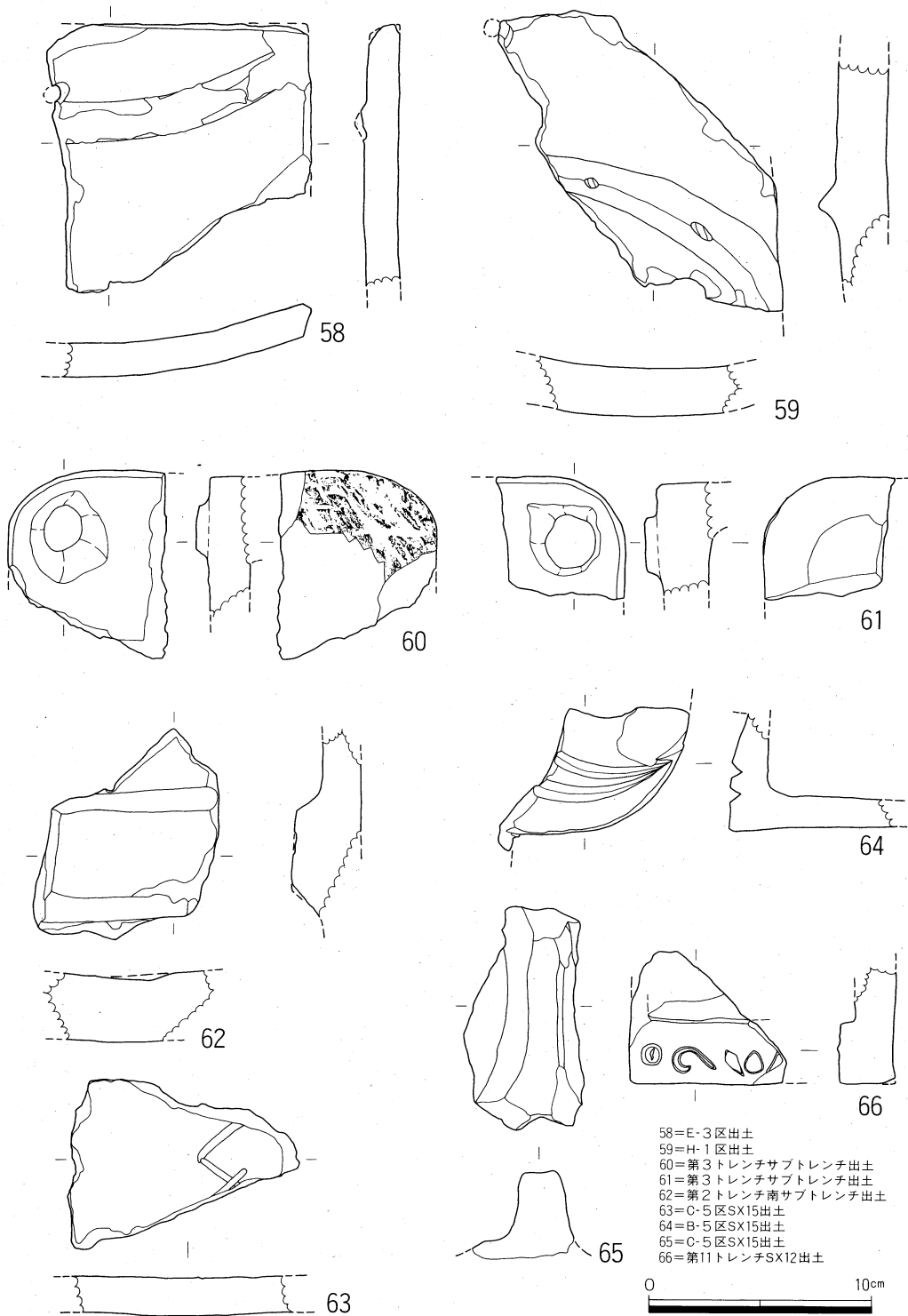
第17図 出土瓦実測図(10)
