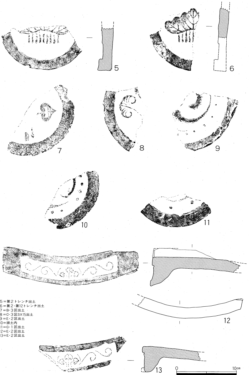
第9図 出土瓦実測図(2)
