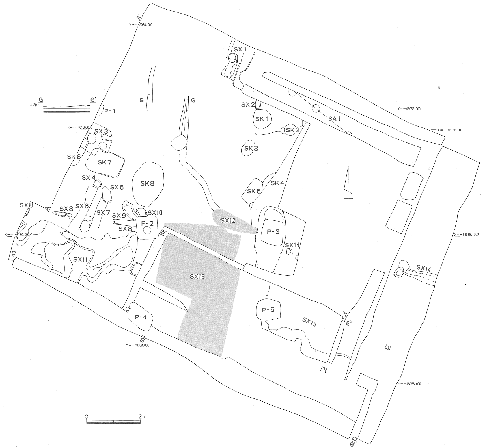
第3図 遺構全体図
