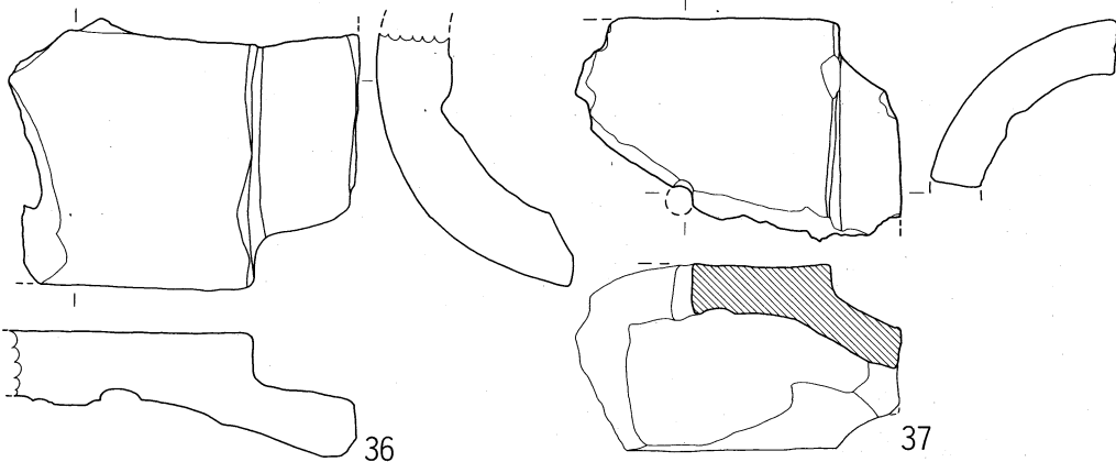
第12図 出土瓦実測図(5)
