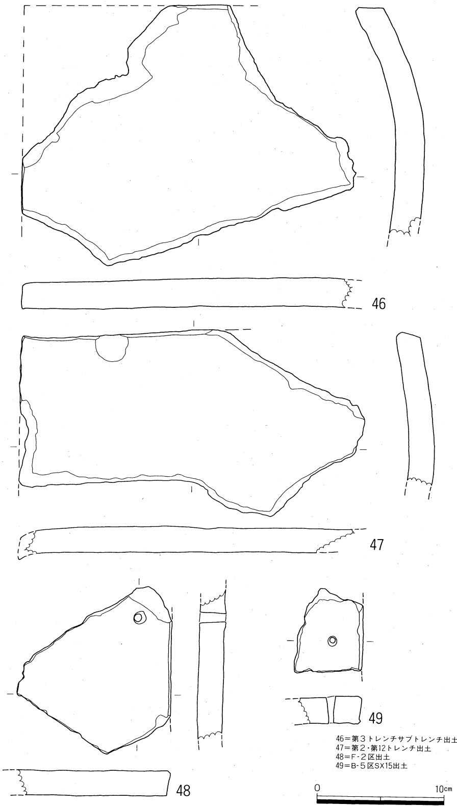
第14図 出土瓦実測図(7)
