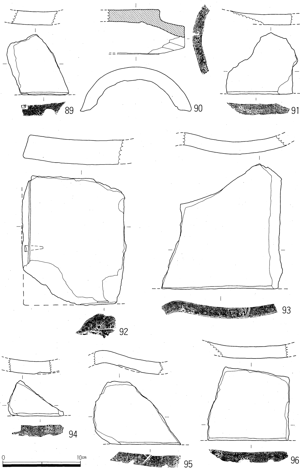
第20図 出土刻印瓦実測図(2)
