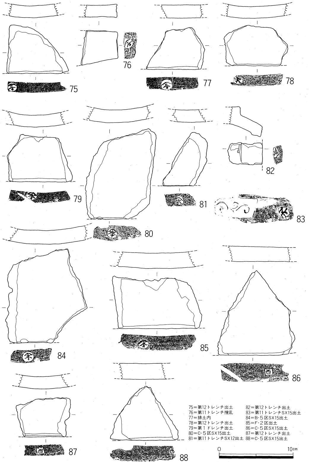
第19図 出土刻印瓦実測図(1)
