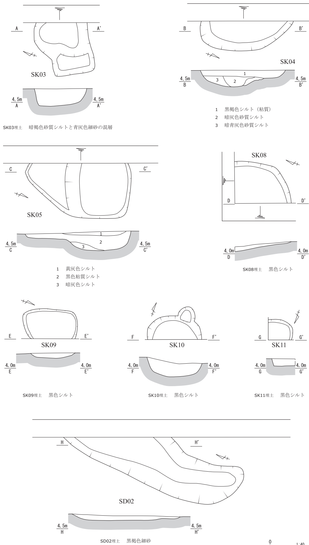
Fig.7 遺構実測図 (1)
