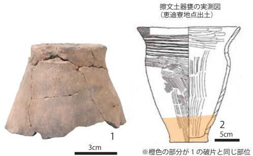
▲ 農学部実験実習棟地点の土器転用支脚（甕の底部片） 第3号竪穴住居址のカマド火床で発見された（擦文中期）。破損した甕の底部を再利用して支脚とした。
