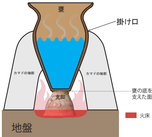
▲恵迪寮地点第1号竪穴住居址で発見された支脚出土状態（模式図）
