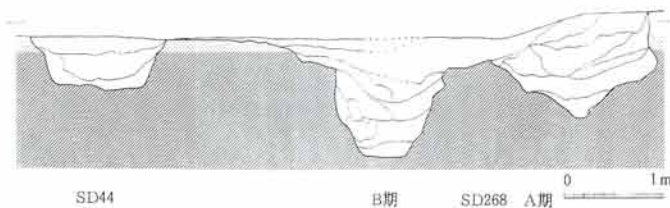
第8図 SD44・268溝跡断面図
