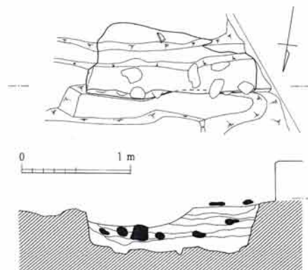
第6図 SB54尼坊跡7-3 礎石掘付掘方断面図
