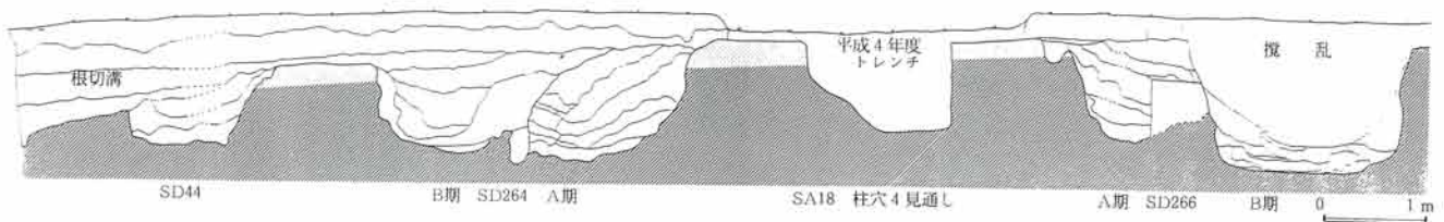
第4図 SD44・264・266溝跡、SA18塀跡断面図
