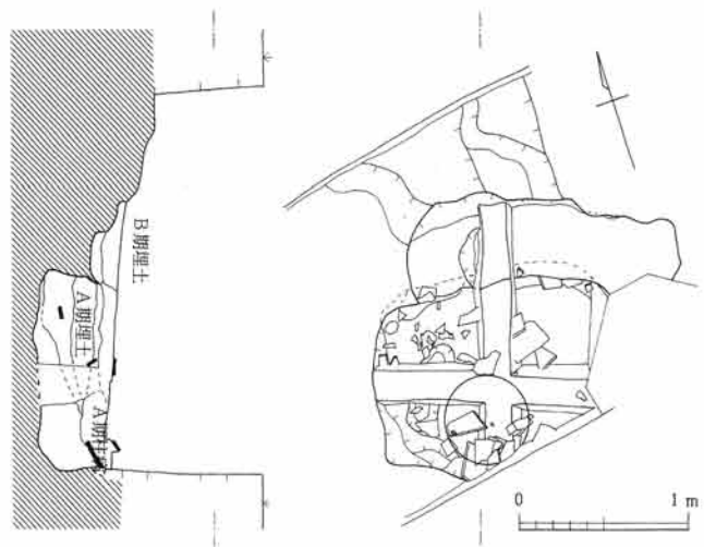
第5図 SX108掘立柱遺構断面図
