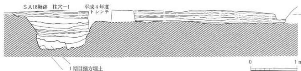
第3図 SB142 推定中門断面図
