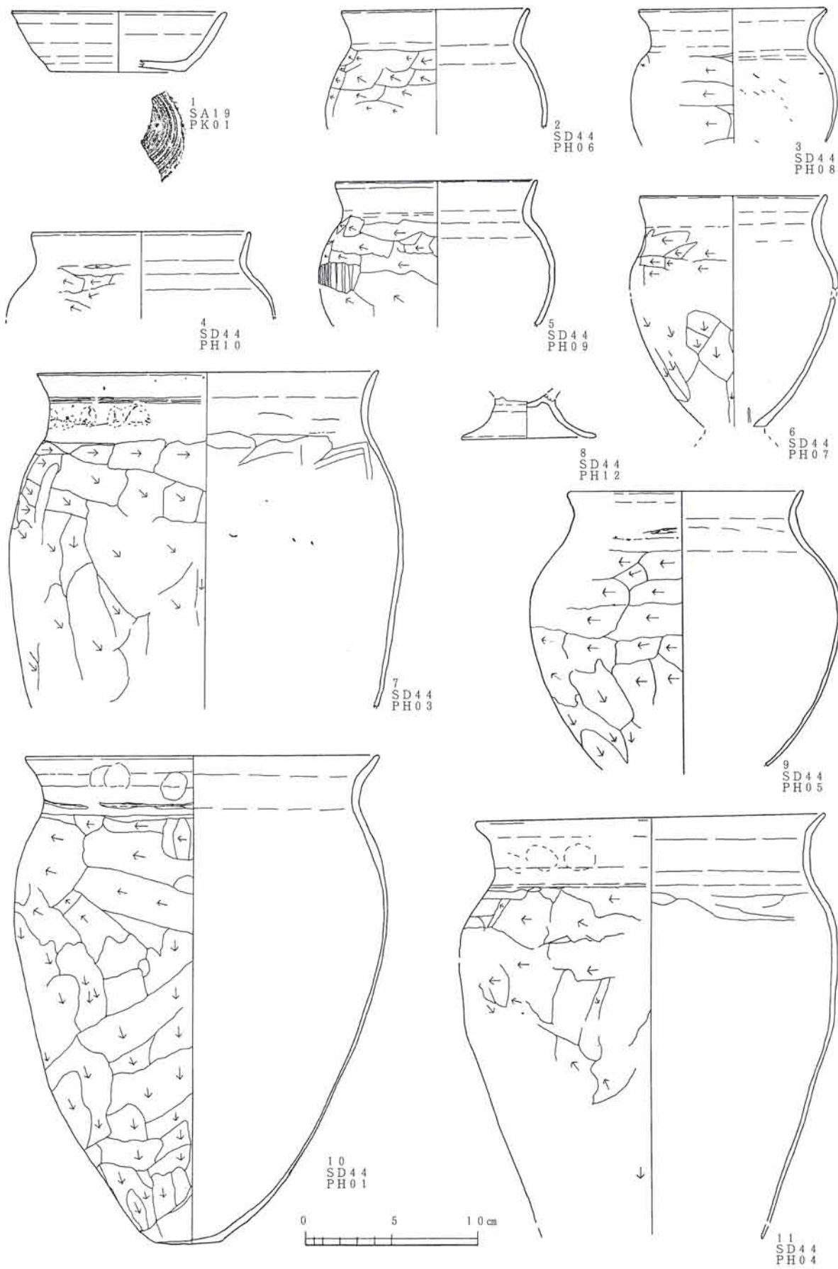
第10图 SA19, SD44 出土土器实测图 (1 : 3)
