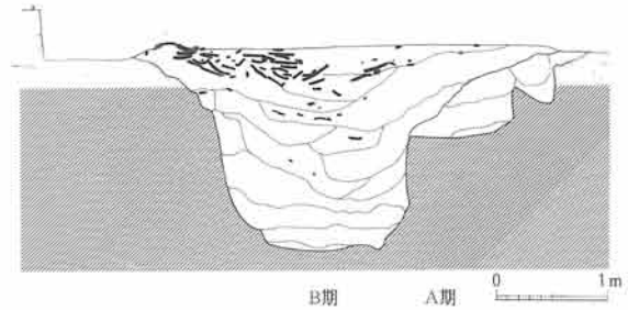
第9図 SD267溝跡断面図
