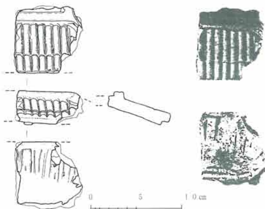
第14図 SD266 出土瓦塔 (1 : 4)
