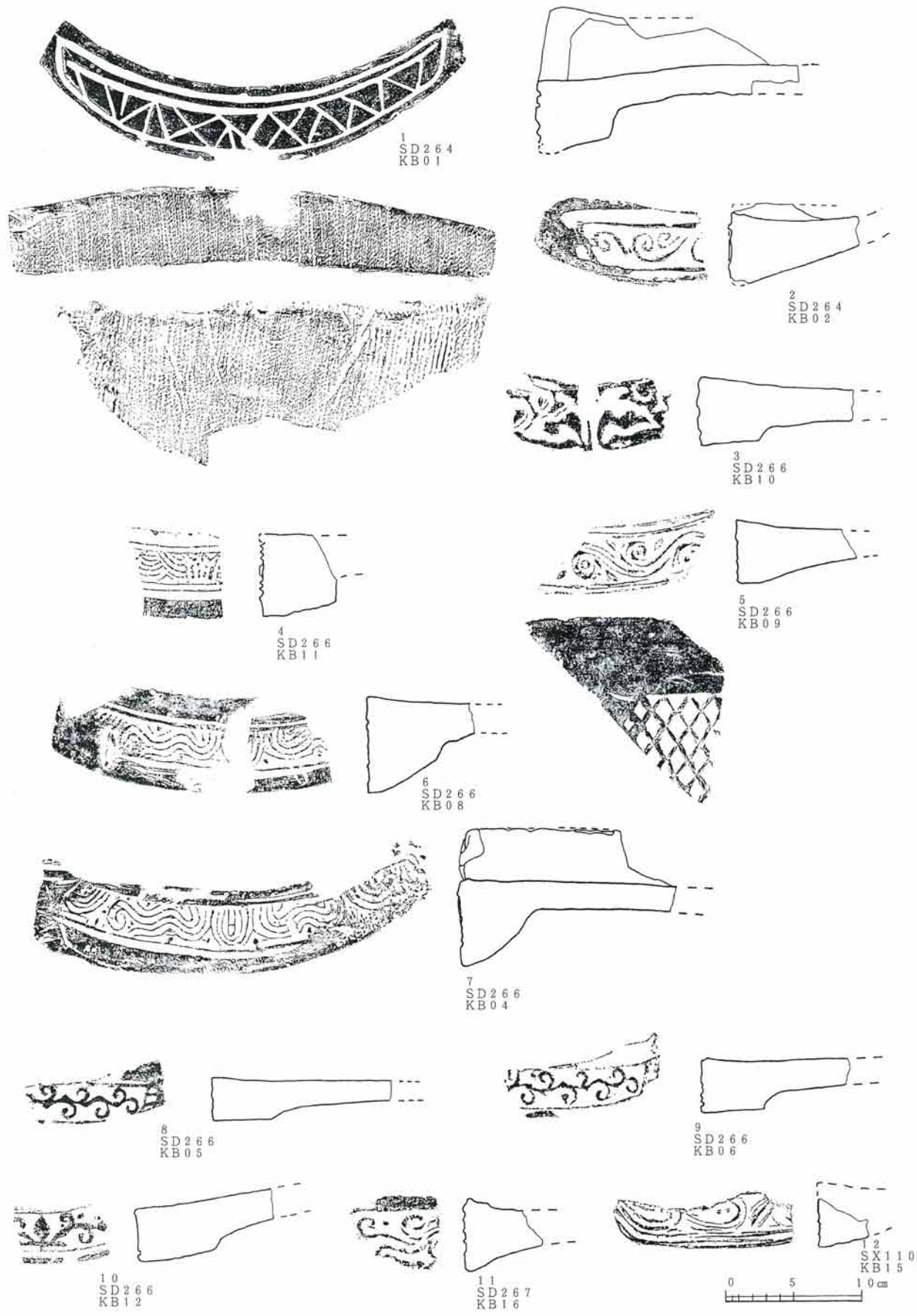
第13图 SD264·266·267. SX110 出土瓦瓦实测图(1:4)
