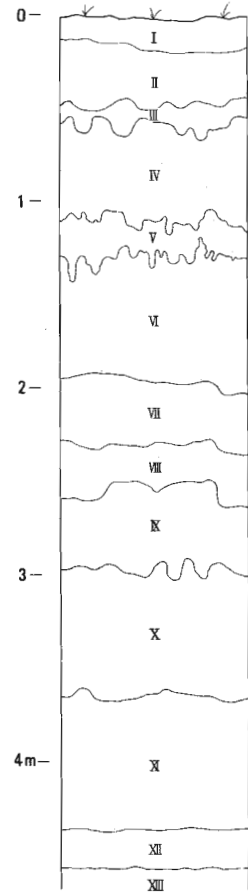
第2図 層序(1/40)
