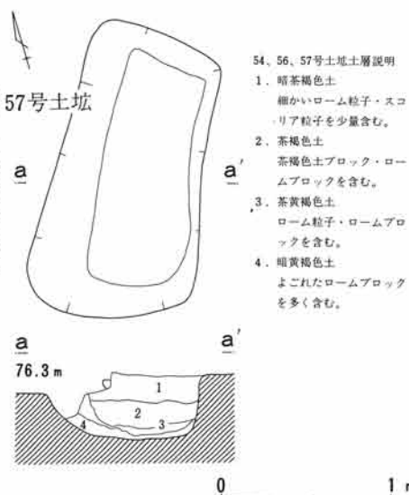
第48図面 55号(勝坂期)52・53・54・56・57号(加曾利E期)土坑
