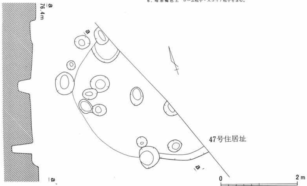
第44図面 46・47号(加曾利E期)住居址
