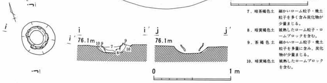
第34図面 34号(加曾利E期)住居址内炉址・埋裏・埋裏炉
