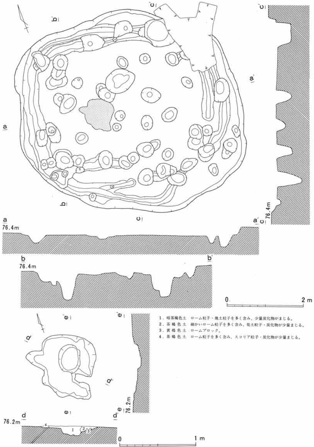
第16図面 37号(勝坂期)住居址・炉址
