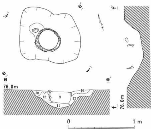
第6図面 27号(勝坂期)住居址・炉址
