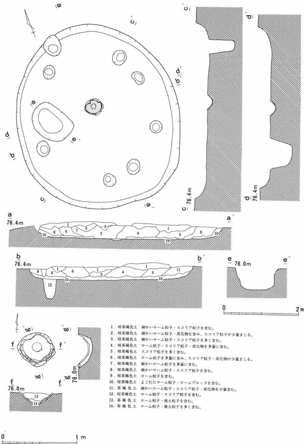
第18図面 42号(勝坂期)住居址・炉址・住内土坑
