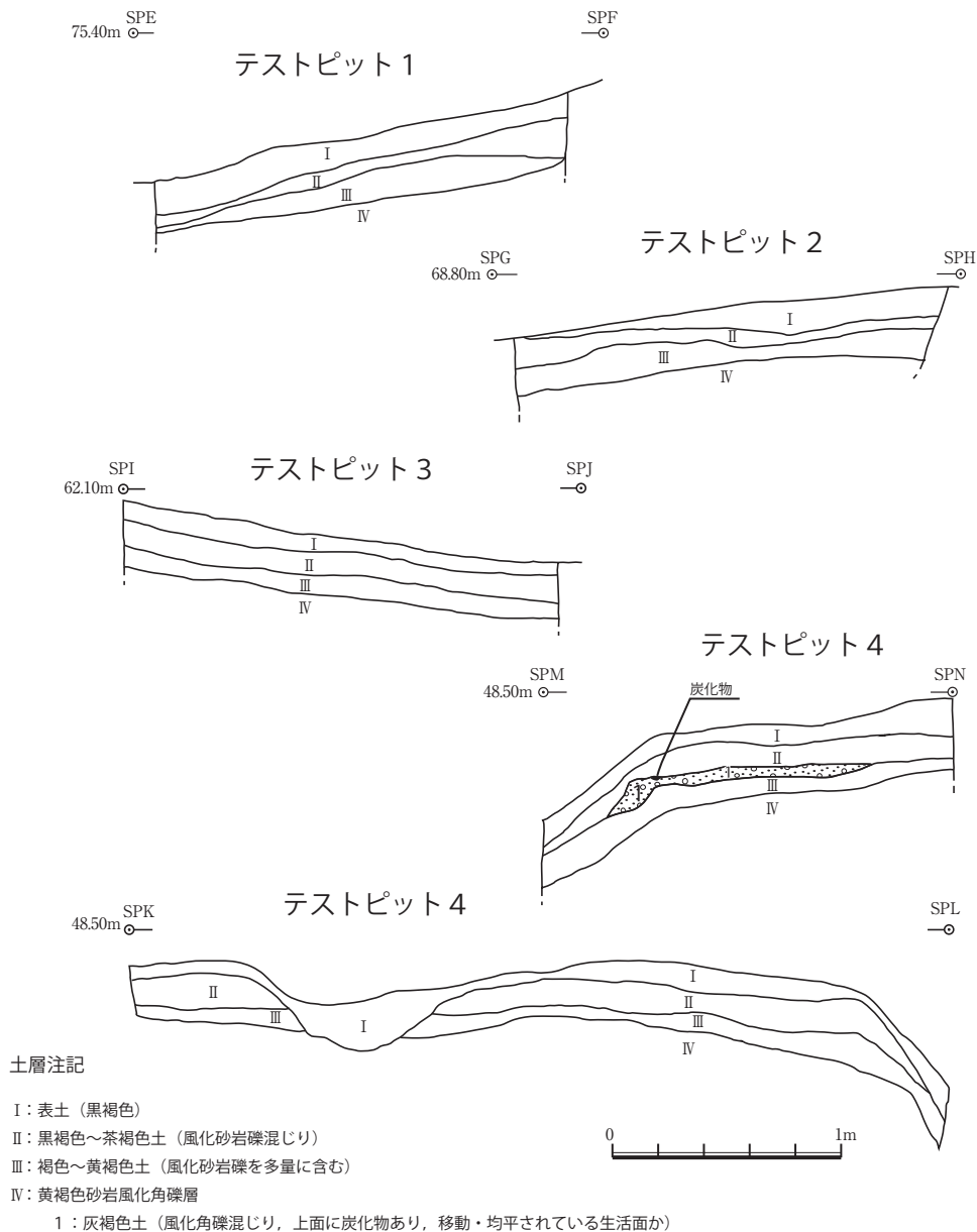
図6：テストピット断面図
