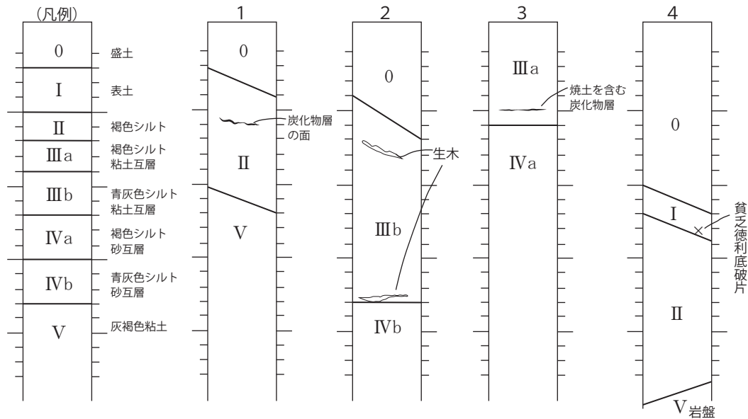
図 12：安部志内川右岸遺跡土層図
