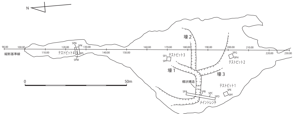
図3；試掘位置と壕
