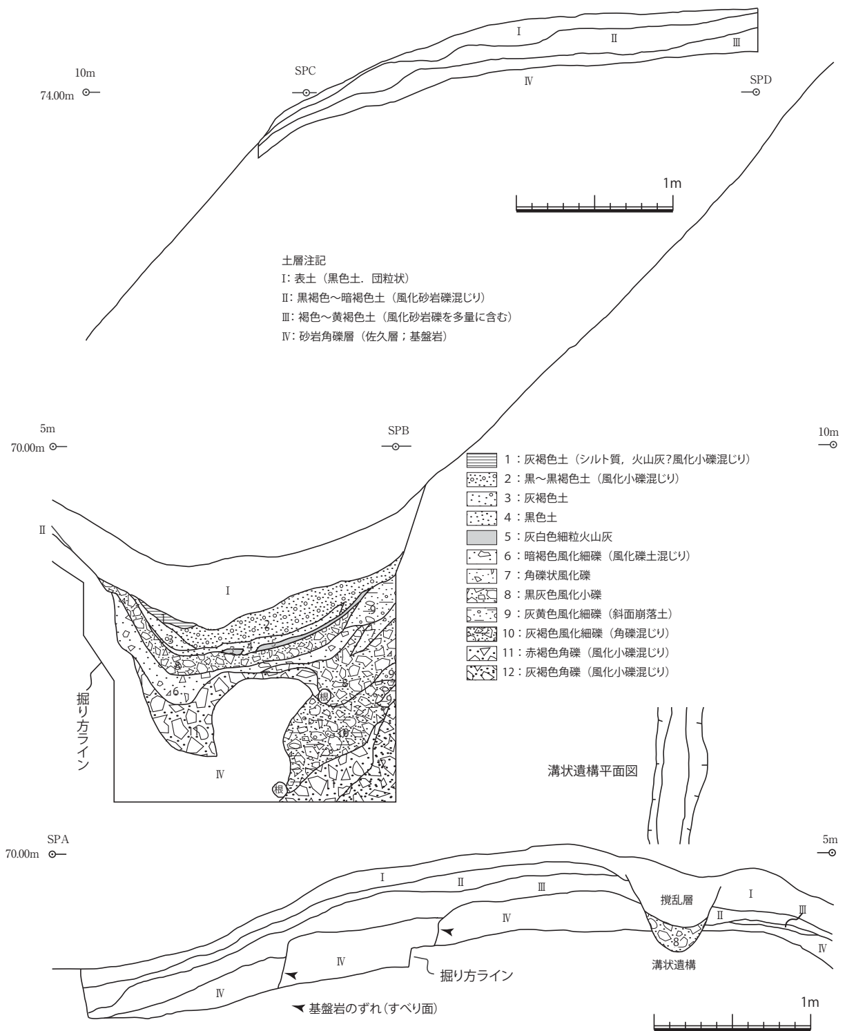
図5：メイトレンチ断面図
