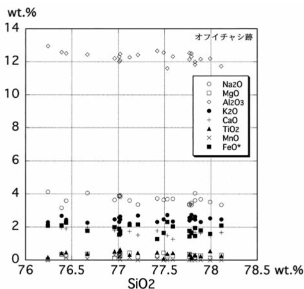
図7：火山ガラスの化学組成値分布
