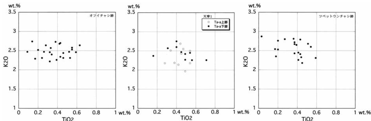
図8:火山ガラスの TiO 2 -K 2 O 分布(オフイチャシ跡テフラ,天寧1 Ta-a テフラ,ツベットウンチャシ跡 Ta-a テフラ)
