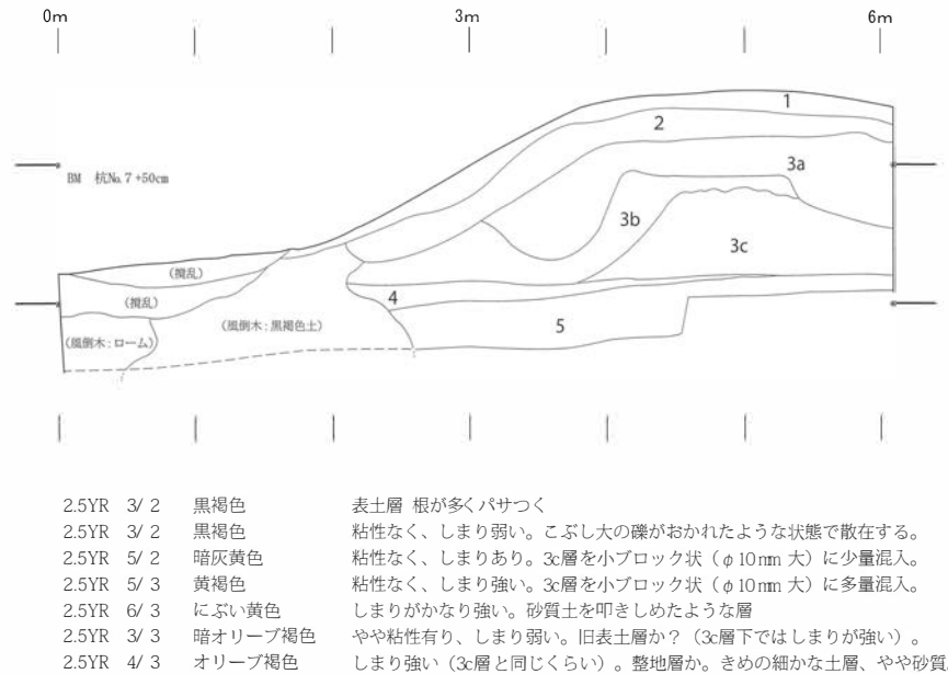
図 28 40 T 土手状遺構土層断面図
