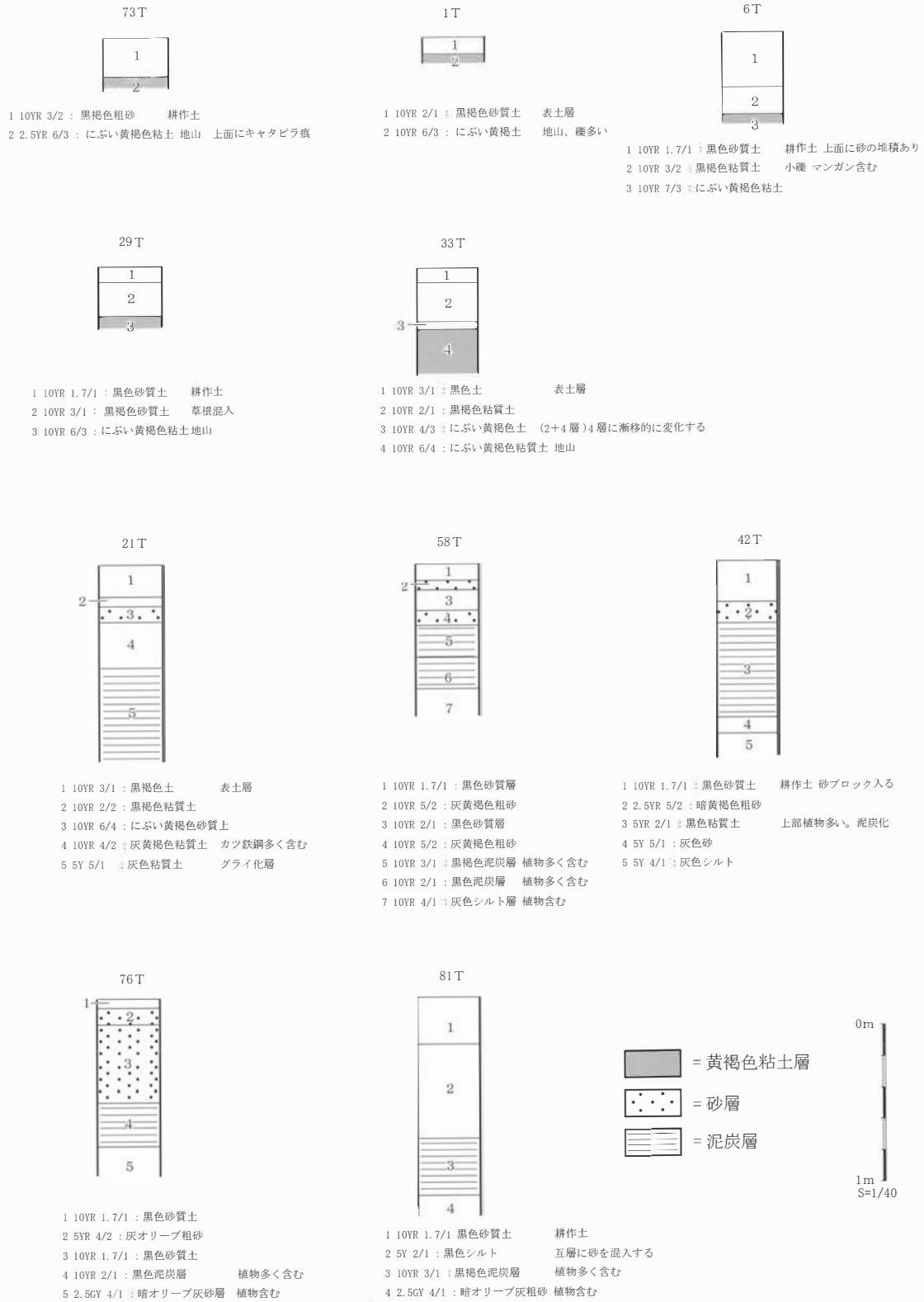
図 68 萱浜・下渋佐地区試掘調査柱状図
