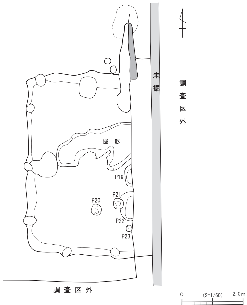
図10 1号住居跡掘形実測図
