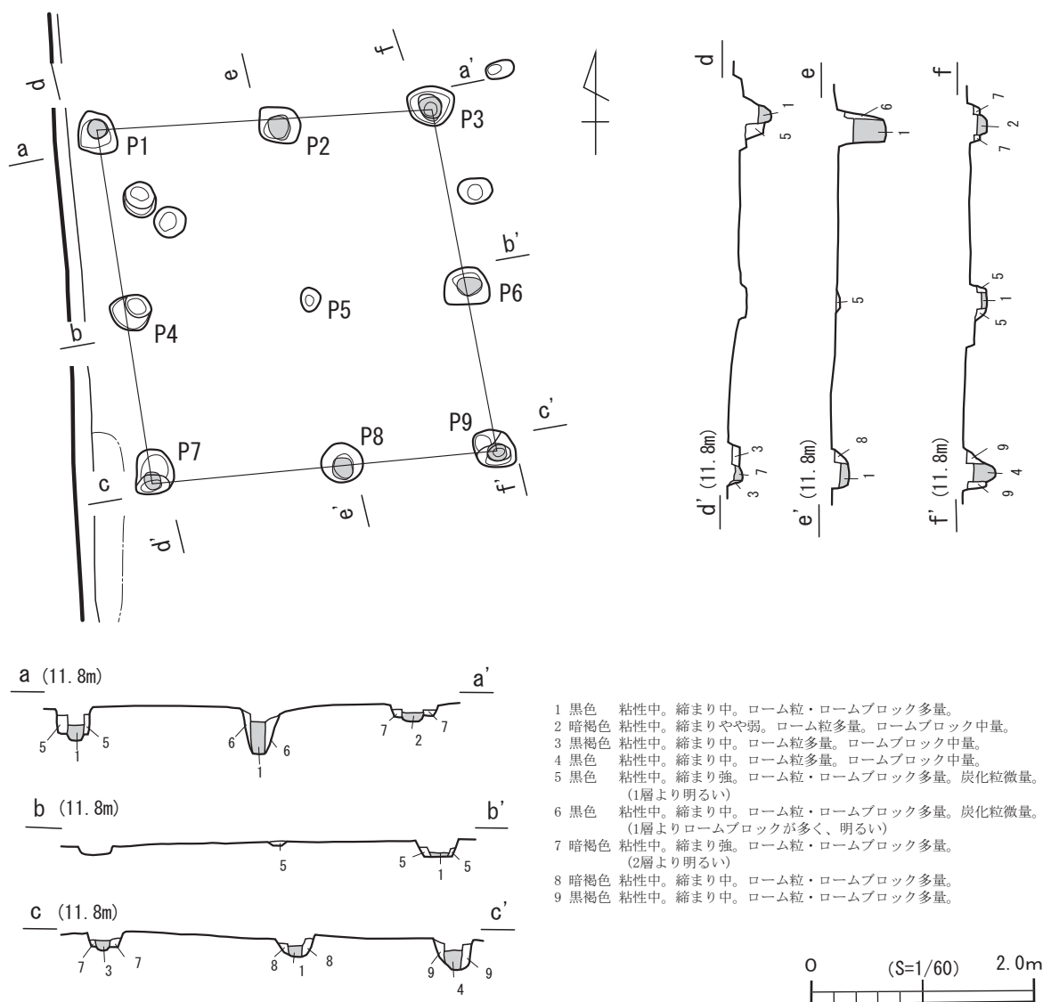
図20 1号掘立柱建物跡実測図
