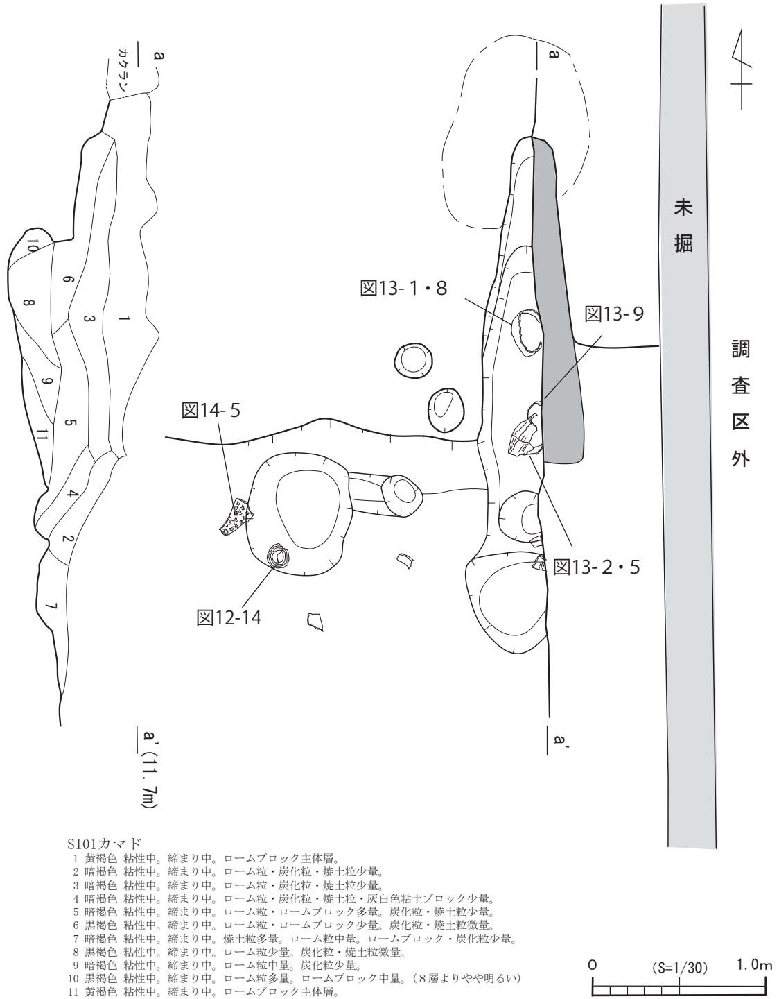
図 11 1号住居跡カマド実測図
