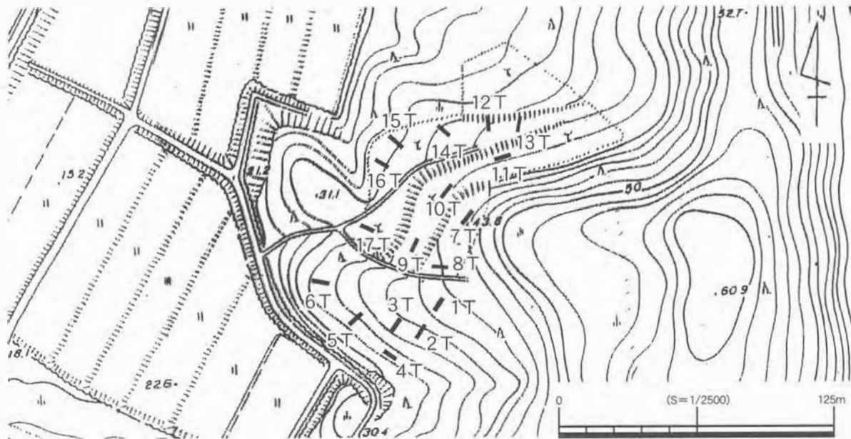
図30 トレンチ配置図
