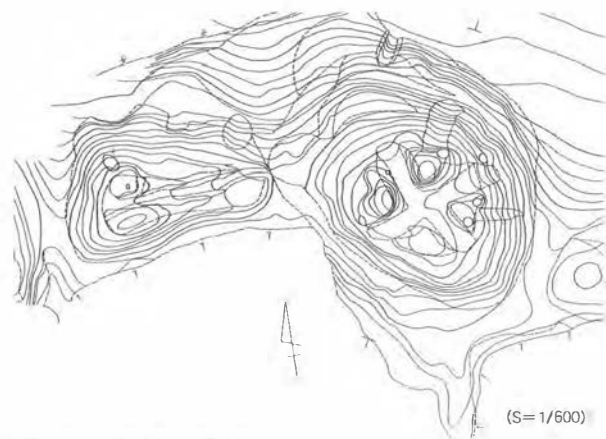
図41 1号墳測量図
