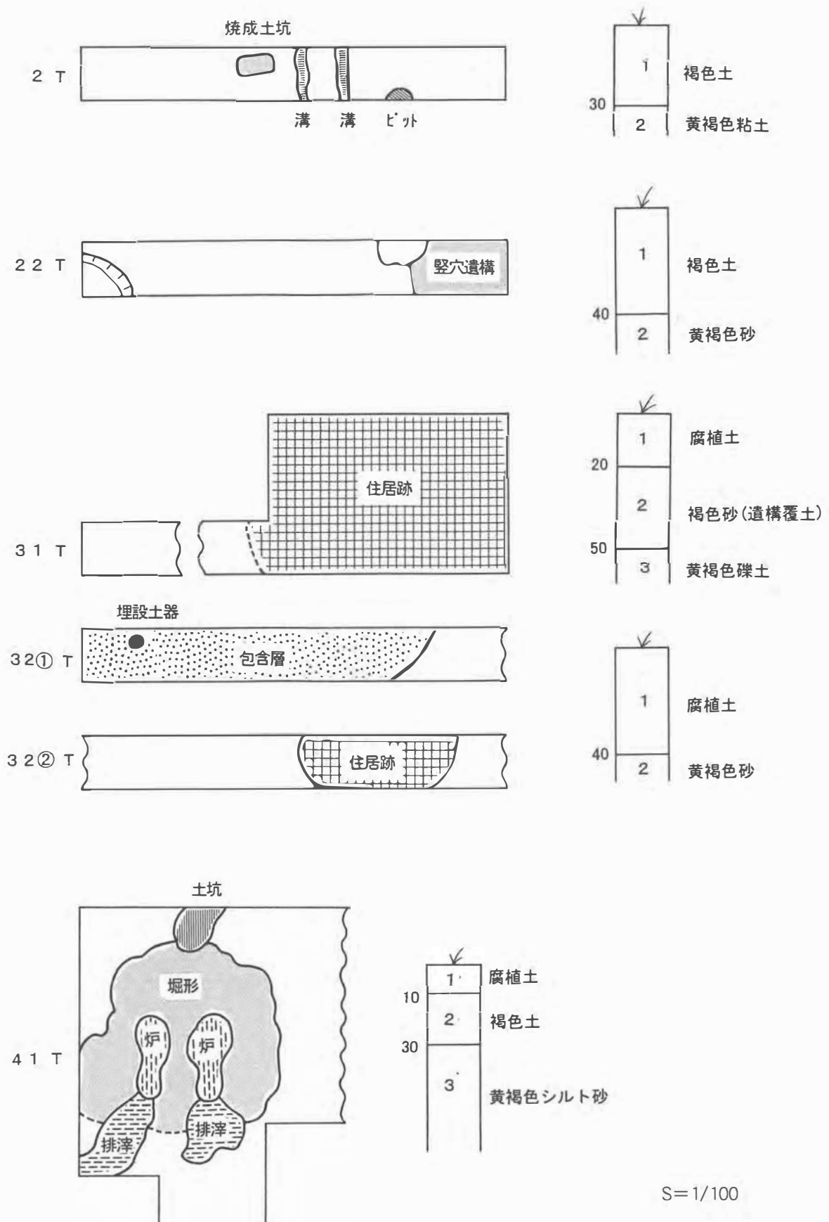
図26 検出遺構平面図 (1)
