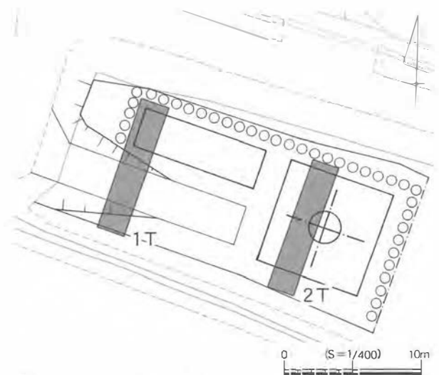
図21 トレンチ配置図
