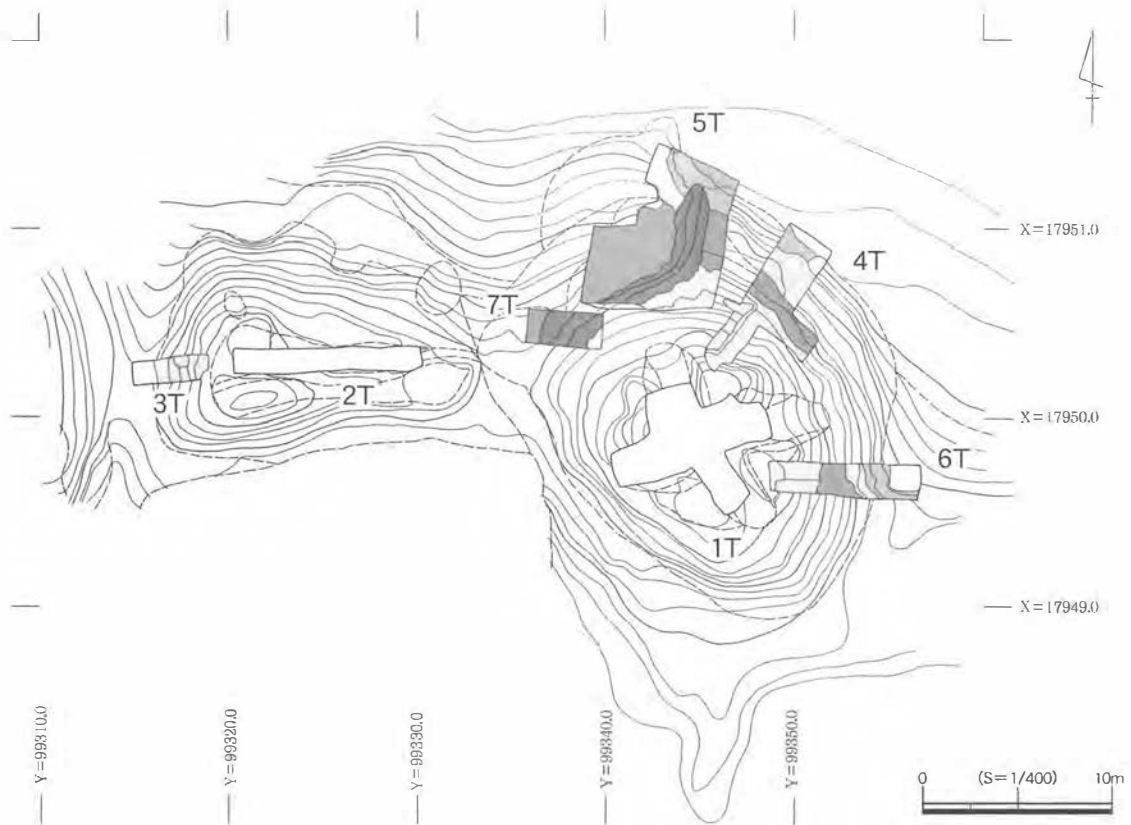
図48 1号墳全体図
