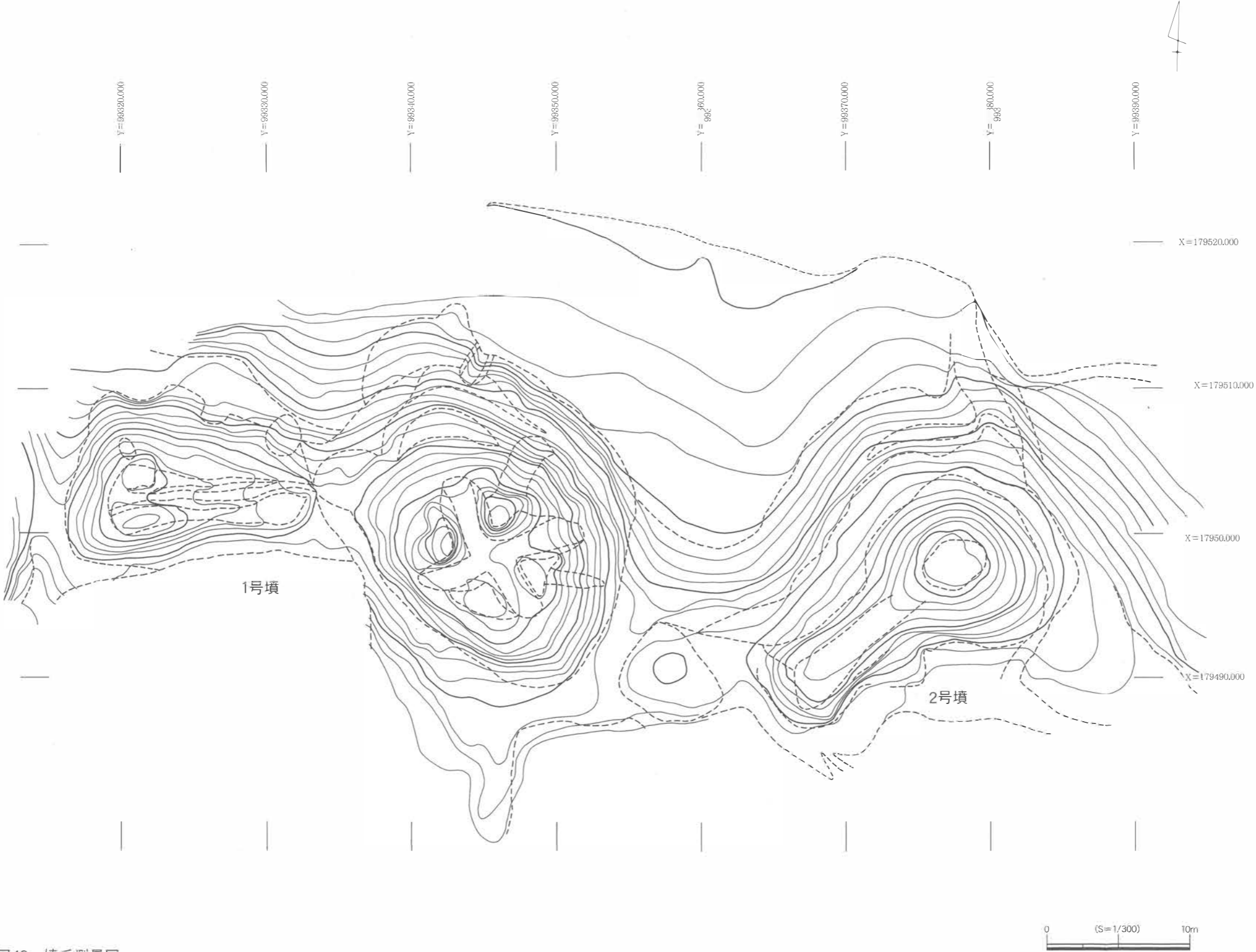
図40 墳丘測量図
