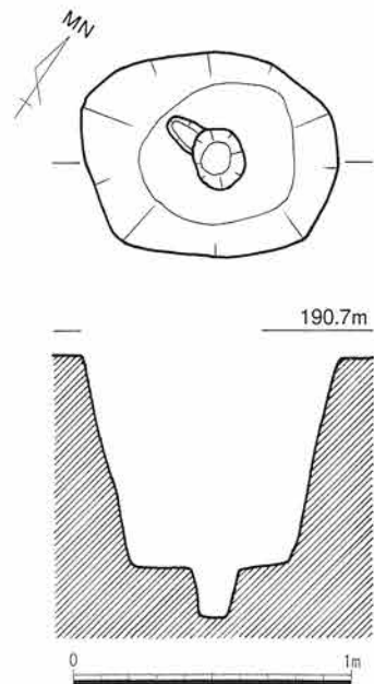
第8図 土壇 (1/30)
