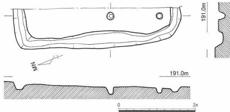
第5図 竪穴住居1(1/60)
