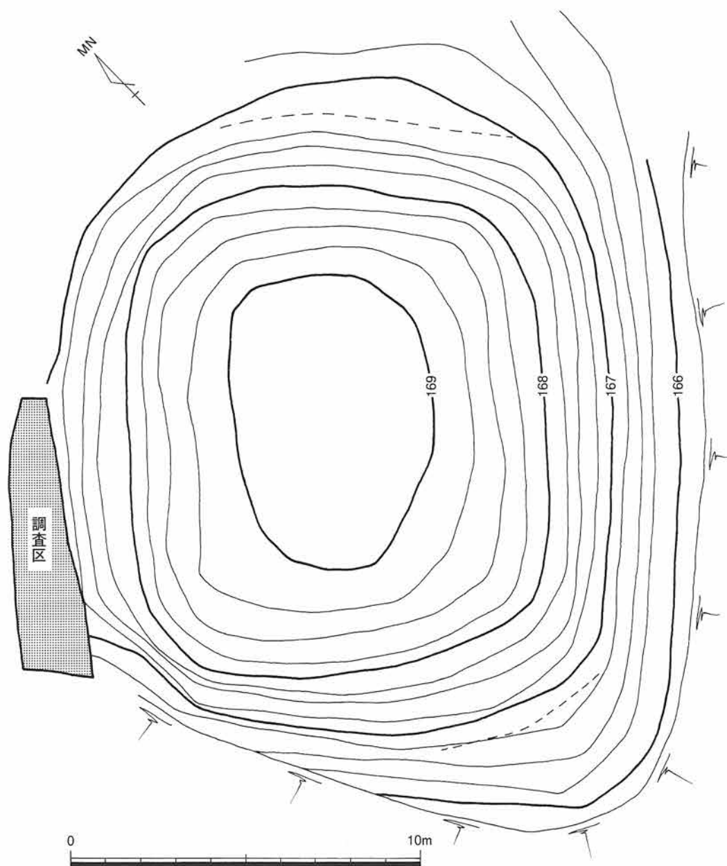
第10図 墳丘測量図 (1/150)
