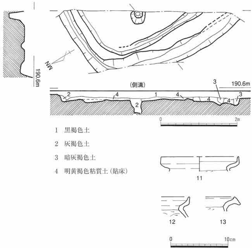
第7図 竪穴住居 3 (1/60) ・出土遺物 (1/4)
