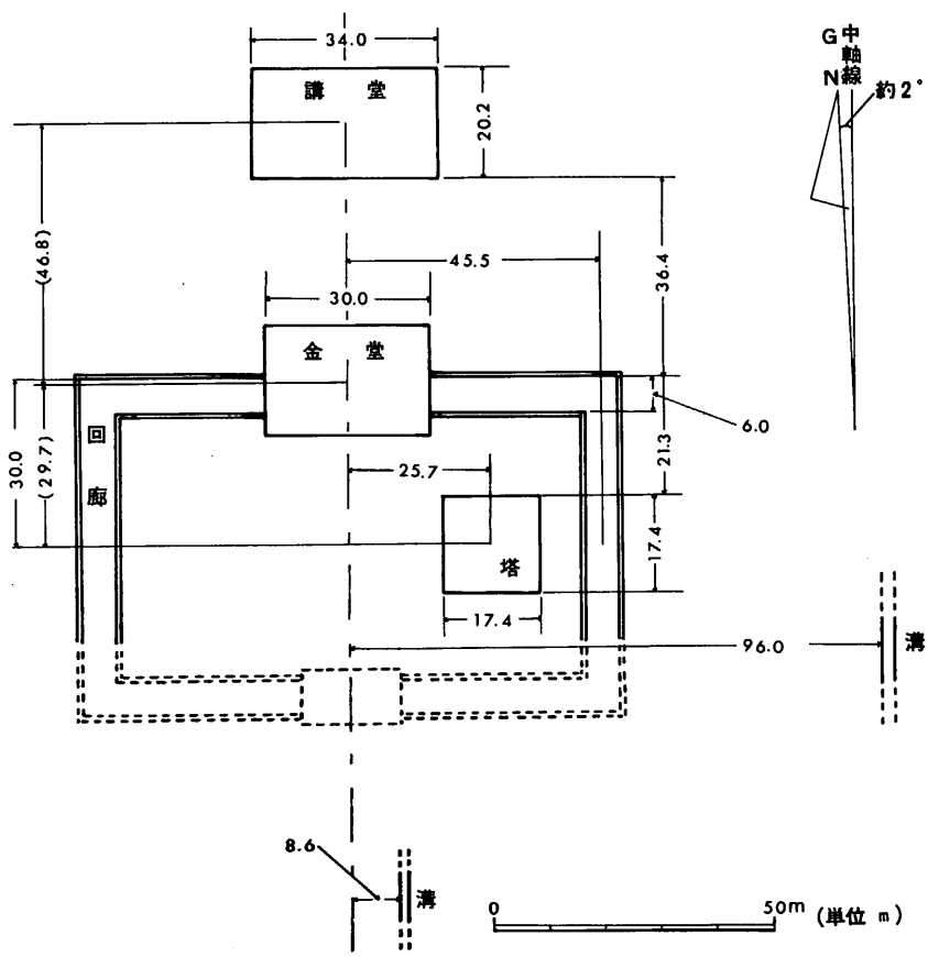
第 26 圖 主要遺構配置圖
