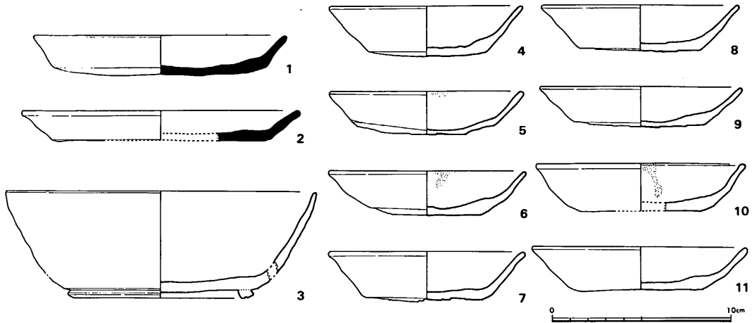
第14図 SC080・SK081・茶色土層出土土器実測図
