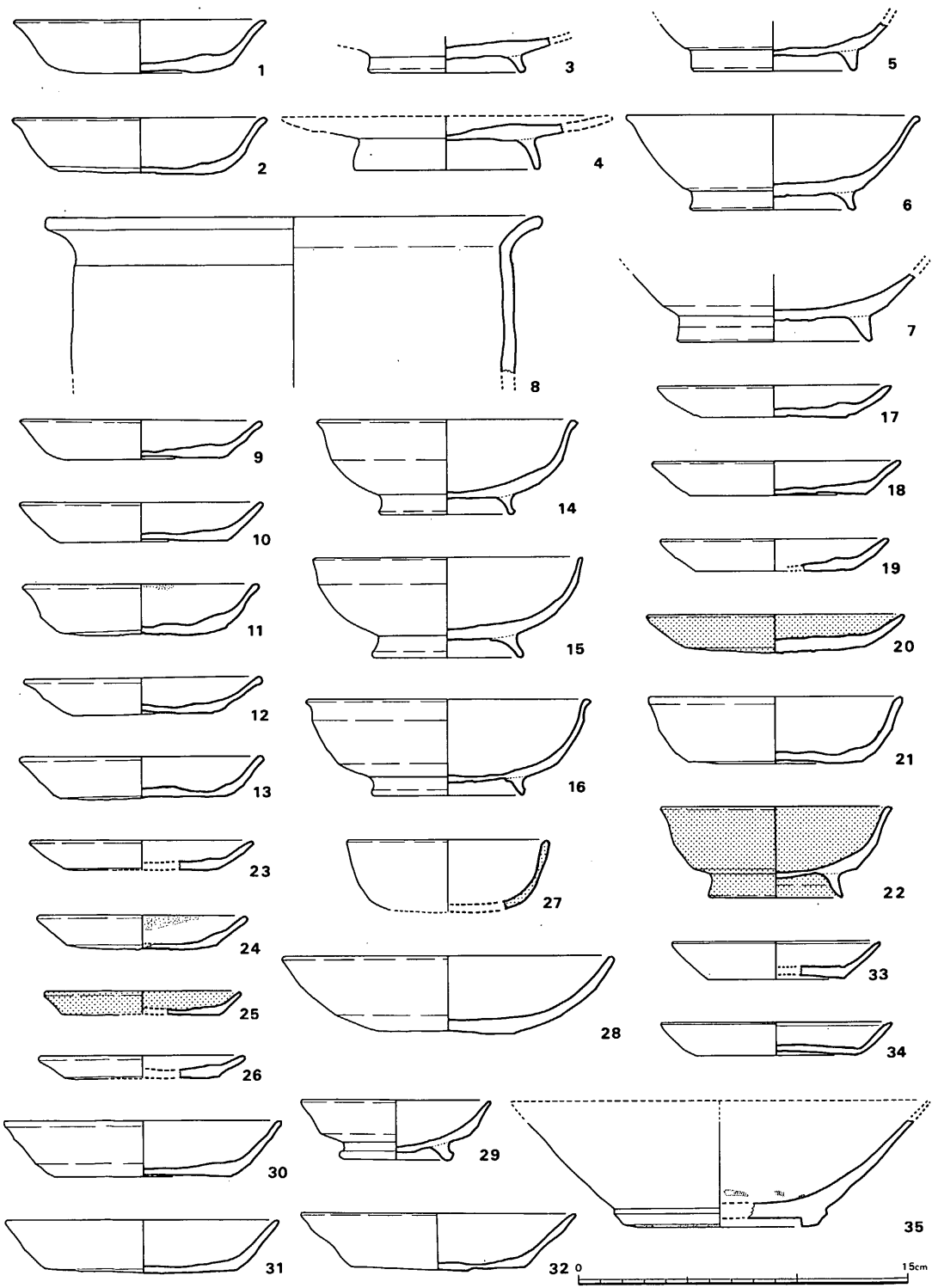
第12図 その他の遺構出土土器実測図
