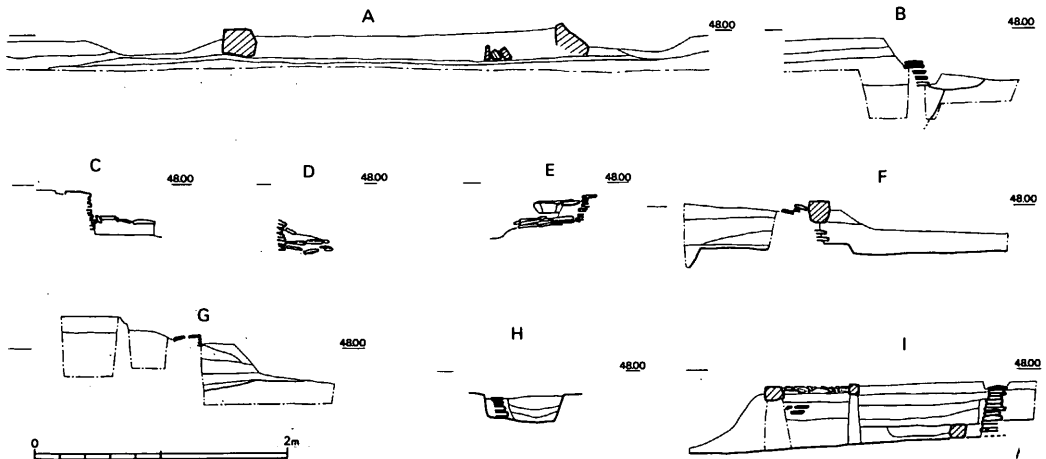
第6図 SB060 土層図
