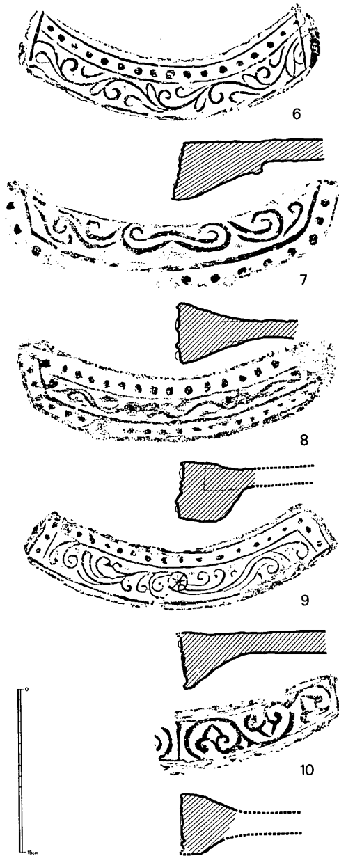
第20図 軒平瓦拓影・実測図
