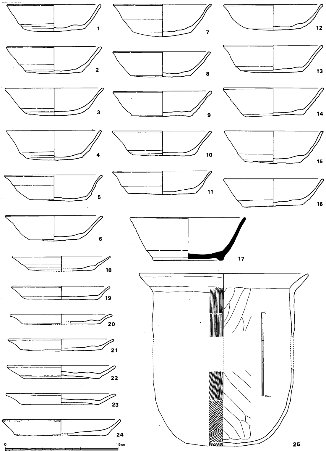
第11図 SK053出土土器実測図
