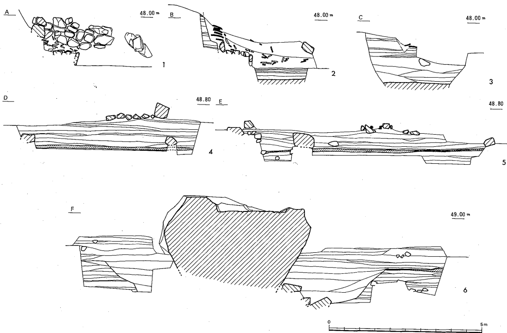
第2図 遺構断面図
