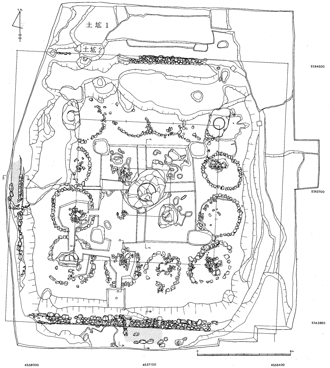
第3図 遺構実測図（座標一国土調査法第Ⅱ座標系）
