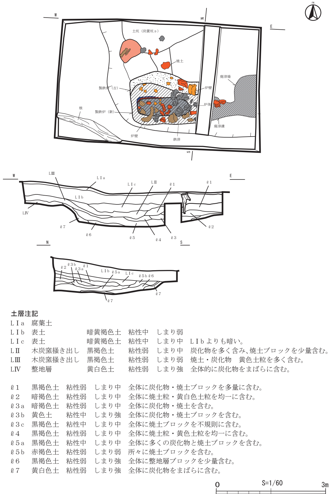
図 12 1 T 製鉄炉跡検出状況
