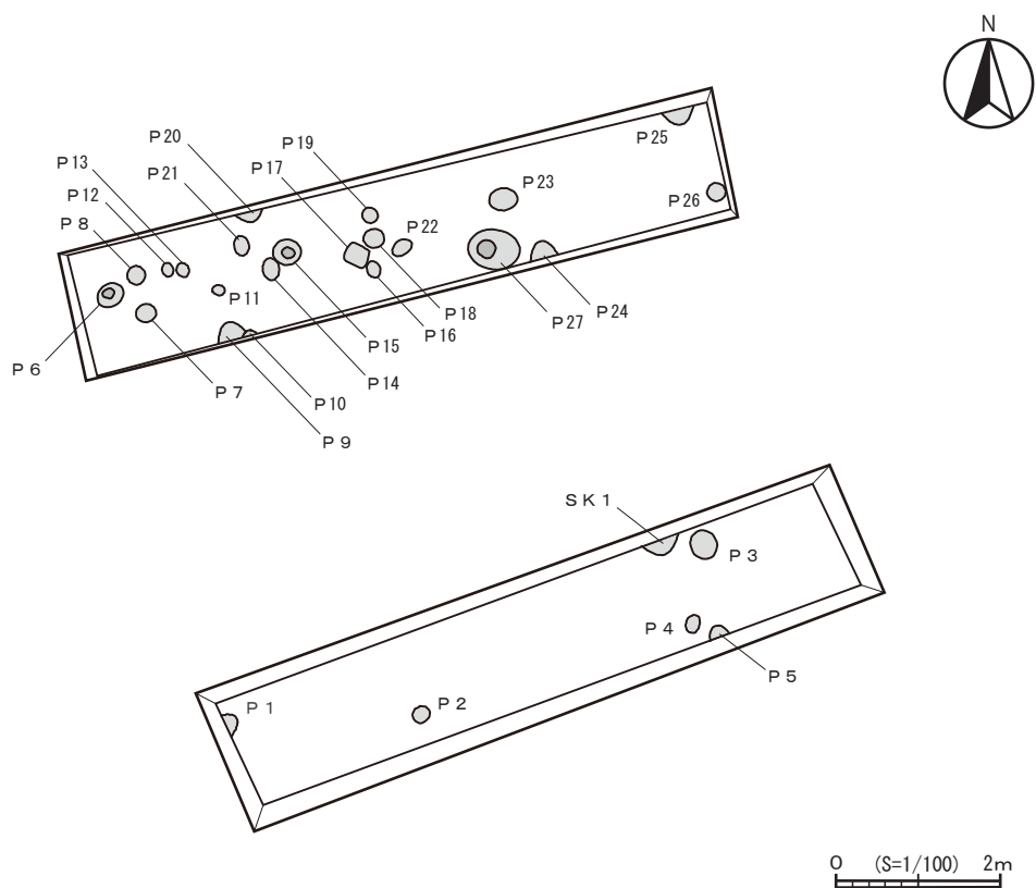
図 46 調査区平面図
