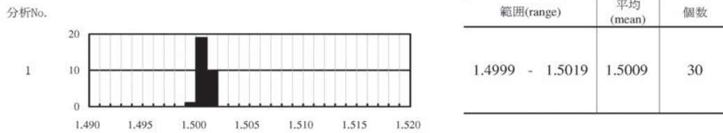
図54 火山ガラスの屈折率測定結果
