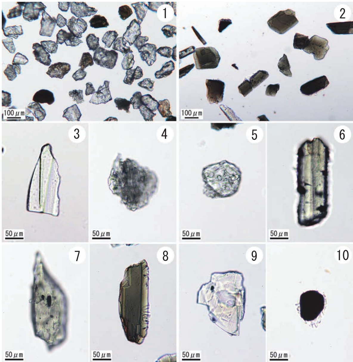
写真155 テフラ試料中の粒子の顕微鏡写真
