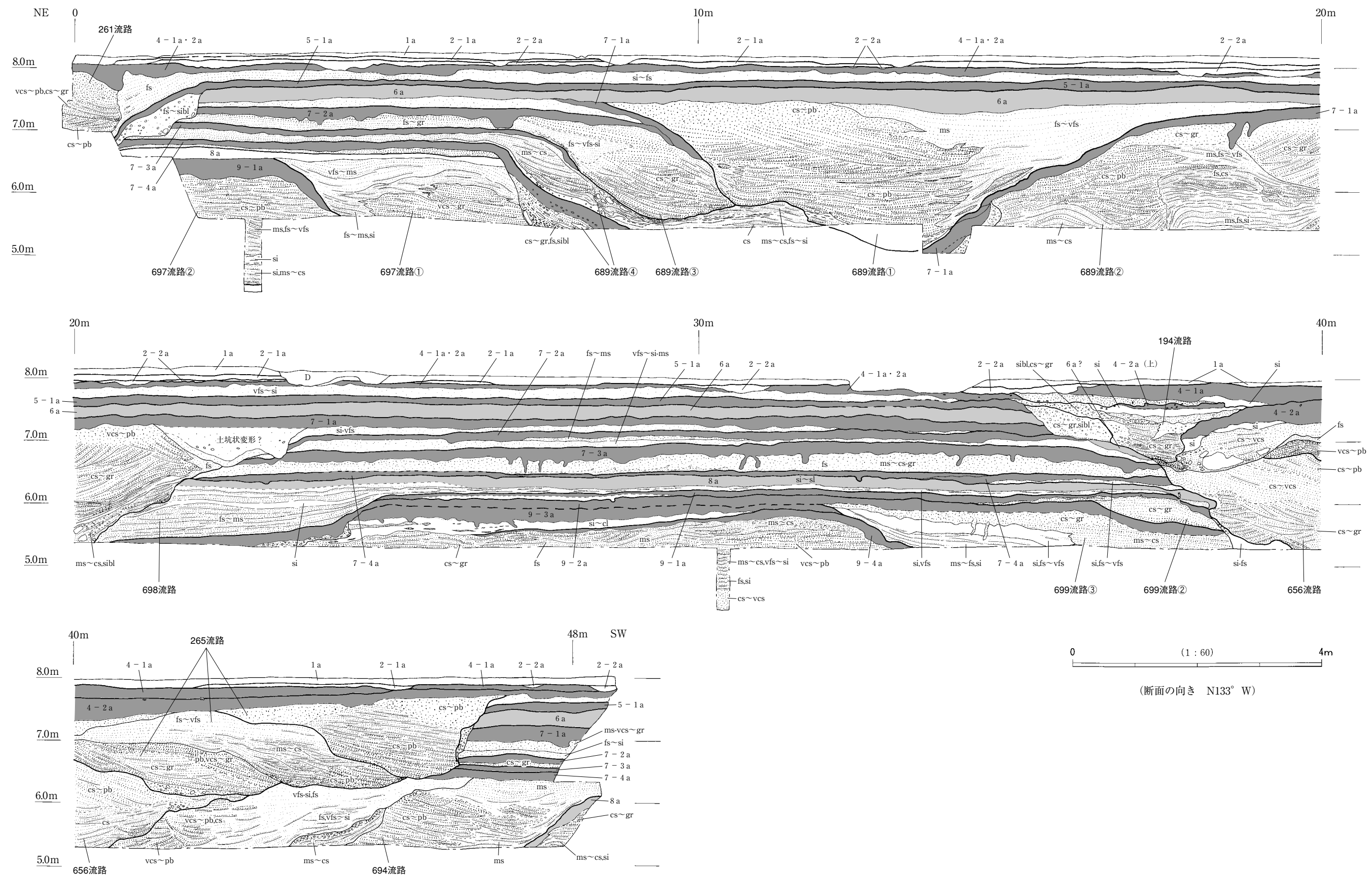
図169 1区(南侧)断面図
