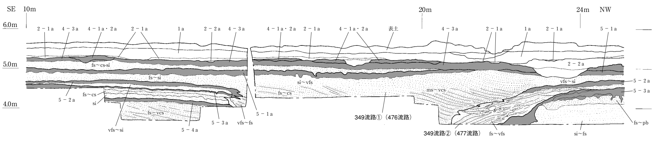
図176 9-a区・9-b区断面図
