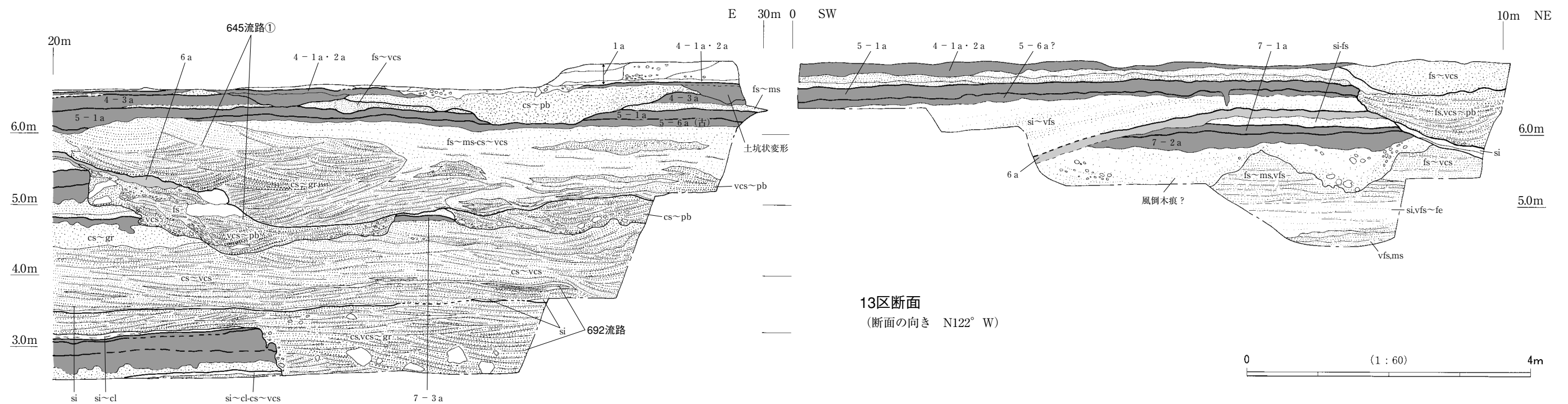
図177 11・14区・13区断面図
