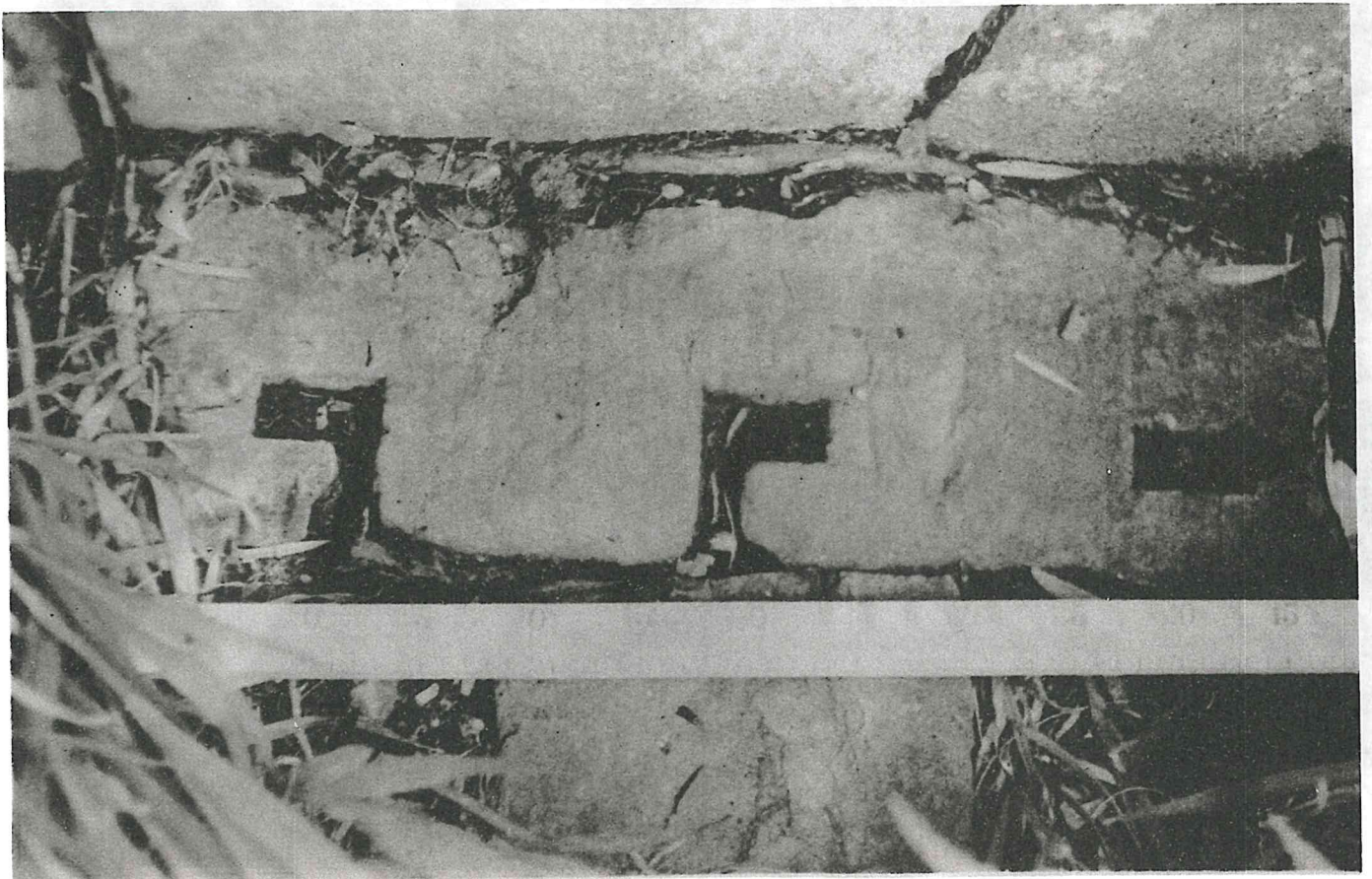
图版 22 中庭内門跡(上)内門敷石(下) 183 神宮
