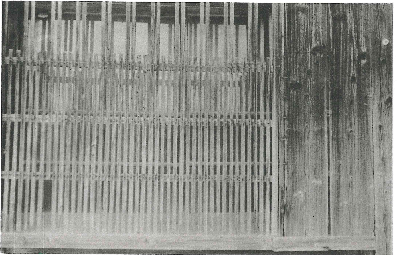
図版 13 文書部屋 外部格子(上) 格子近景(下)
