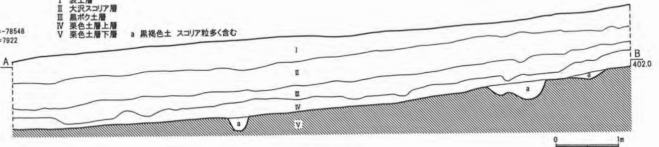
第10図 2トレンチ実測図
