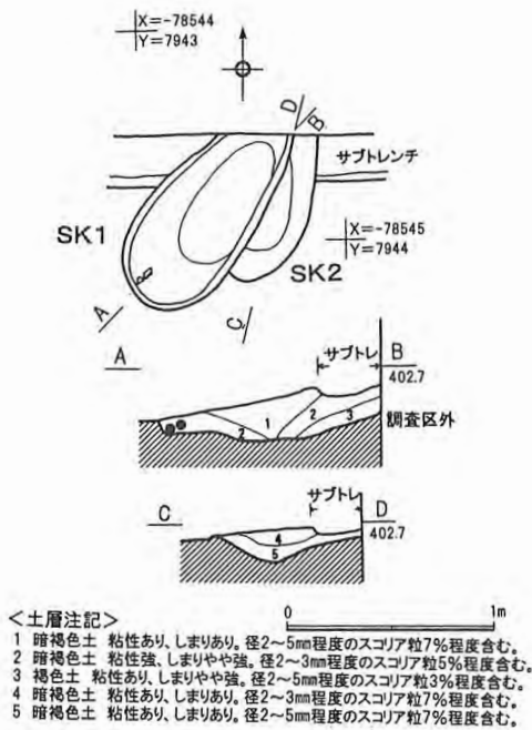
第12図 SK1・SK2実測図
