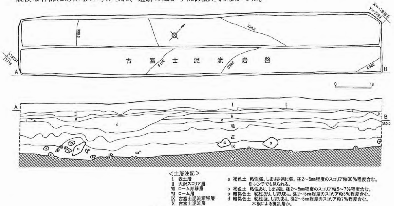
第22図 9トレンチ実測図
