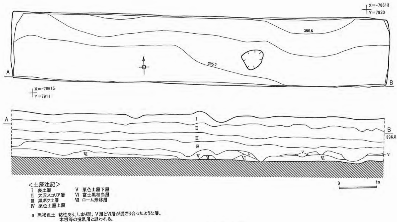
第14図 5 トレンチ実測図
