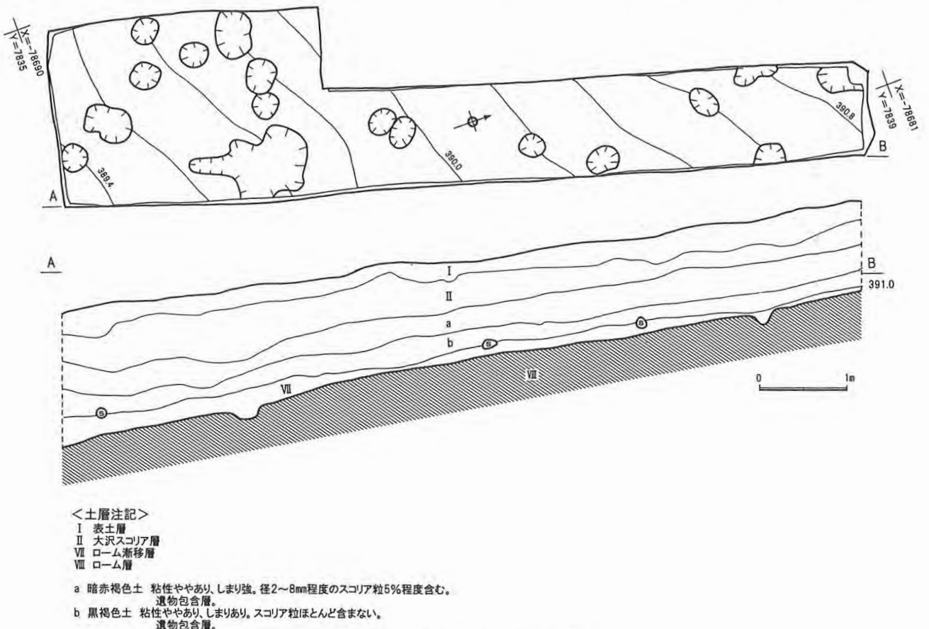
第19図 7トレンチ実測図
