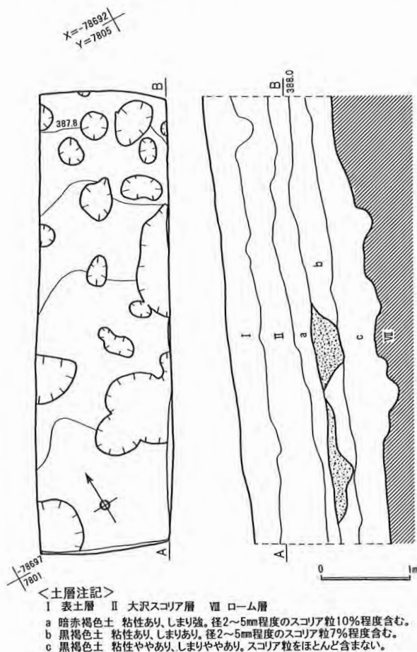
第21図 8トレンチ実測図
