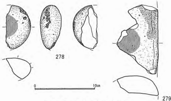
第37図 出土石器実測図②
