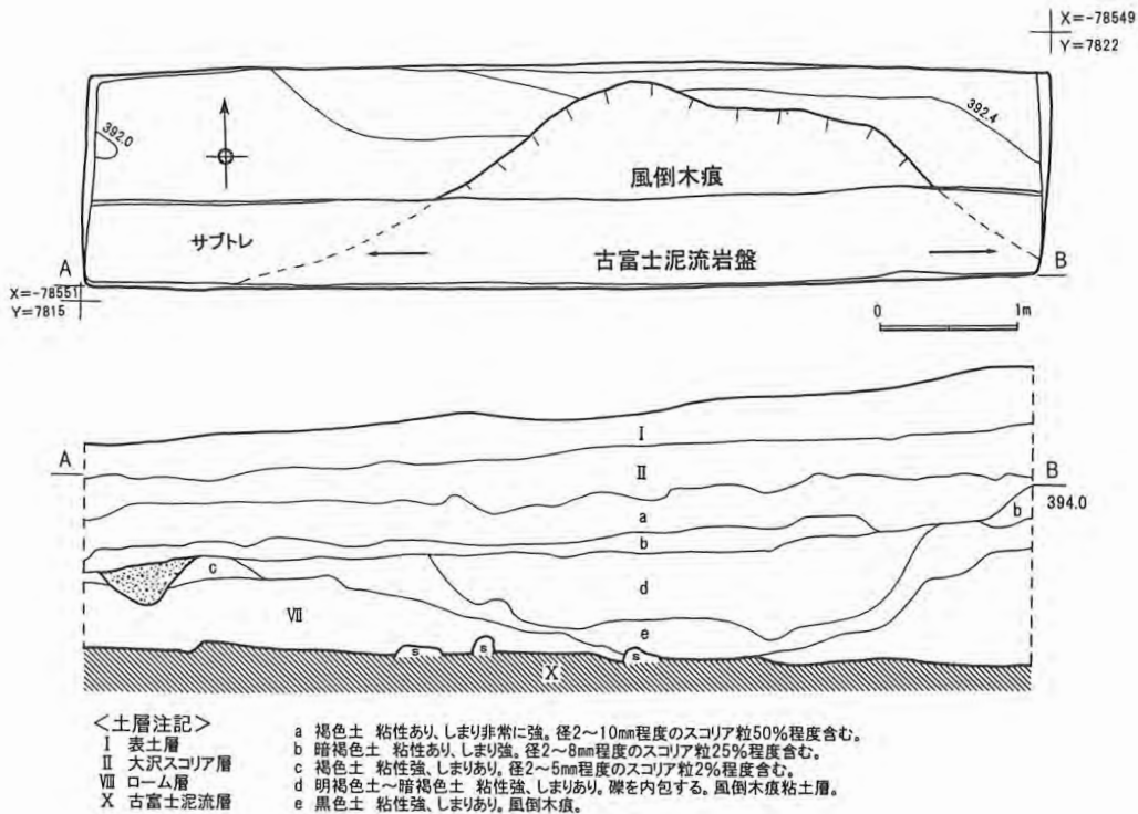
第23図 10トレンチ実測図
