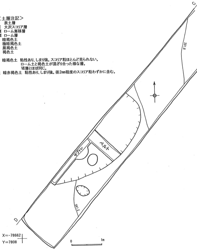
第16図 6トレンチ実測図②
