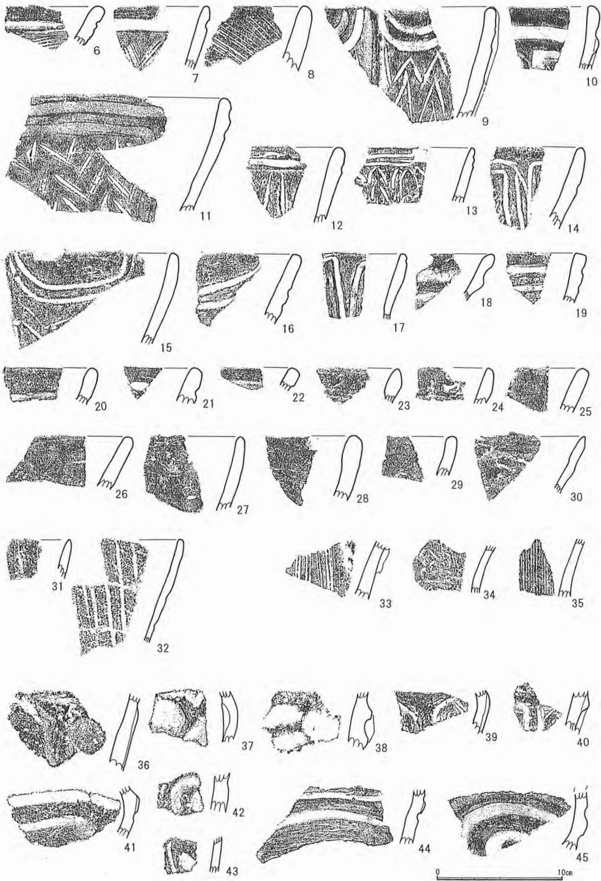
第25図 6トレンチ出土土器実測図①
