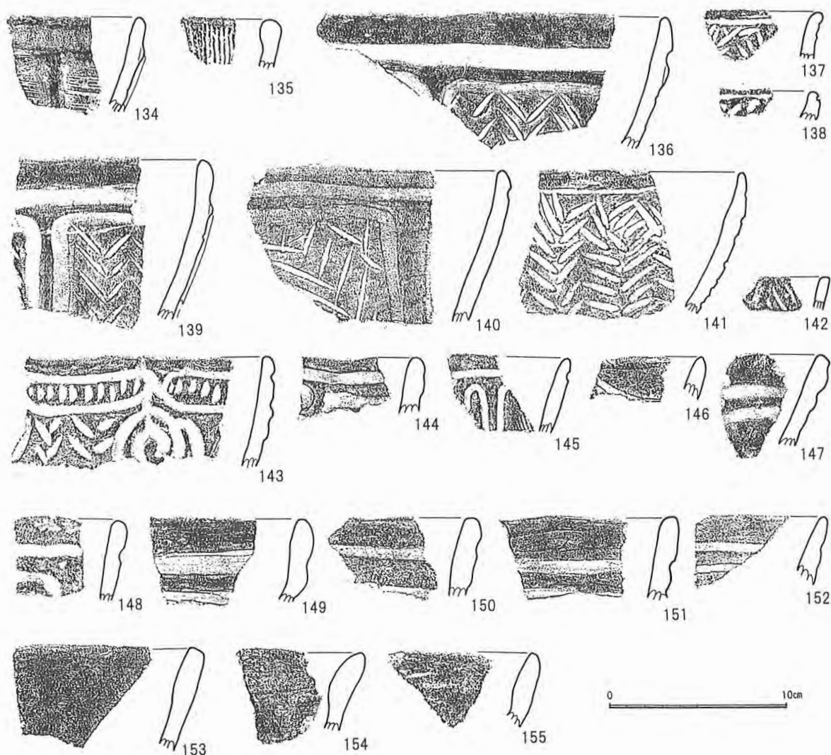
第30図 7トレンチ出土土器実測図①
