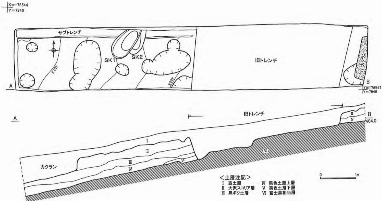
第11図 3トレンチ実測図
