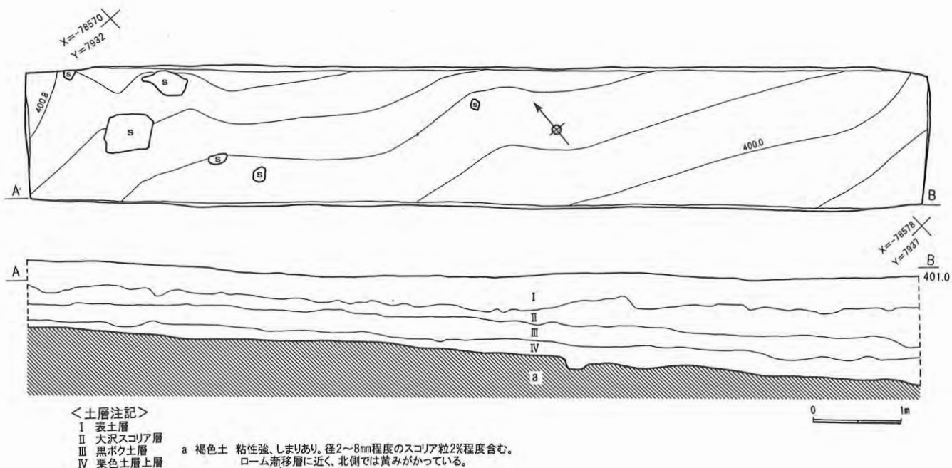
第13図 4 トレンチ実測図
