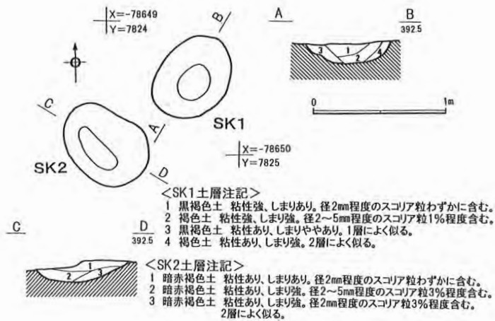
第18図 6トレンチSK1・SK2実測図
