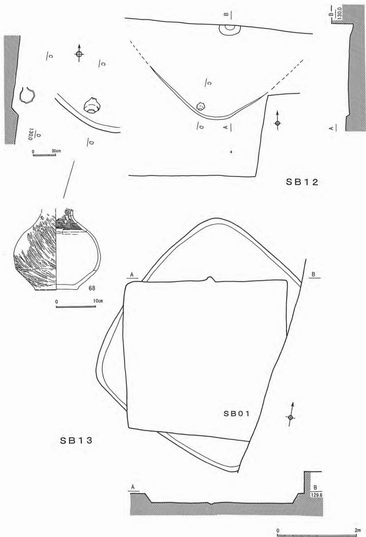
第20図 SB12・SB13 実測図
