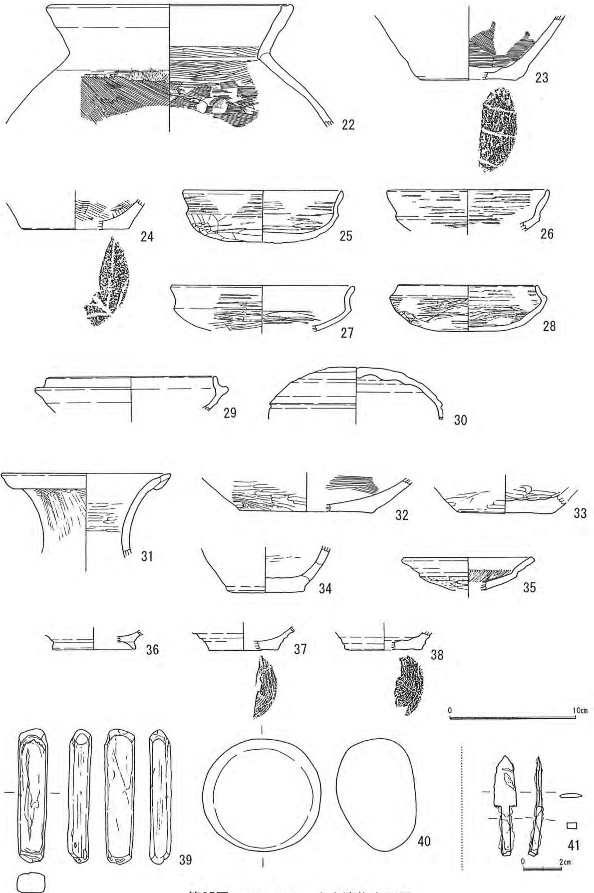
第25图 SB02 出土遺物実測图
