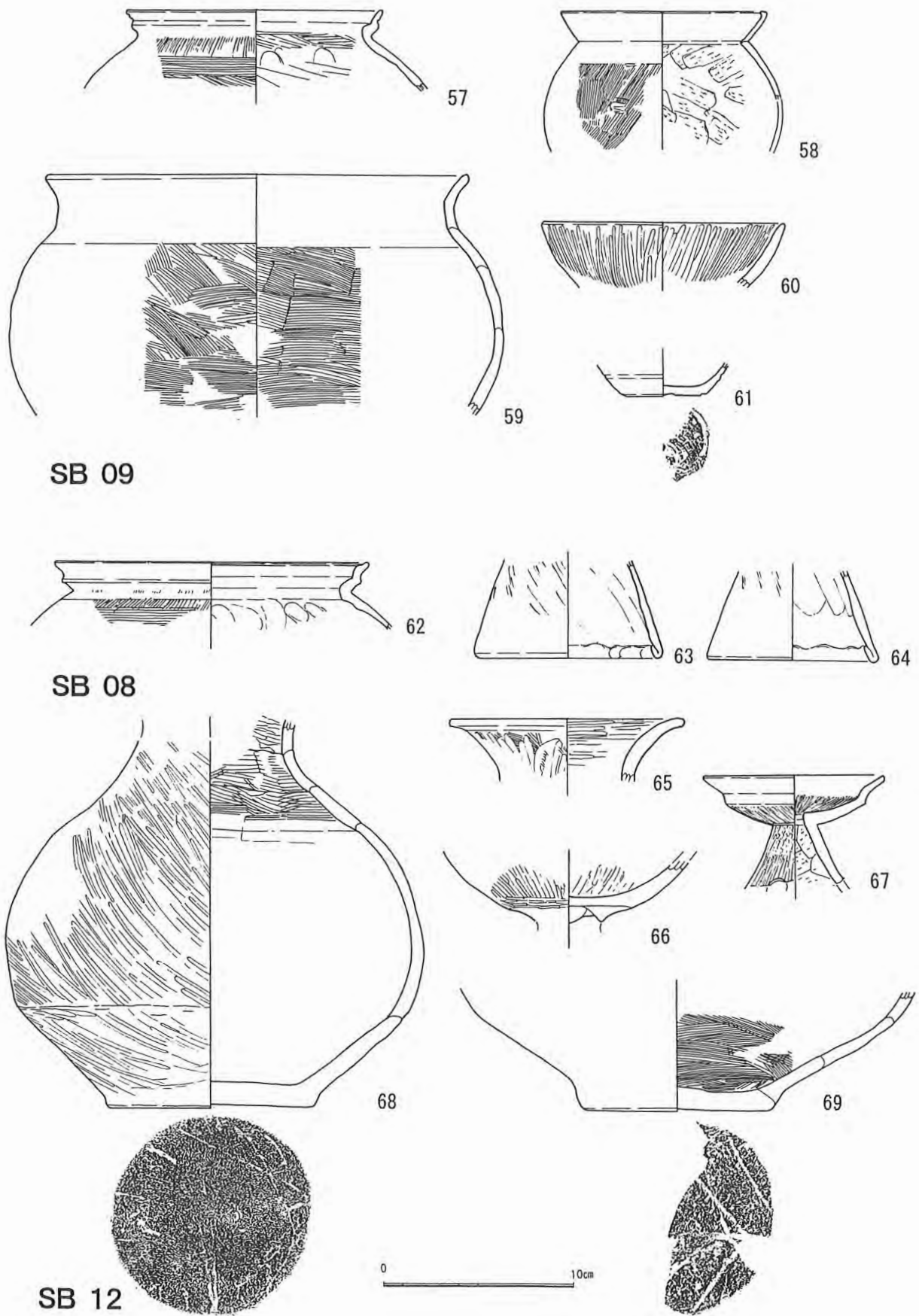
第27图 竖穴住居址出土遺物実測图②
