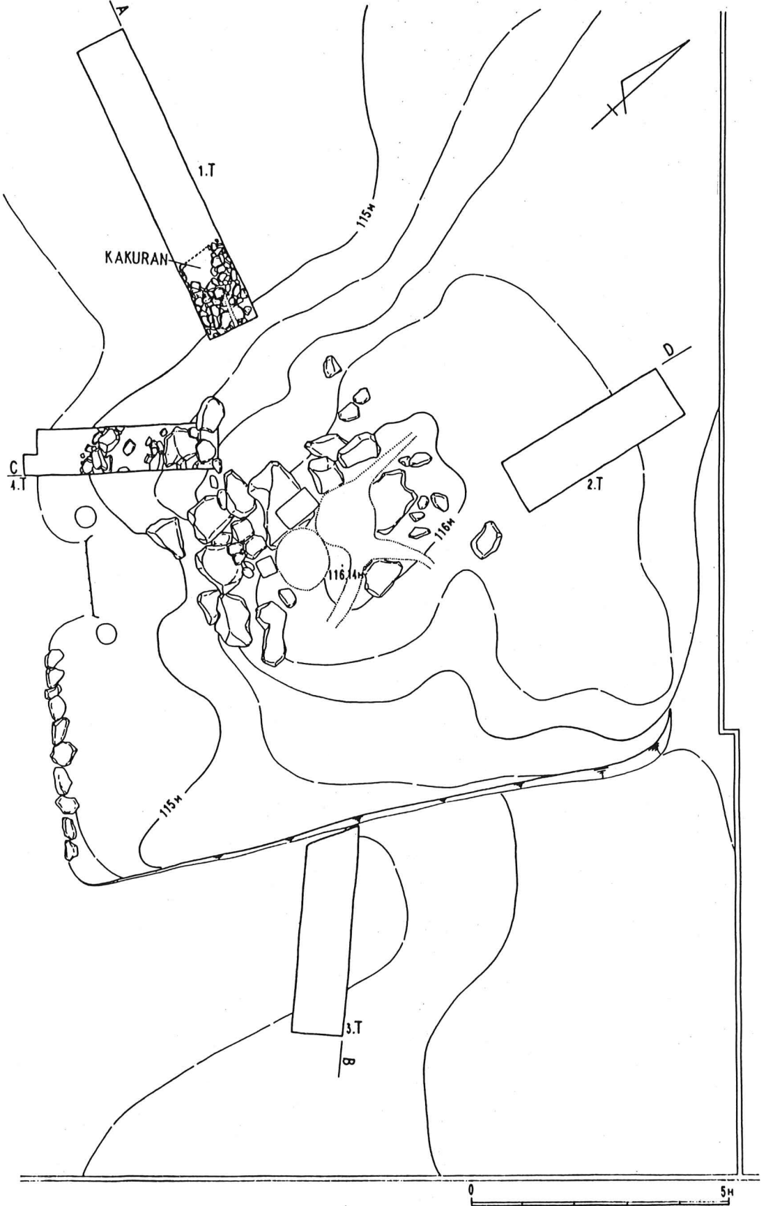
図-7 虚空蔵社古墳墳丘実測図
