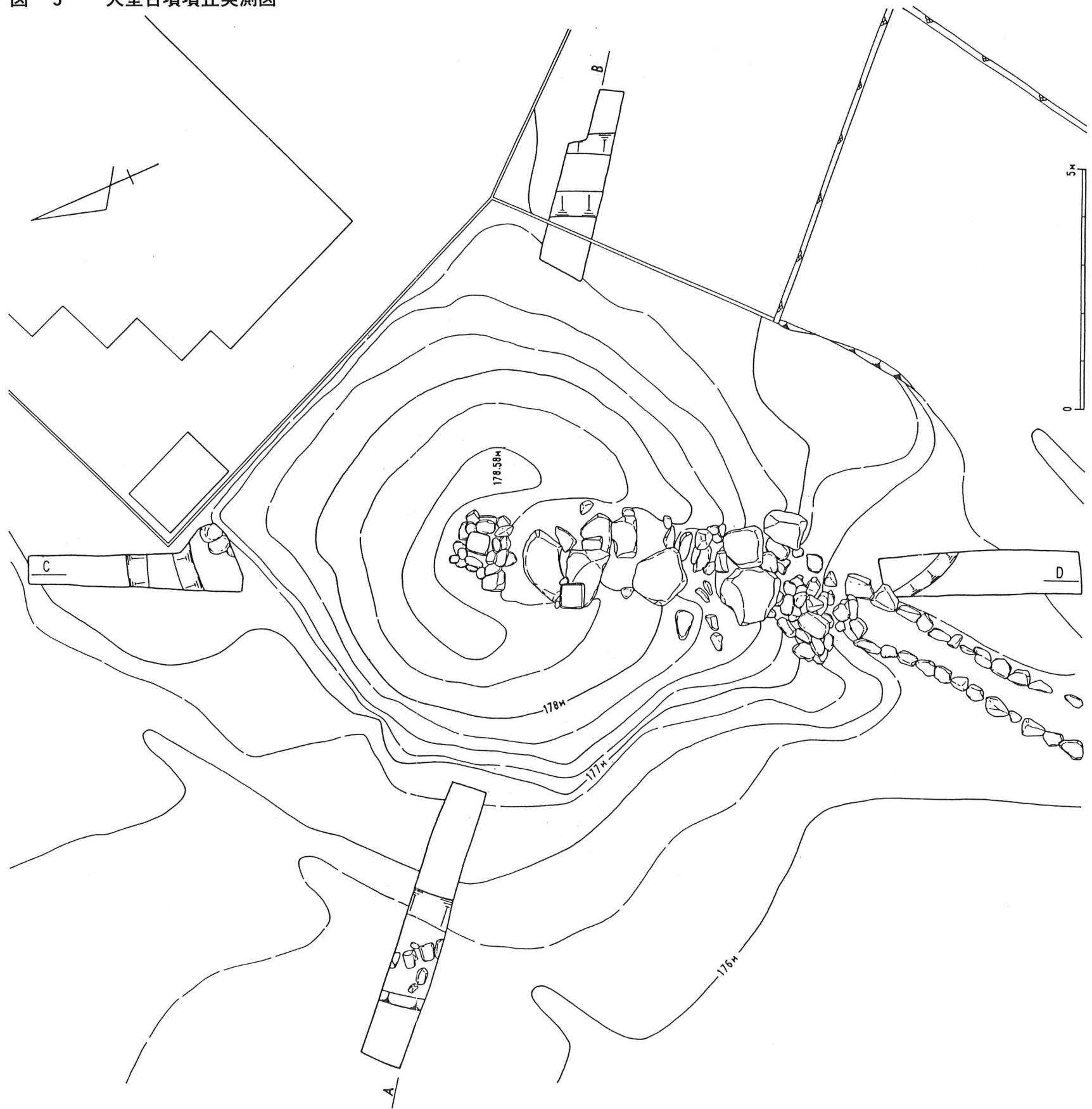
図-3 大室古墳墳丘実測図
