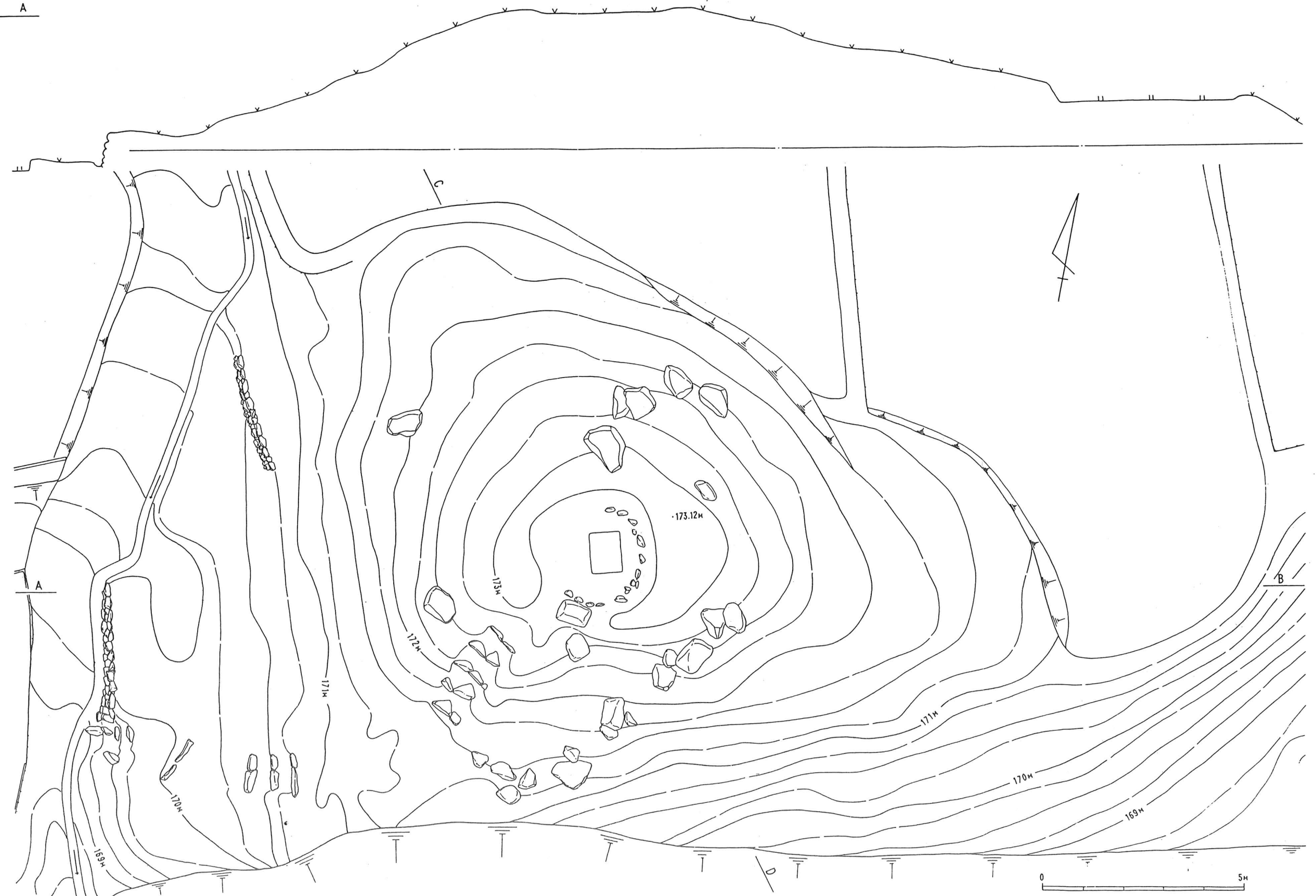
図一五 別所稻荷塚古墳墳丘実測図
