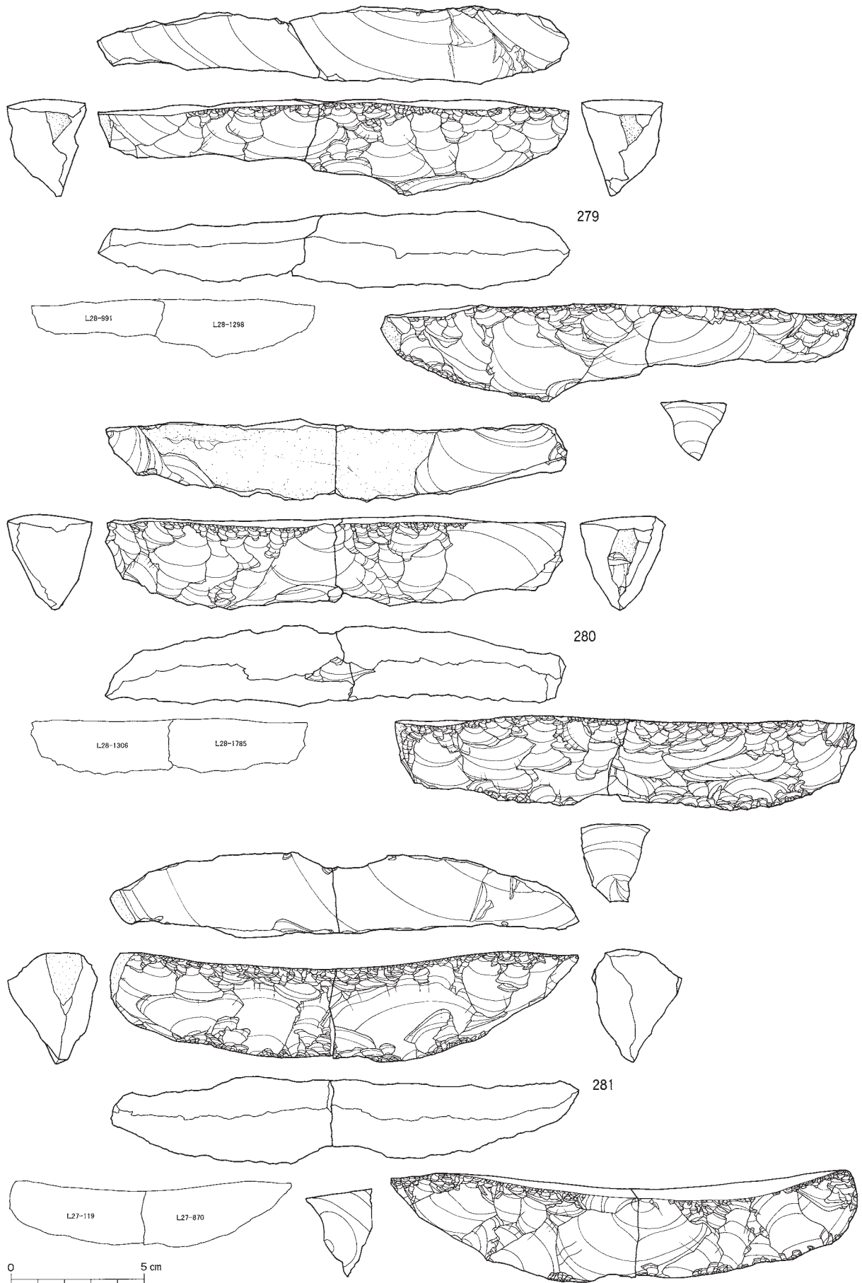
図Ⅲ-247 I区(Sb-91~96)の石器(30) 舟底形石器
