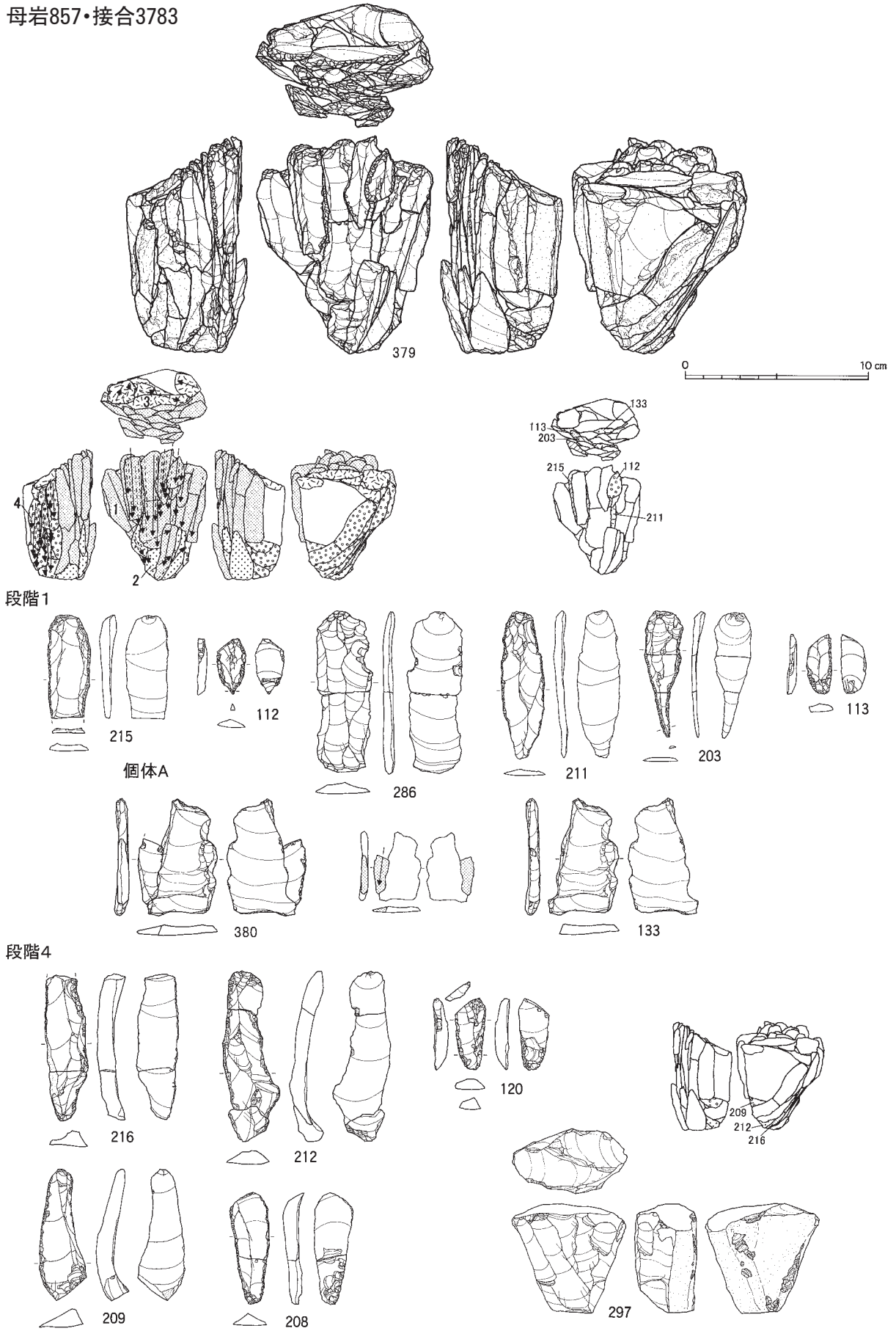
図Ⅲ-340 I区(Sb-91~96)の石器(105) 母岩857・接合3783(1)
