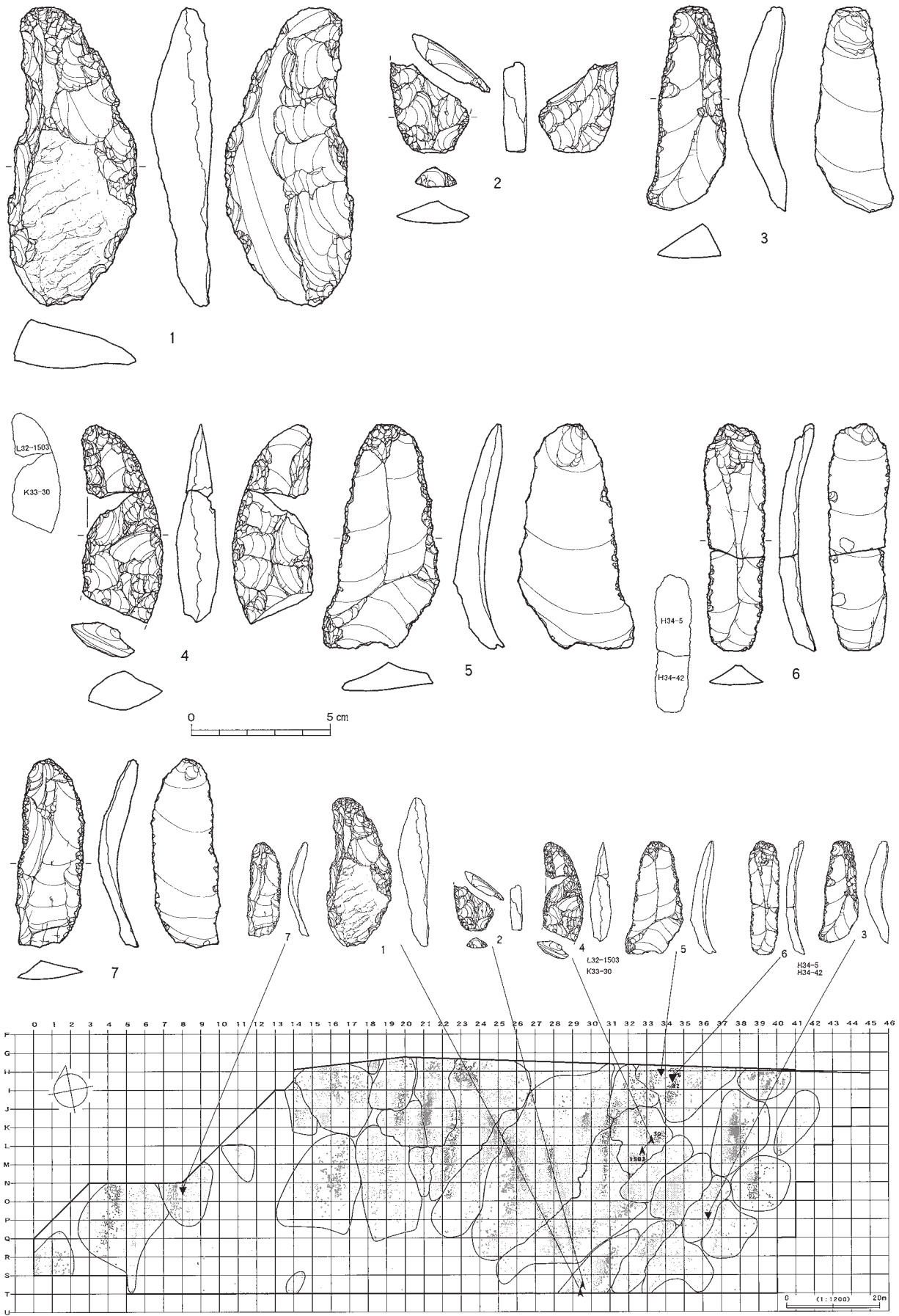
図Ⅲ-513 追加報告の石器(1) 尖頭器・削器、追加報告の石器分布図
