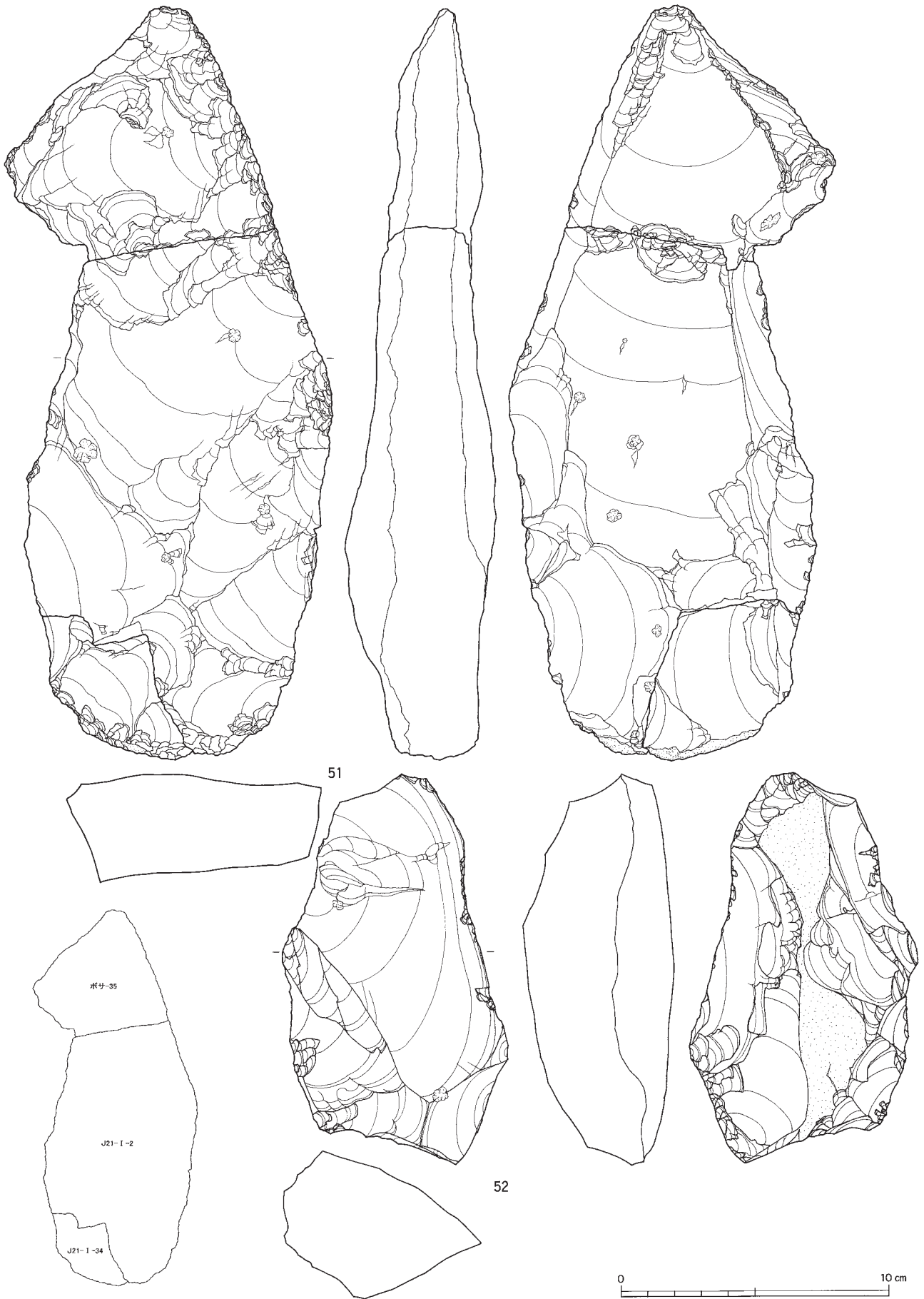
図Ⅲ-379 J区(Sb-97~107)の石器(11) 両面調整石器
