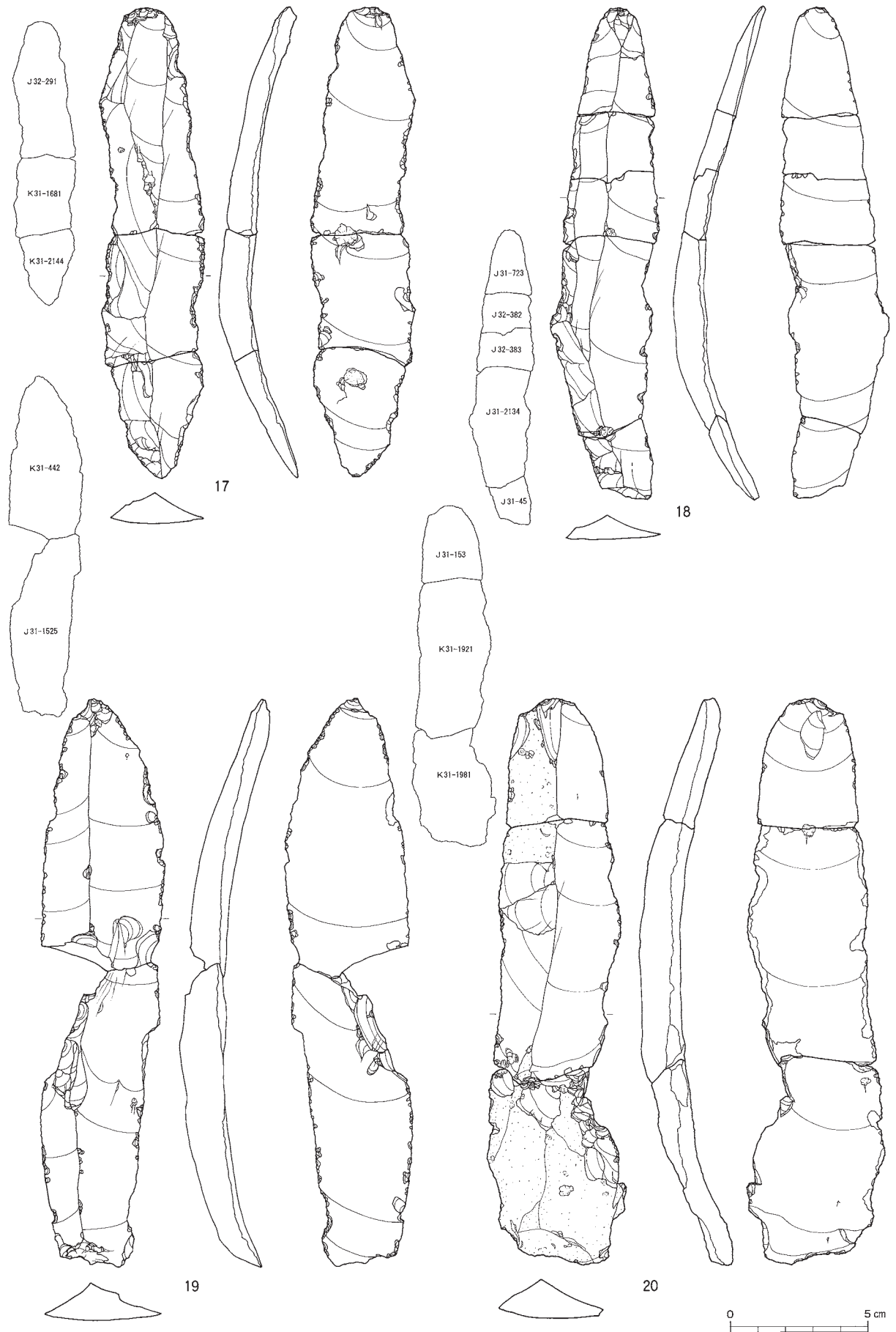
図III-178 H区(Sb-90)の石器(3) 石刃
