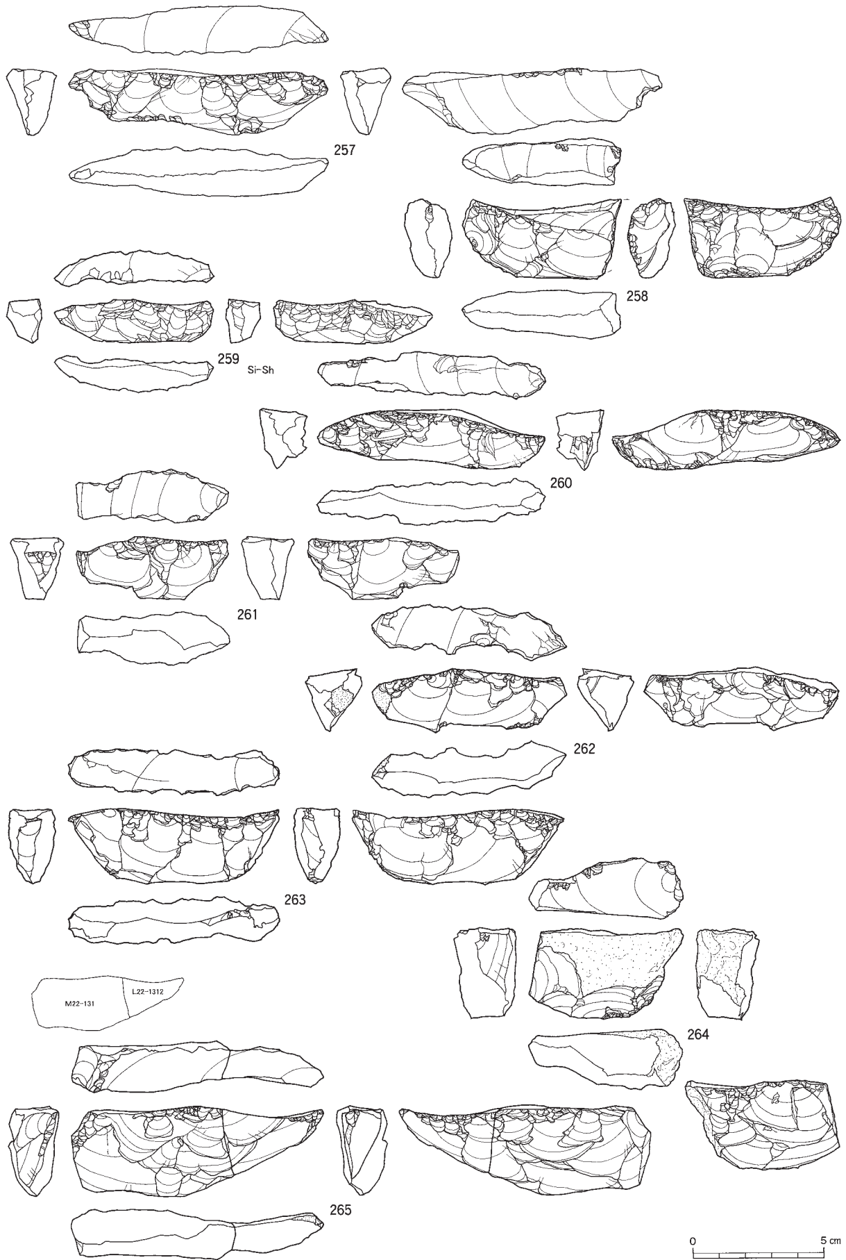
図Ⅲ-396 J区(Sb-97~107)の石器(28) 舟底形石器
