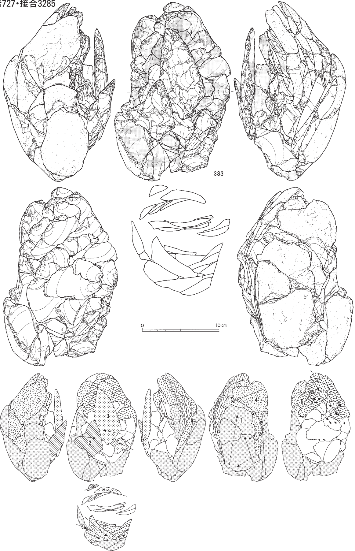
図Ⅲ-277 I区(Sb-91~96)の石器(42) 母岩727・接合3285(1)
