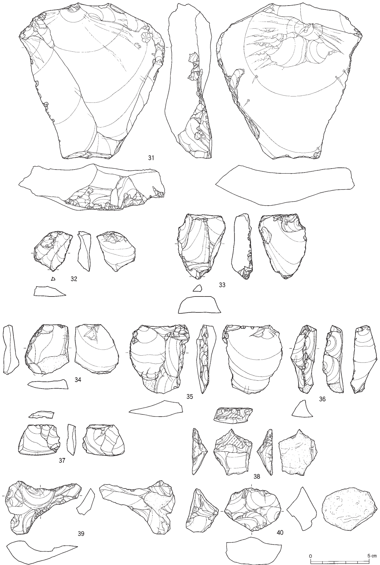
図Ⅲ-45 Sb-64~70の石器(3) 搔器・錐形石器・削器・縦長剥片・石核
