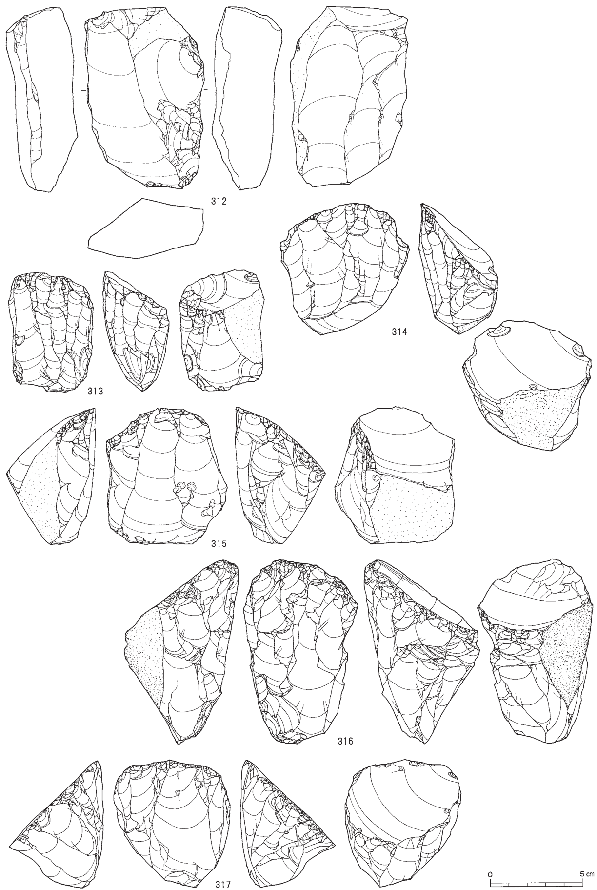
図Ⅲ-404 J区(Sb-97~107)の石器(36) 石刃核
