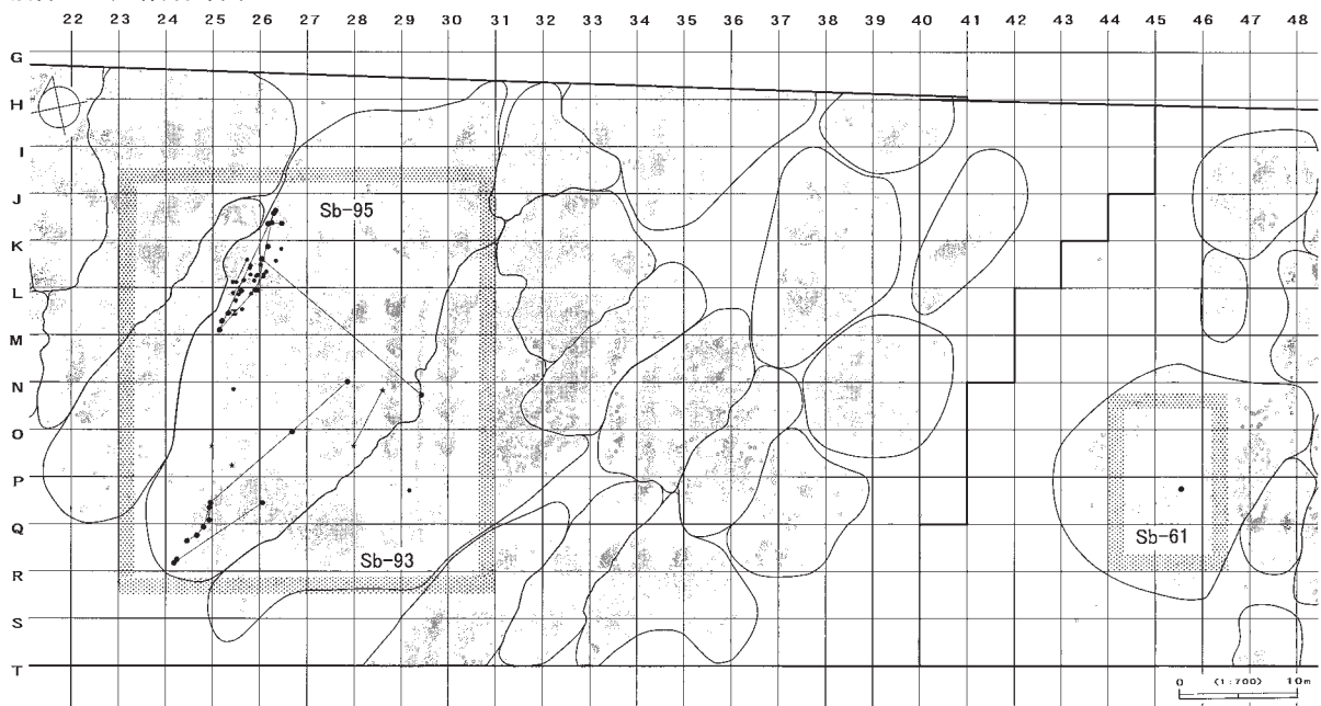
図Ⅲ-327 I区(Sb-91~96)の石器(92) 母岩933・接合4061(2)
