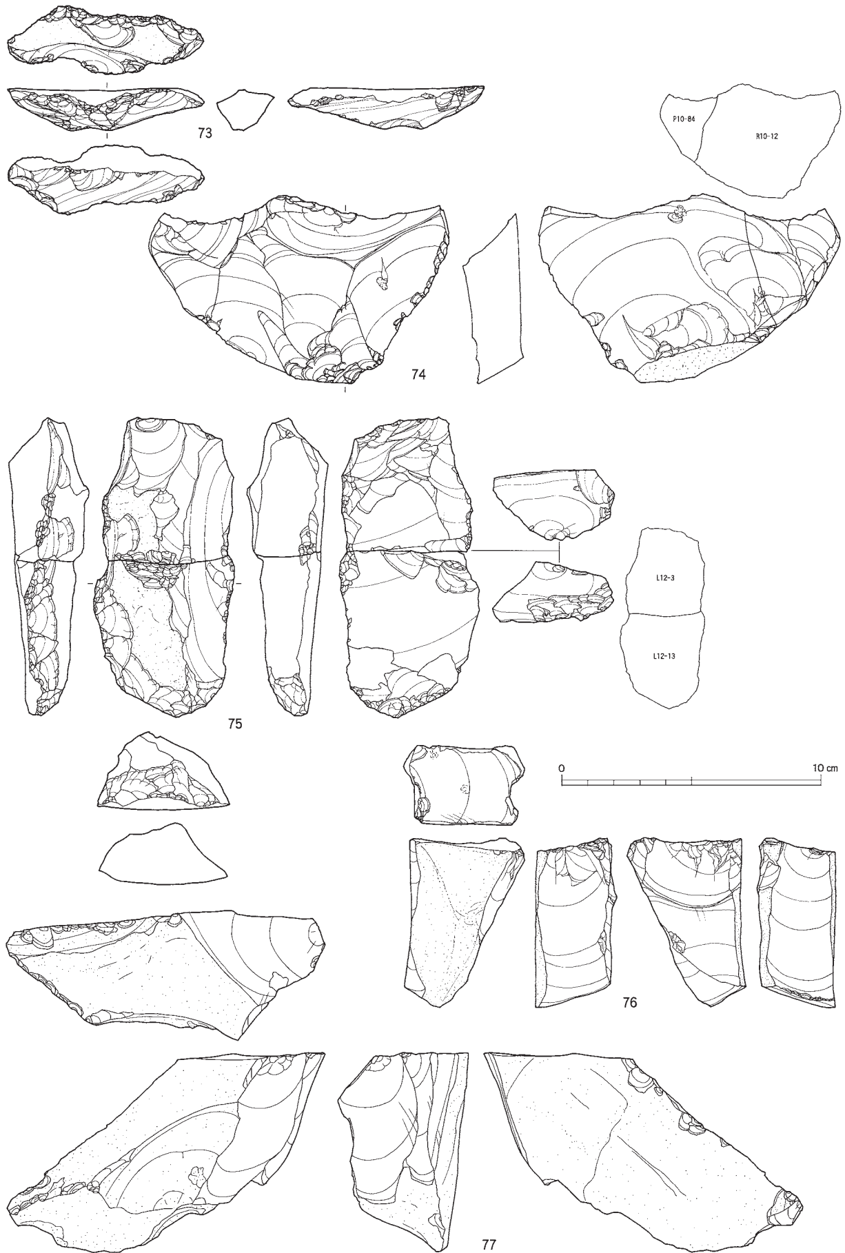
図Ⅲ-87 Sb-72~79の石器(12) 石核
