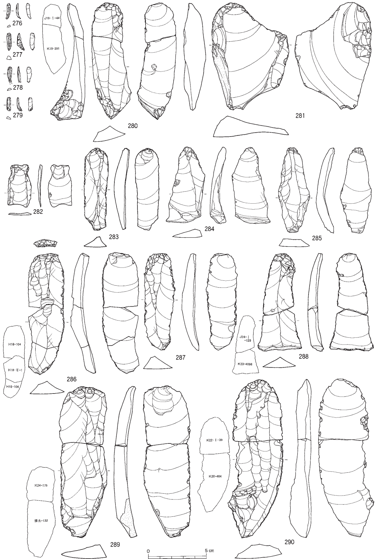
図Ⅲ-399 J区(Sb-97~107)の石器(31) 舟底形石器削片・二次加工ある剥片・つまみ付きナイフ・石刃
