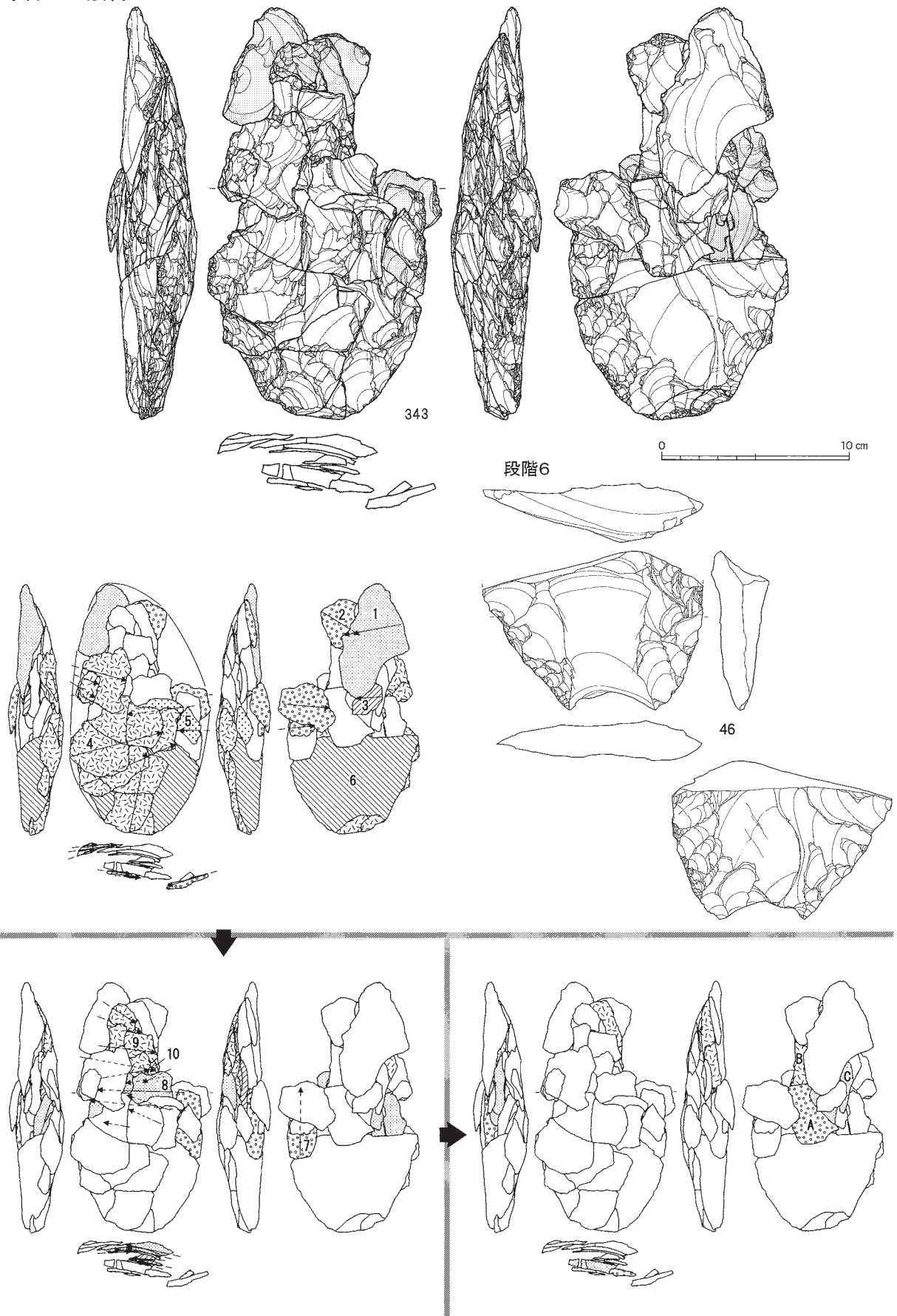
図Ⅲ-294 I区(Sb-91~96)の石器(59) 母岩807・接合3583(1)
