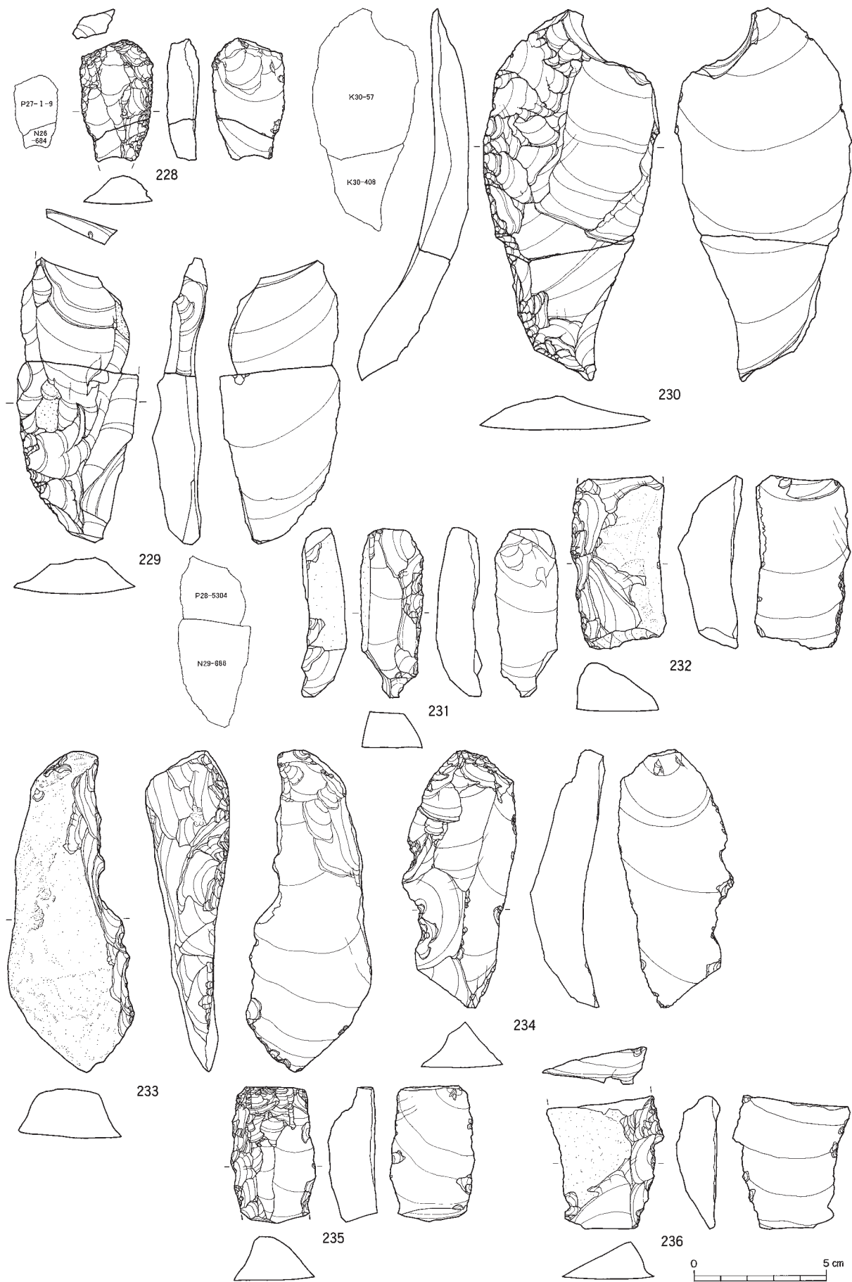
図Ⅲ-242 I区(Sb-91~96)の石器(25) 削器
