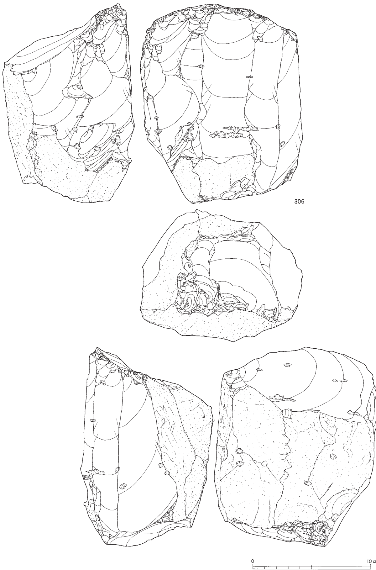
図Ⅲ-402 J区(Sb-97~107)の石器(34) 石刃核
