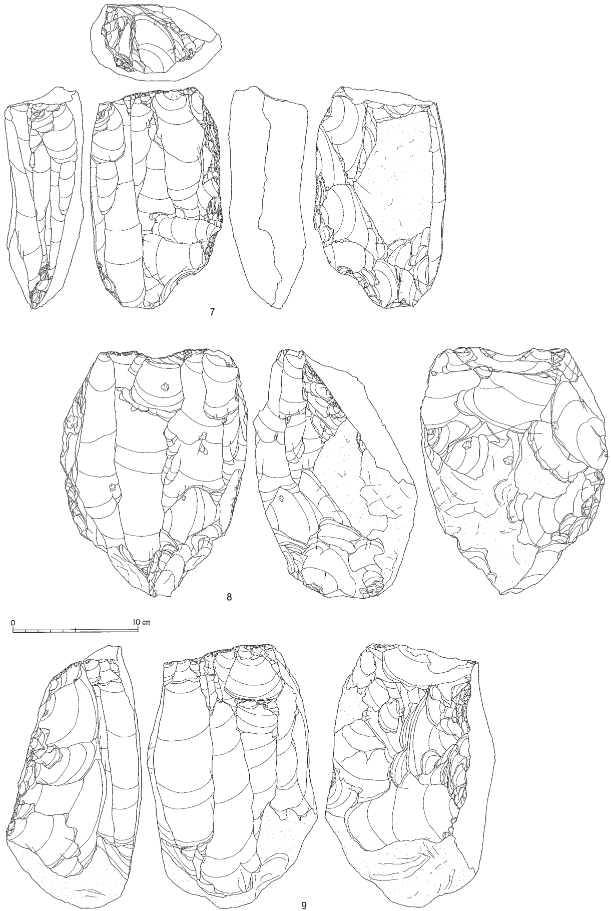
図Ⅲ-512 表土(重機調査)の石器(2) 石刃核
