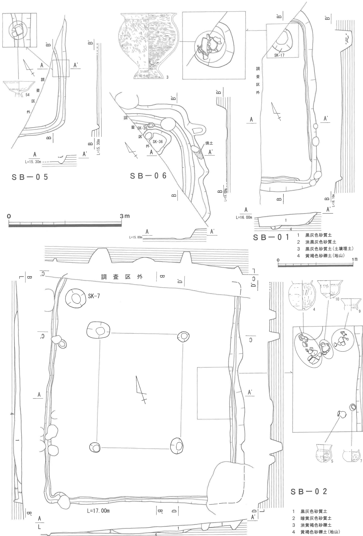
第11図 遺構実測図-1 (1/60・1/30)
