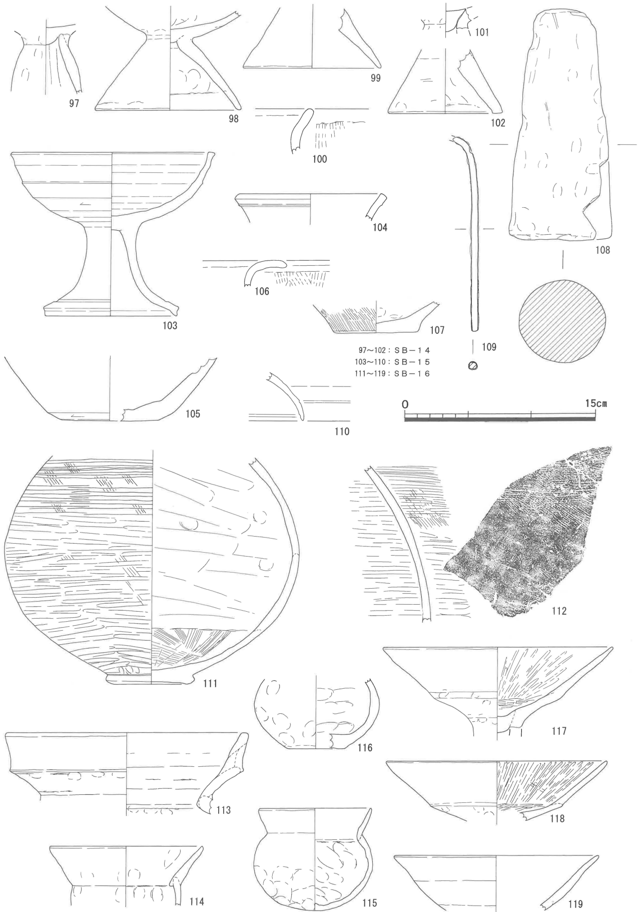
第28图 出土遺物実測図一6 (1/3)
