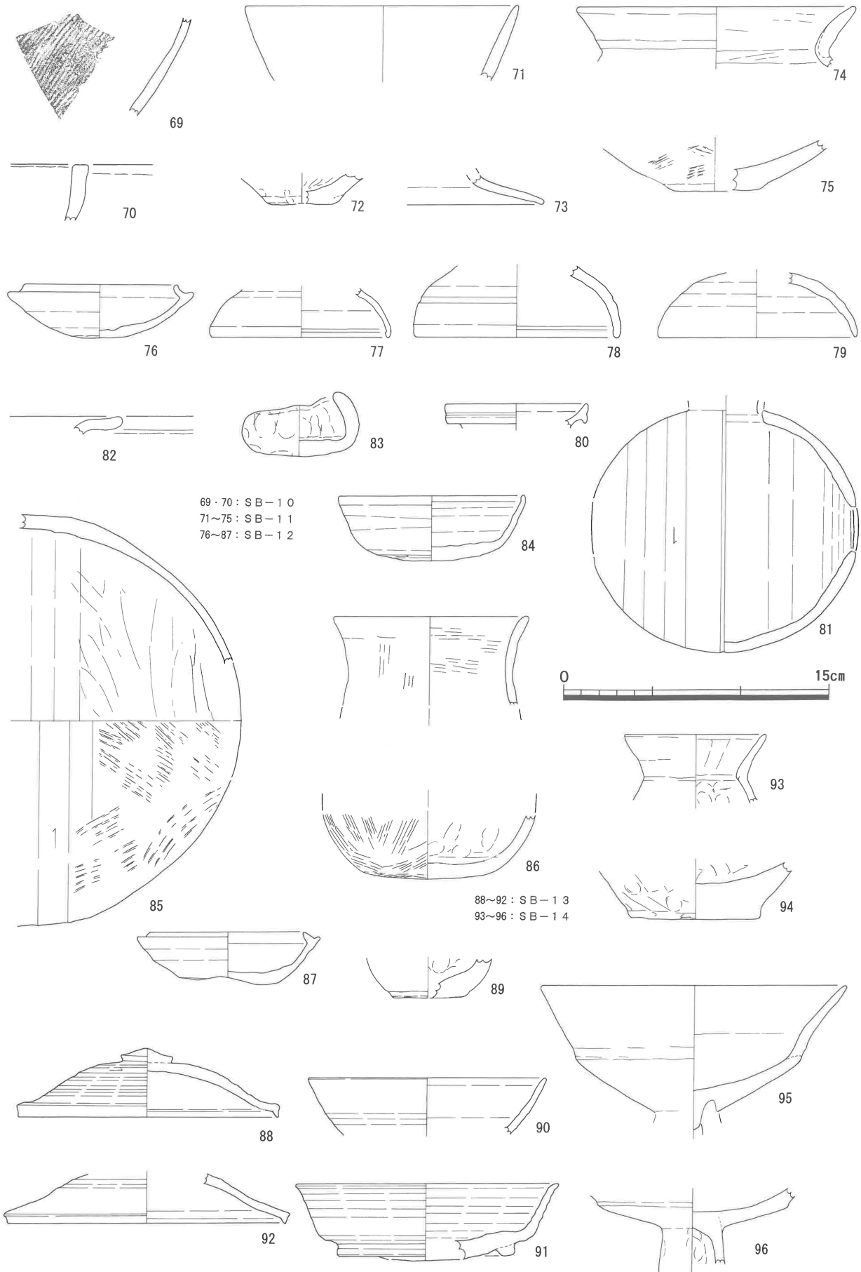
第27図 出土遺物実測図一5(1/3)
