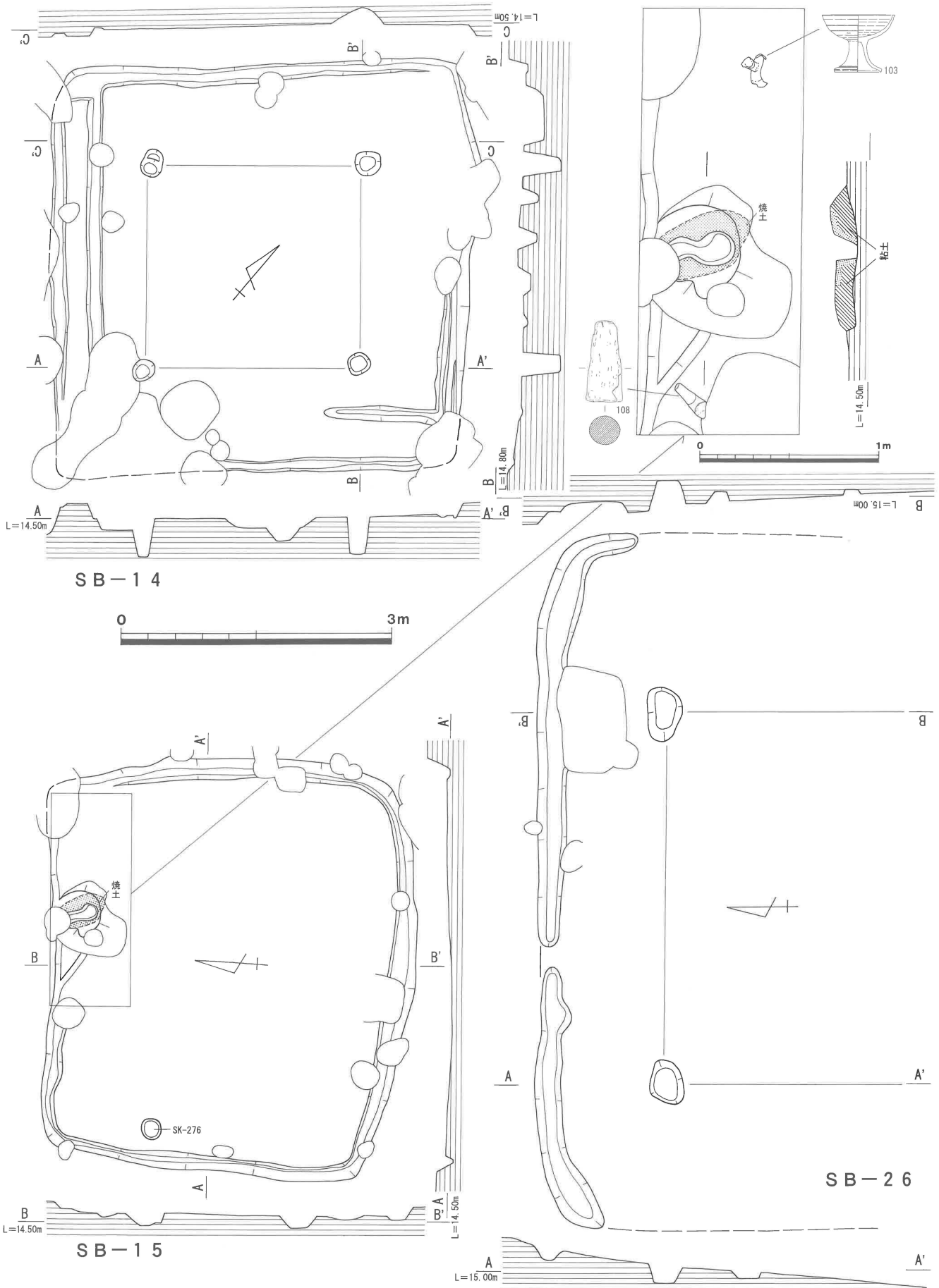
第15图 遺構実測図一5 (1/60・1/30)
