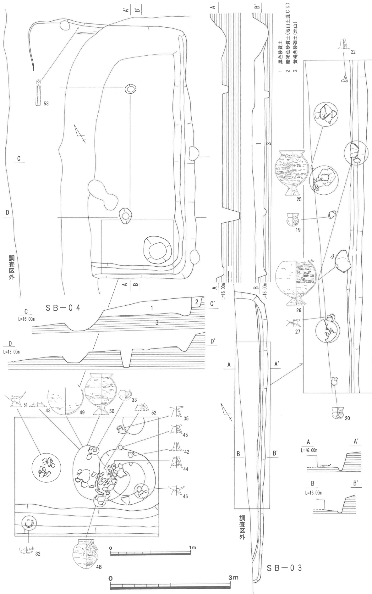
第12図 遺構実測図-2 (1/60・1/30)
