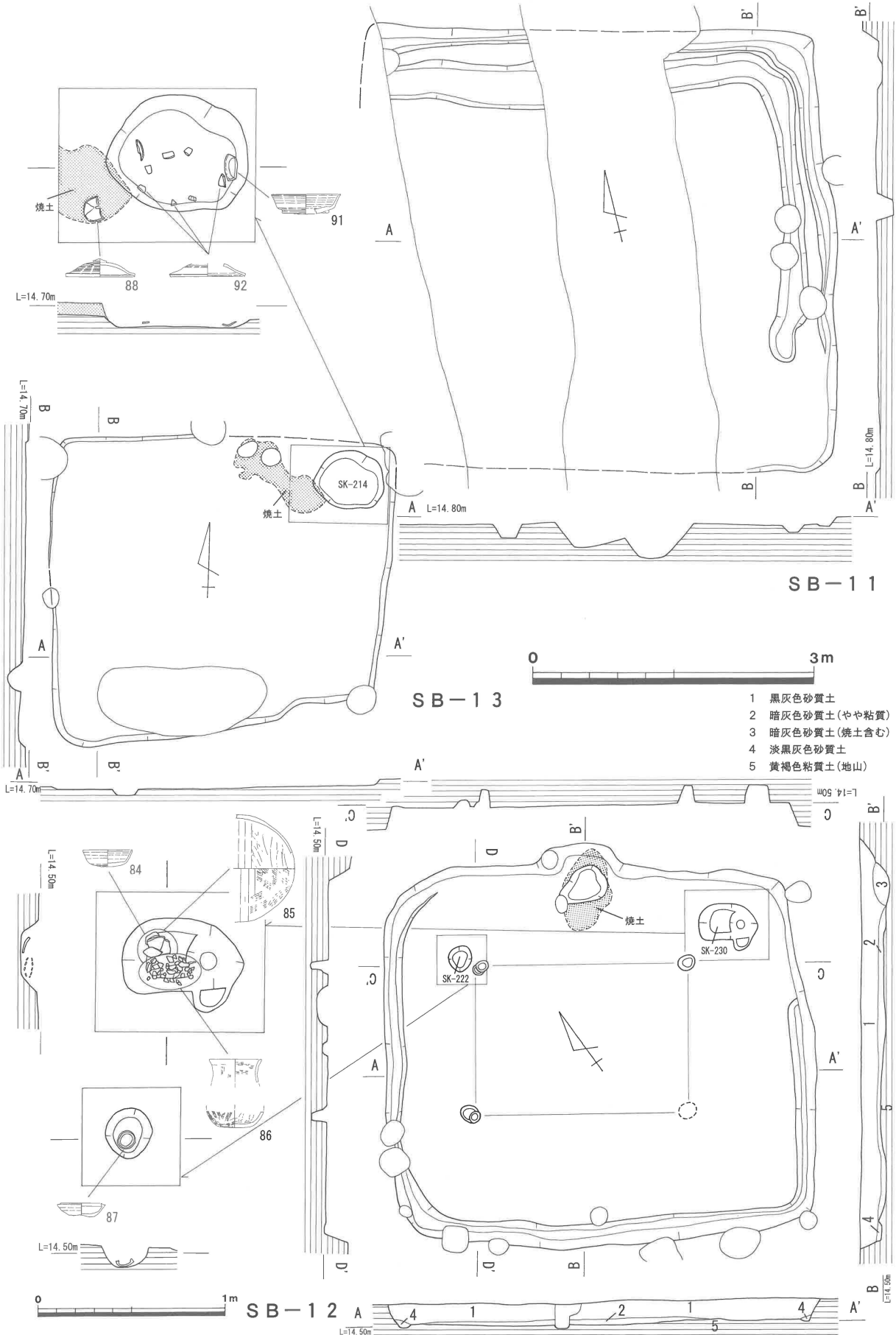
第14図 遺構実測図-4 (1/60・1/30)
