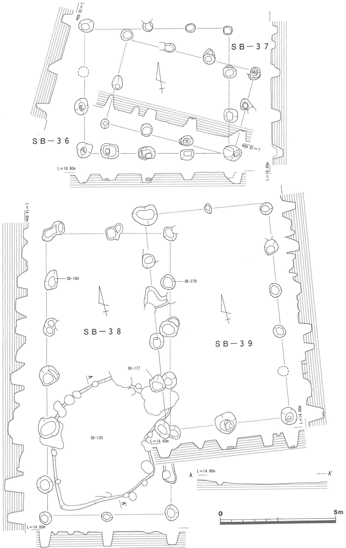
第22図 遺構実測図-12 (1/100)
