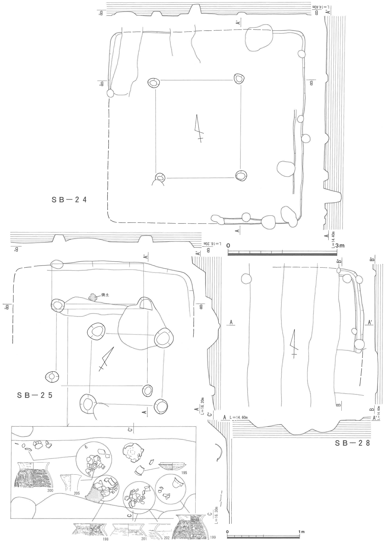
第19图 遺構実測図-9 (1/60・1/30)
