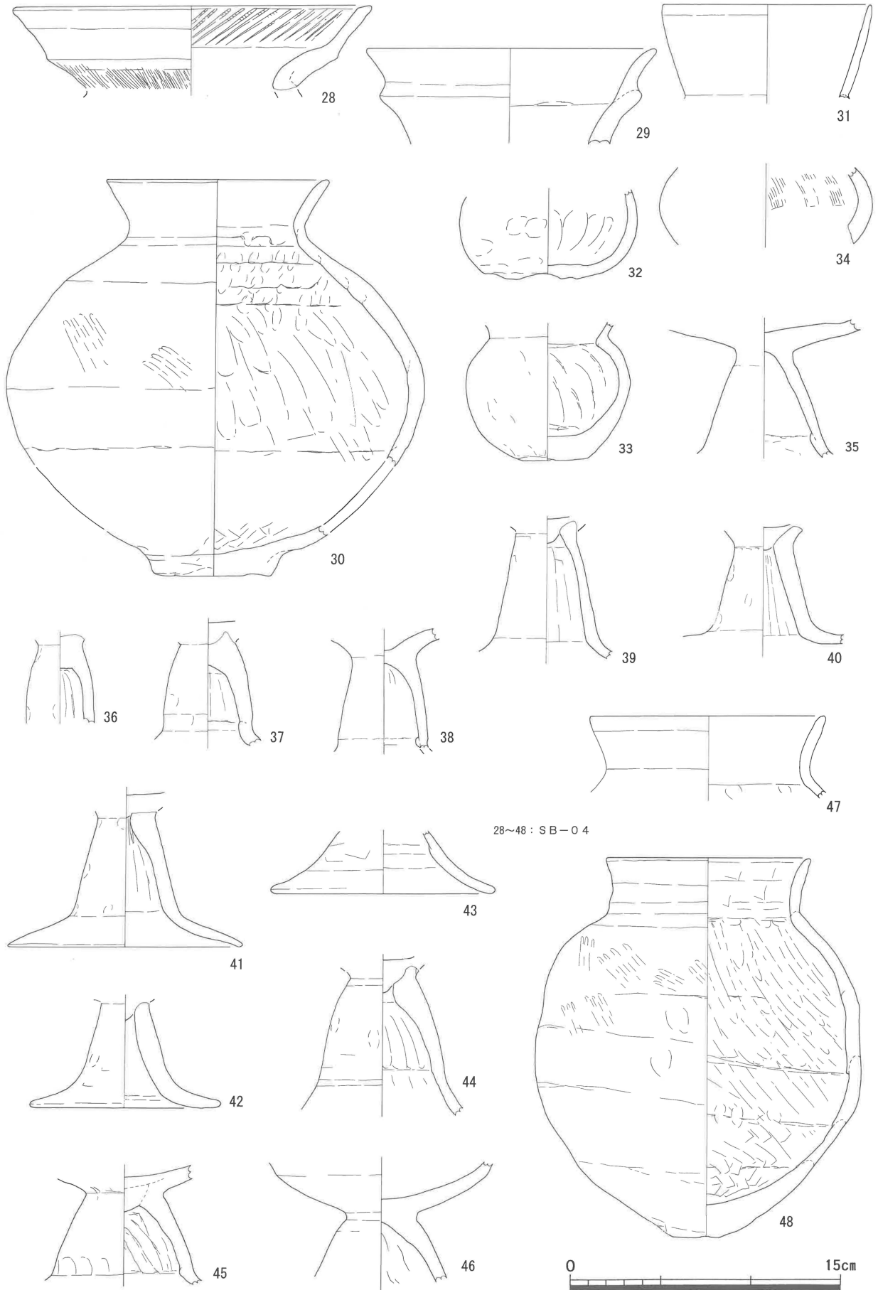
第25图 出土遺物実測図一3 (1/3)
