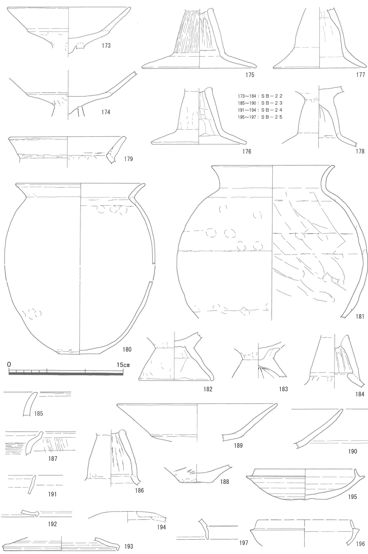
第31图 出土遺物実測図一9 (1/3)
