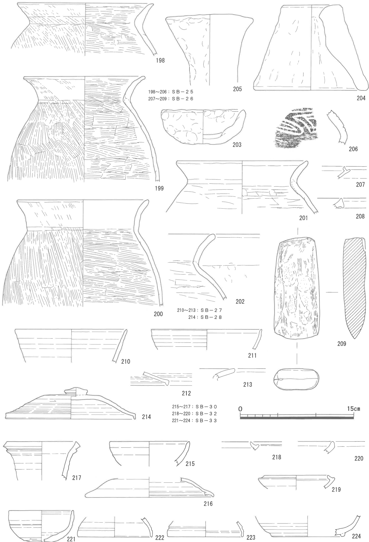
第32图 出土遺物実測図-10 (1/3)
