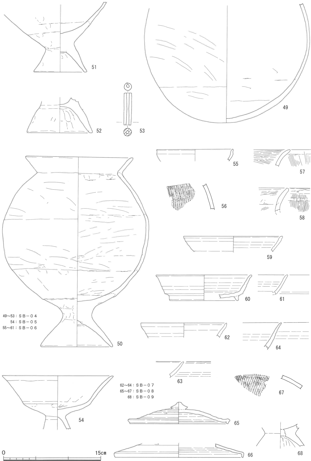
第26图 出土遺物実測図一4 (1/3)
