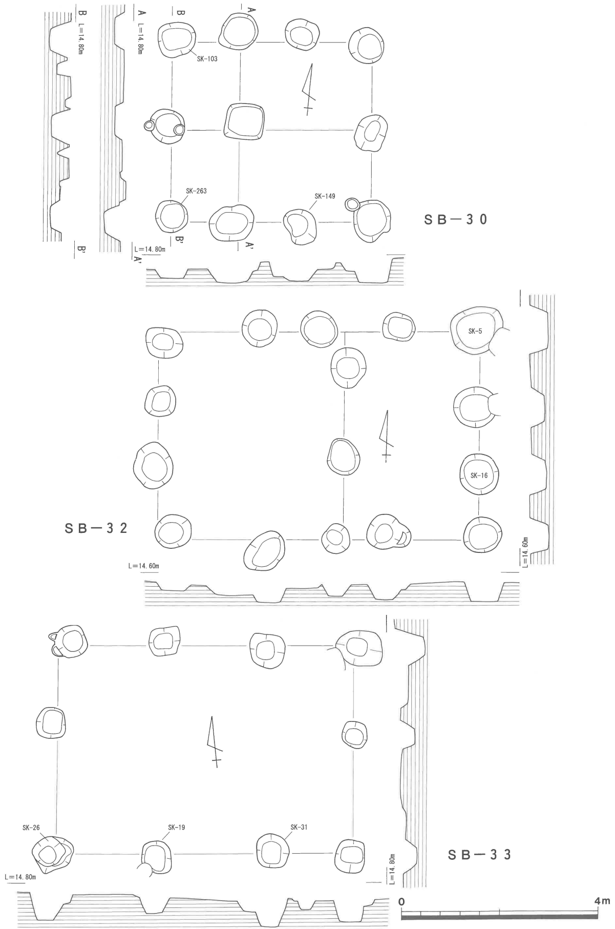
第21図 遺構実測図一11 (1/80)
