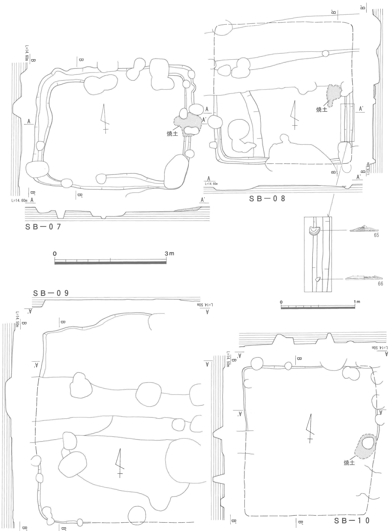
第13図 遺構実測図一3 (1/60・1/30)
