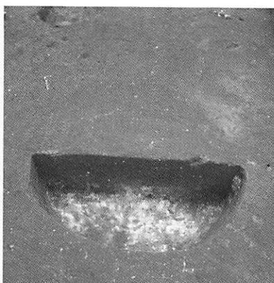
P1311 セクション NE →
