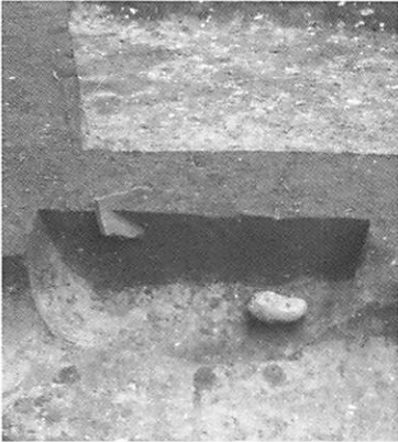
P1400 セクション (外 H60) NE →
