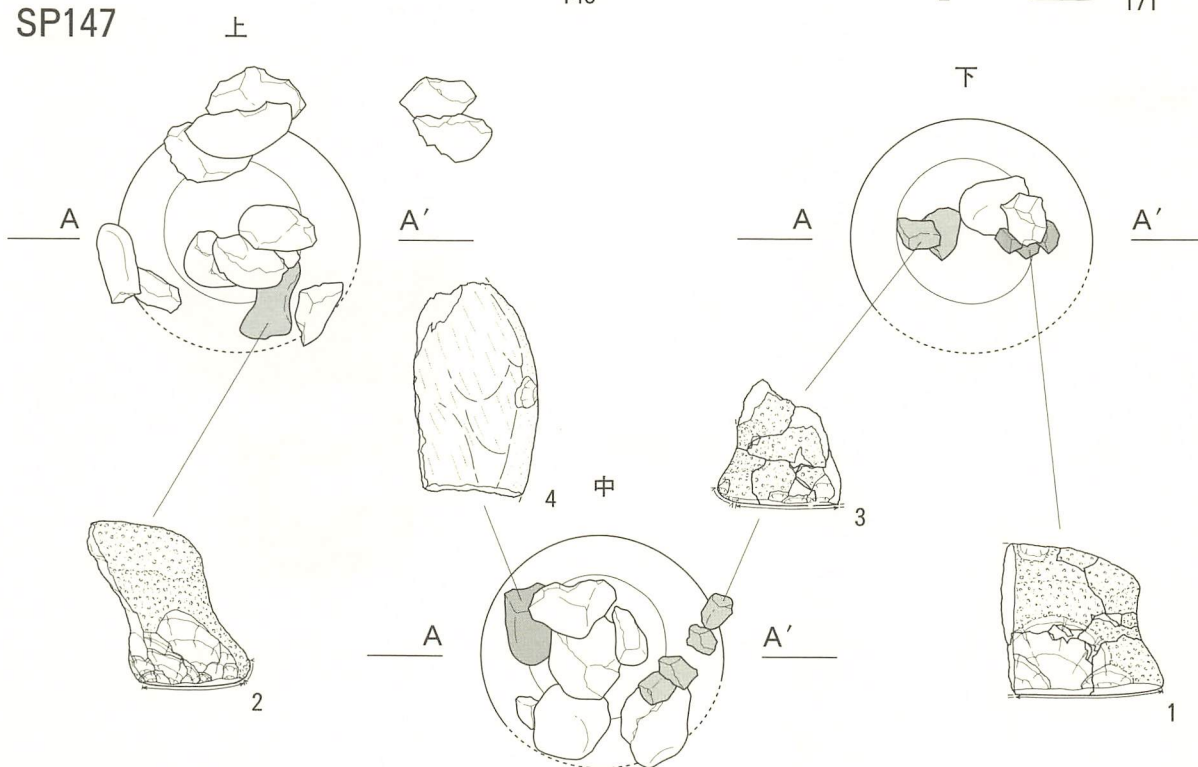
図IV-147 SP263~266 平面図・断面図 SP50・SP62・SP147遺物出土状況図
