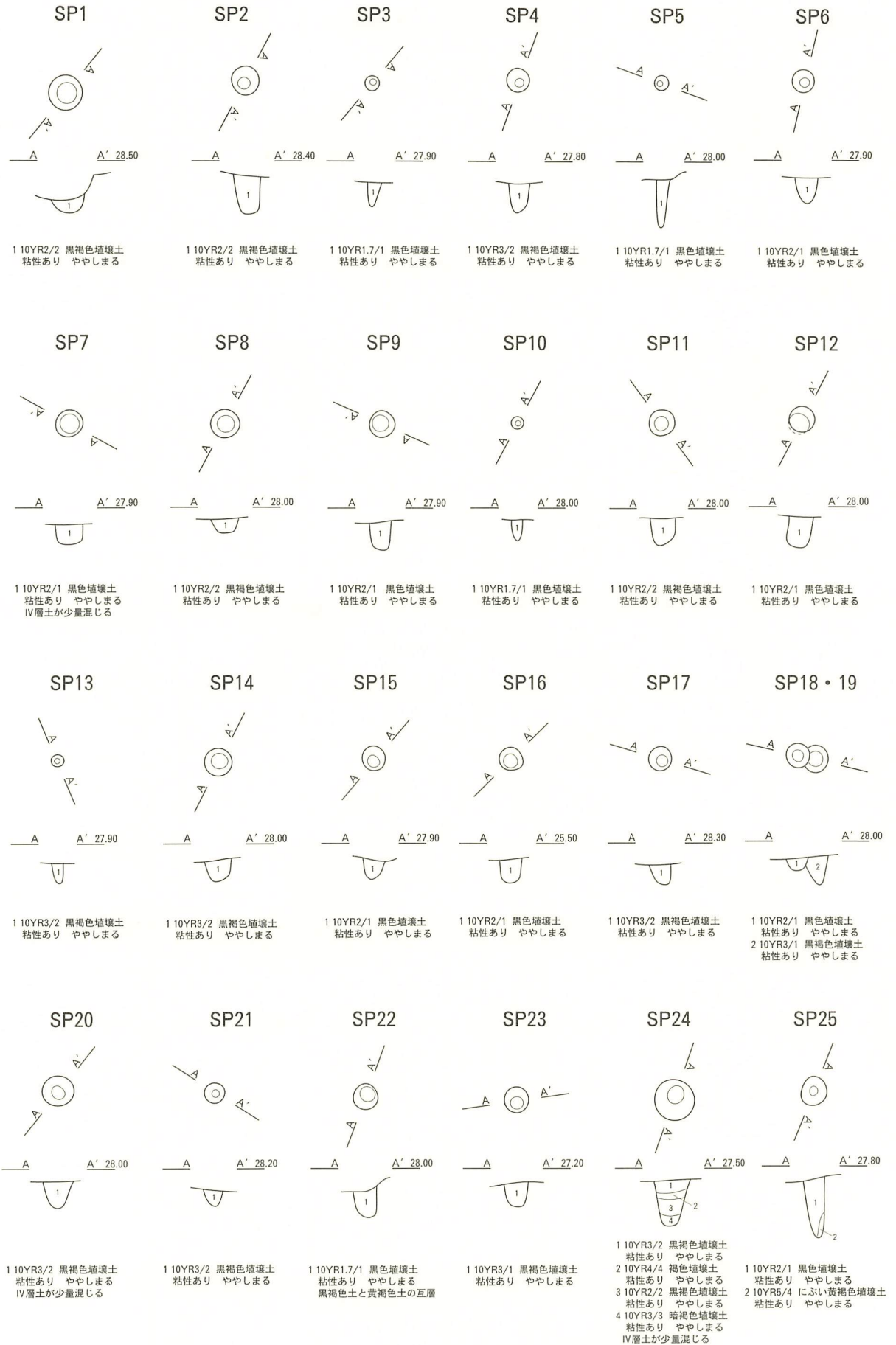
図IV-136 SP1~25 平面図・断面図
