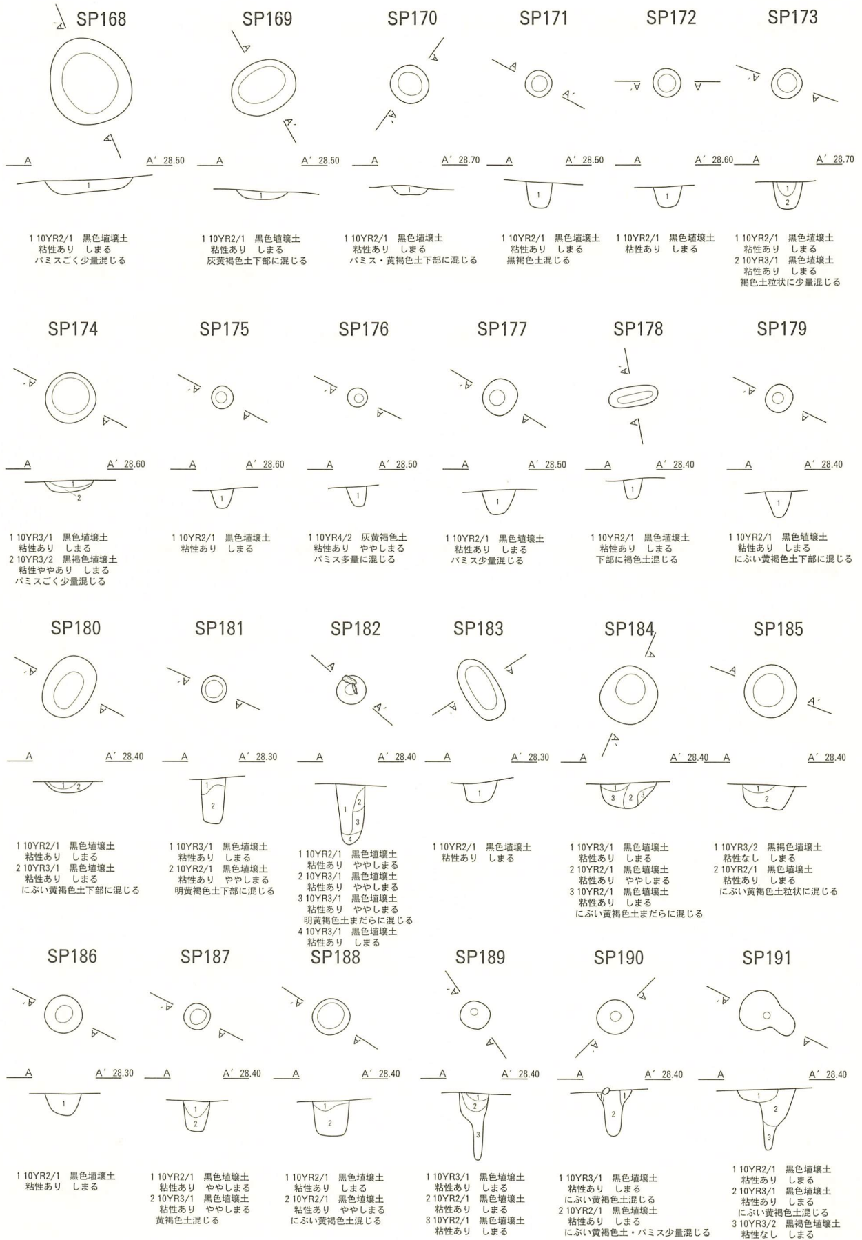
図IV-143 SP168~191平面図・断面図
