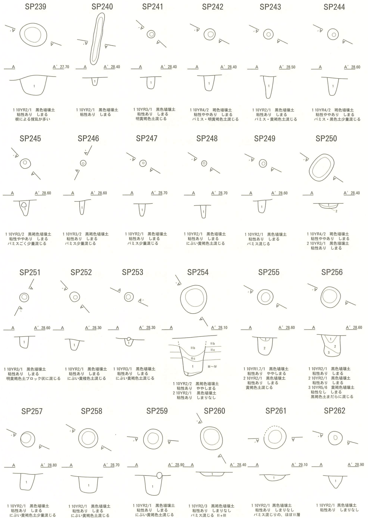
図IV-146 SP239~262平面図・断面図
