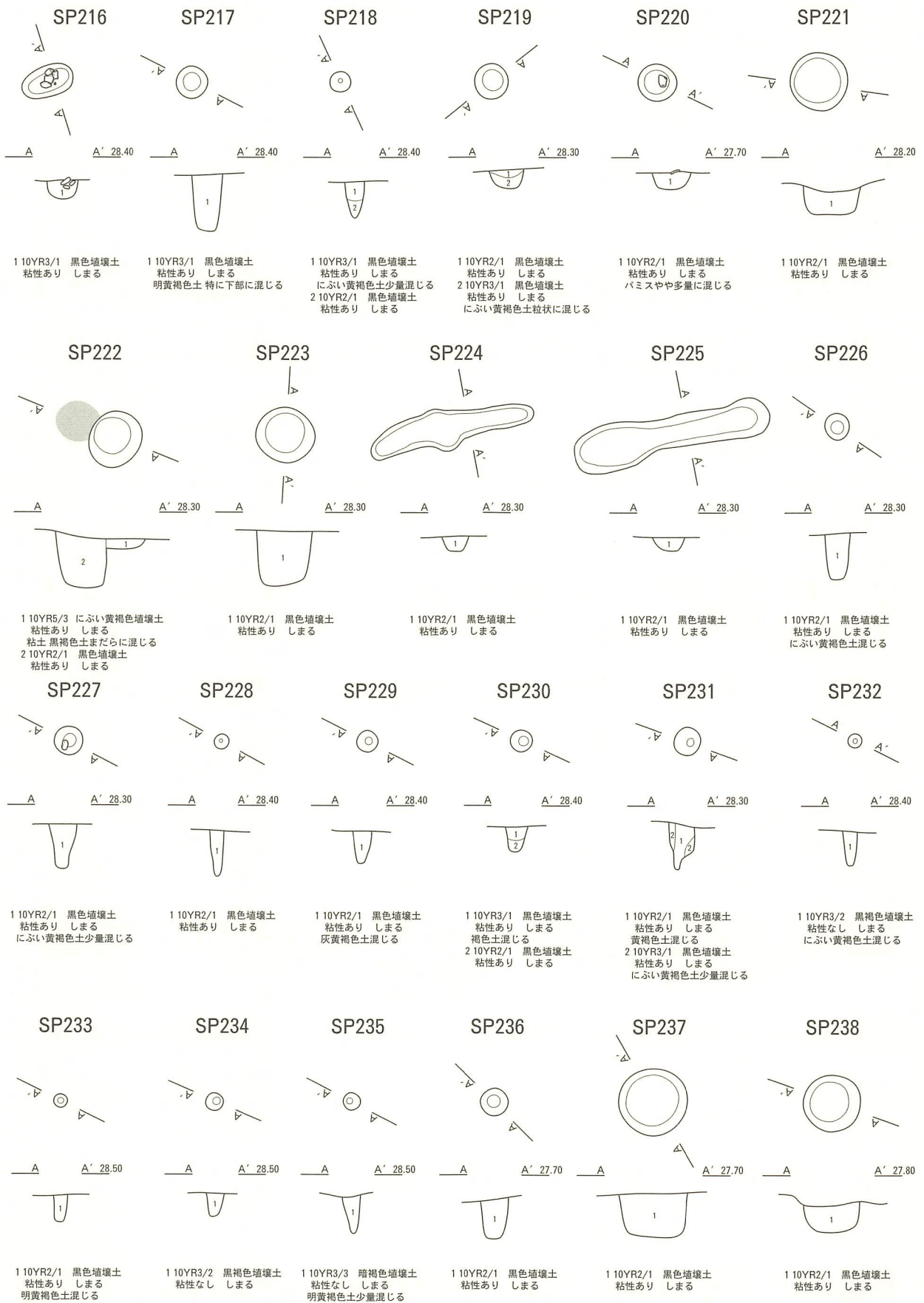
図IV-145 SP216~238平面図・断面図
