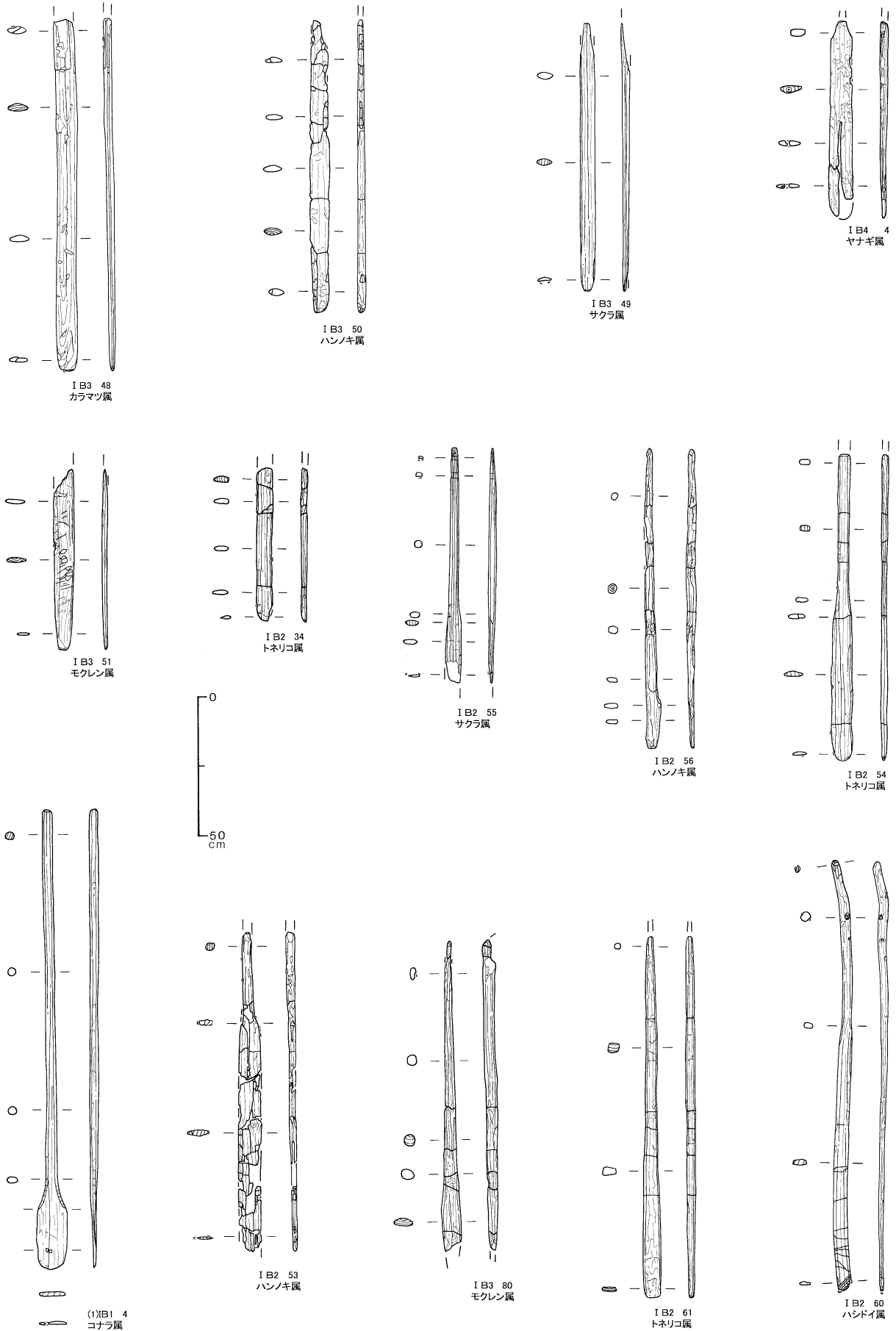
図 - 5 車輻(2)・早樫
