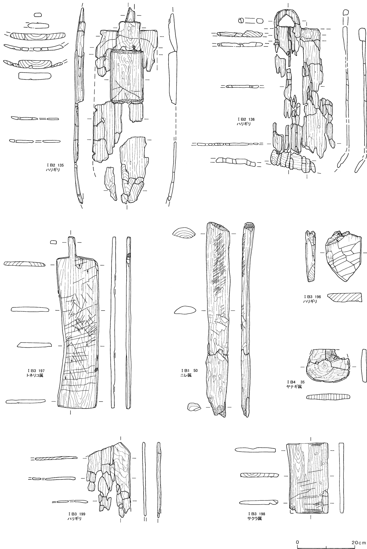
図 - 14 まな板・作業台
