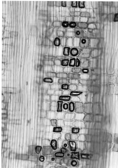
70 現生ヤマザクラの根材 c × 205
