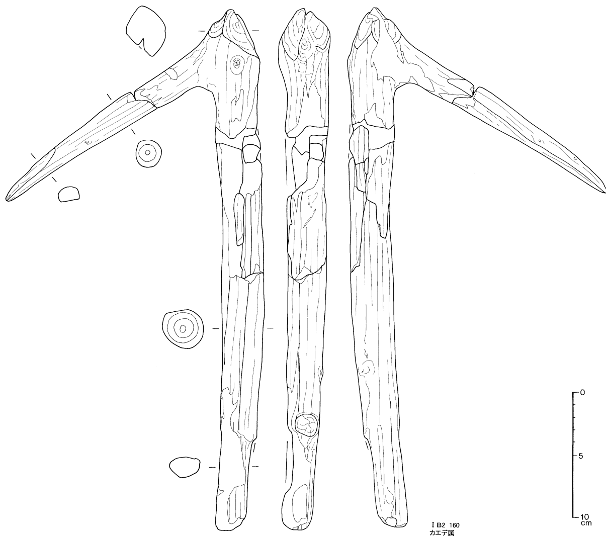
図 - 3 修正木製品(3)
