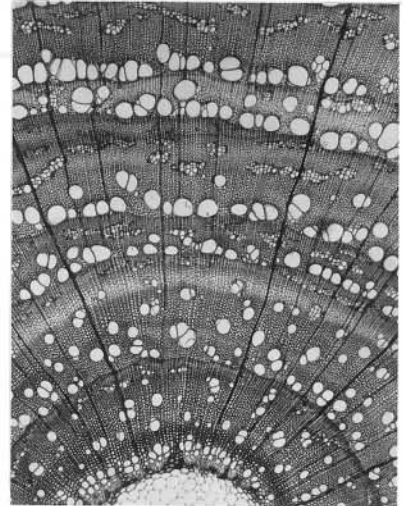
8 現生オヒヨウの枝材 a × 28
