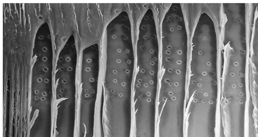
91 アスナロの分野壁孔
