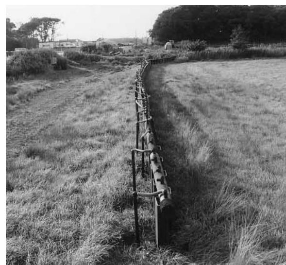
ウエル・ポイント吸水管・集水管
