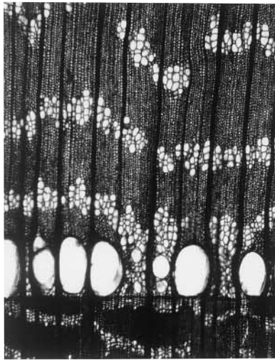
33 現生ハリギリの主幹材 a × 28
