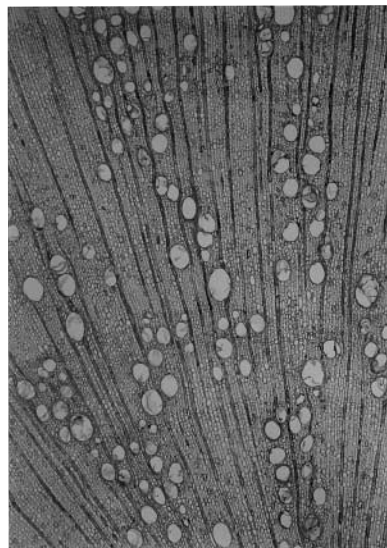
48 現生コシアブラの根材 a × 20.5
