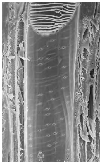
78 サワフタギ 道管のらせん肥厚 × 240
