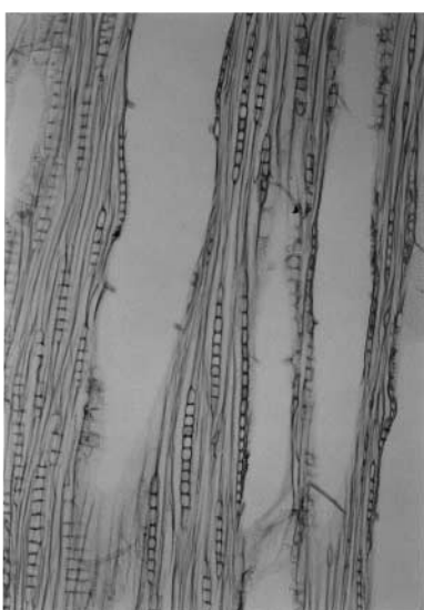
67 現生ヤマナシ類の根材 b × 51 3
