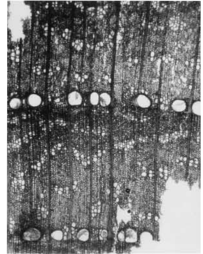
38 出土材ハリギリの主幹材 a × 28
