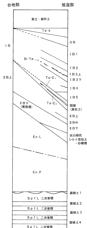
図 - 11 土層模式図
