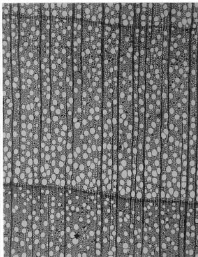
54 現生ナナカマドの主幹材 a × 28
