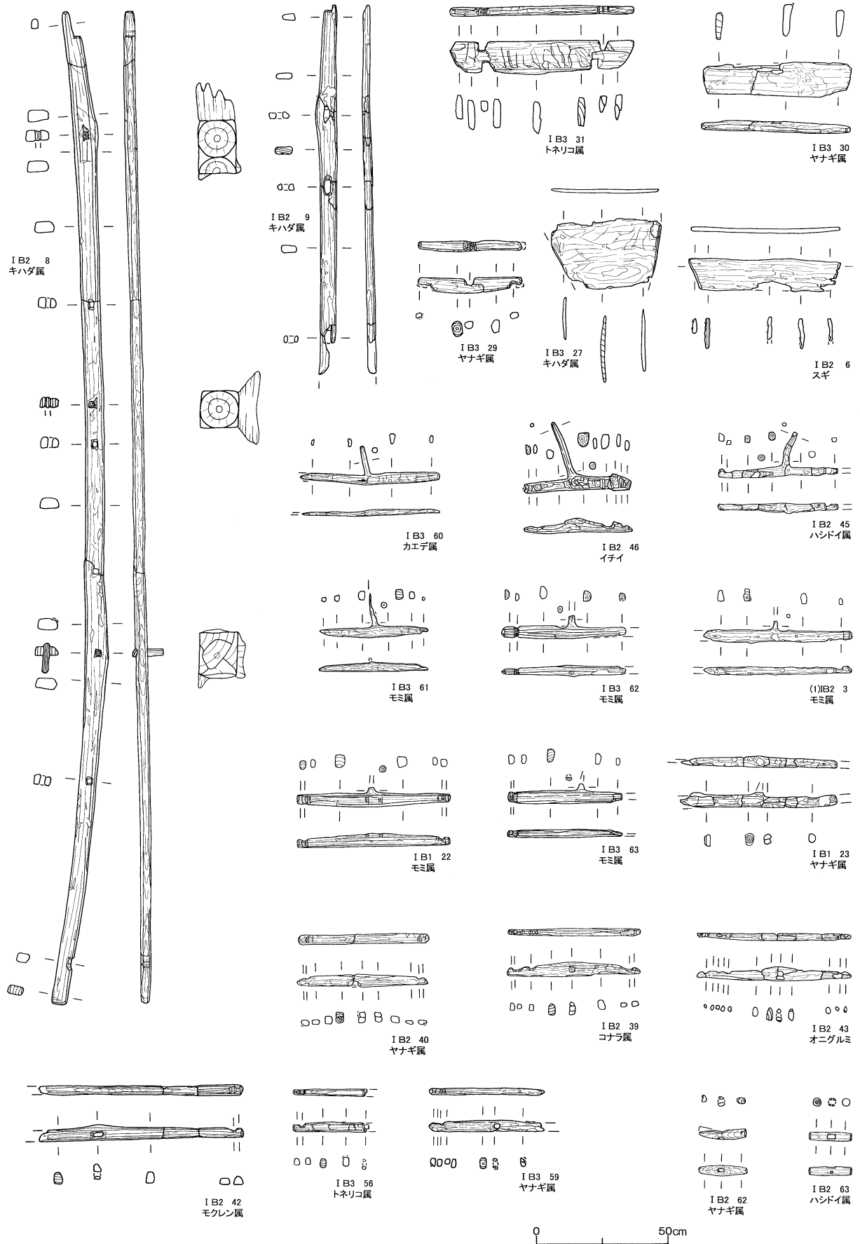
図 - 3 舟部材・車輻受台部等
