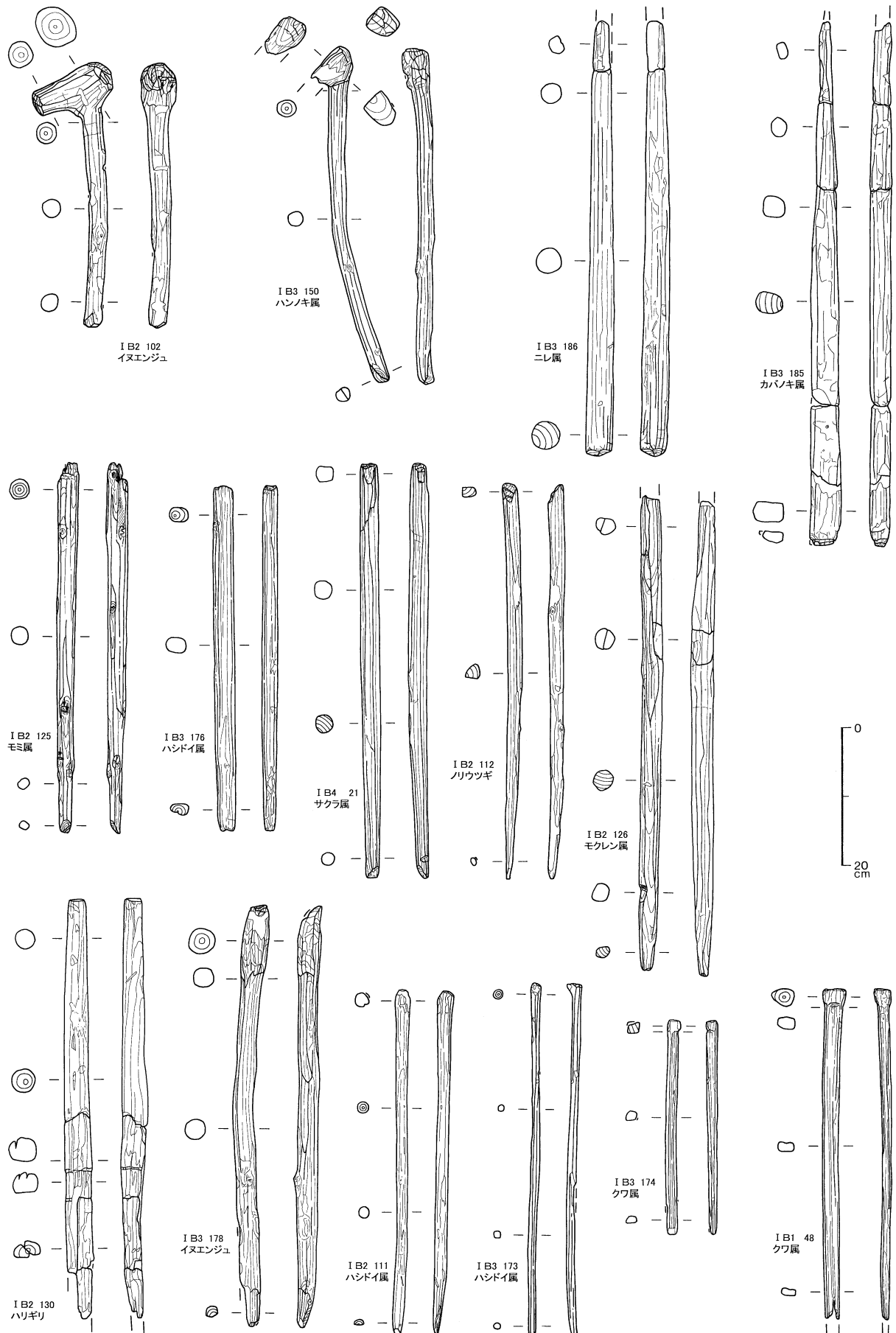
図 - 9 斧柄・柄類 (1)
