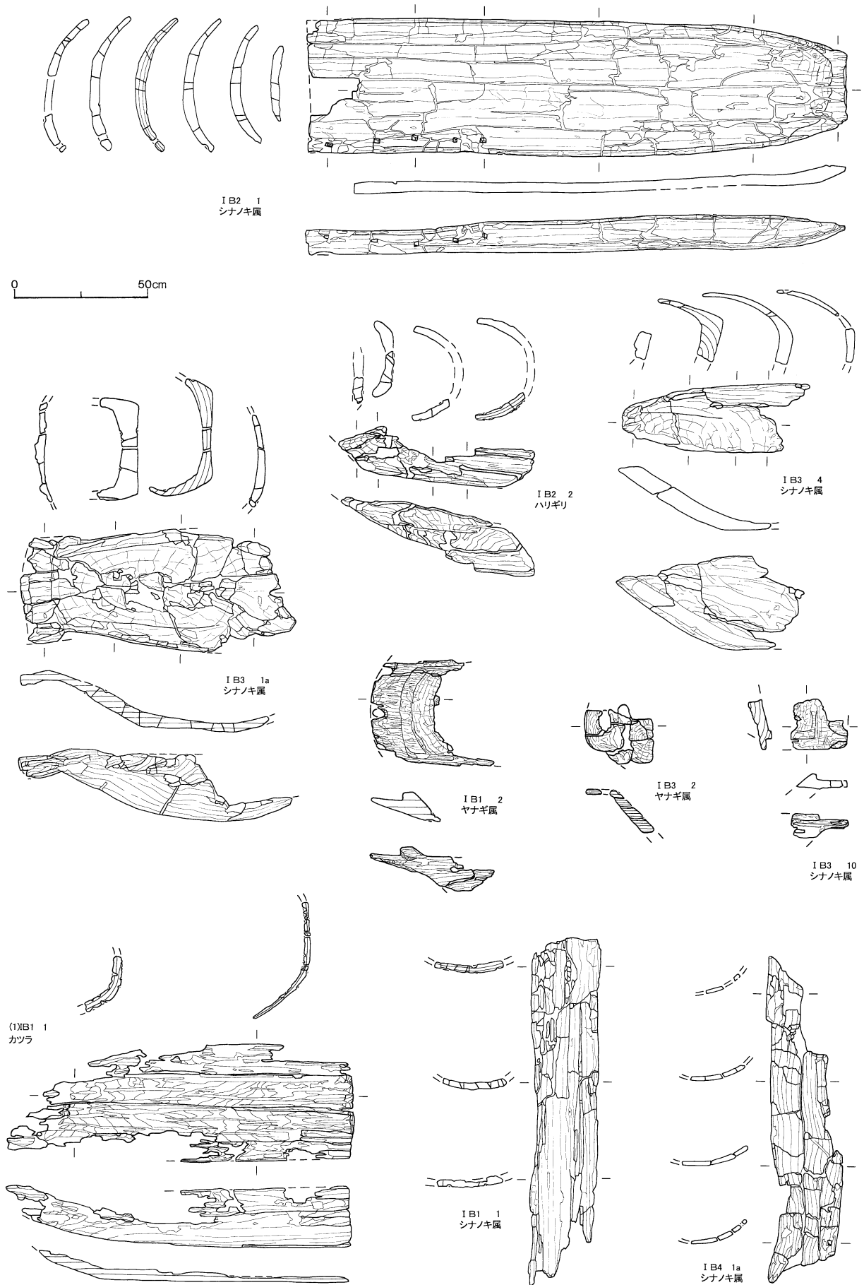
図 - 1 舟敷・舟材
