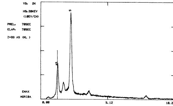
蒔絵加飾 (金彩) 石黄 (As 2 S 3 )
