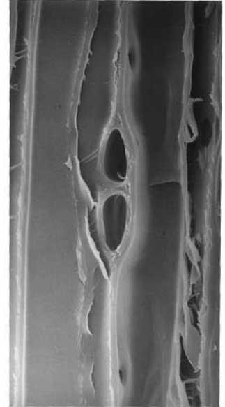
94 ヒノキの放射組織 b×860
