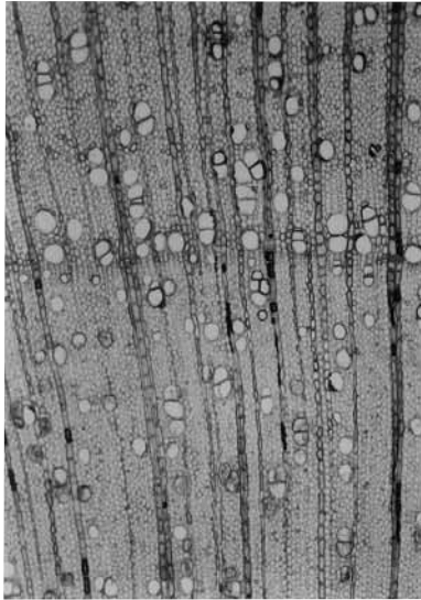
69 現生ヤマザクラの根材 a × 51.3
