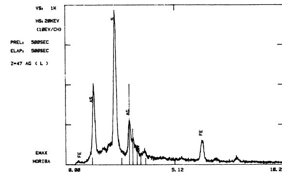
蒔絵加飾 (金彩) 銀+石黄 (Ag+As+S)
