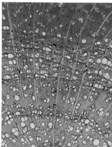
13 現生ハルニレの主幹材 a × 28
