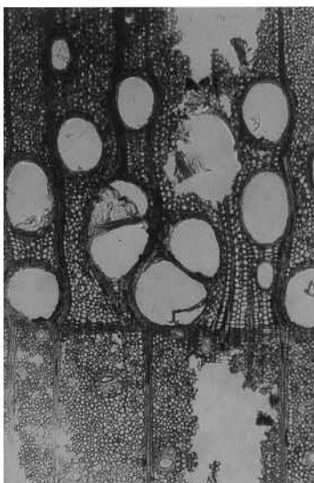
3 トネリコ属 木口面 X40
