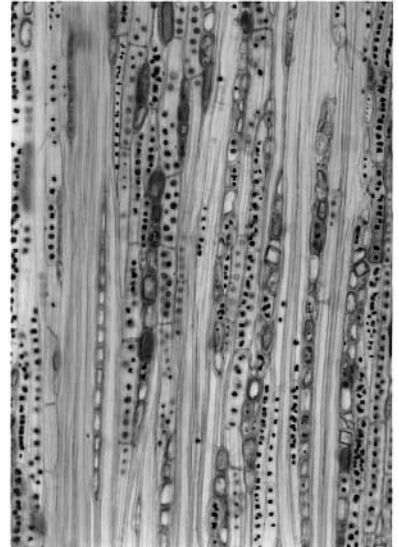
52 現生マテバシの根材 b × 20 5
