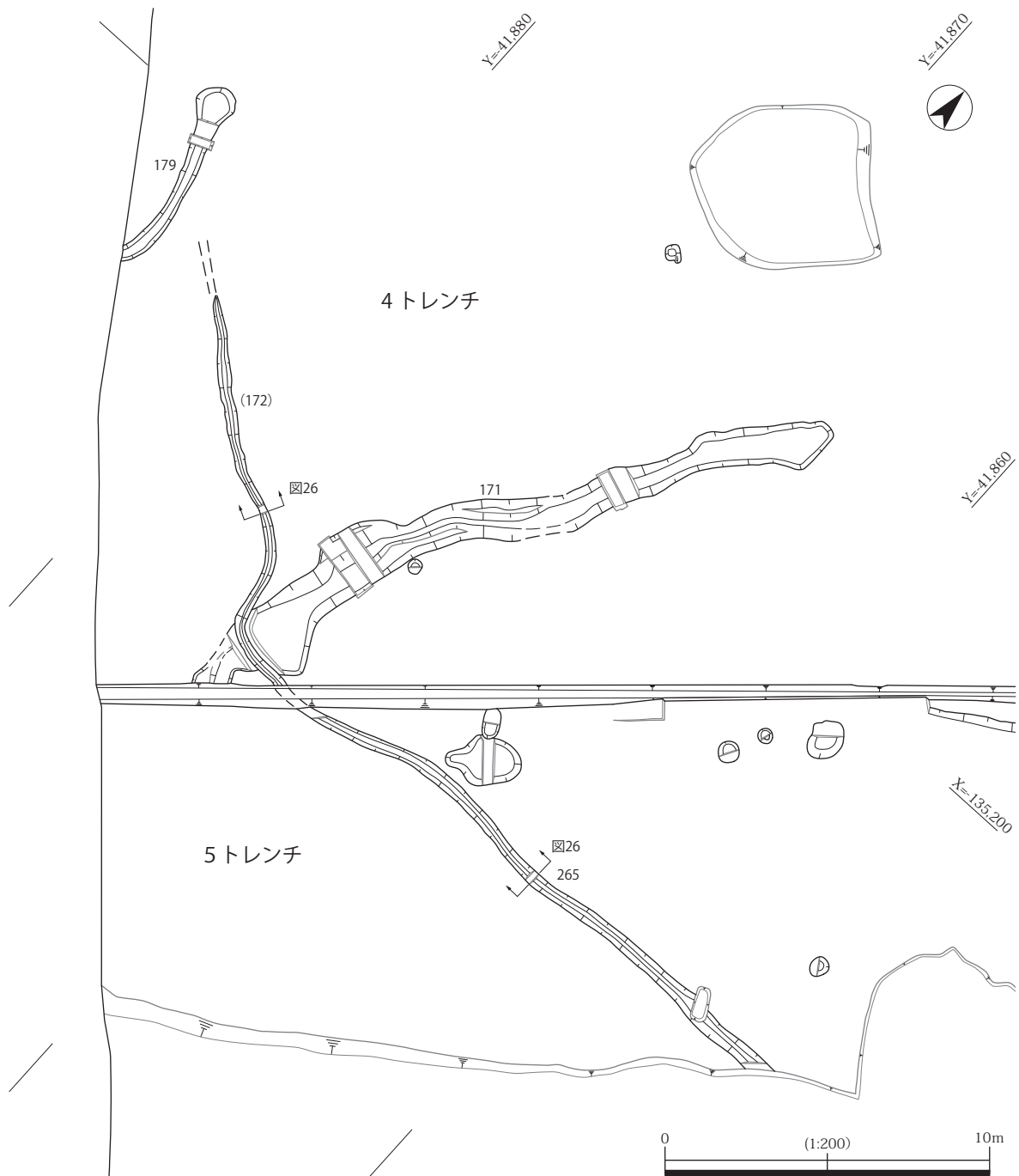
図 25 265 (172) 溝平面図
