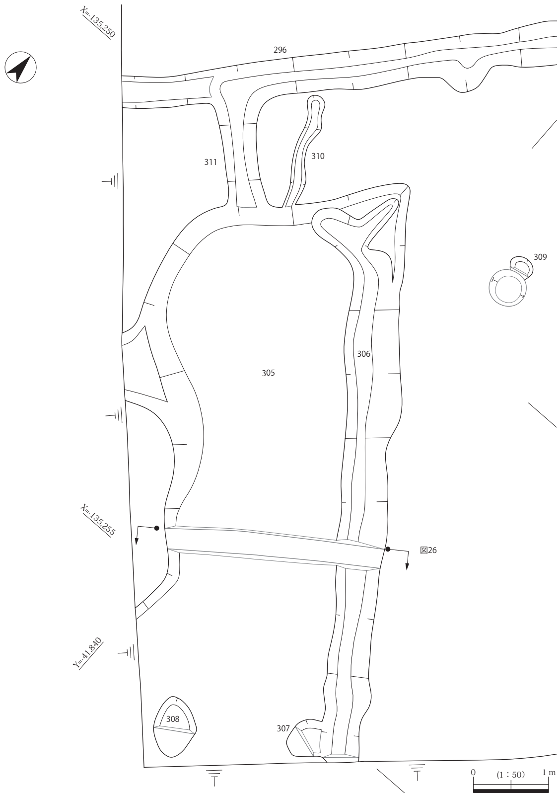
図 27 305 落込平面図
