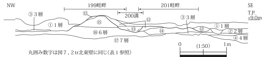
図 12 坪境断面図
