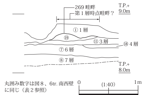
図 17 269 畦畔断面図
