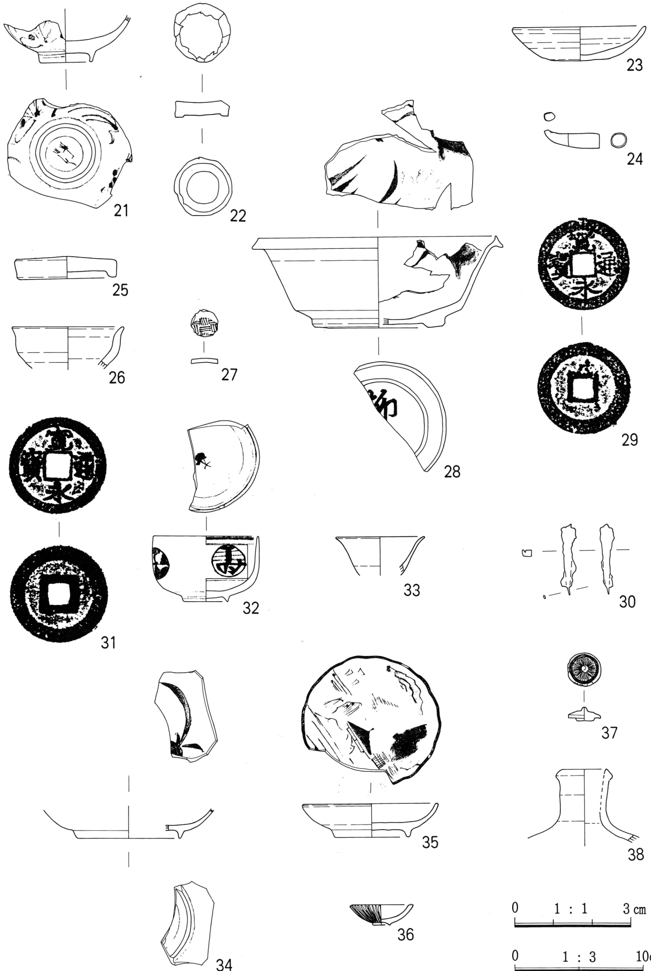
図版9 遺物実測図 (29・31は原寸、他は1/3)
