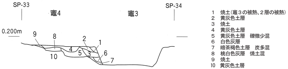
竈3、竈4断面図(1:20)
