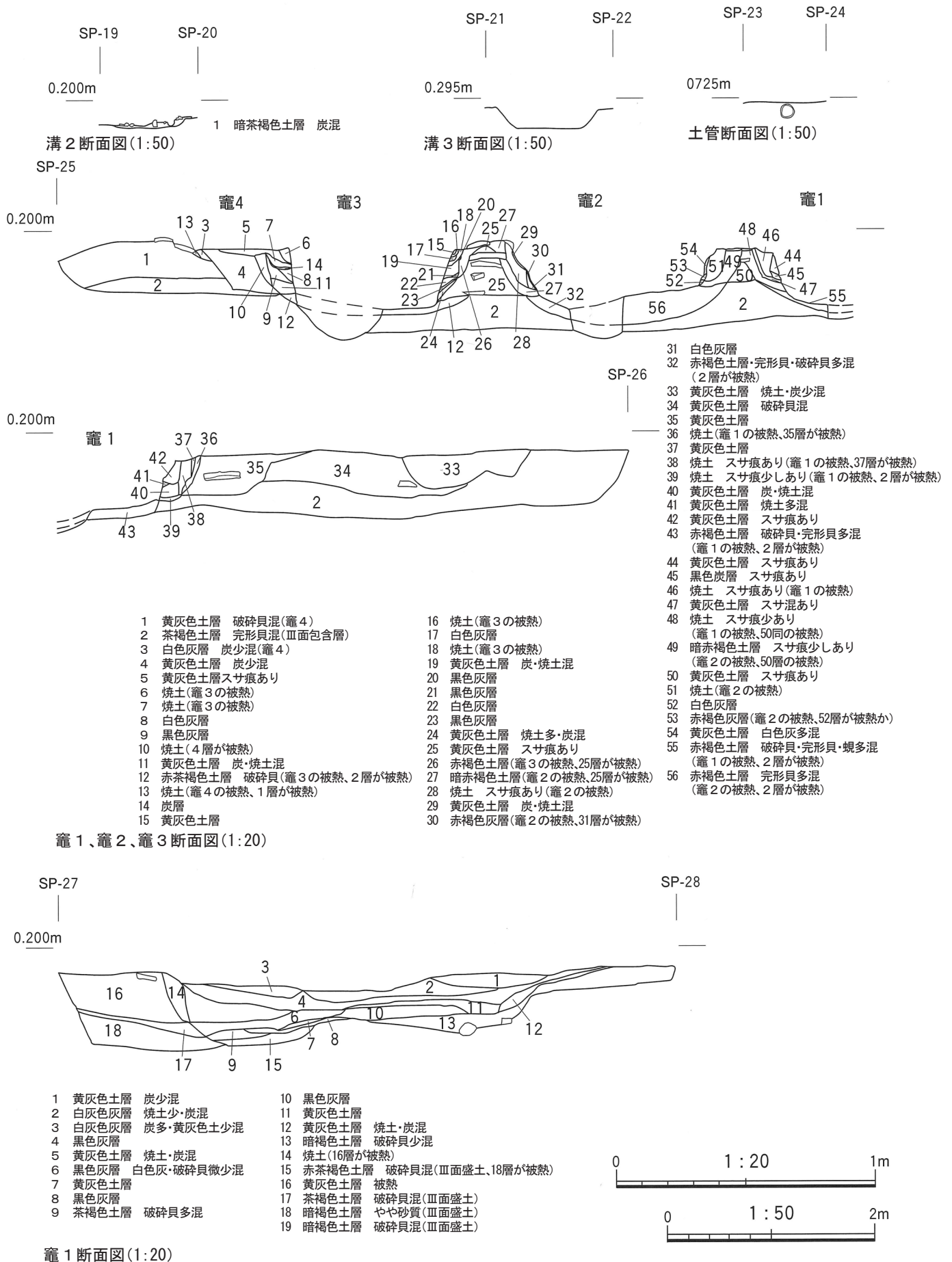
図版 4 Ⅲ面断面図
