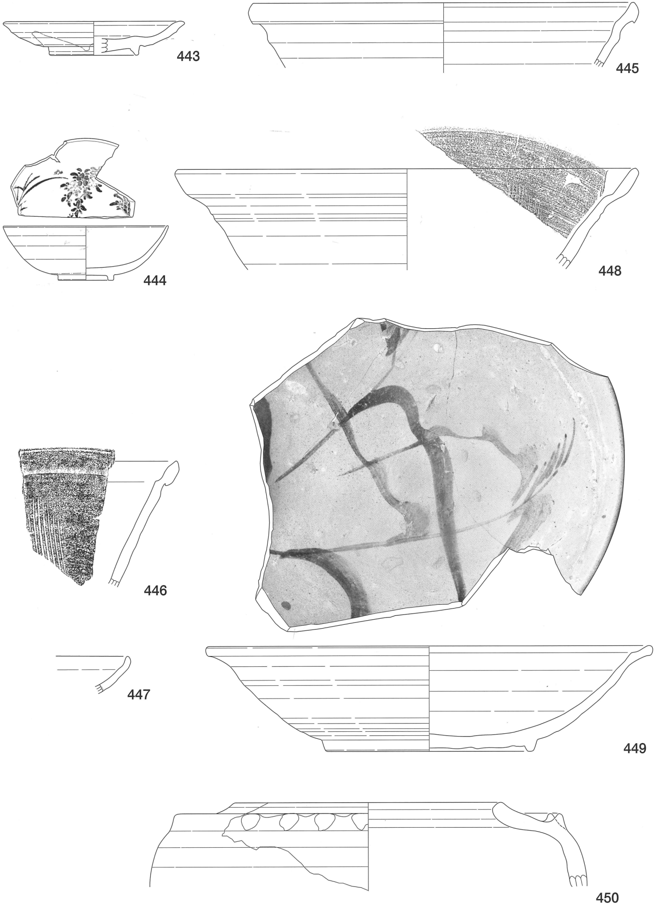
図版40 遺物実測図(1/3)
