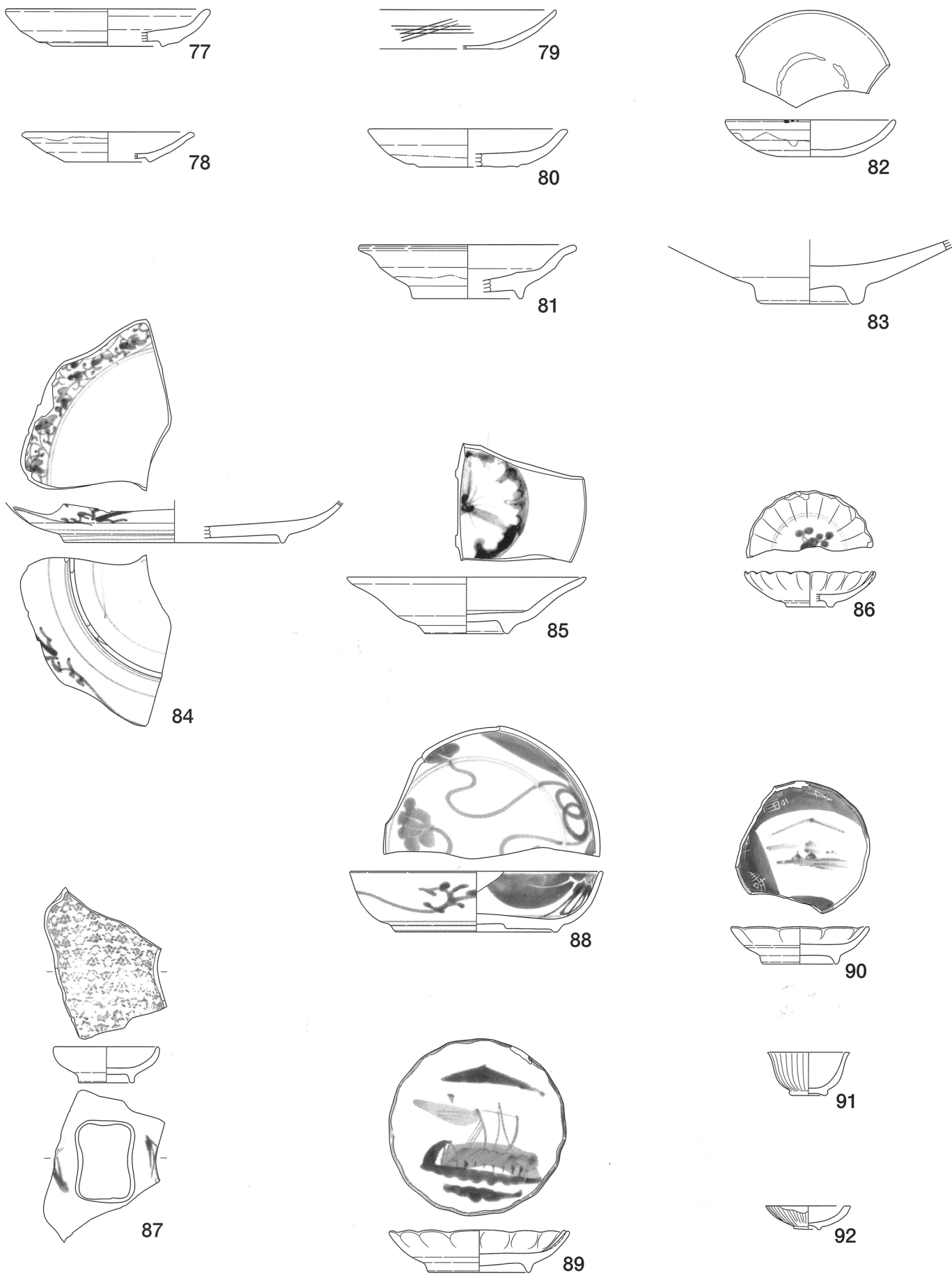
图版15 遺物実測図(1/3)
