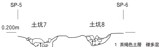
土坑7、土坑8断面図(1:50)
