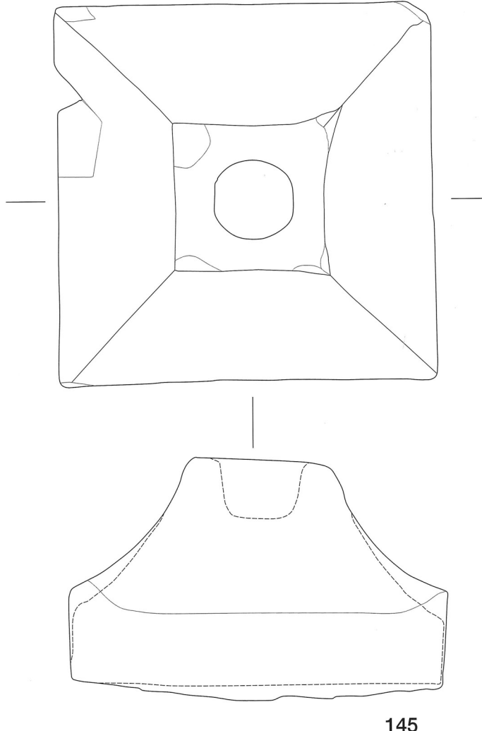
図版20 遺物実測図(137・139・140・141・142・144は原寸、他は1/3)
