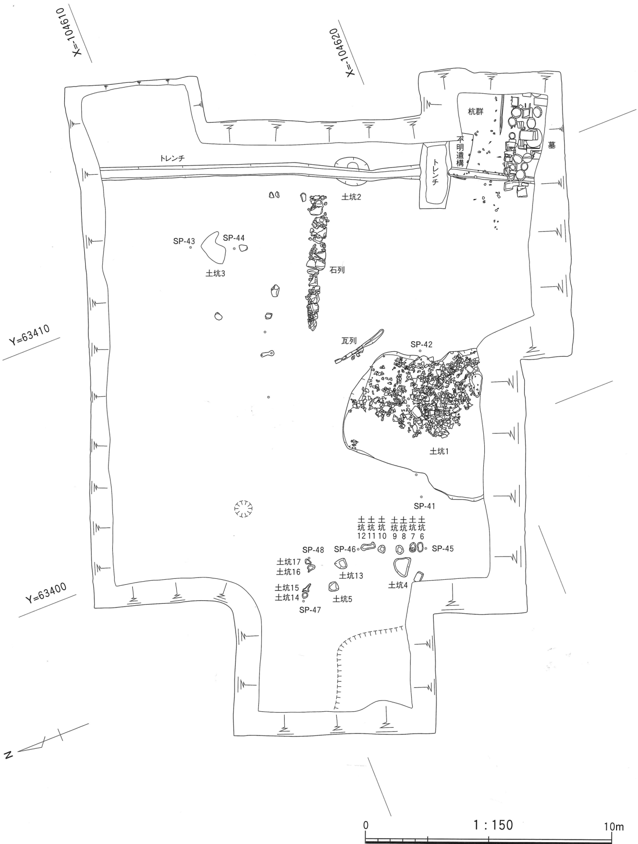
図版7 IV面平面図(1:50)
