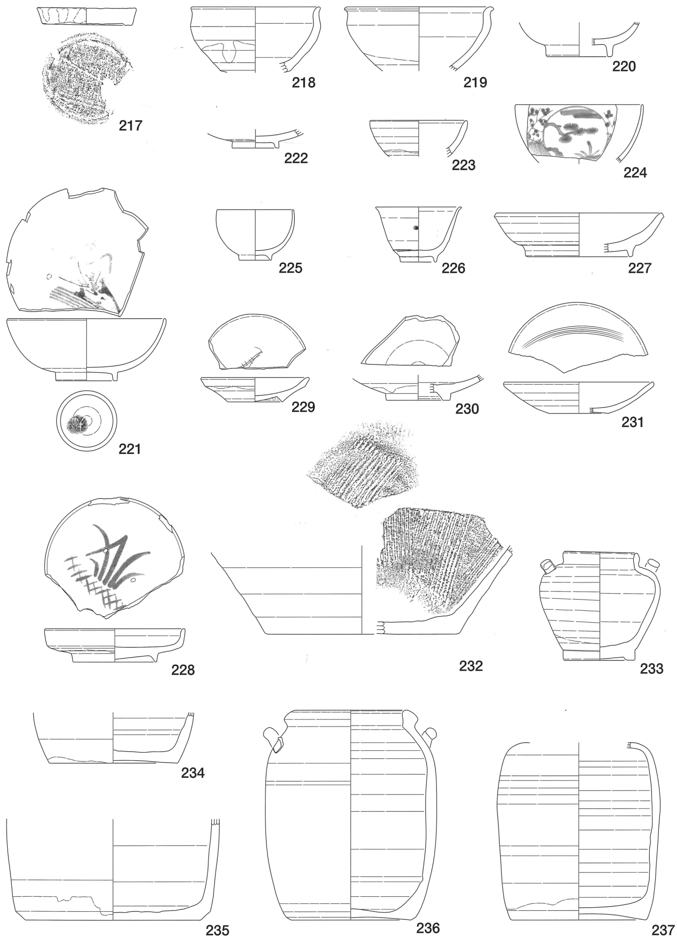
図版26 遺物実測図(1/3)
