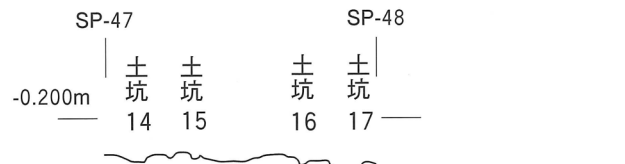
IV面 土坑14・土坑15・土坑16・土坑17断面図(1:50)
