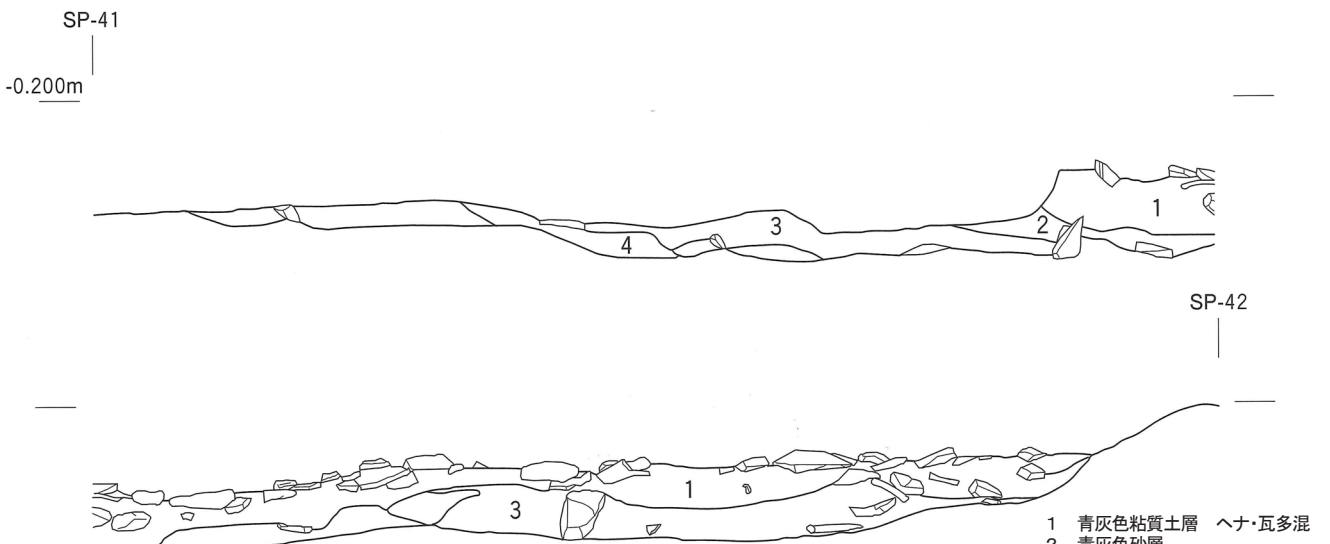
IV面 土坑1断面図(1:20)
