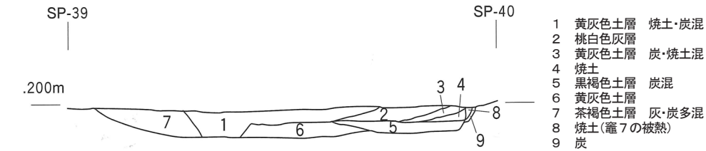
III面 竈7断面図(1:20)
