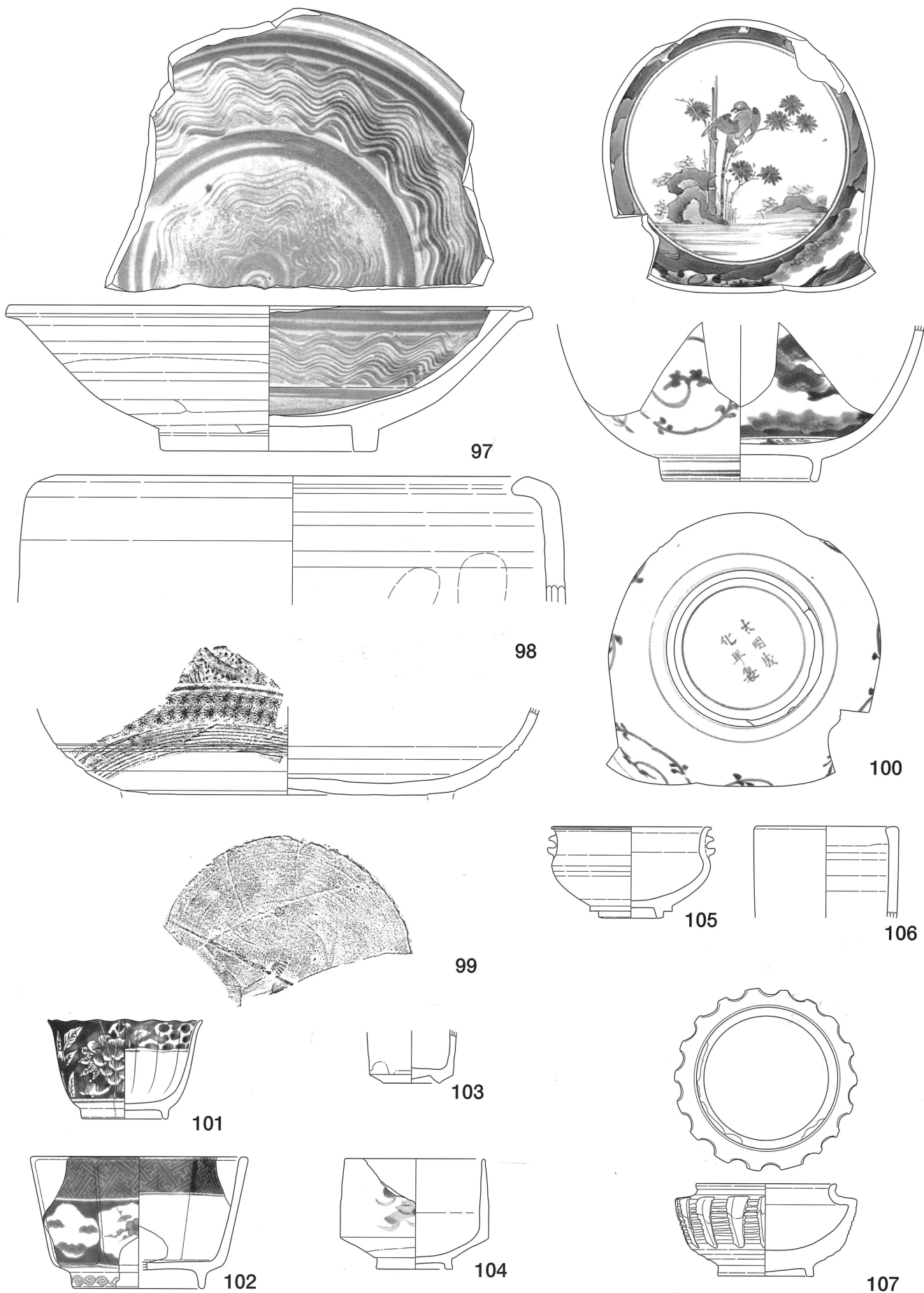
图版17+ 遺物実測図(1/3)
