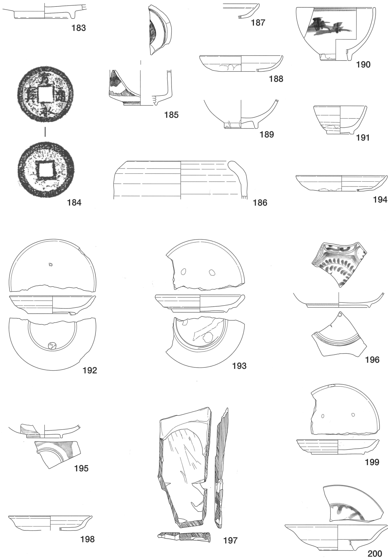
図版23 遺物実測図(184は原寸、他は1/3)
