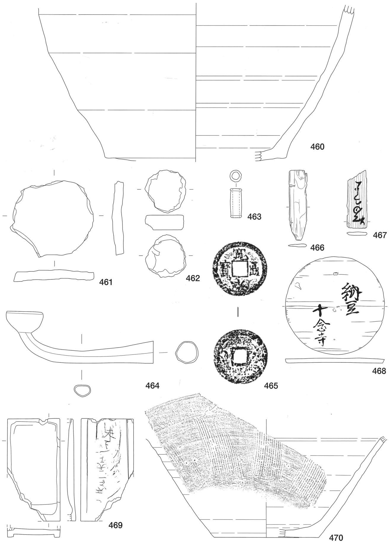
図版42 遺物実測図(464・465は原寸、他は1/3)
