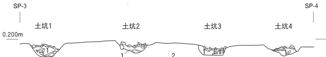
土坑1、土坑2、土坑3、土坑4断面図(1:50)
