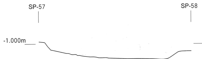
土坑 3 断面図(1:50)
