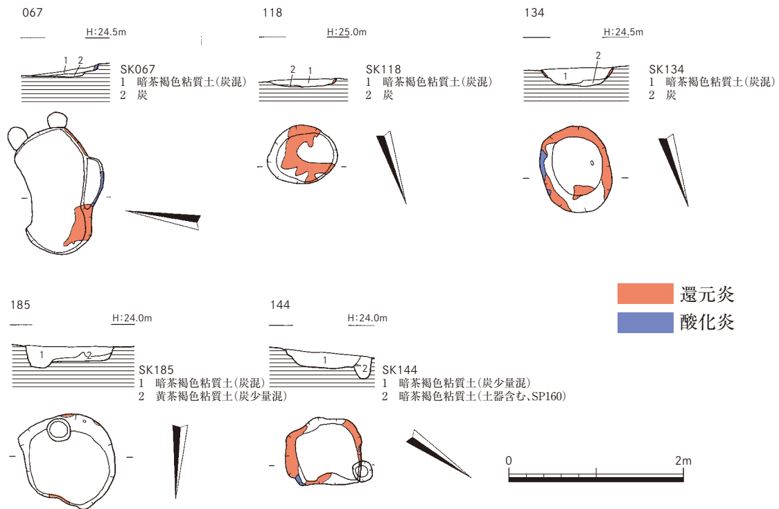
第9 図 SK067・118・134・144・185 実測図 (1/60)
