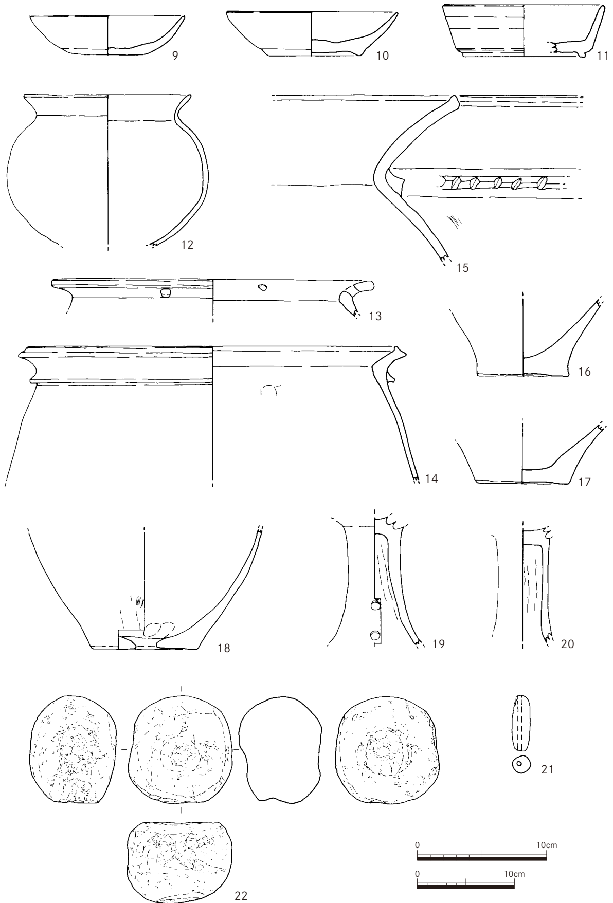
第12図 包含層出土遺物実測図 (14は1/2、他は1/3)
