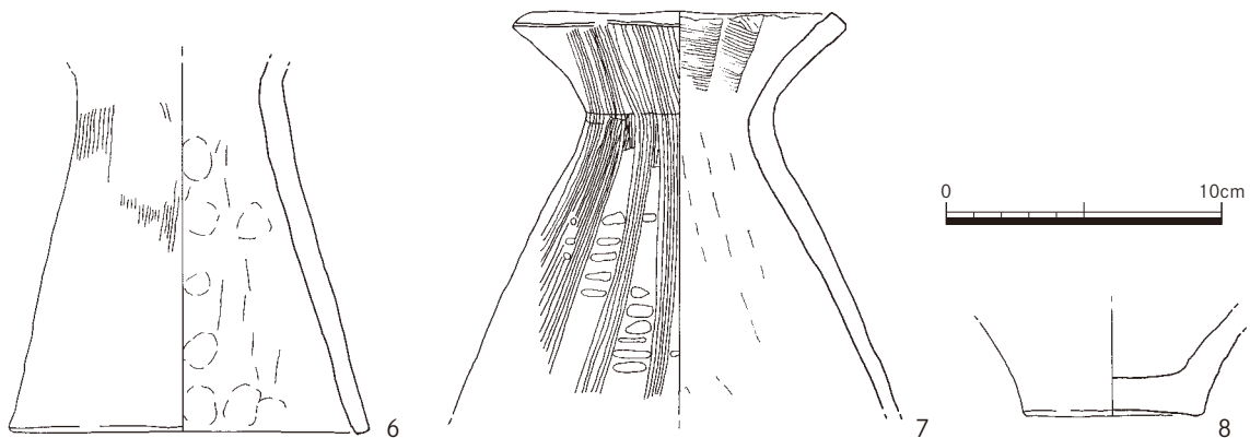
第10 図 ピット出土遺物実測図 (1/3)
