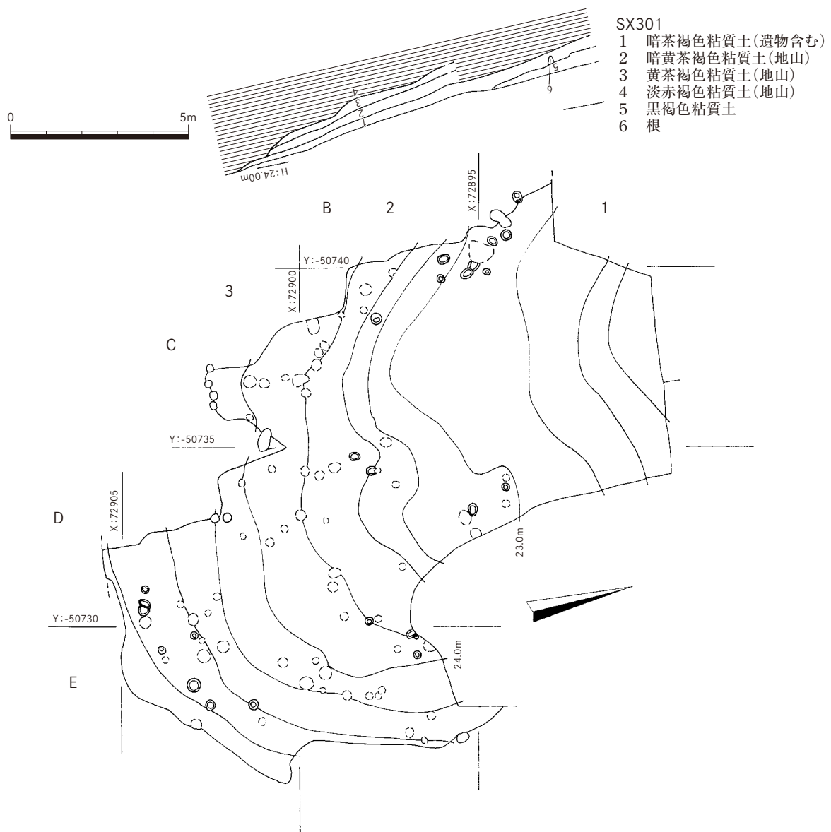
第11図 調査区2面全体図(1/150)
