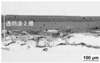
写真4 漆塗膜構造
