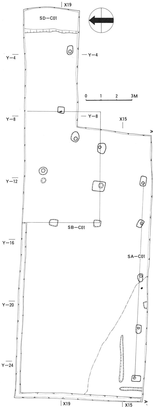
C区 遺構平面図(長岡京期)
