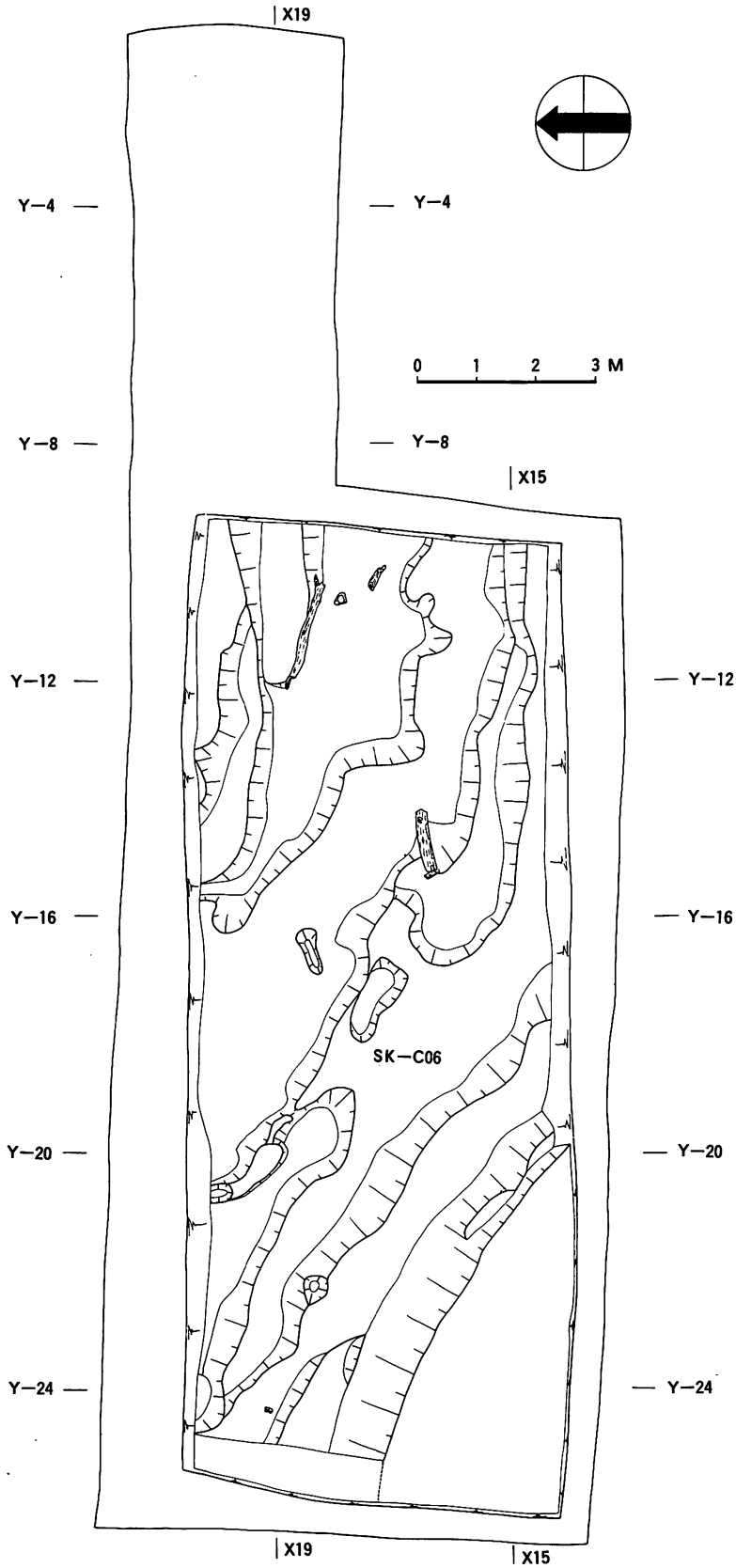
C区 遺構平面図 (長岡京期以前)
