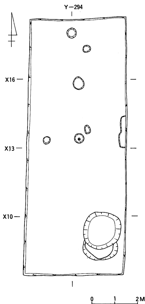
図4 試掘1 平面図
