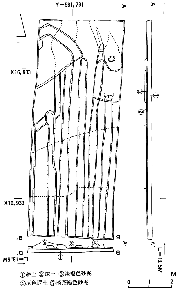
図9 試掘6 平面図
