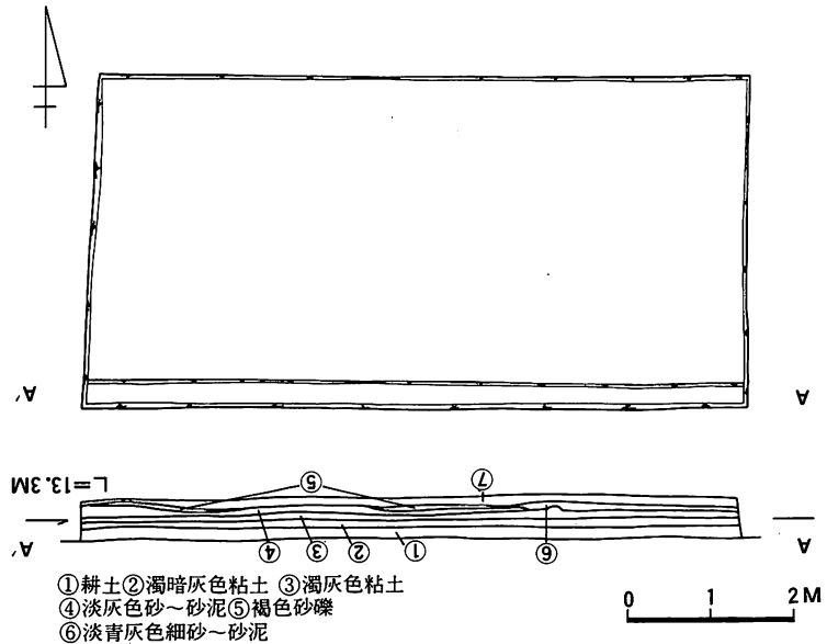
図11 試掘8 平面図
