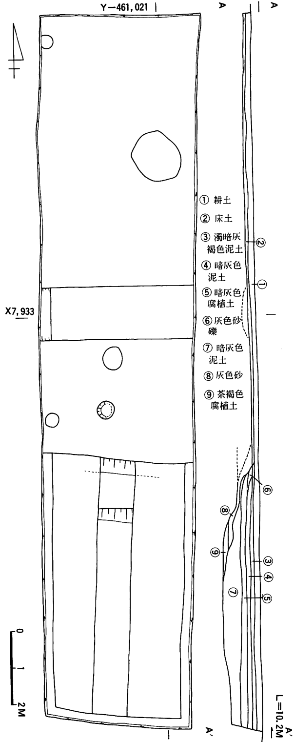
図6 試掘3 平面図
