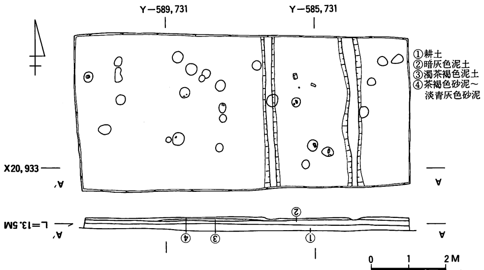
図10 試掘7 平面図
