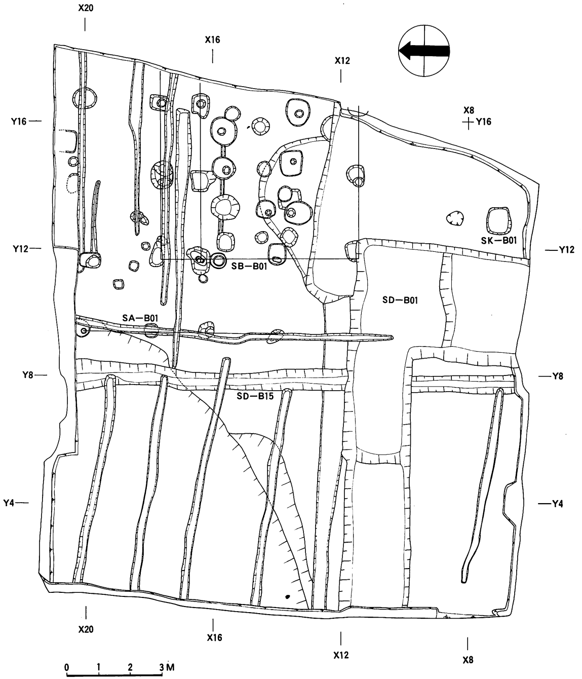
B区 遺構平面図（長岡京期）
