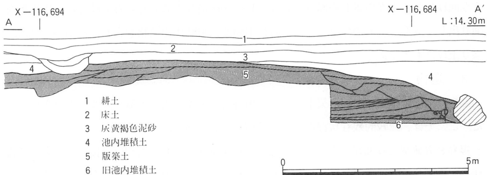
图17 西壁断面图
