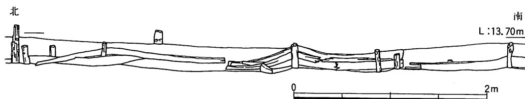
図9 SX4 立面図
