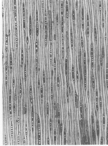
杭98 モミ板目(×40)
