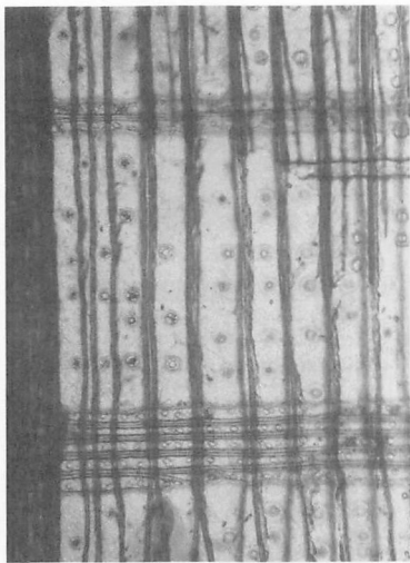
杭47 スギ柁目(×100)
