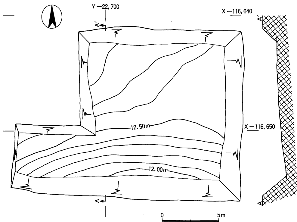
図3 遺構実測図
