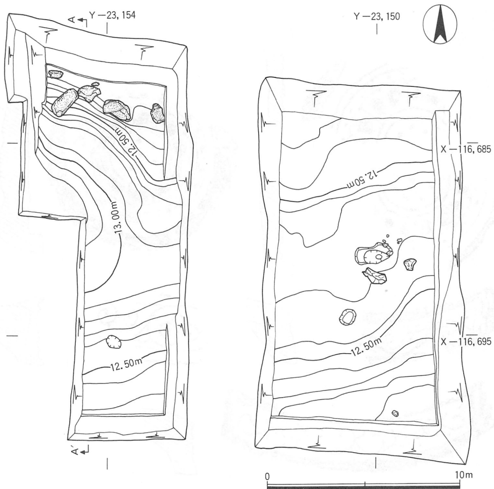
图16 遗构实测图
