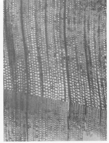
杭67 ツガ木口(×40)
