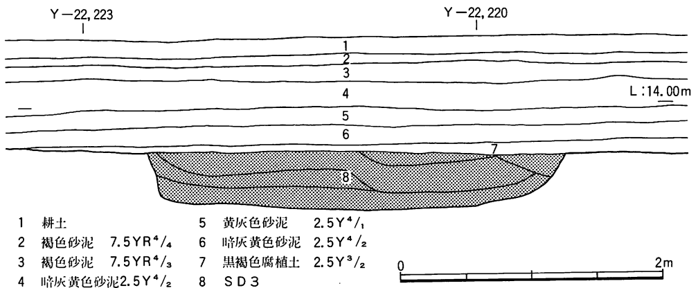
図8 北壁断面図
