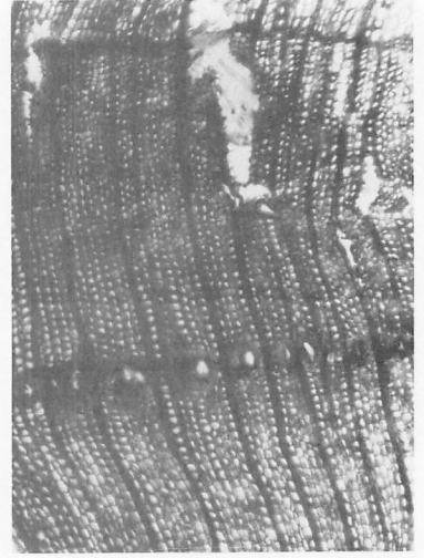
杭98 モミ木口(×40)
