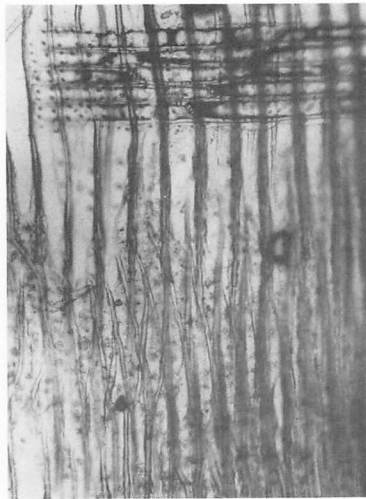
杭67 ツガ柎目(×100)
