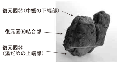
第26図 中甑・結合部・湯だめ接合資料（実測番号 0173）
