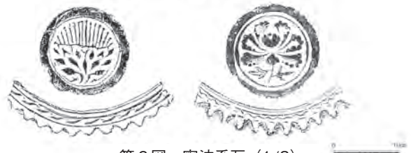
第6図 寧波系瓦（1/8）
