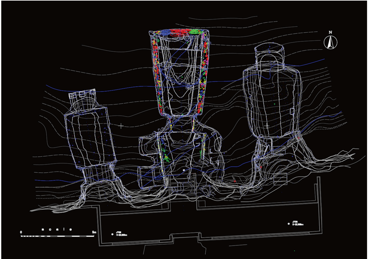
直牒洞三窟平面图
