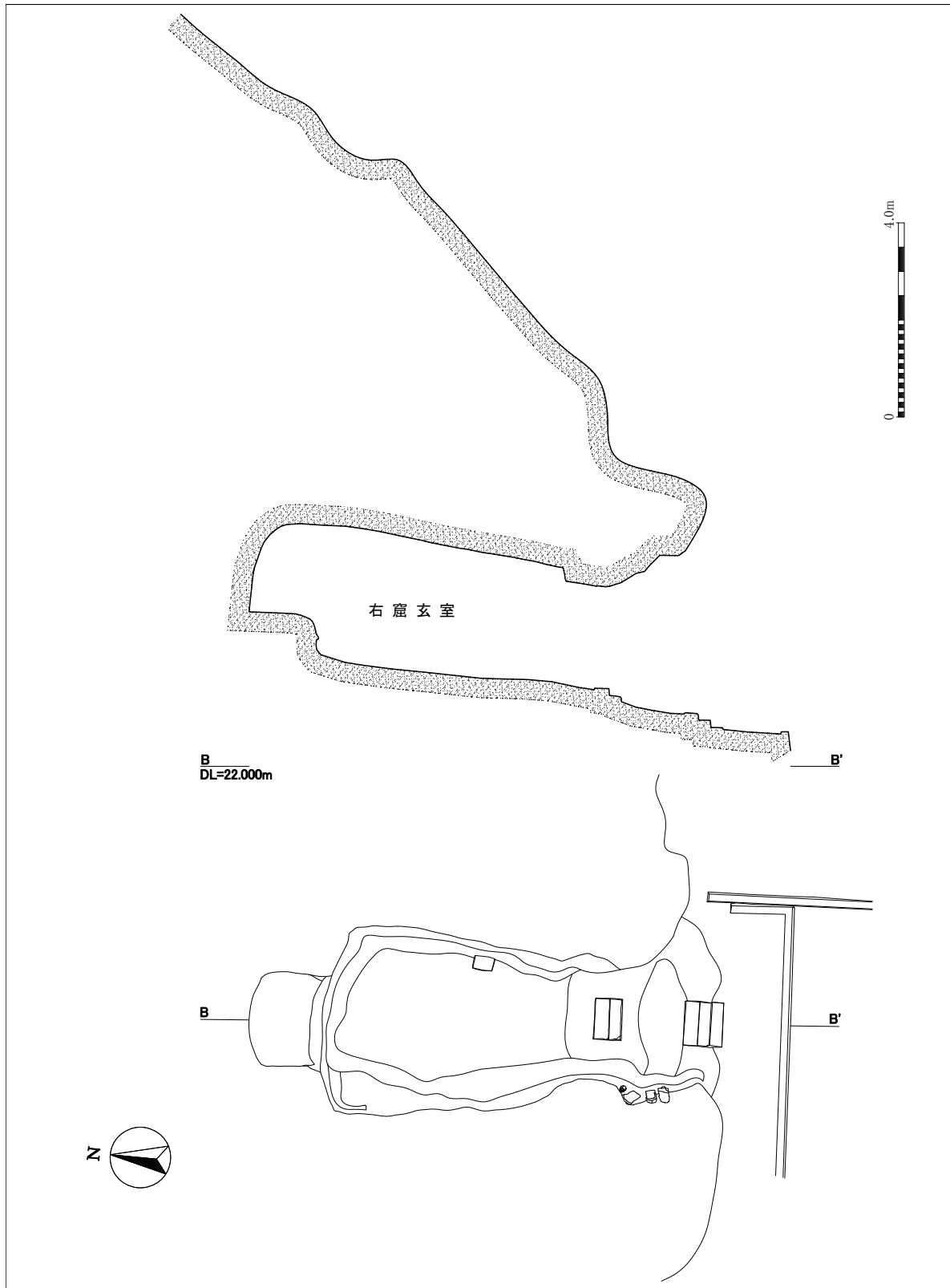
第3-8図 右窟と地形エレベーション図
