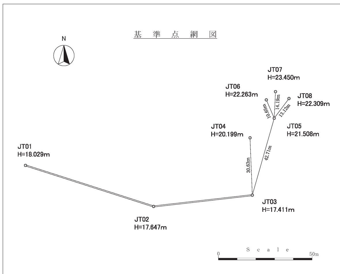
第3-2図 基準点網図
