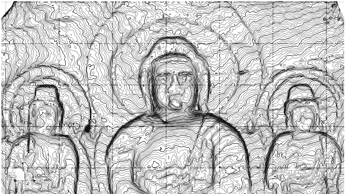
第3-40図 3次元等高線図 (阿弥陀三尊拡大)
