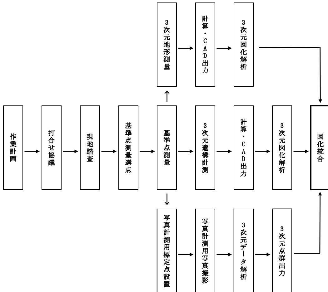
第3-1図 直牒洞測量・計測調査フロー
