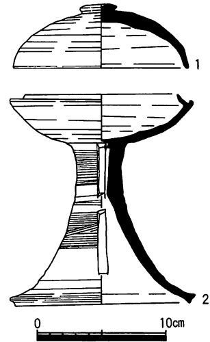
図3 4号墳出土土器
