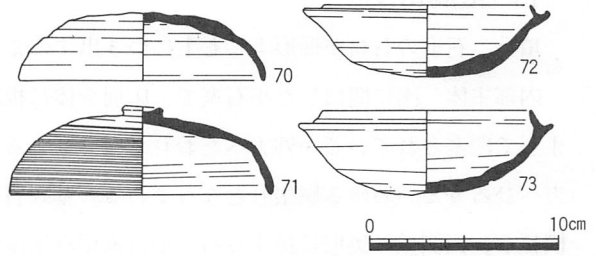
図18 17号墳出土土器
