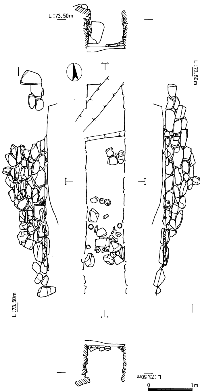
図6 9号墳石室実測図
