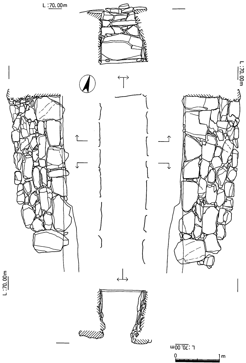
图14 13号填石室实测图
