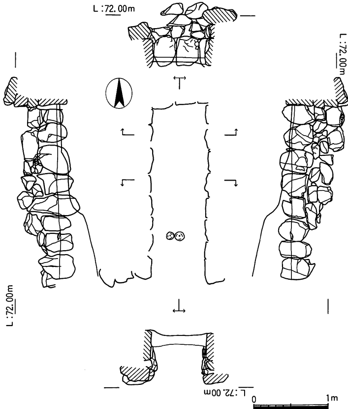
図22 20号墳石室実測図
