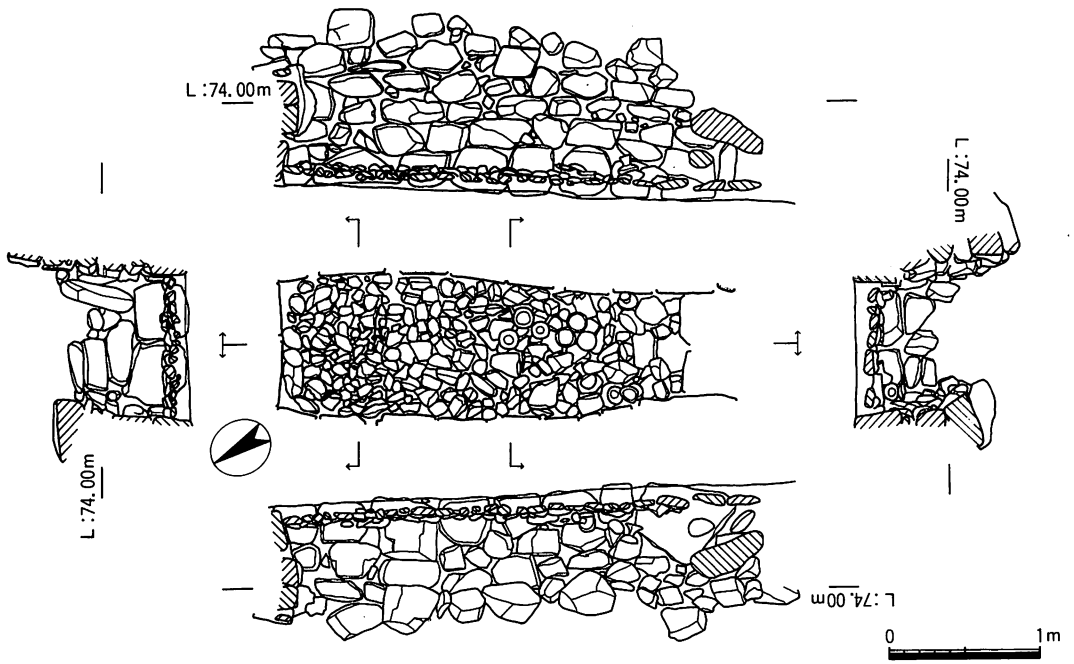
图4 8号墳石室实测图
