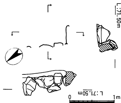
図20 19号墳石室実測図
