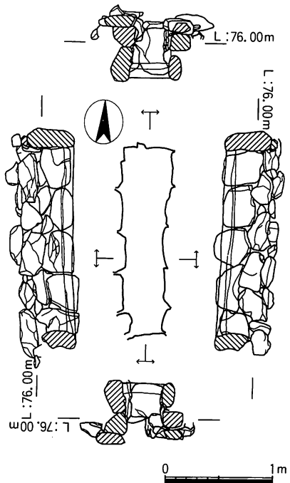
図2 醍醐3号墳石室実測図
