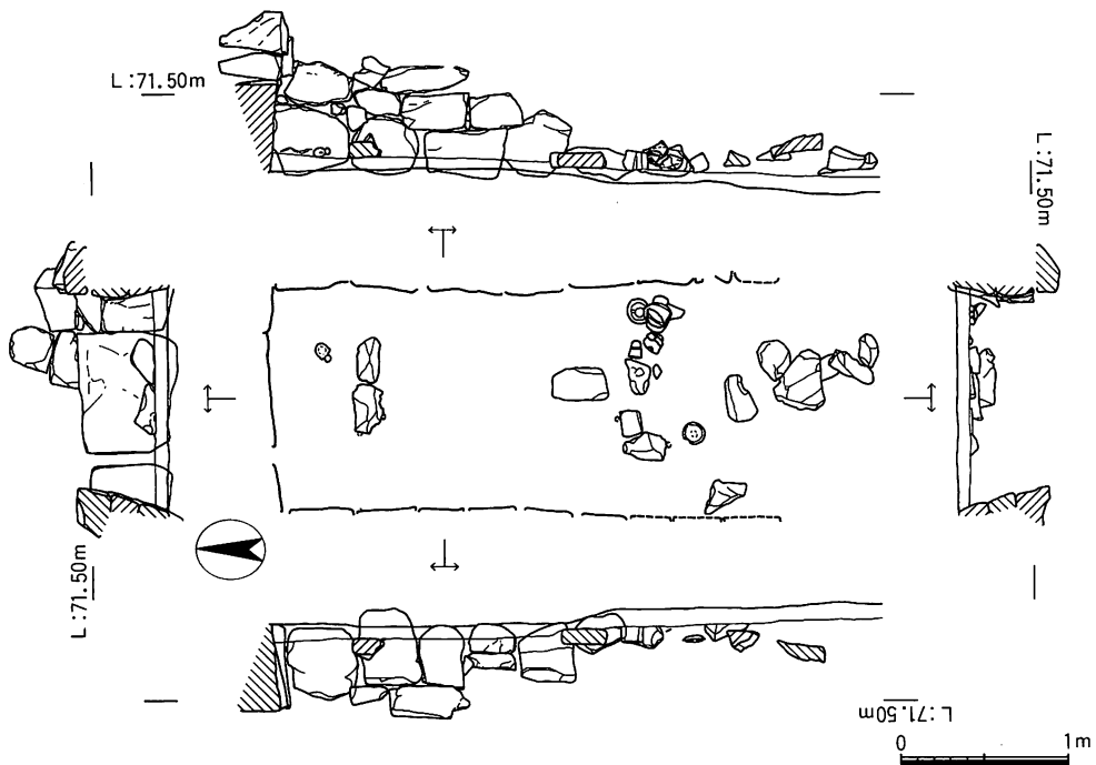
図12 12号墳石室実測図
