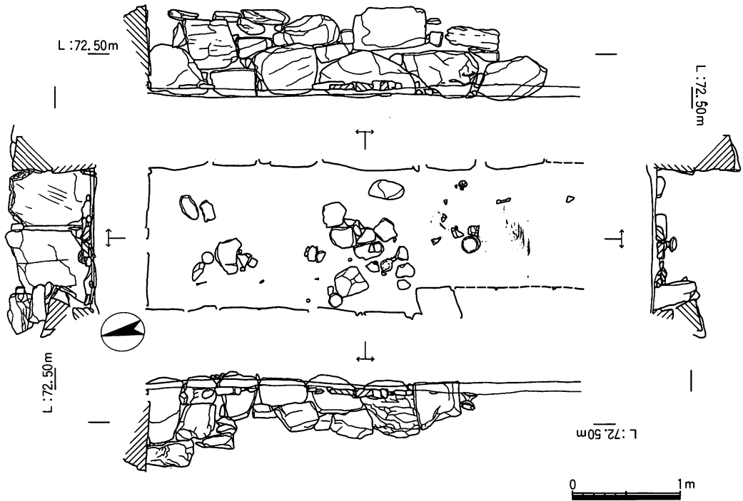
図8 10号墳石室実測図
