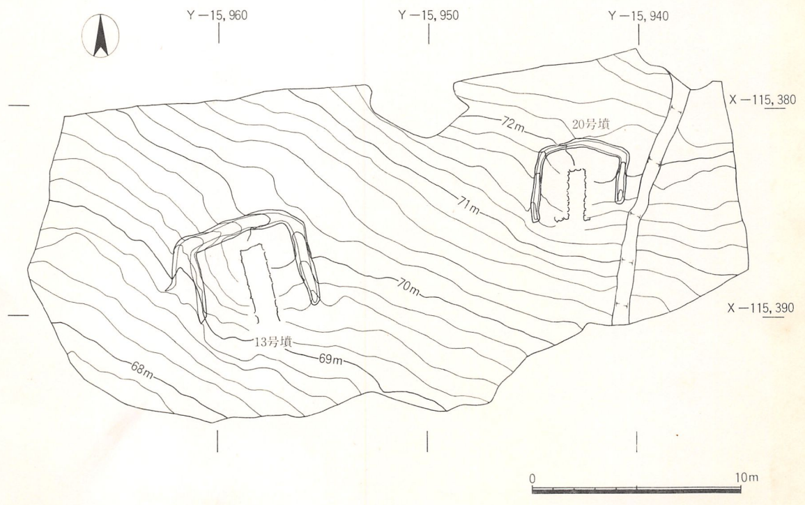
2 西拡張区地形測量図 (1:250)
