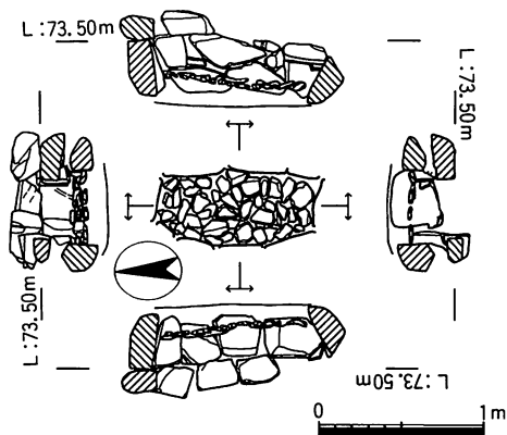
図19 18号墳石室実測図
