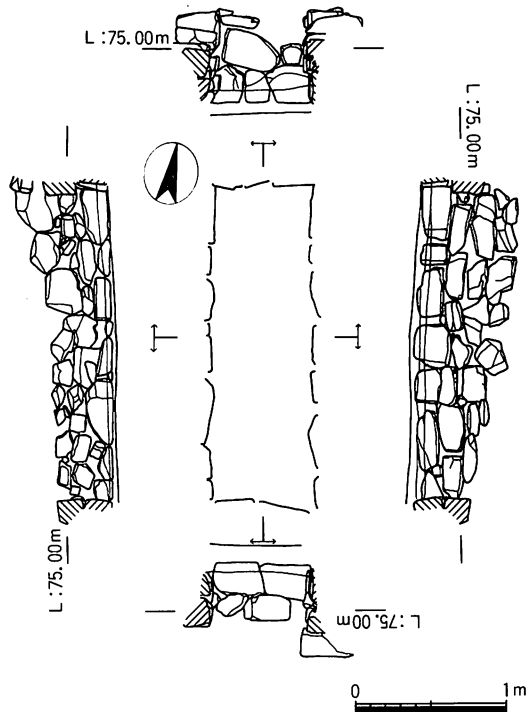
図17 16号墳石室実測図
