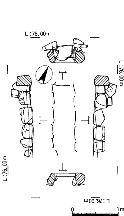
図16 15号墳石室実測図
