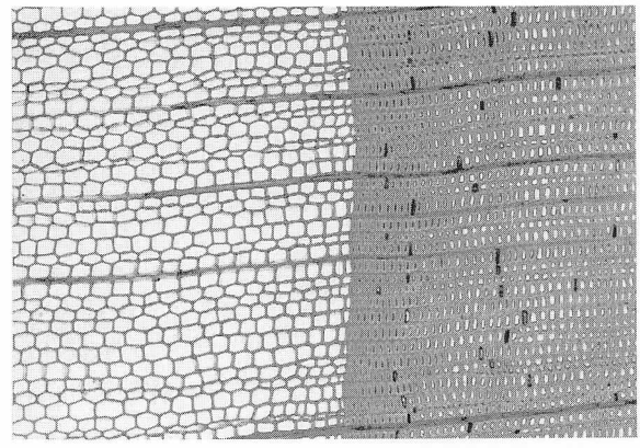
木口面の光学顕微鏡写真
