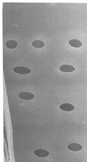
柱目面の光学顕微鏡と走査電子顕微鏡写真
