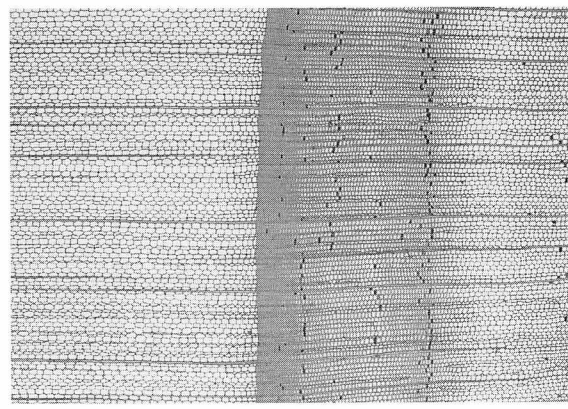
木口面の光学顕微鏡写真
