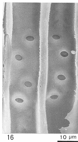
柁目面の光学顕微鏡と走査電子顕微鏡写真
