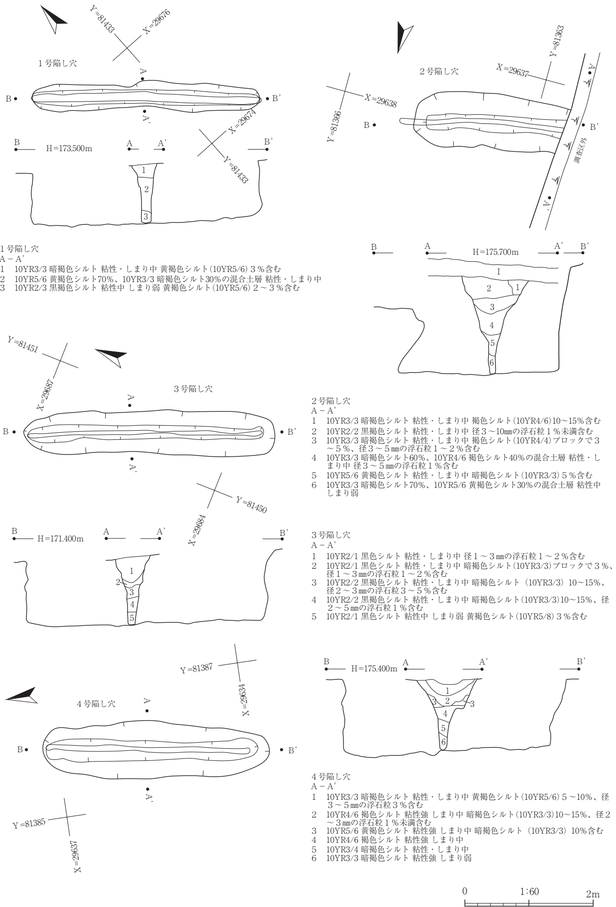
第5図 1~4号陥し穴状遺構
