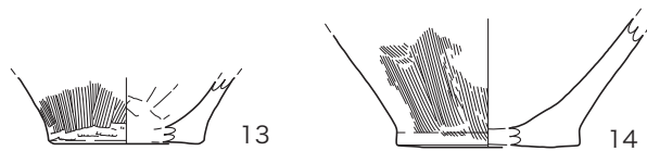
図9 遺物実測図 (1:4)
