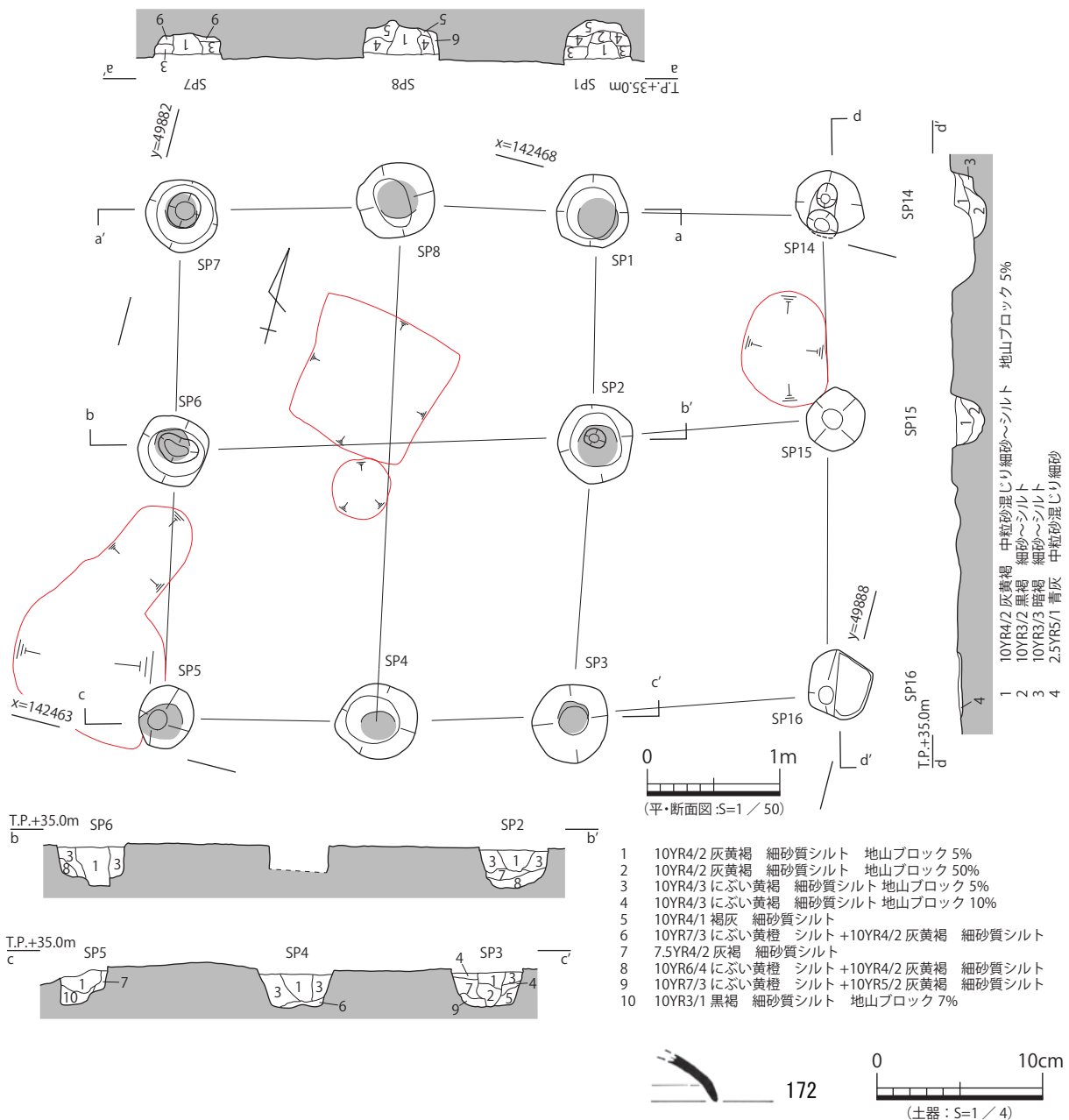
図68 9-掘立1 平・断面図、出土遺物実測図
