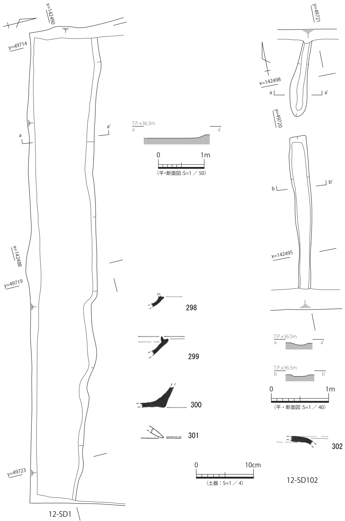
図 111 12-SD 1・102 平・断面図、出土遺物実測図
