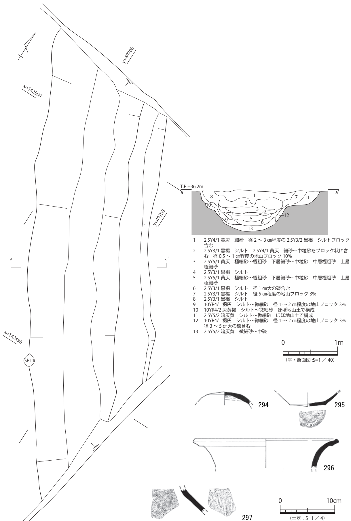
図 110 11-SD 1 平・断面図、出土遺物実測図
