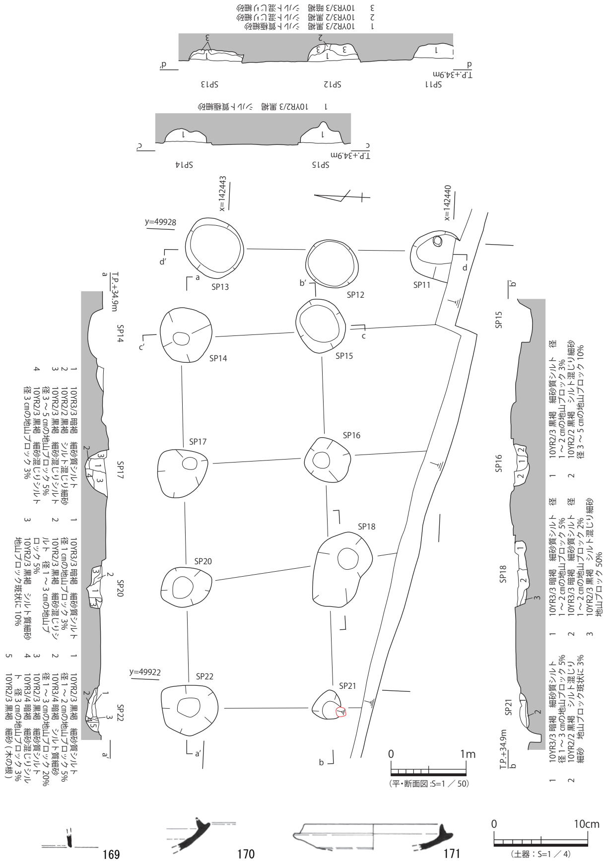
図 66 2・5-掘立6 平・断面図、出土遺物実測図
