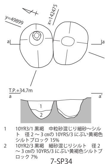
図 93 1-SP25、4-SP41、7-SP34、15-SP 2 平・断面図、出土遺物実測図
