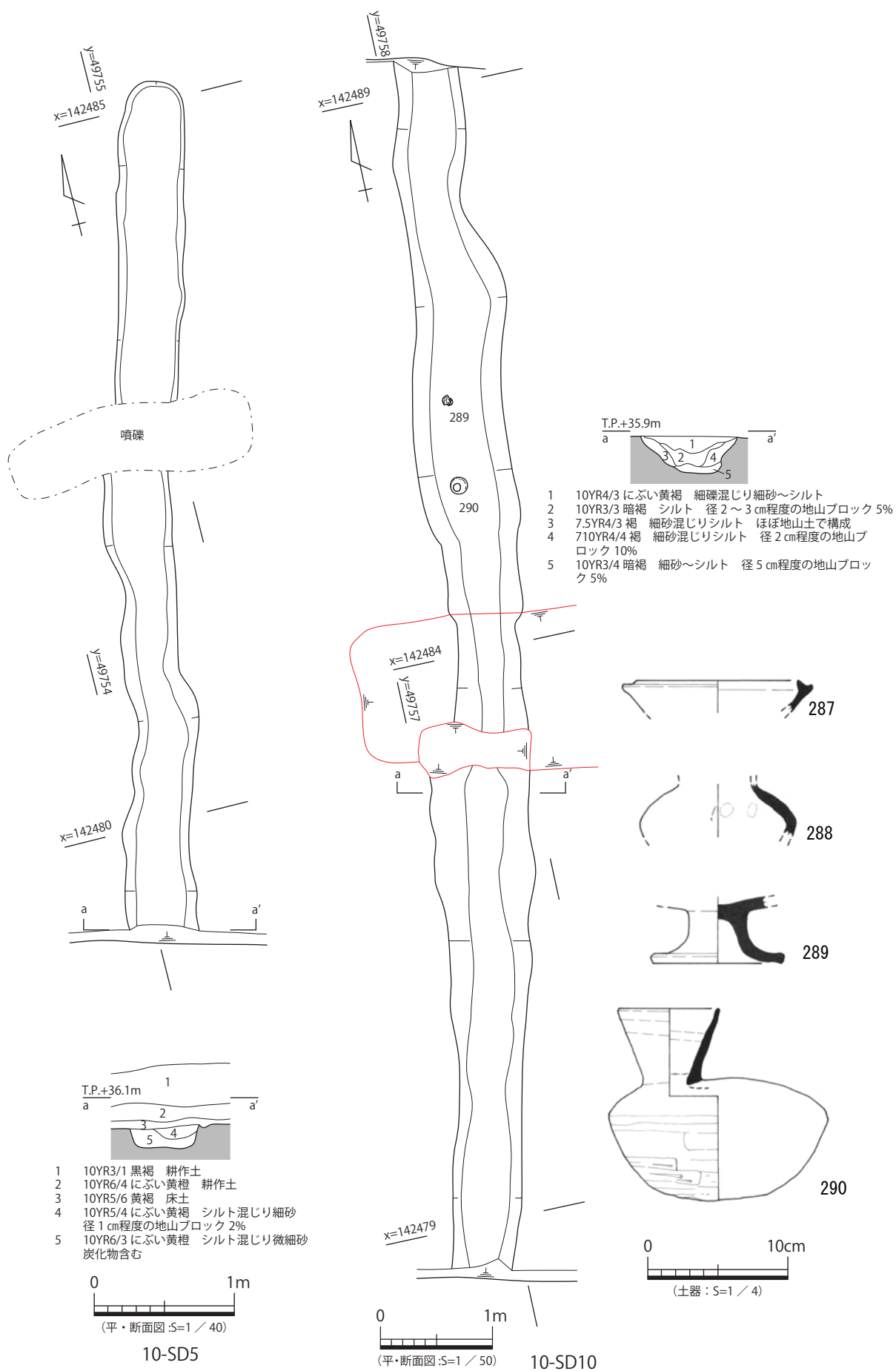
図 108 10-SD 5・10 平・断面図、出土遺物実測図
