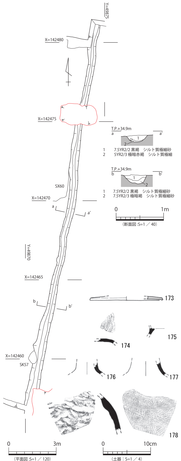
図 70 1・16-SD20 平・断面図、出土遺物実測図
