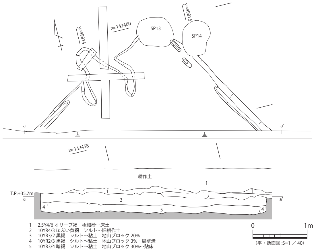
図5 26- 竖穴 45 平・断面図
