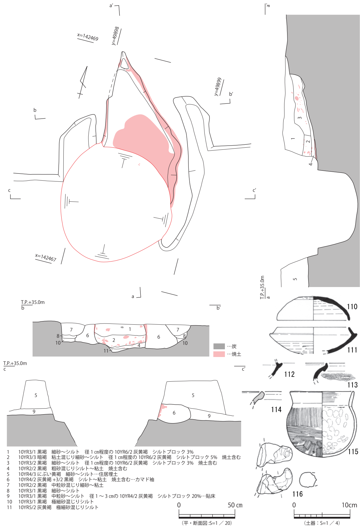
図 49 7- 竖穴 11 カマド 平・断面図、出土遺物実測図
