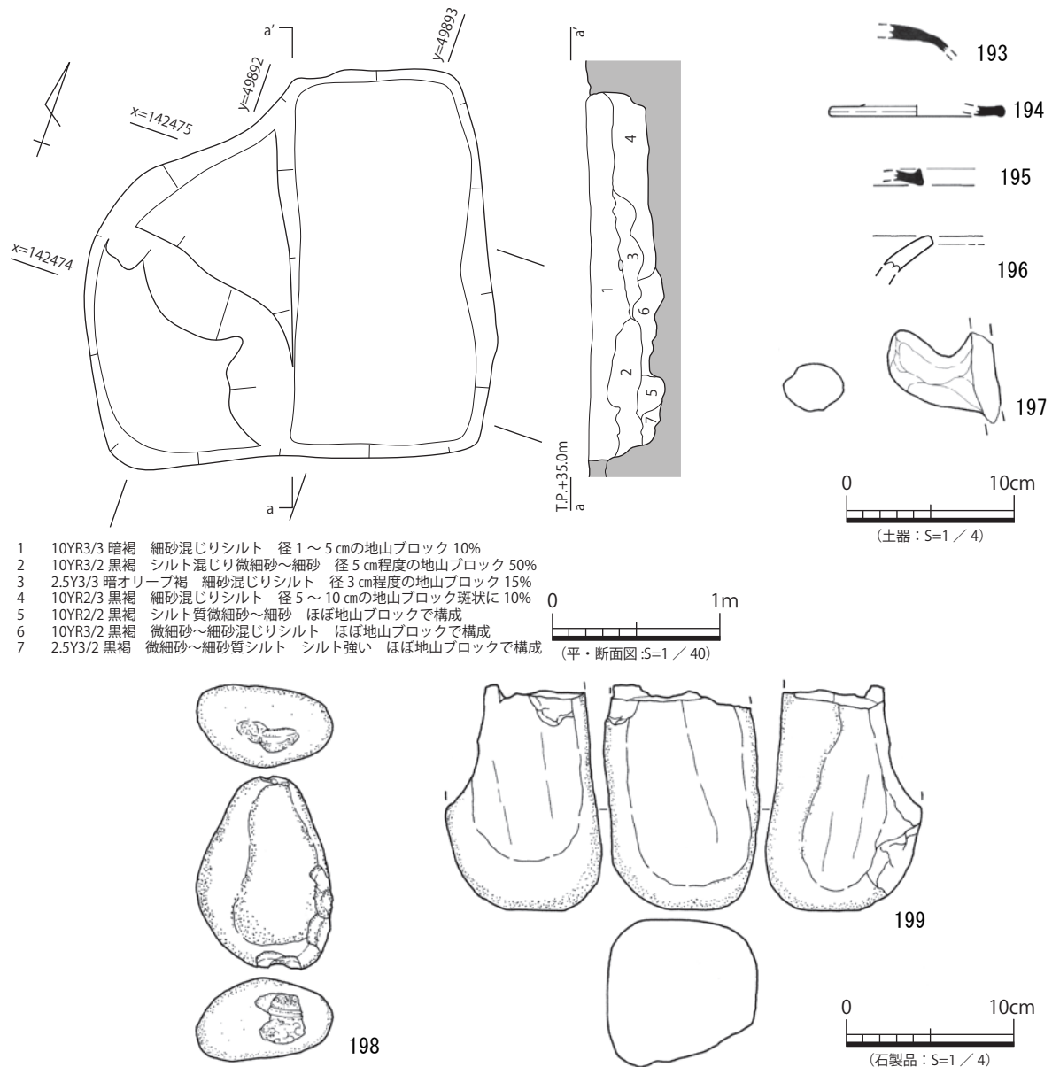
図 87 7-SK23 平・断面図、出土遺物実測図
