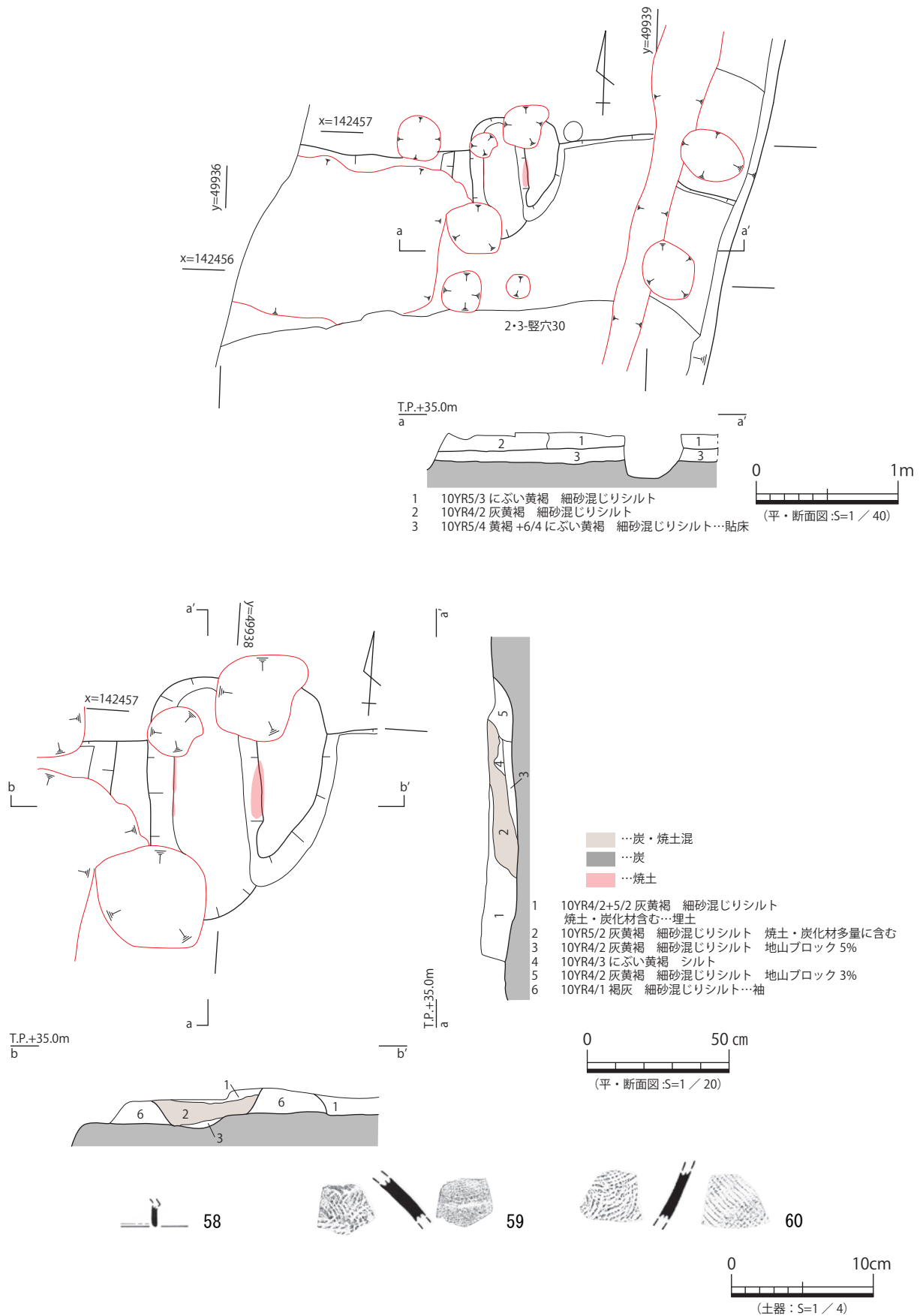
図 30 3- 竪穴 100 平・断面図、カマド 平・断面図、出土遺物実測図
