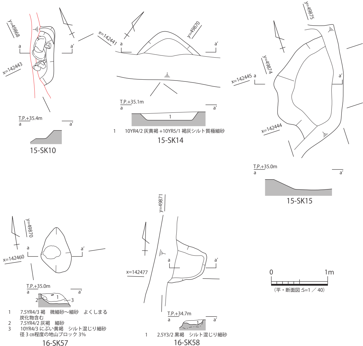
図 92 15-SK10・14・15、16-SK57・58 平・断面図
