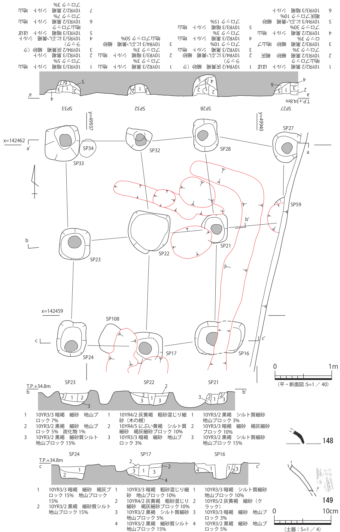
図 62 4-掘立3 平・断面図、出土遺物実測図
