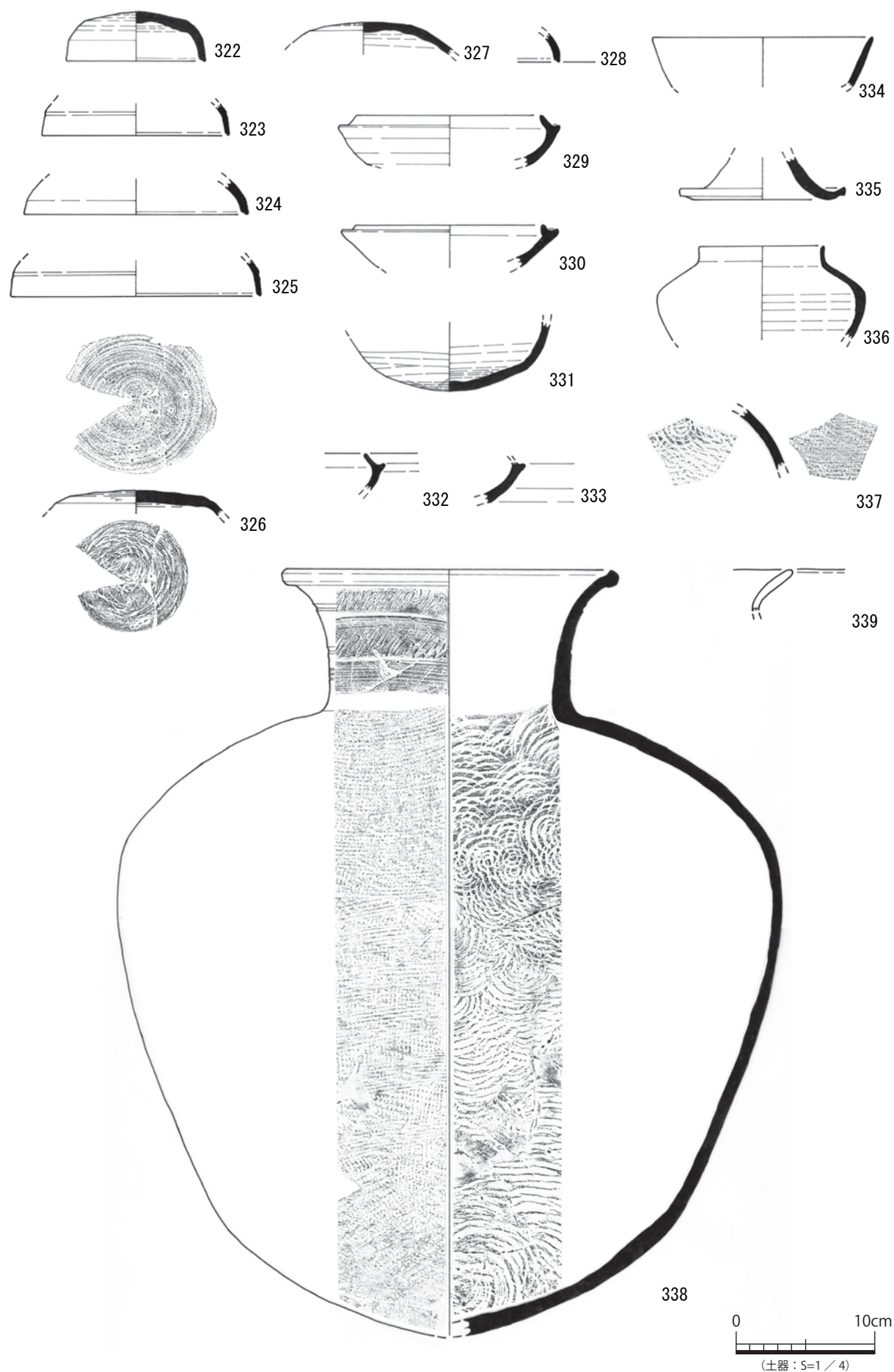
図 119 12-SX 2 出土遺物実測図
