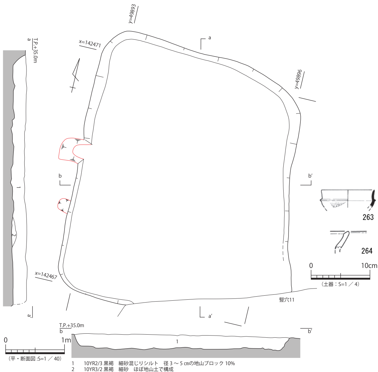
図 100 7-SX 4 平・断面図、出土遺物実測図
