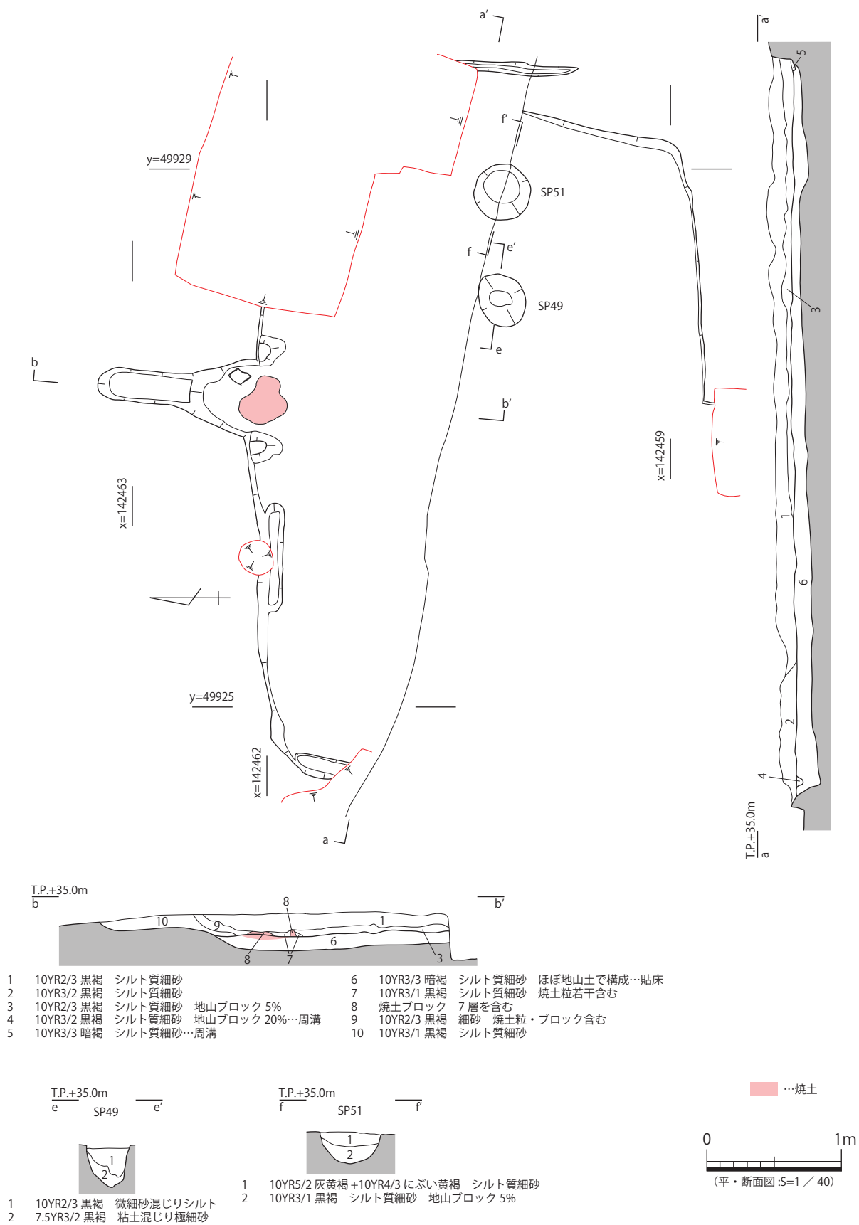
図 26 2・4- 竪穴 58 平・断面図
