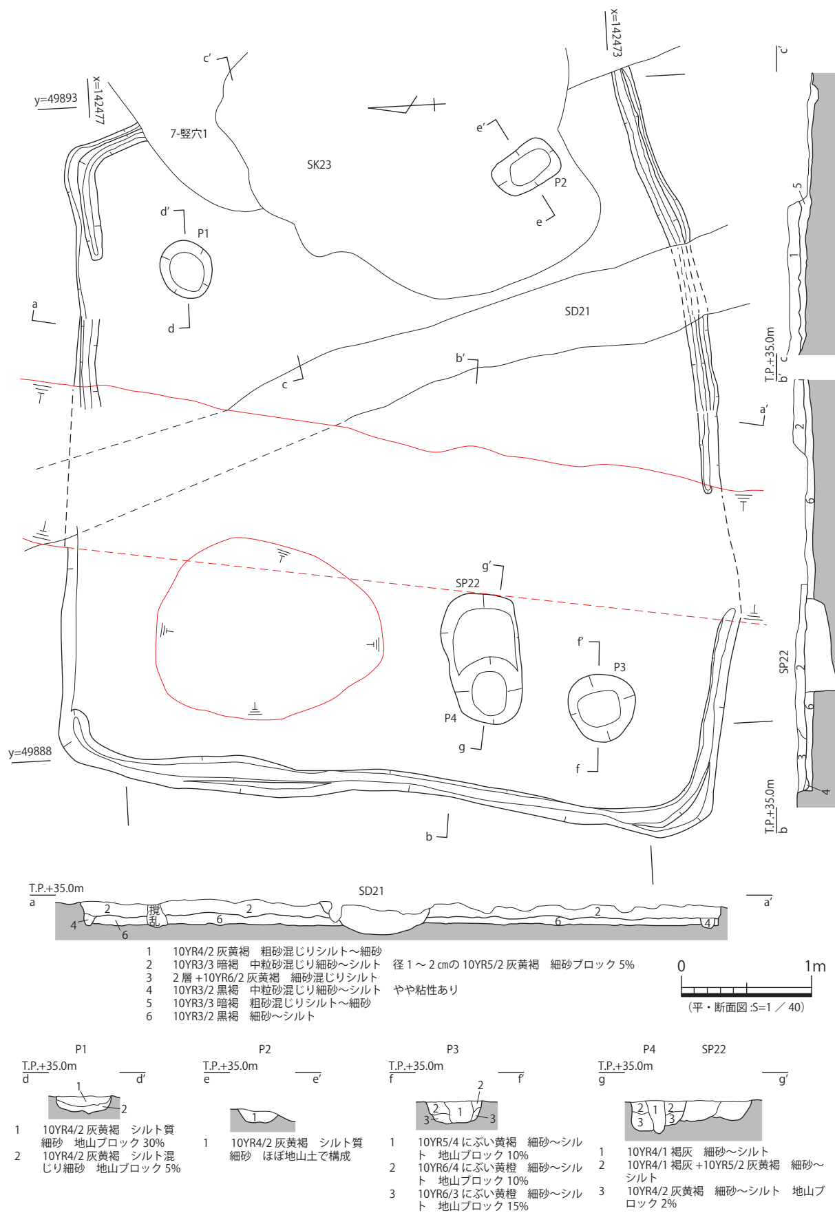
図 37 7・9- 竪穴 2 平・断面図
