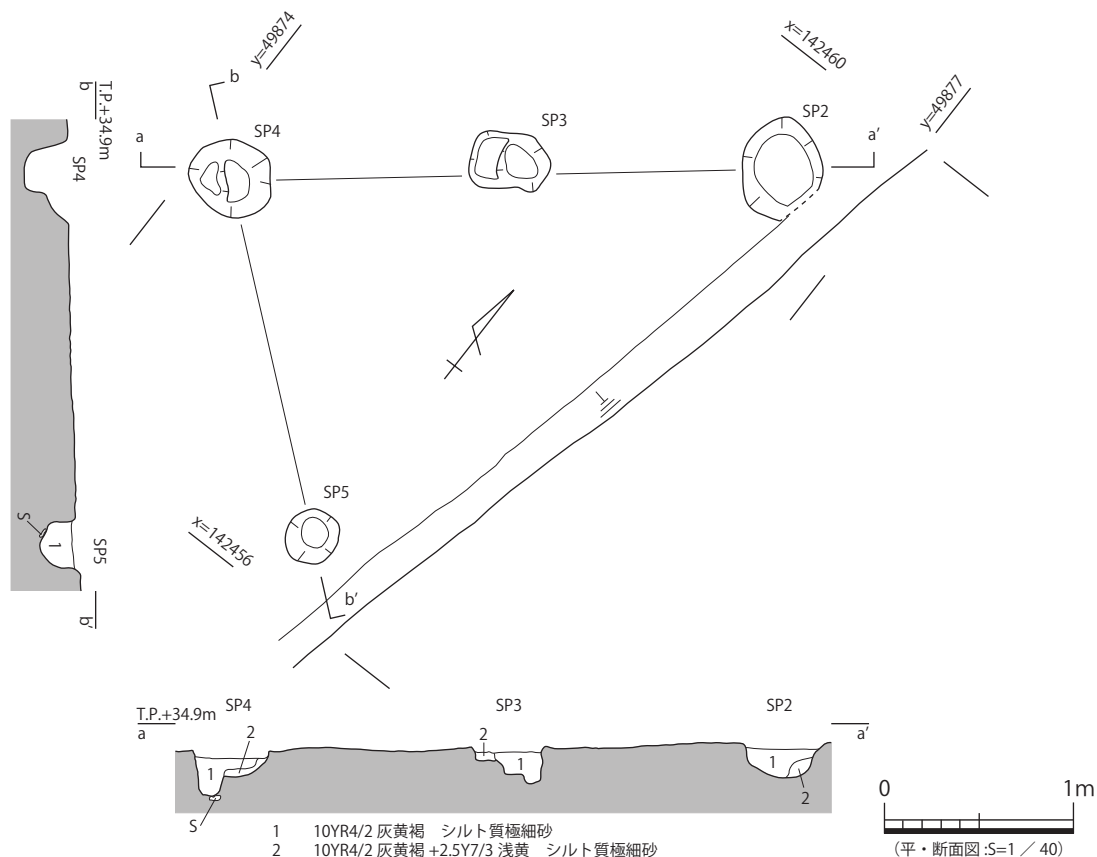
図 59 1－掘立1 平・断面図
