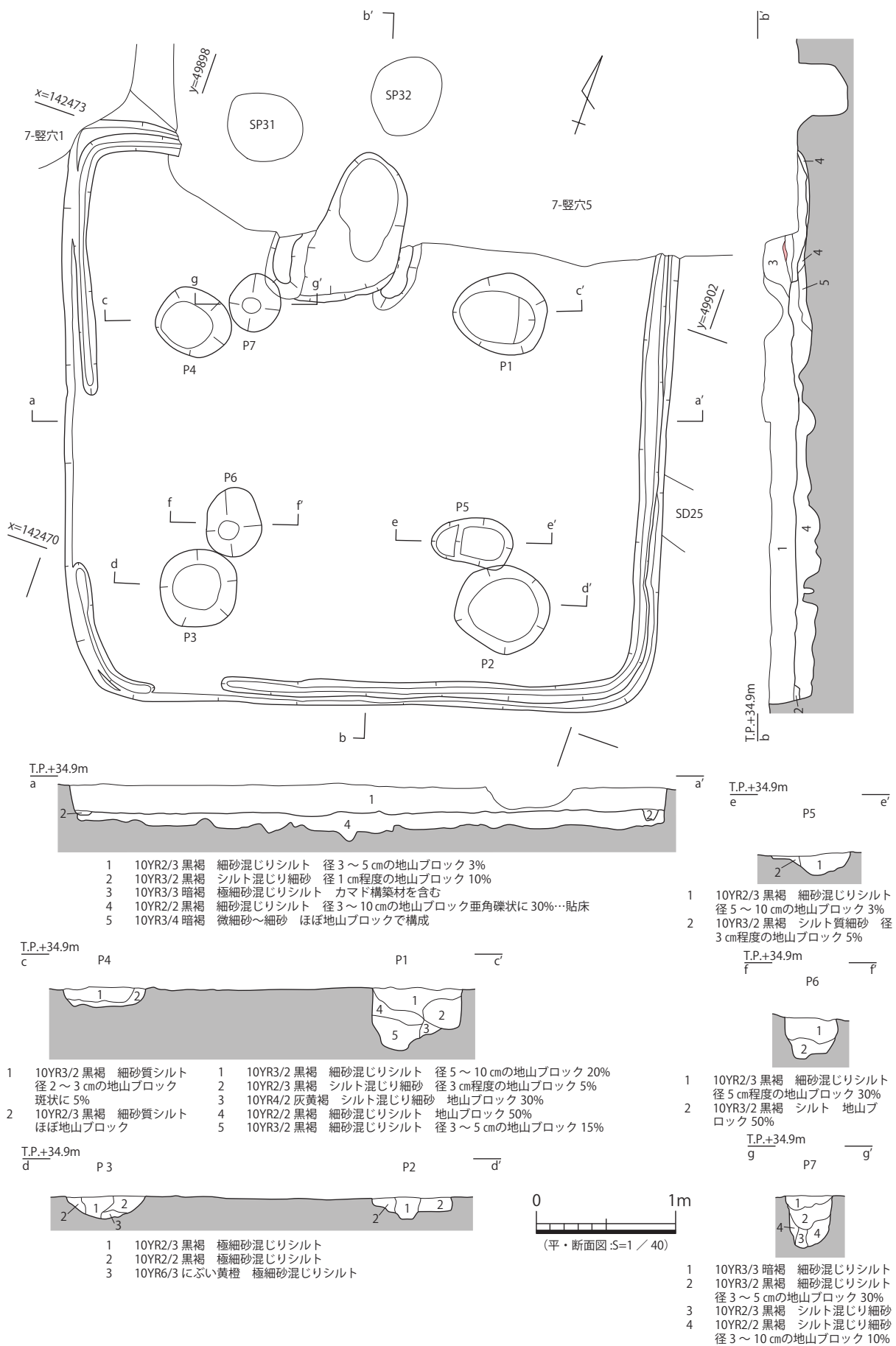
図 42 7-竪穴6 平・断面図
