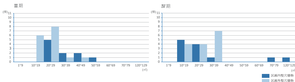
図 127 建物規模分布図
