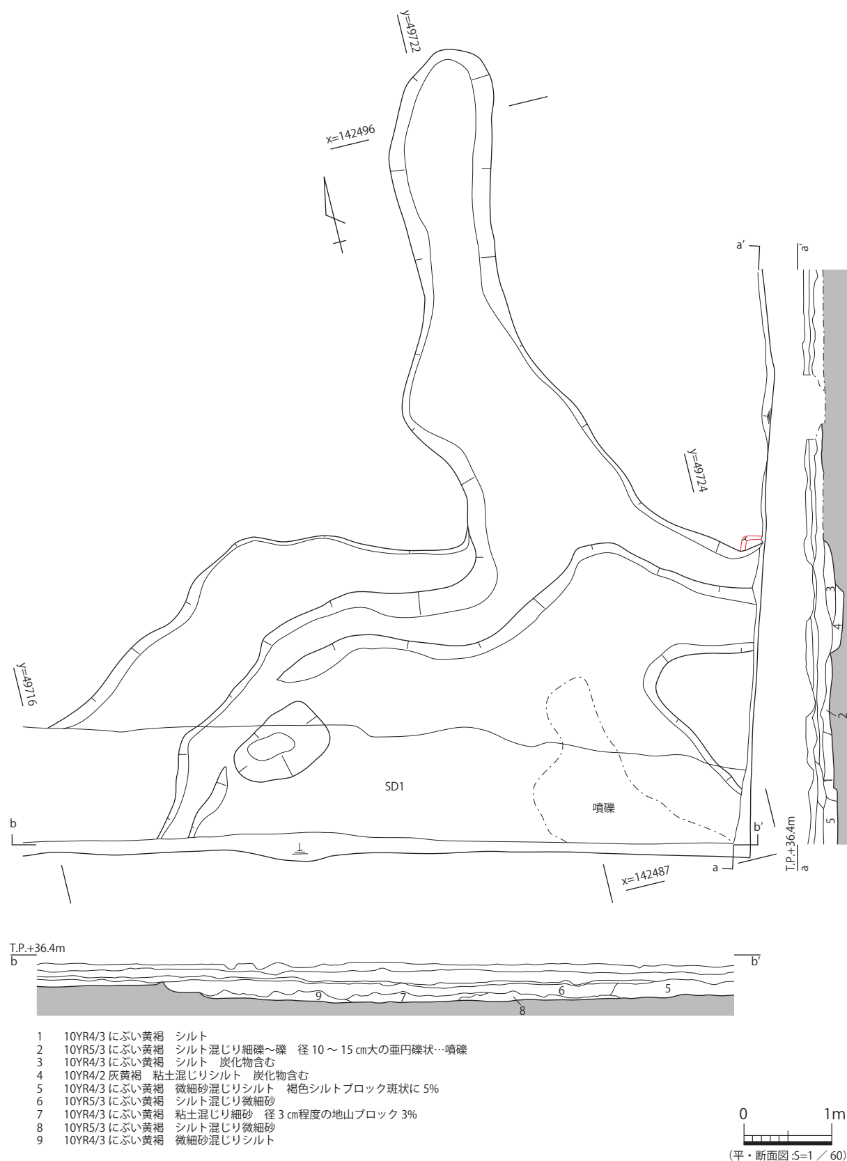
図 118 12-SX 2 平・断面図
