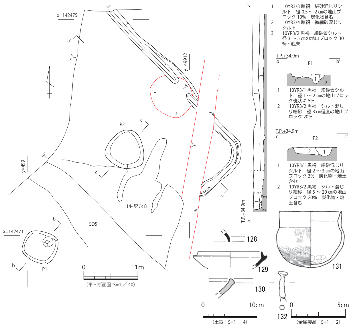
図 57 14- 竪穴 10 平・断面図、出土遺物実測図
