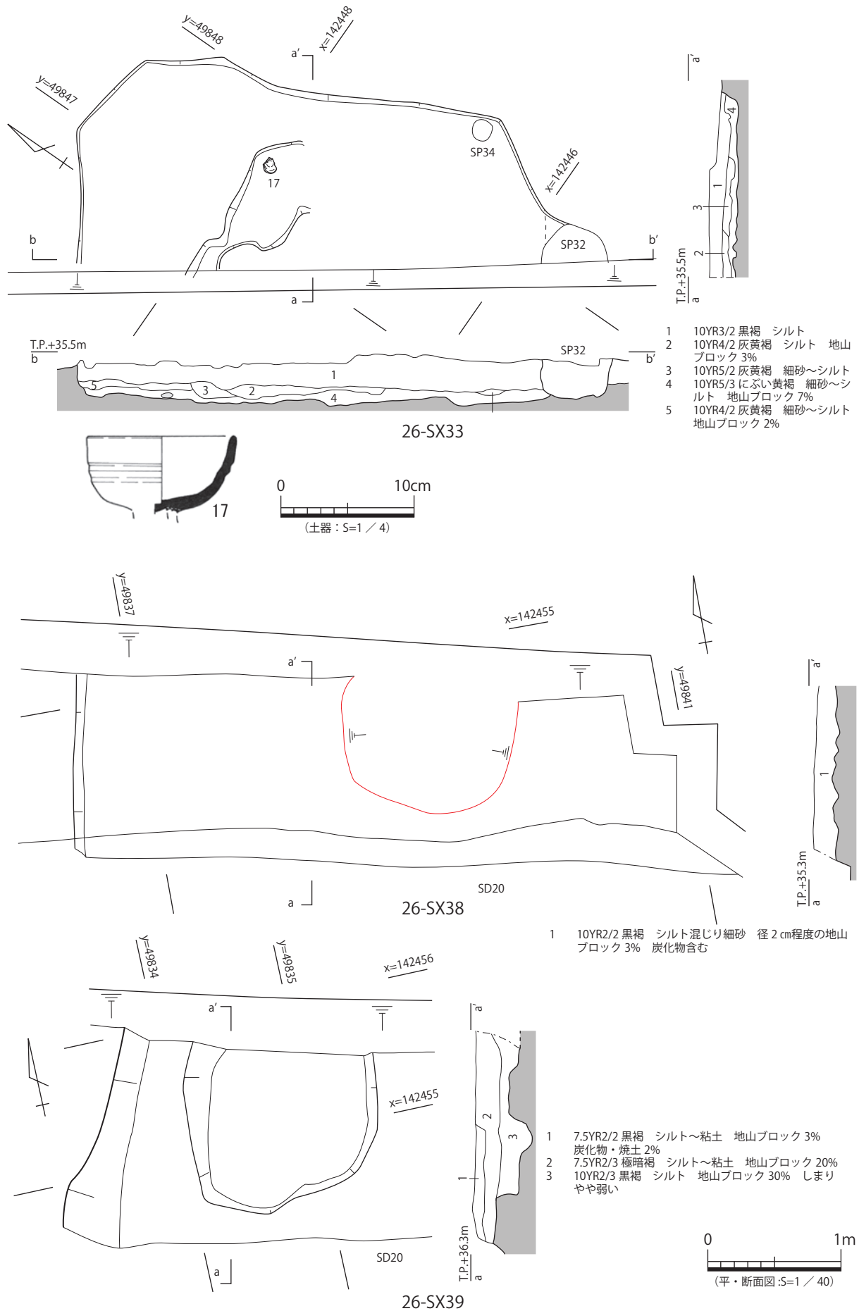
図 18 26-SX33・38・39 平・断面図、出土遺物実測図
