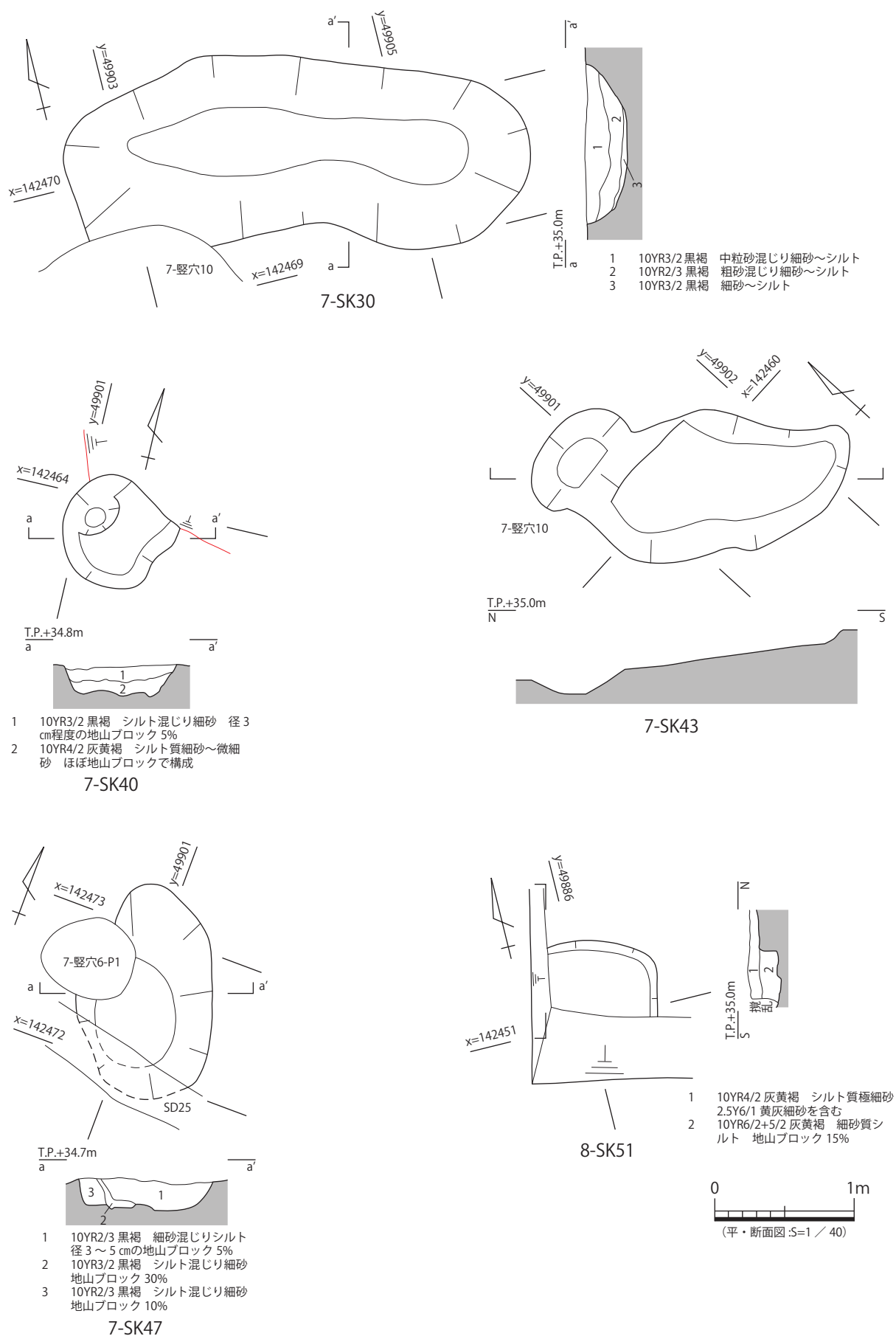
図 89 7-SK30・40・43・47、8-SK51 平・断面図
