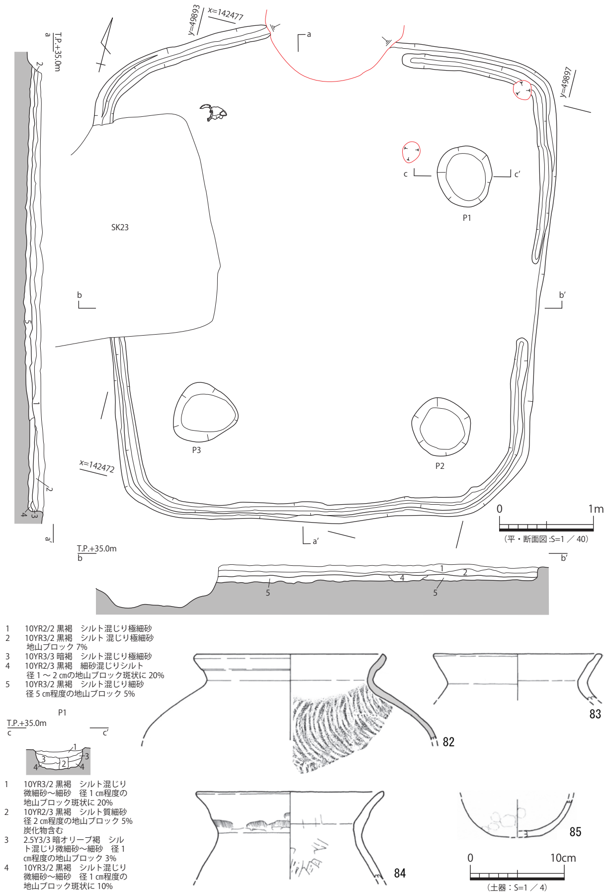
図 36 7- 竪穴 1 平・断面図、出土遺物実測図
