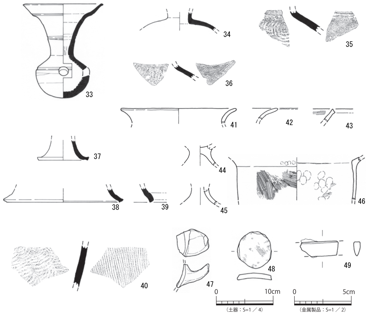
図 25 2・3- 竪穴 30 出土遺物実測図 (2)
