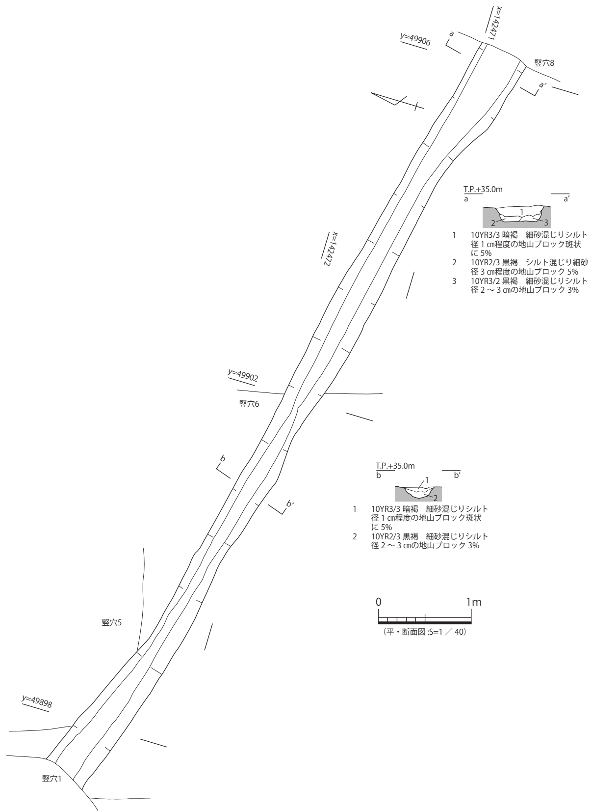
図 77 7-SD25 平・断面図
