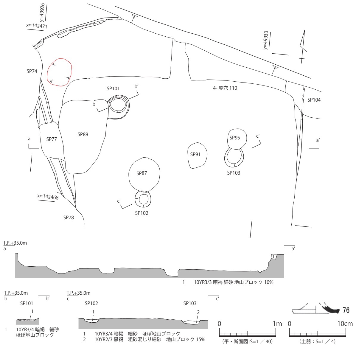
図 34 4- 竪穴 120 平・断面図、出土遺物実測図
