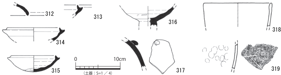
図 116 11-SX 2 平・断面図、出土遺物実測図
