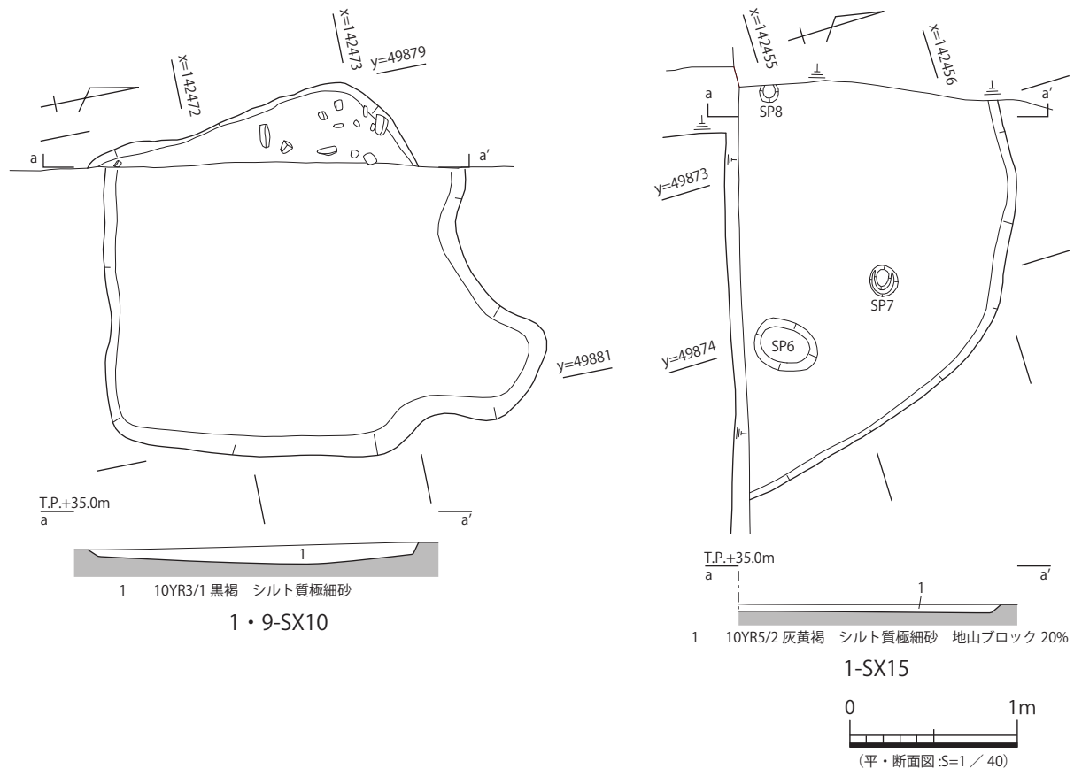
図 94 1・9-SX10、1-SX15 平・断面図
