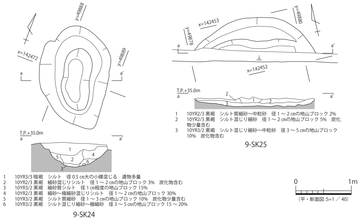
図 91 9-SK24・25 平・断面図
