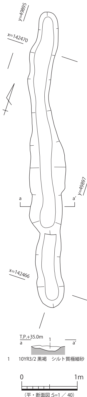
図 78 7-SD39 平・断面図
