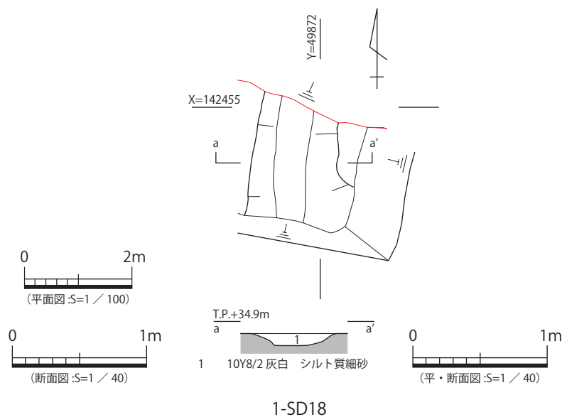
図 69 1-SD17・18 平・断面図
