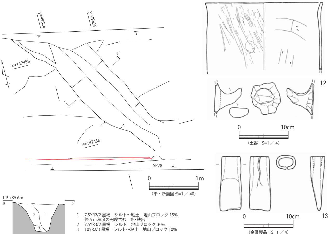
図 11 26-SD29 平・断面図、出土遺物実測図
