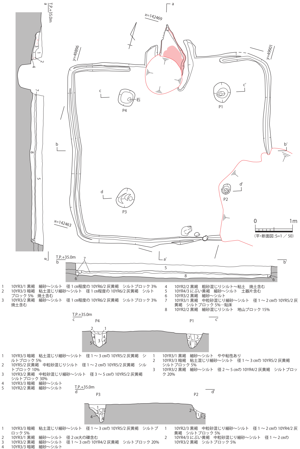
図 48 7- 竪穴 11 平・断面図
