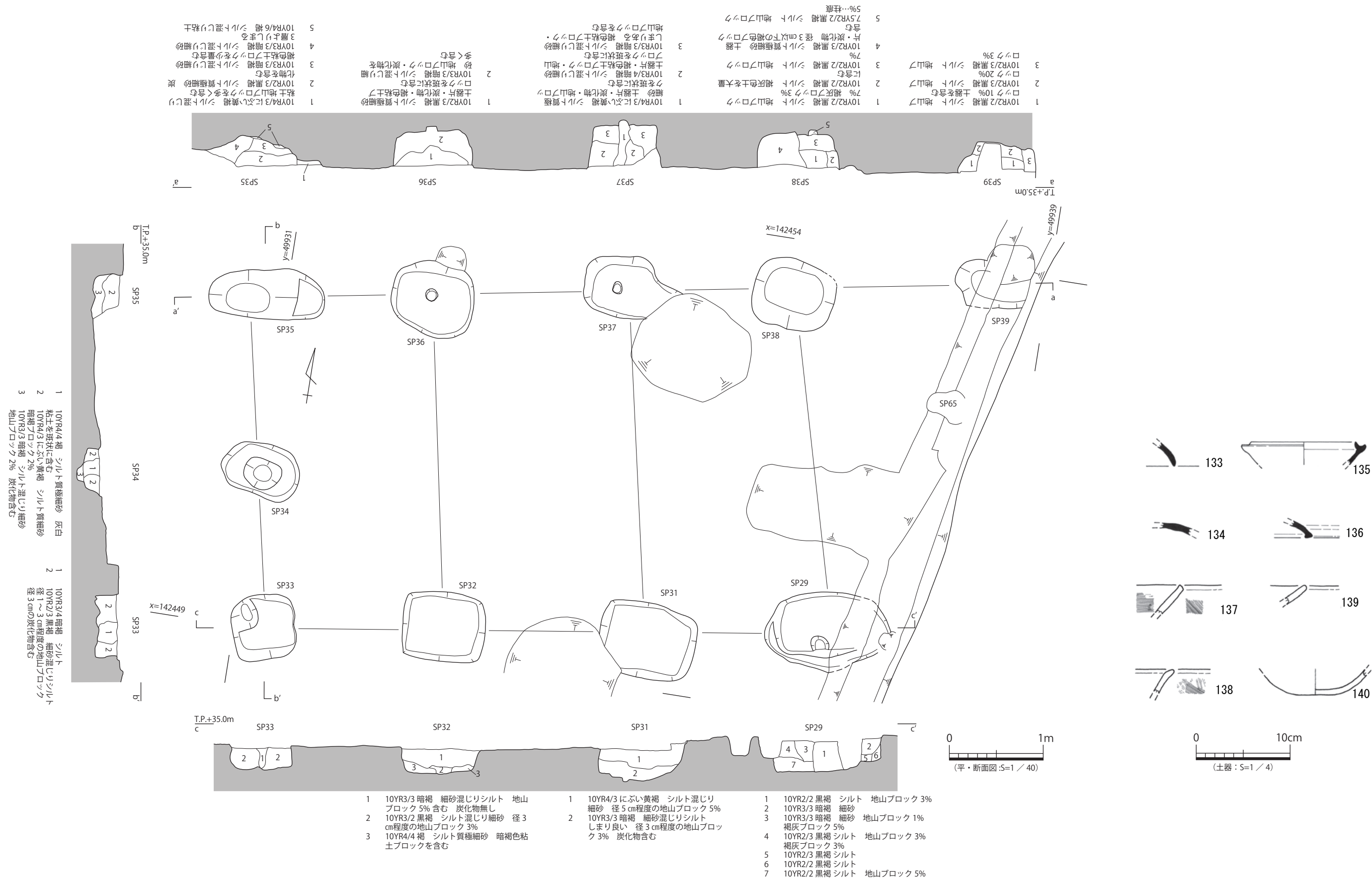
図 60 2・3-掘立1 平・断面図、出土遺物実測図
