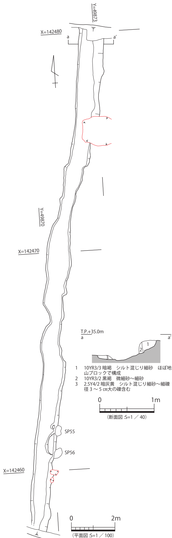
図 71 16-SD50 平・断面図
