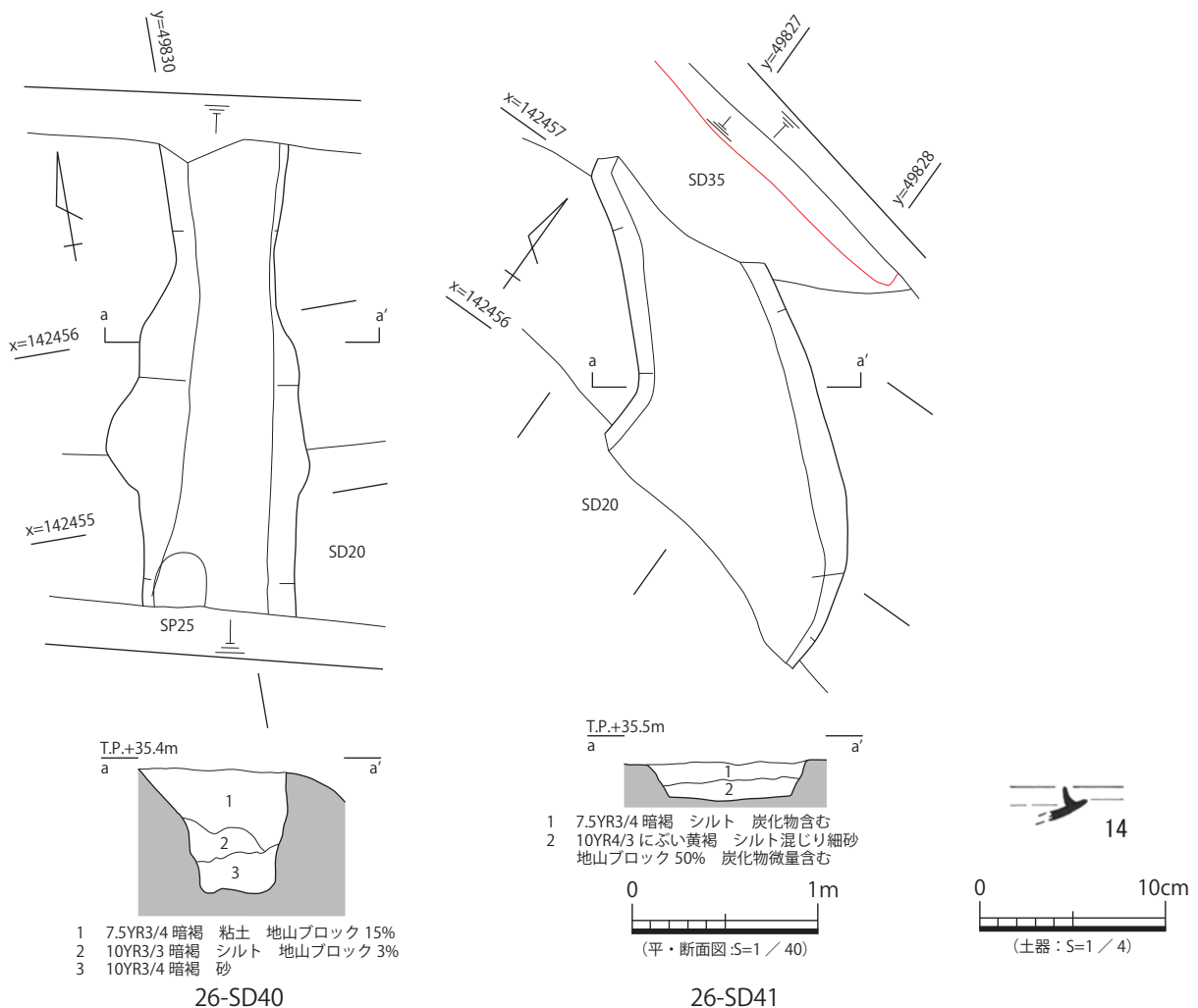
図 13 26-SD40・41 平・断面図、出土遺物実測図
