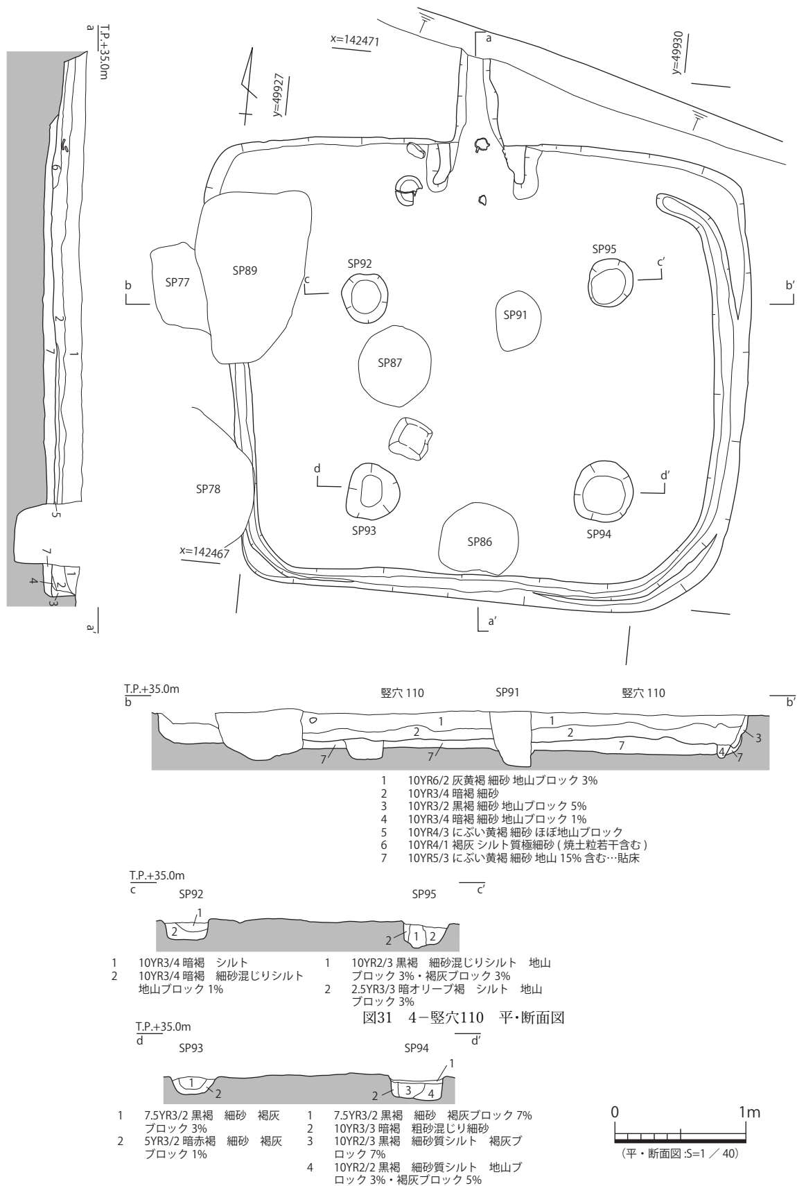
図 31 4- 竪穴110 平・断面図
