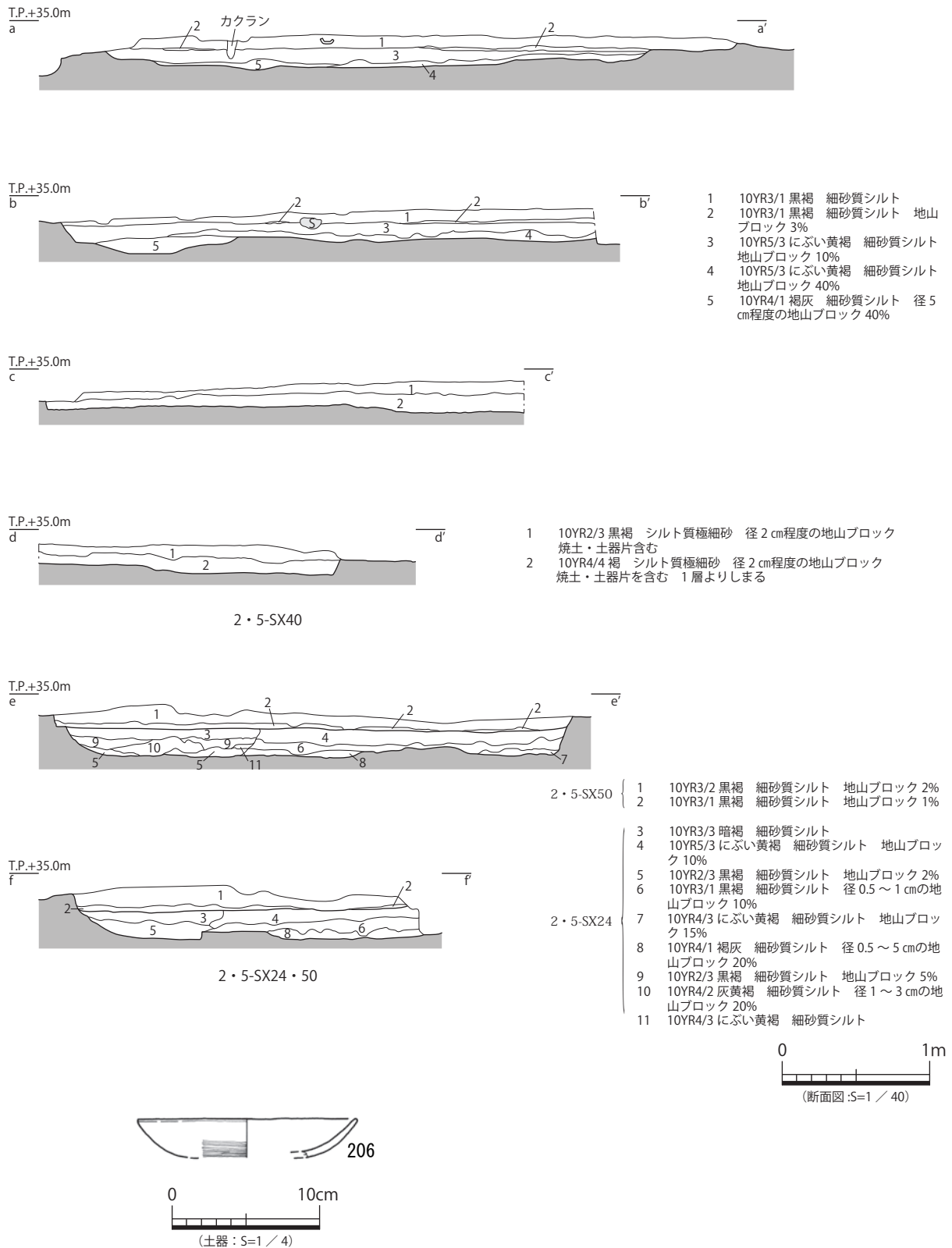
図 97 2・5-SX24・40・50 断面図、2・5-SX24 出土遺物実測図
