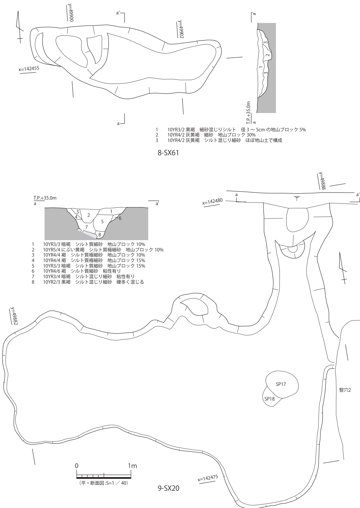
図 103 8-SX61、9-SX20 平・断面図
