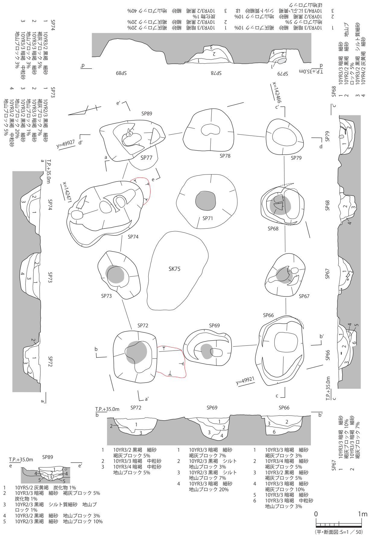
図 63 4-掘立 4 平・断面図
