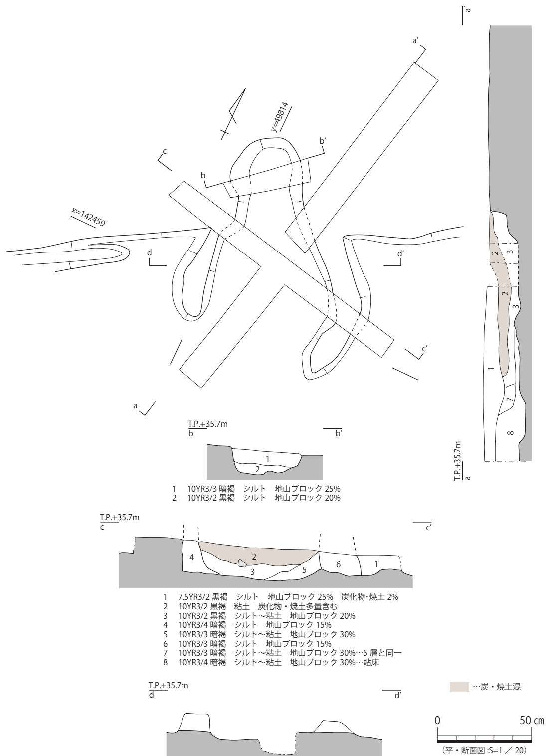
図6 26- 竪穴45カマド 平・断面図
