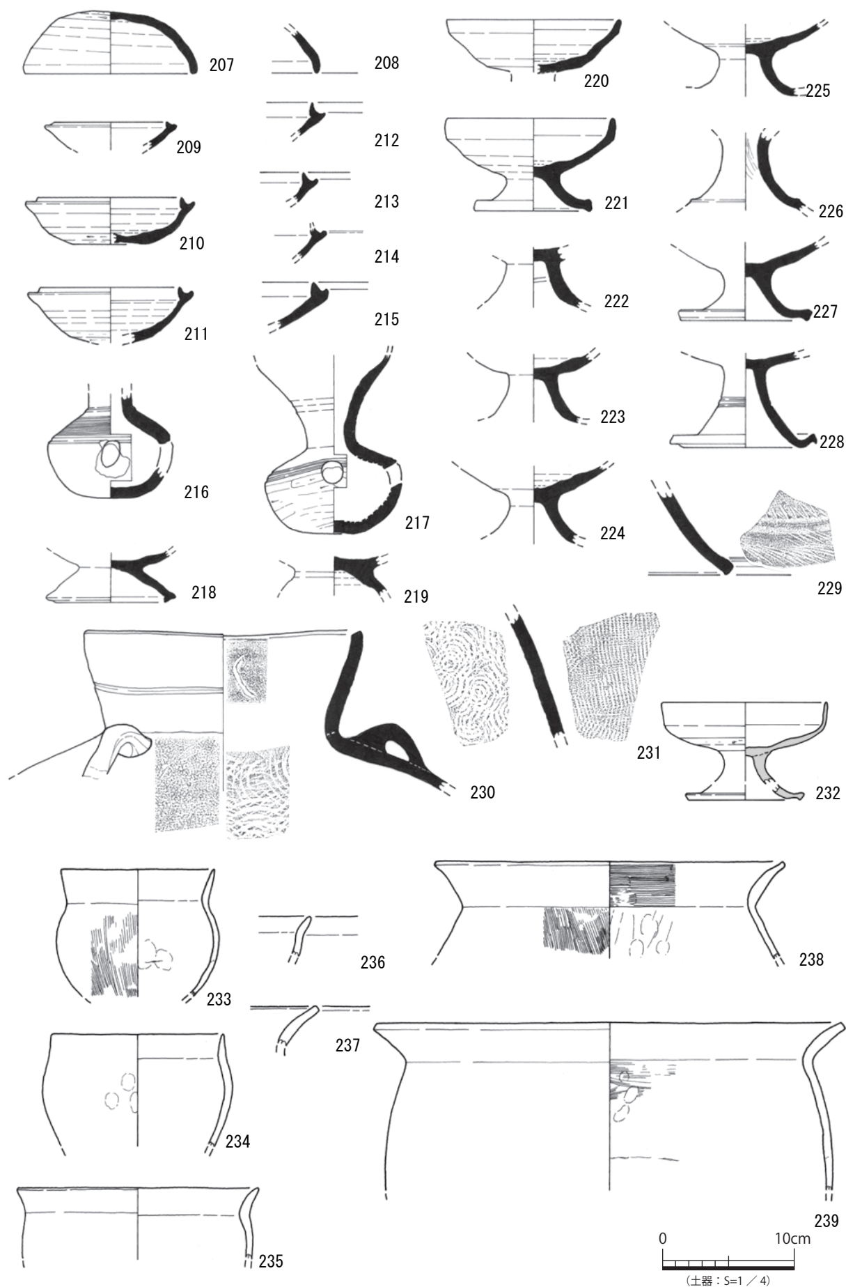
図 98 2・5-SX40 出土遺物実測図
