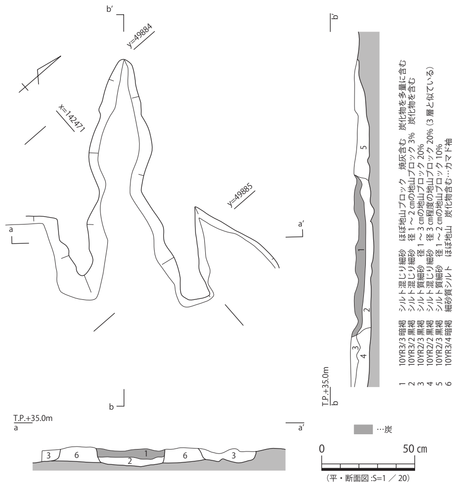
図 39 7・9- 竪穴3カマド 平・断面図
