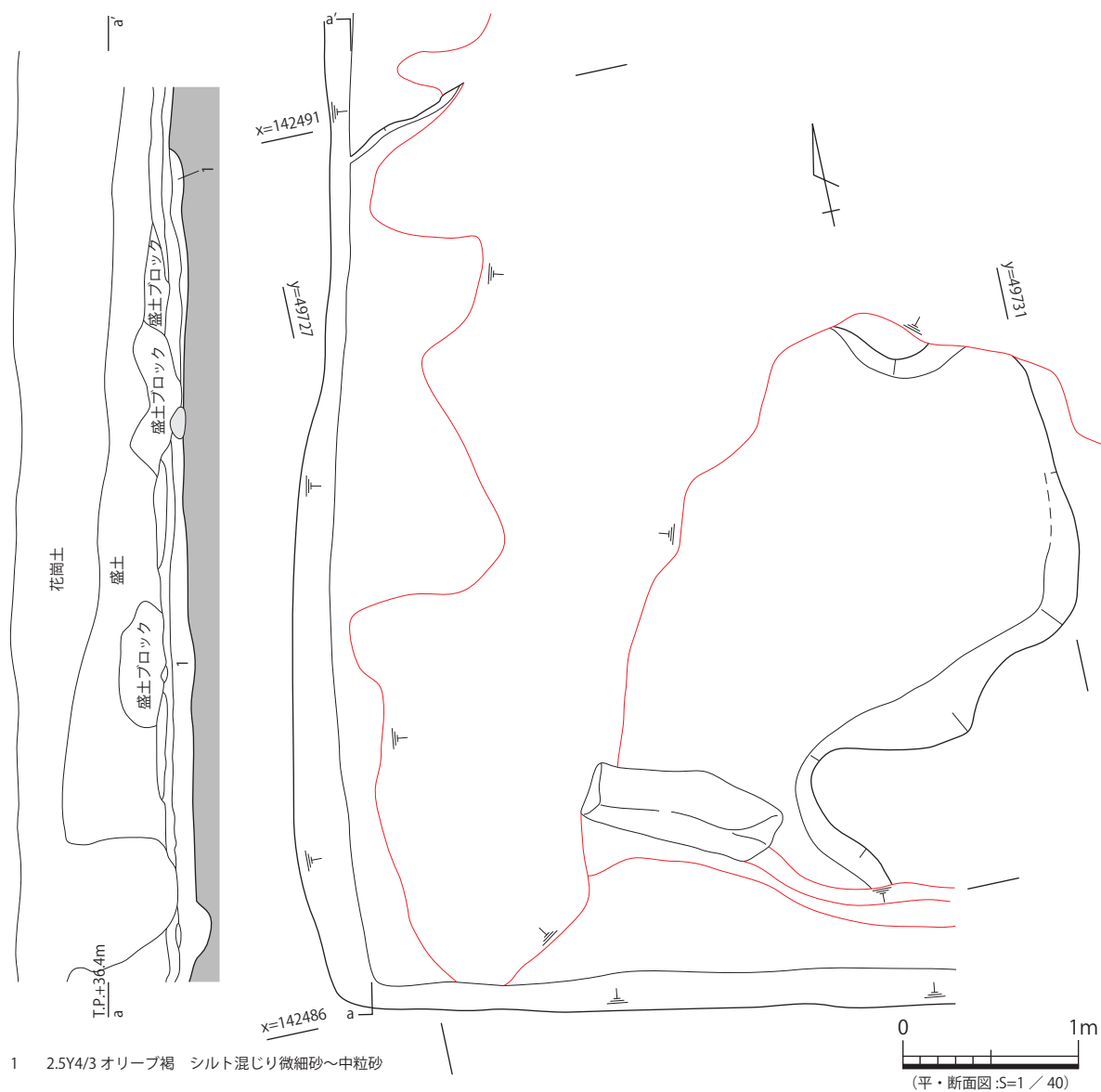
図 120 13-SX 2 平・断面図
