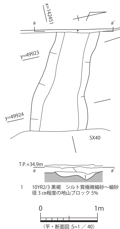
図 75 5-SD 2 平・断面図
