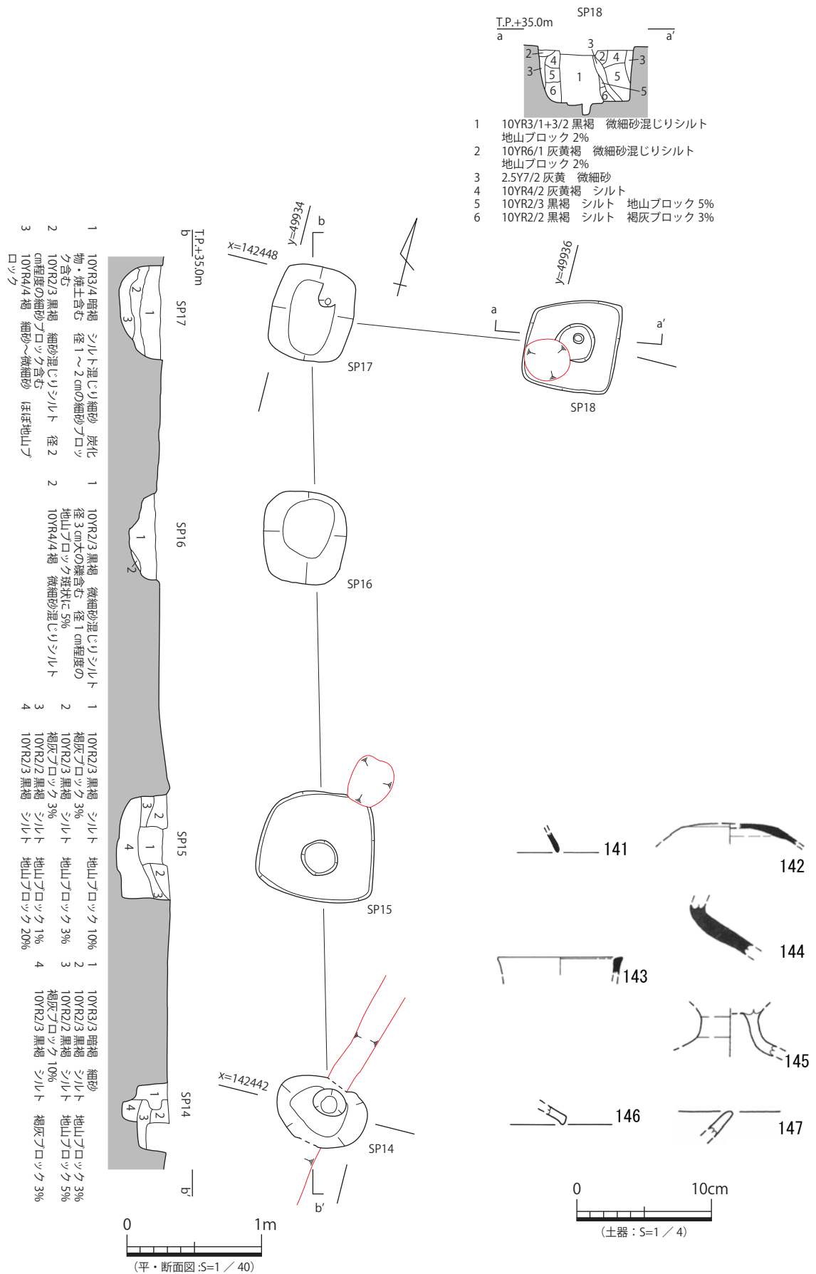
図 61 2・3-掘立2 平・断面図、出土遺物実測図
