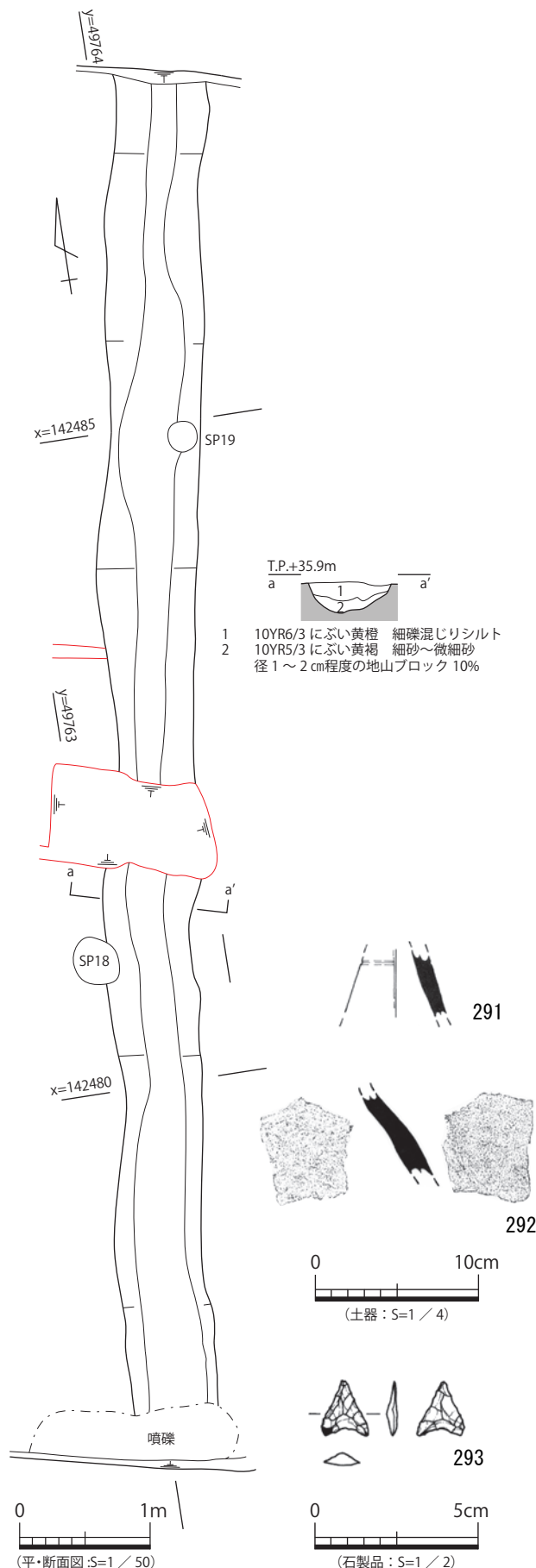
図 109 10-SD15 平・断面図、出土遺物実測図
