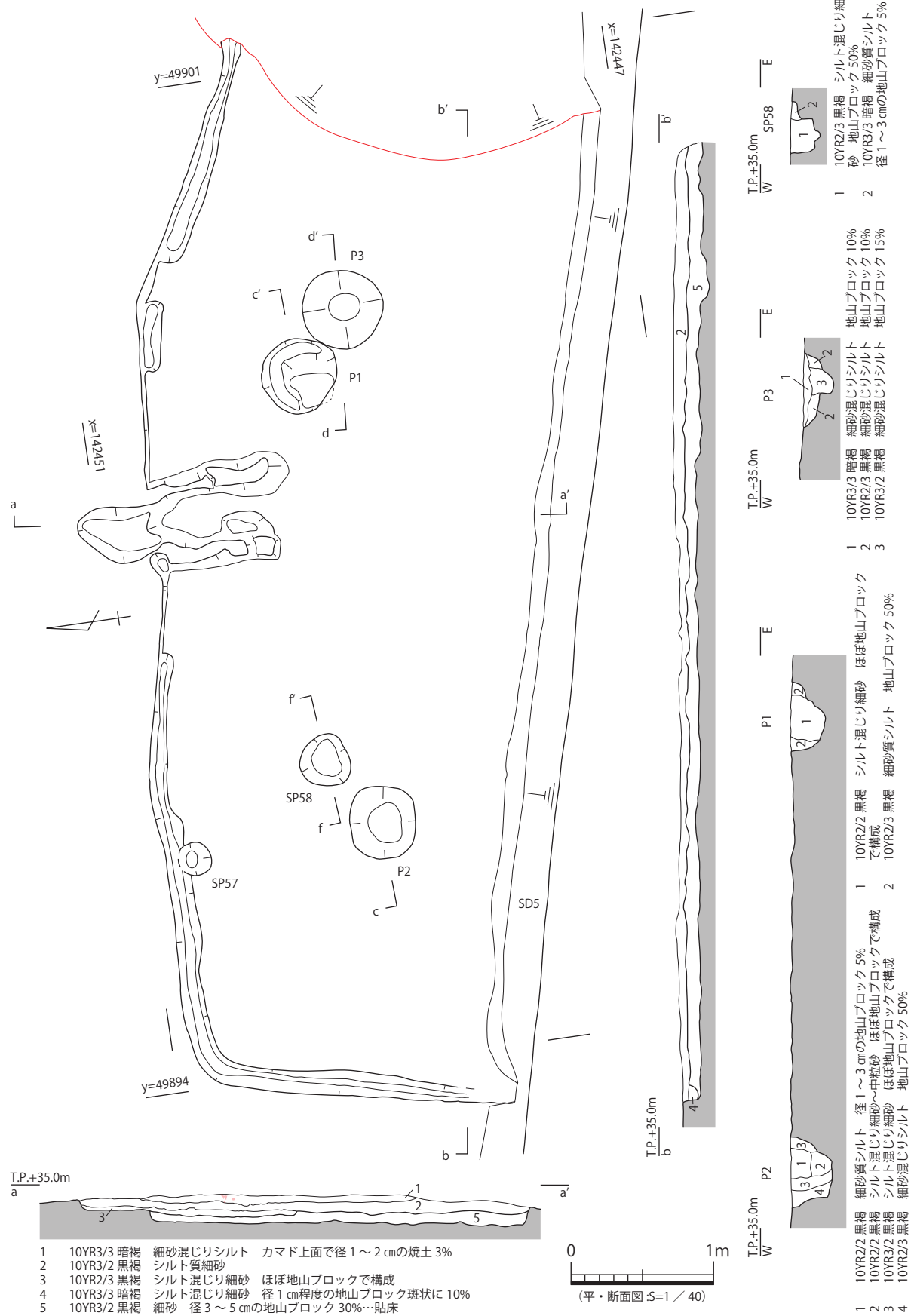
図 50 8- 竪穴 12 平・断面図
