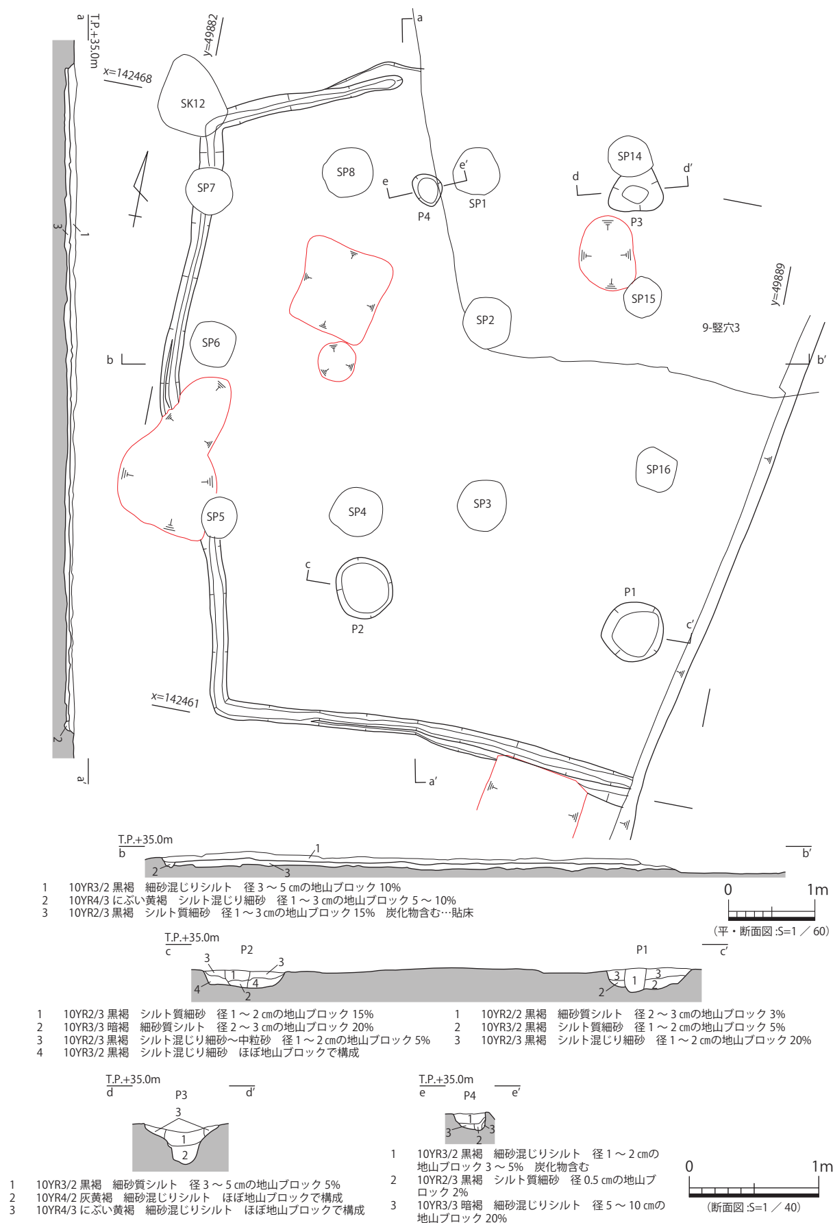
図 54 9- 竪穴 1 平・断面図
