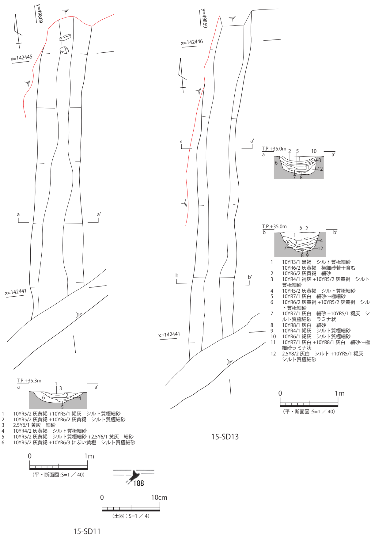
図 81 15-SD11・13 平・断面図、出土遺物実測図
