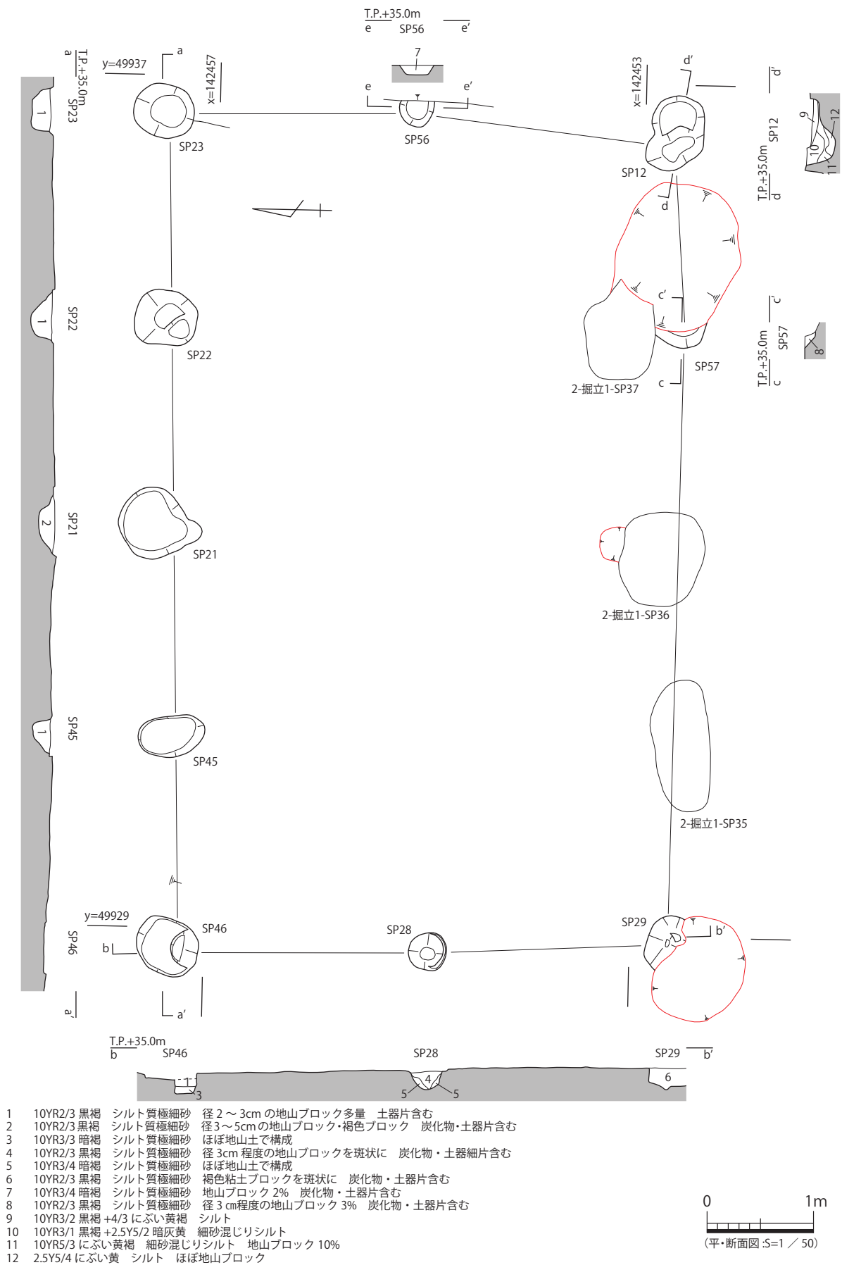
図 67 2・3-掘立7 平・断面図
