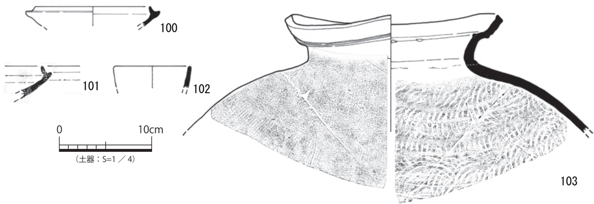
図 45 7- 竪穴 7 出土遺物実測図
