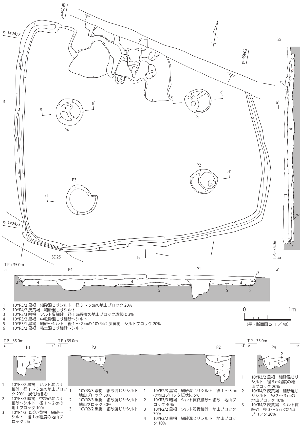
図 40 7- 竪穴 5 平・断面図
