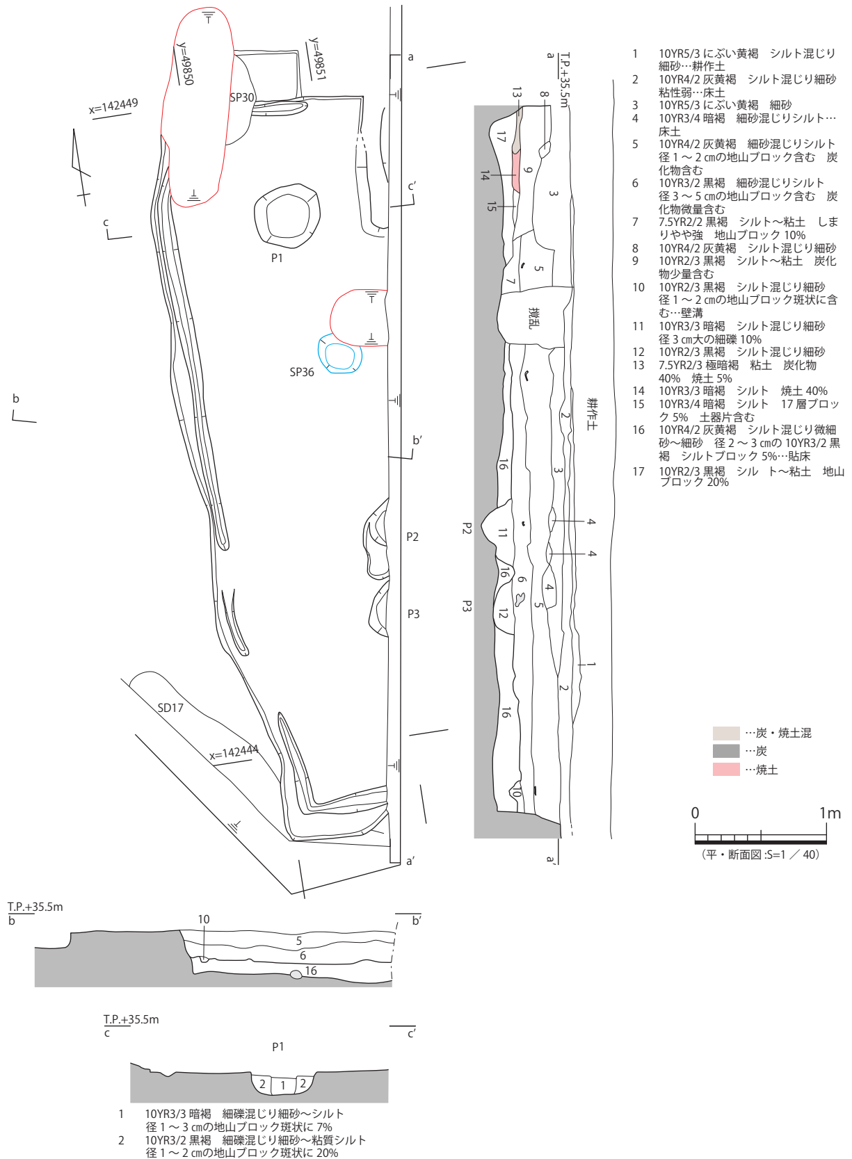
図3 26- 竖穴 18 平・断面図
