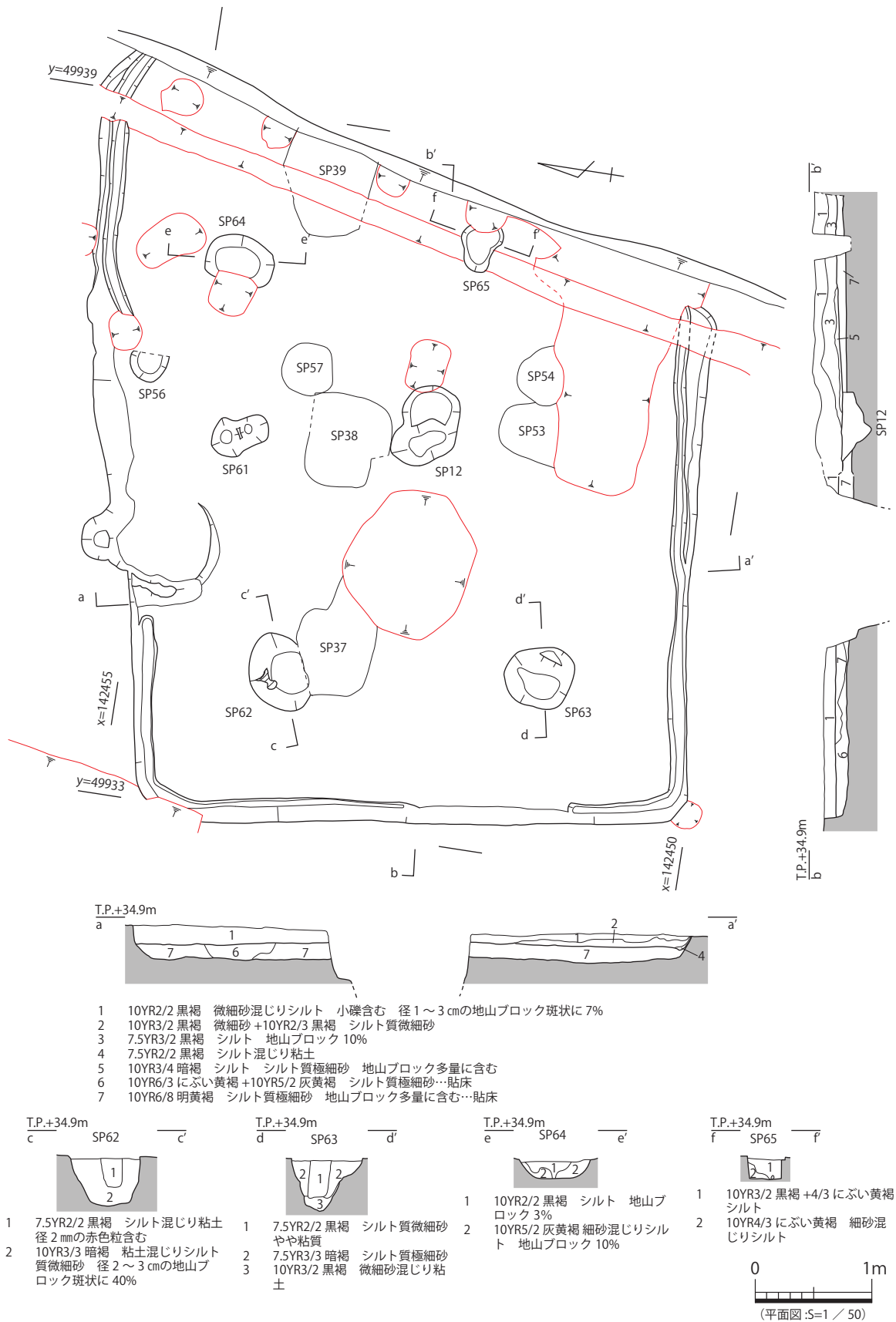
図 23 2・3- 竪穴 30 平・断面図
