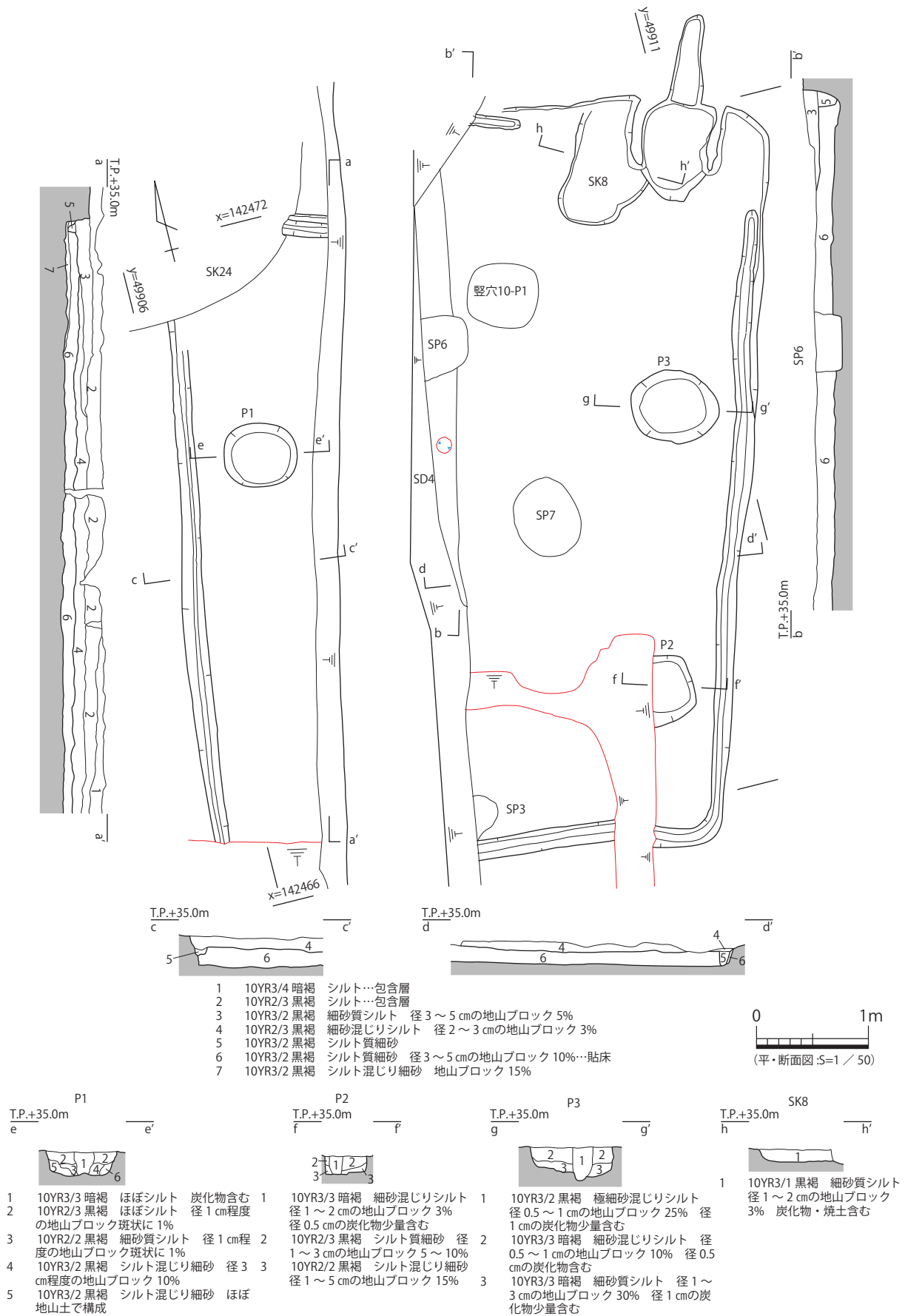
図 55 7・14- 竪穴 8 平・断面図
