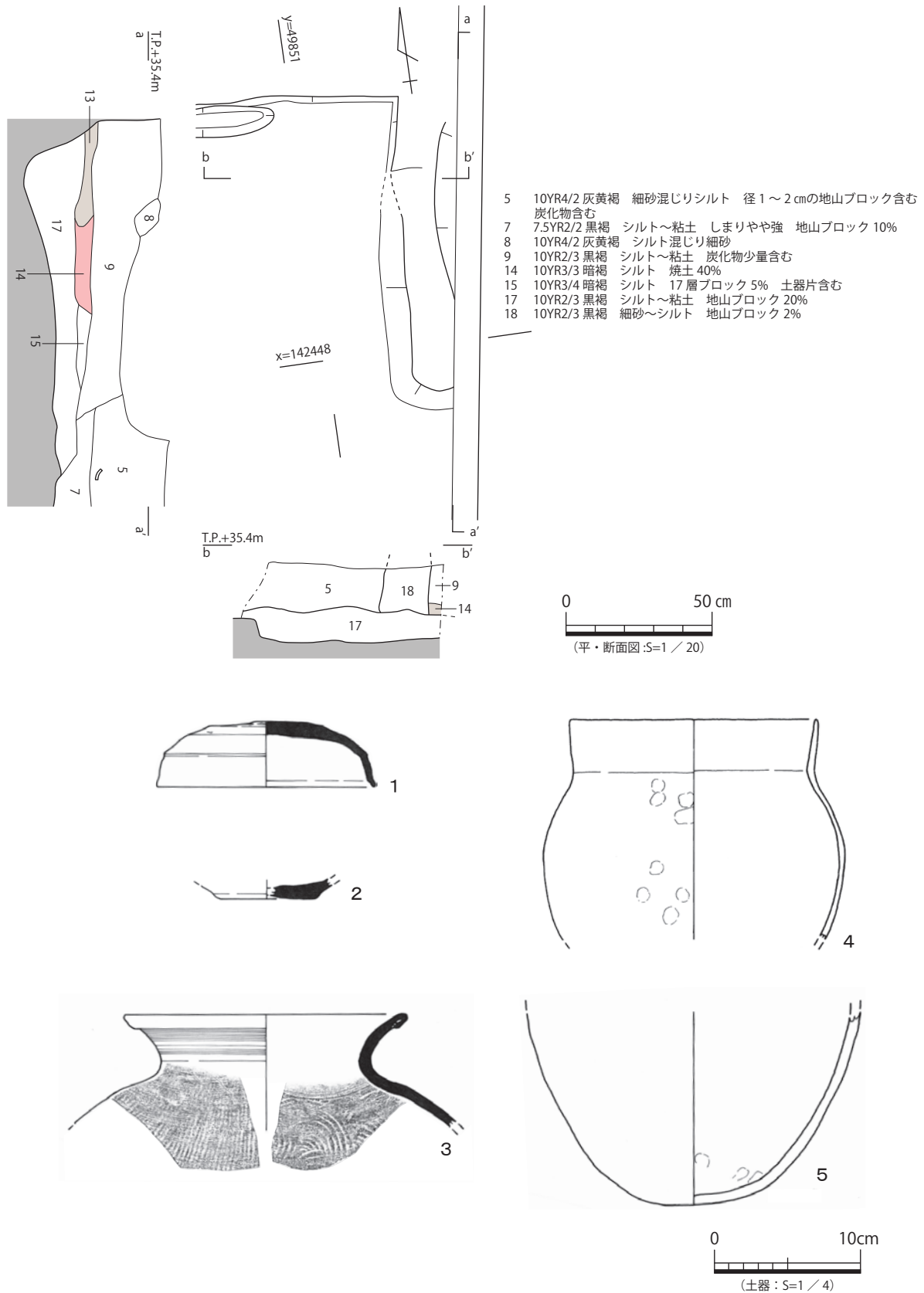
図4 26- 竪穴 18 カマド 平・断面図、出土遺物実測図
