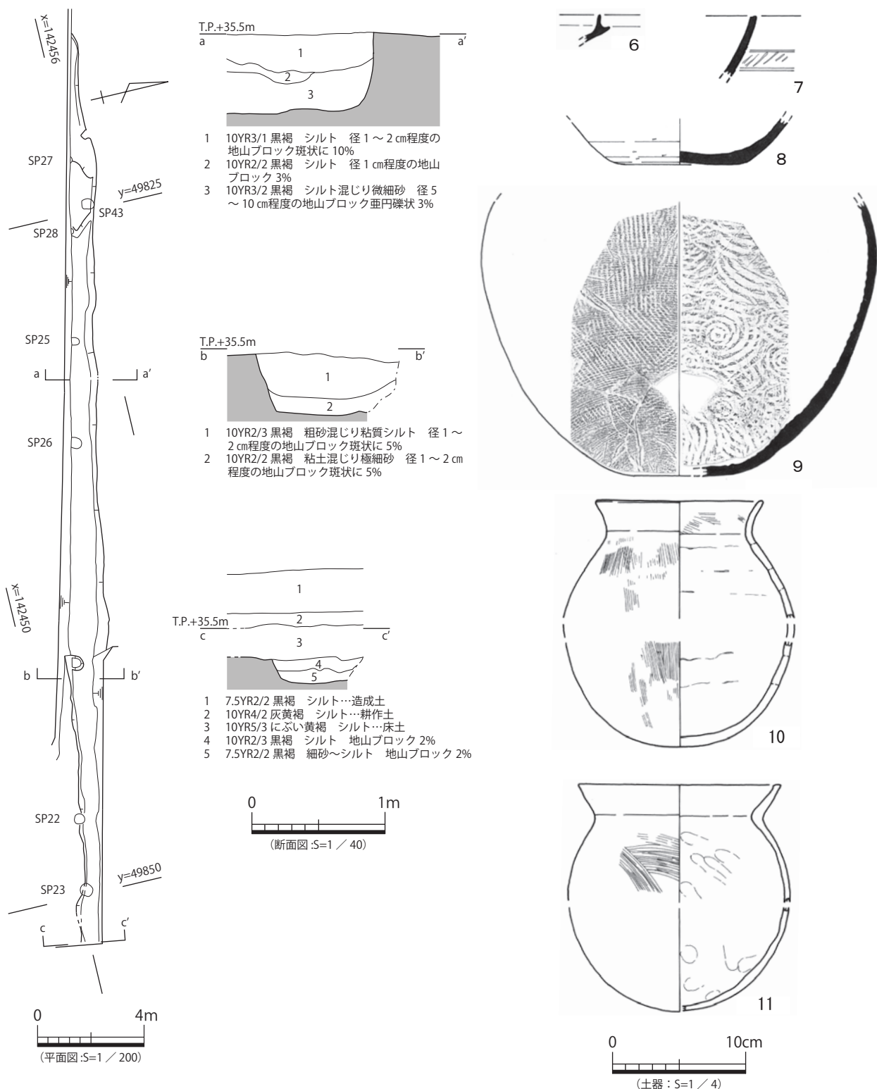
図10 26-SD20 平・断面図、出土遺物実測図
