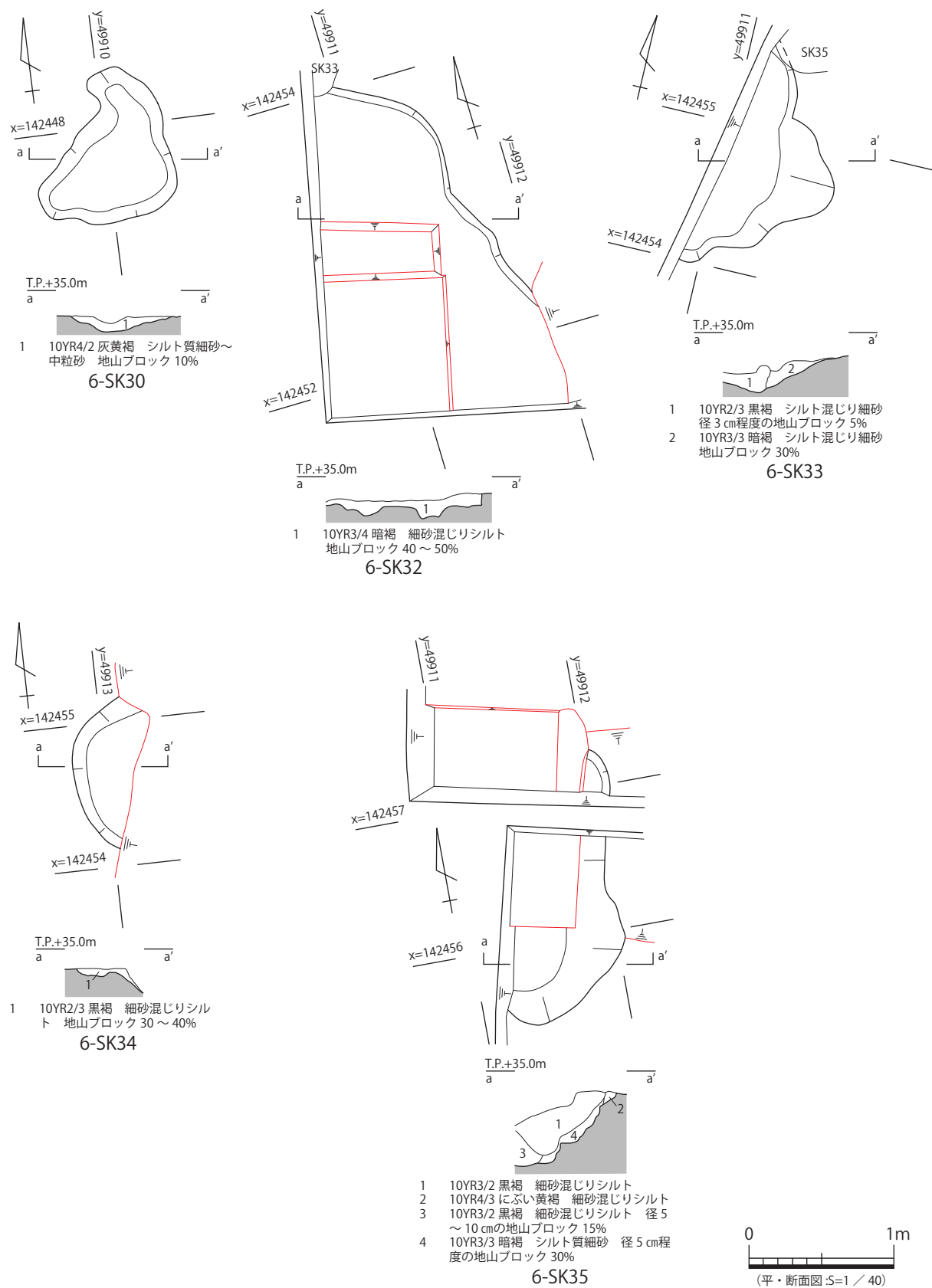
図 86 6-SK30・32～35 平・断面図
