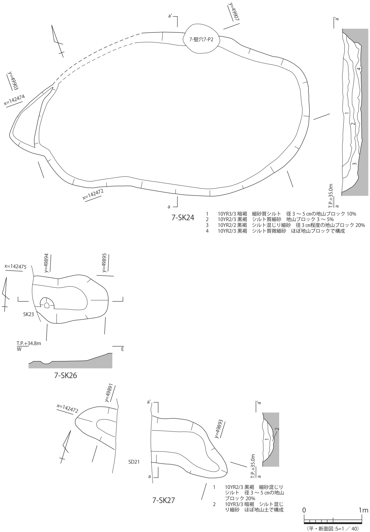
図 88 7-SK24・26・27 平・断面図
