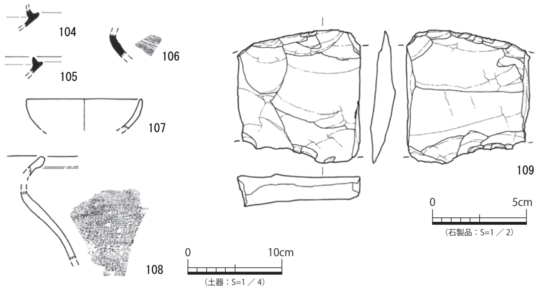
図 47 7- 竪穴 10 出土遺物実測図
