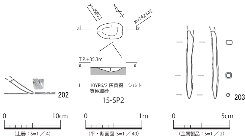
図 93 1-SP25、4-SP41、7-SP34、15-SP 2 平・断面図、出土遺物実測図
