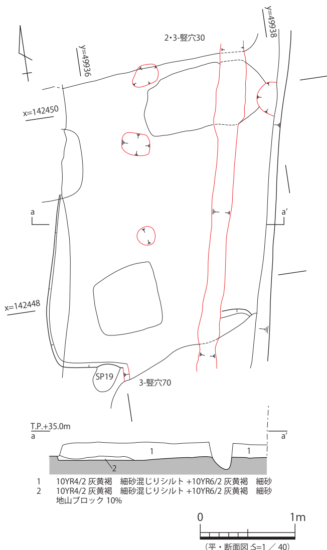
図 29 3- 竪穴 90 平・断面図
