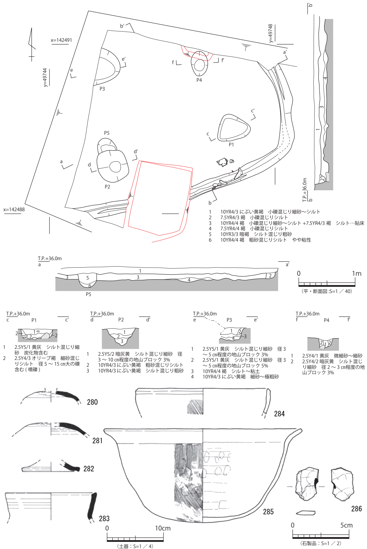
図 107 10- 竪穴 1 平・断面図、出土遺物実測図
