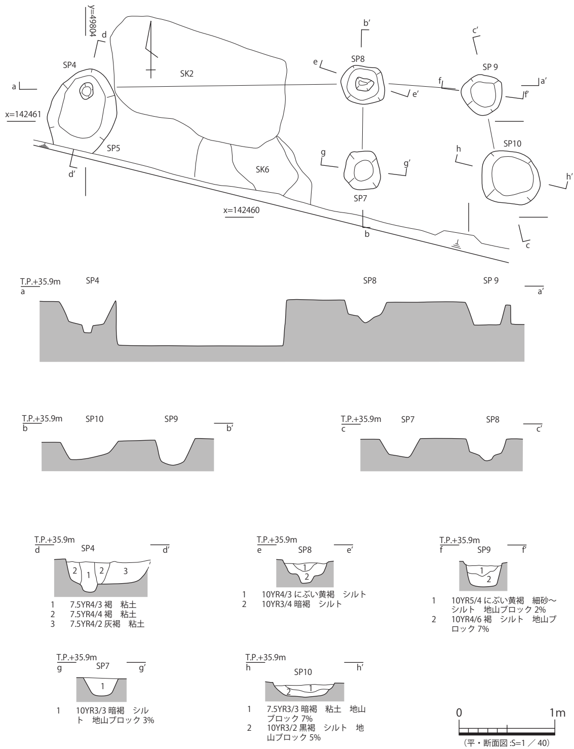
図 7 26- 掘立 52 平・断面図
