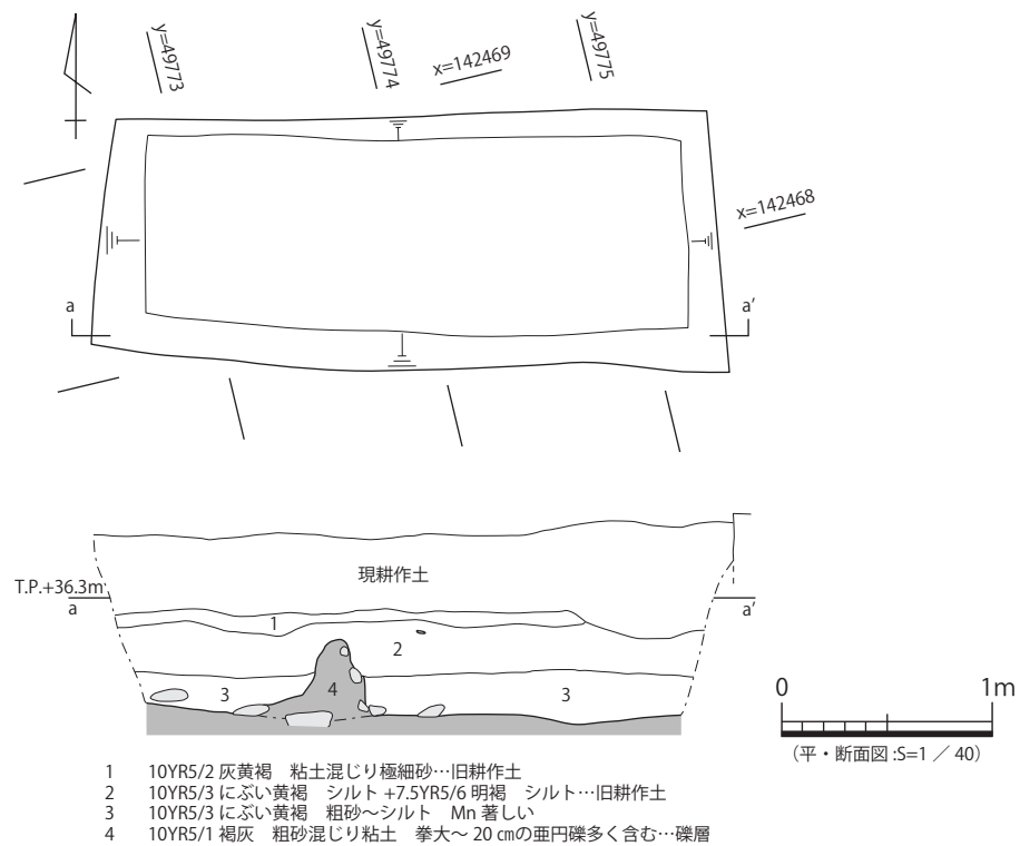
図122 第25調査区 平・断面図
