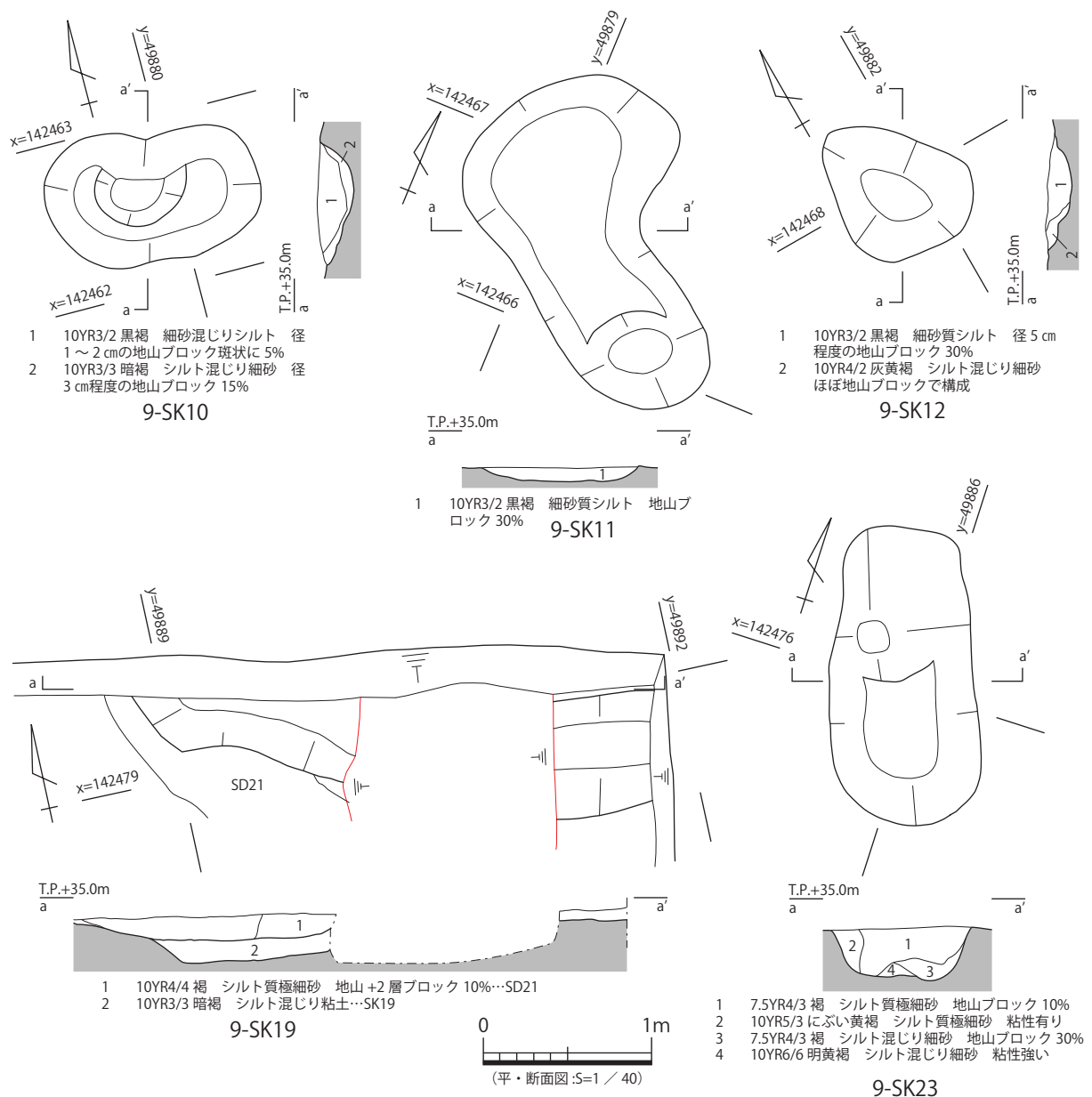
図 90 9-SK10 ~ 12・19・23 平・断面図
