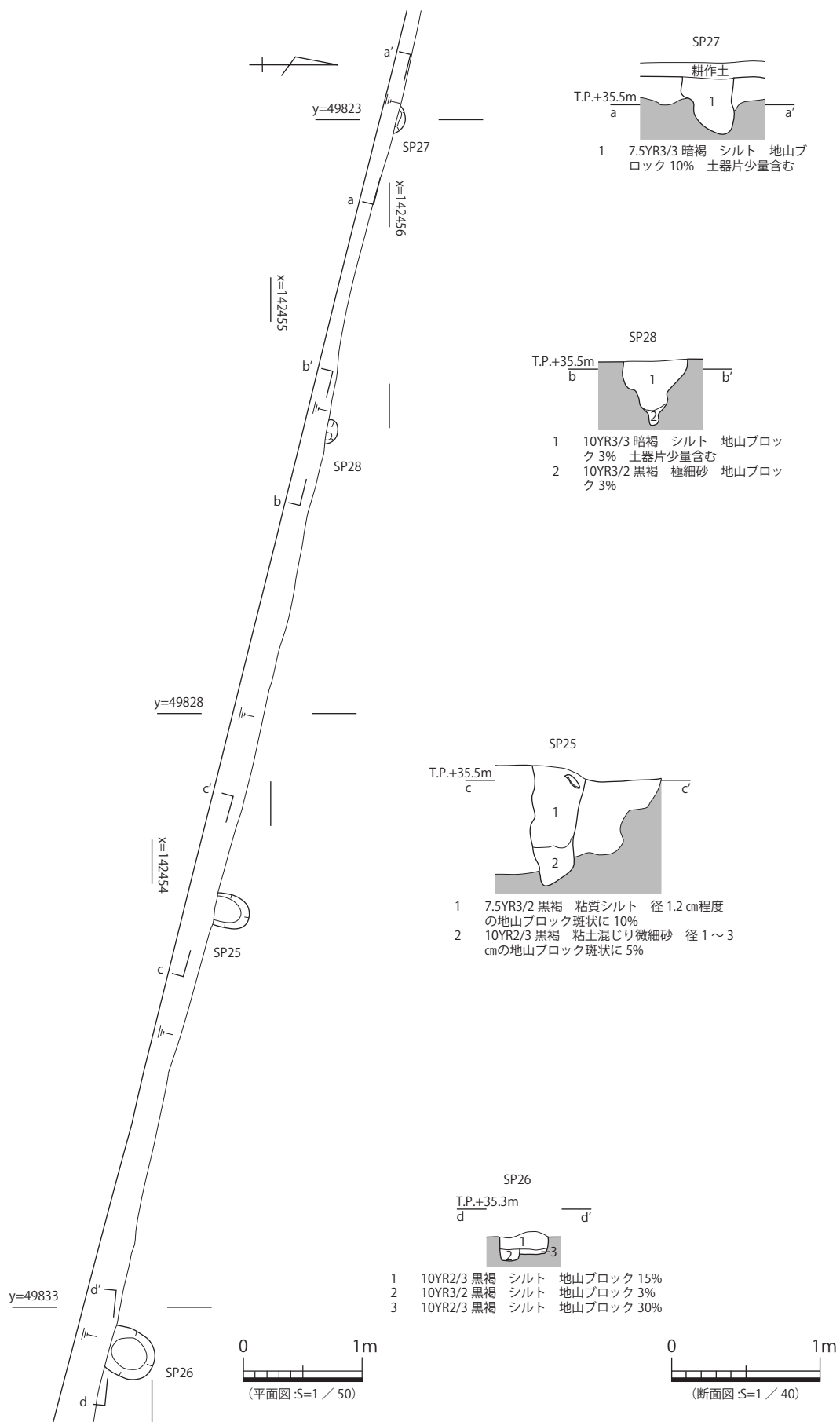
図 17 26- 柵列 55 平・断面図
