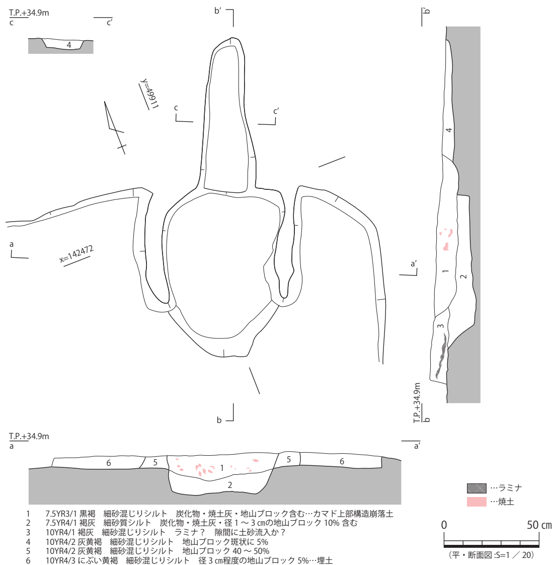
図56 7・14－竪穴8カマド 平・断面図
