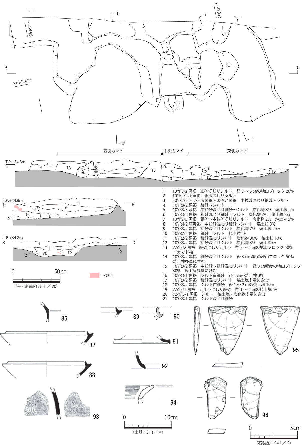
図 41 7- 竪穴5カマド 平・断面図、出土遺物実測図
