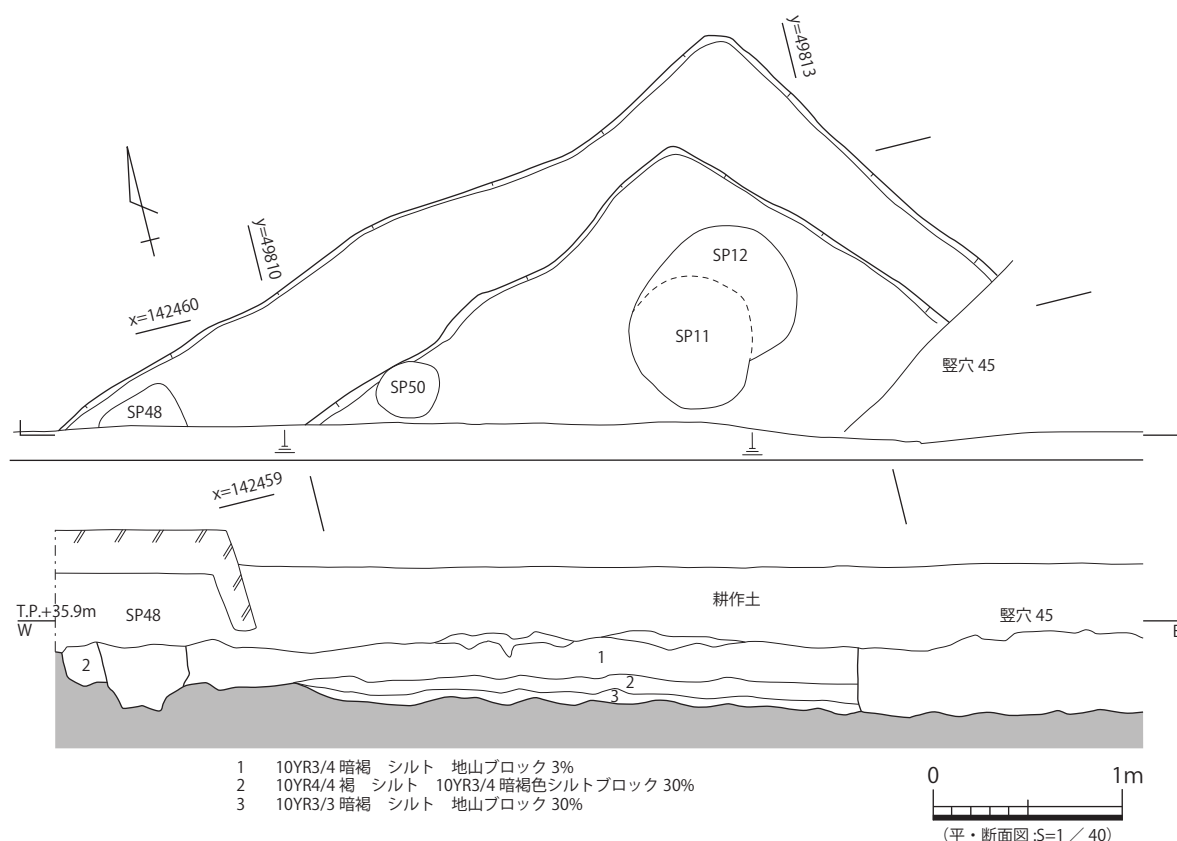
図 19 26-SX51 平・断面図
