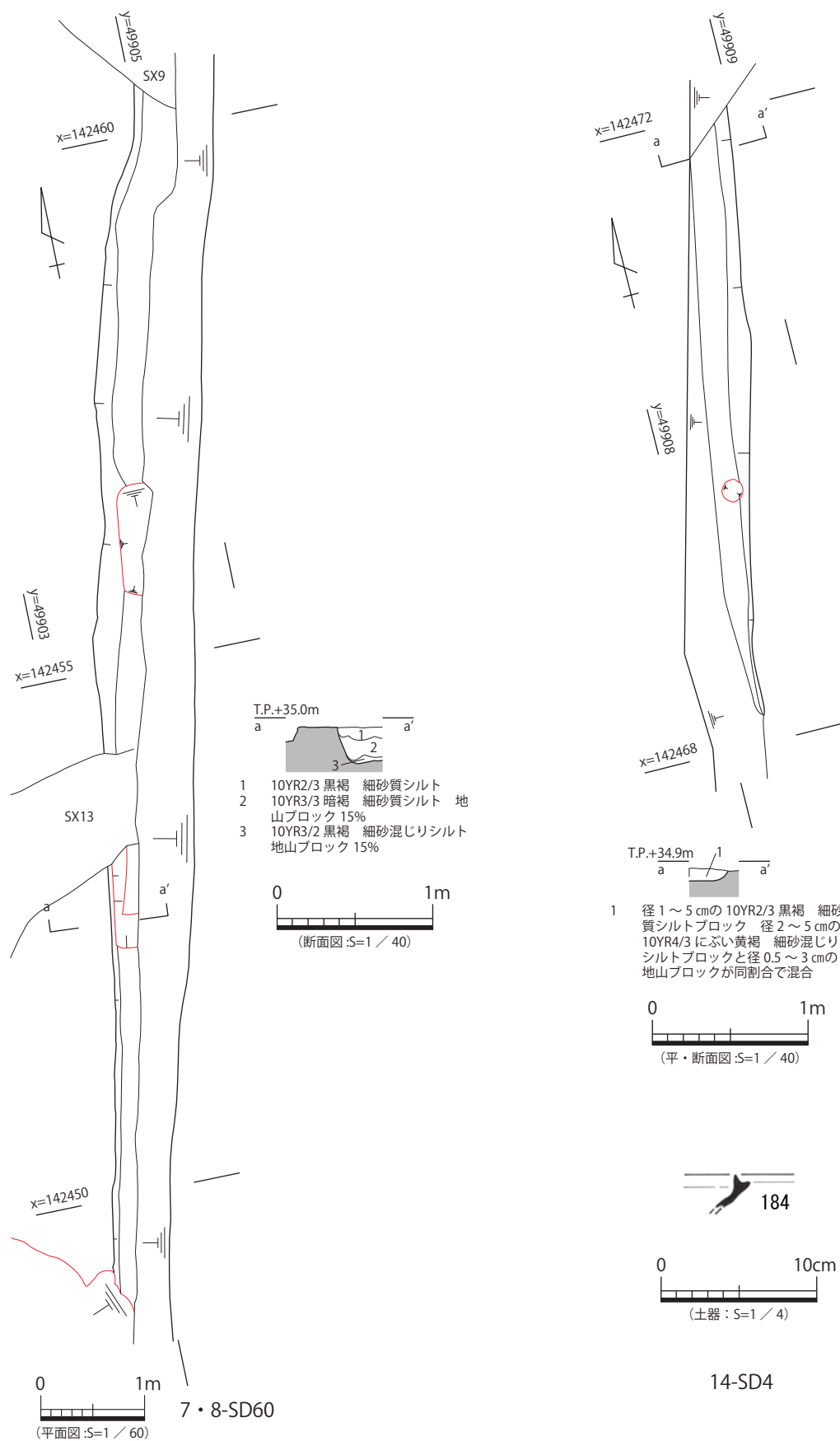
図 79 7・8-SD60、14-SD 4 平・断面図、出土遺物実測図
