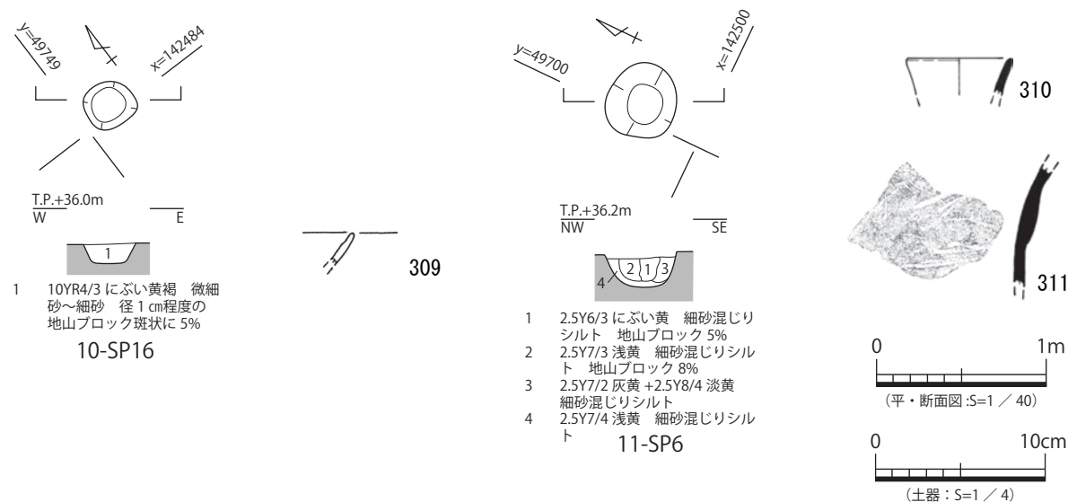
図 115 10-SP16、11-SP 6 平・断面図、出土遺物実測図
