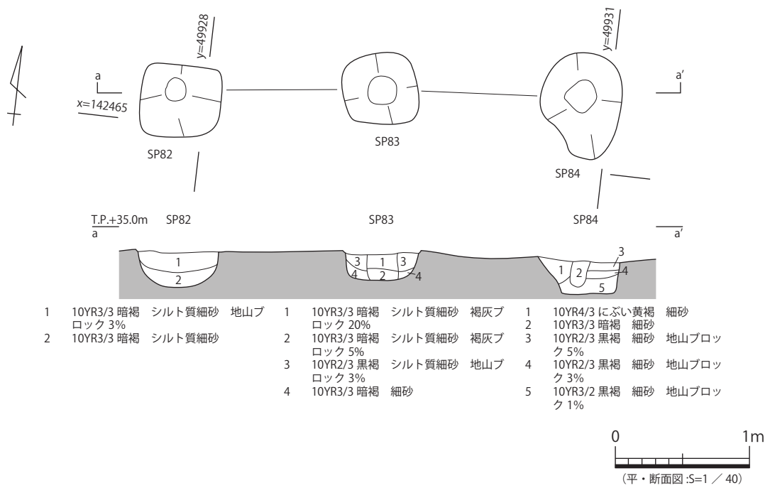
図 65 4-掘立 5 平・断面図
