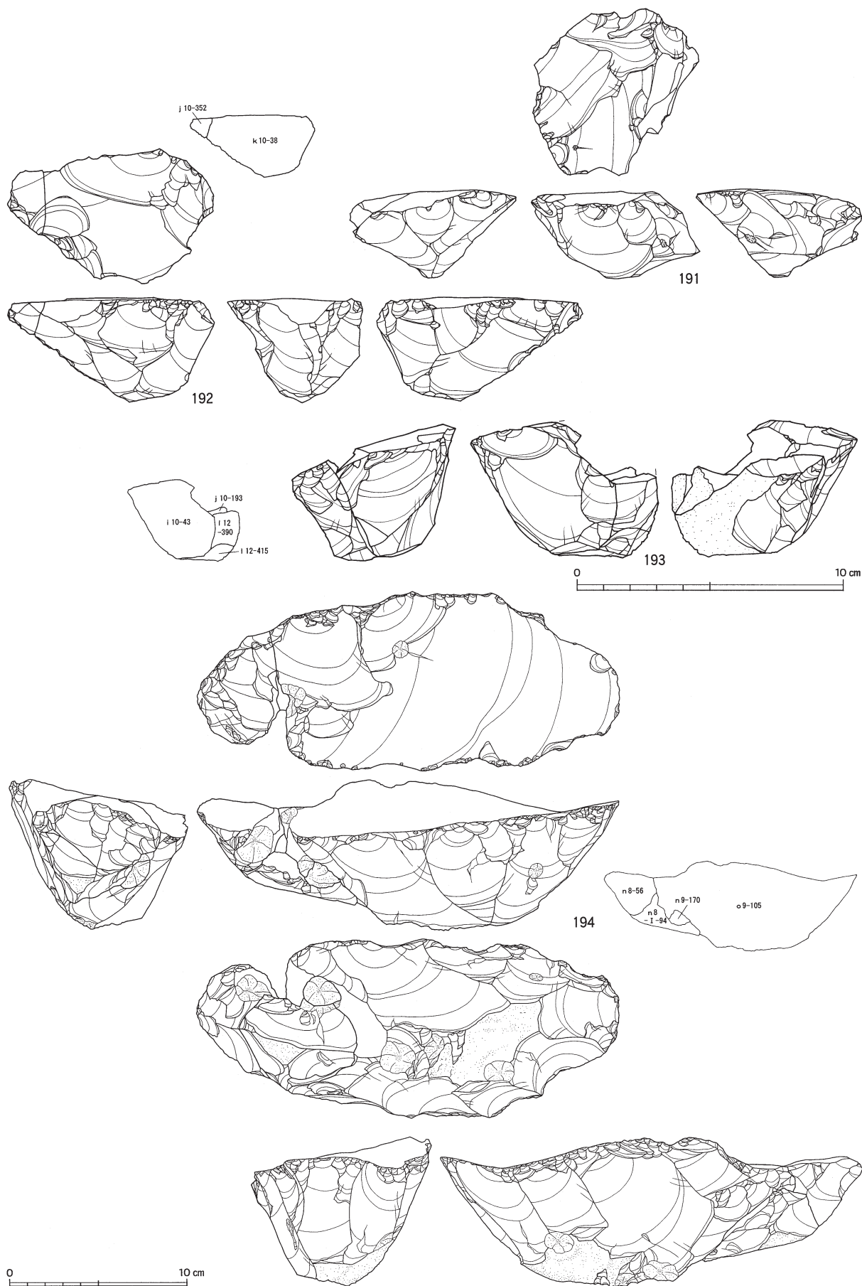
図Ⅲ-378 Sb-38~44の石器(30) 石核
