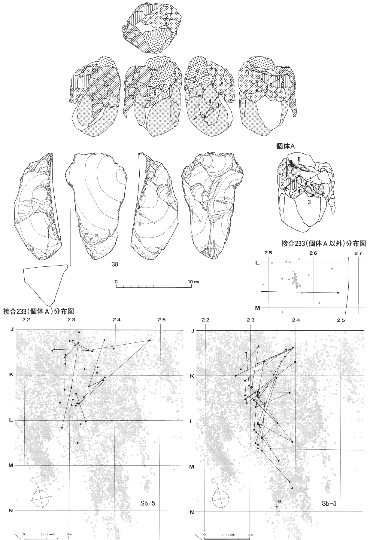
図IV-46 Sb-5の石器(23) 母岩81・接合233(2)
