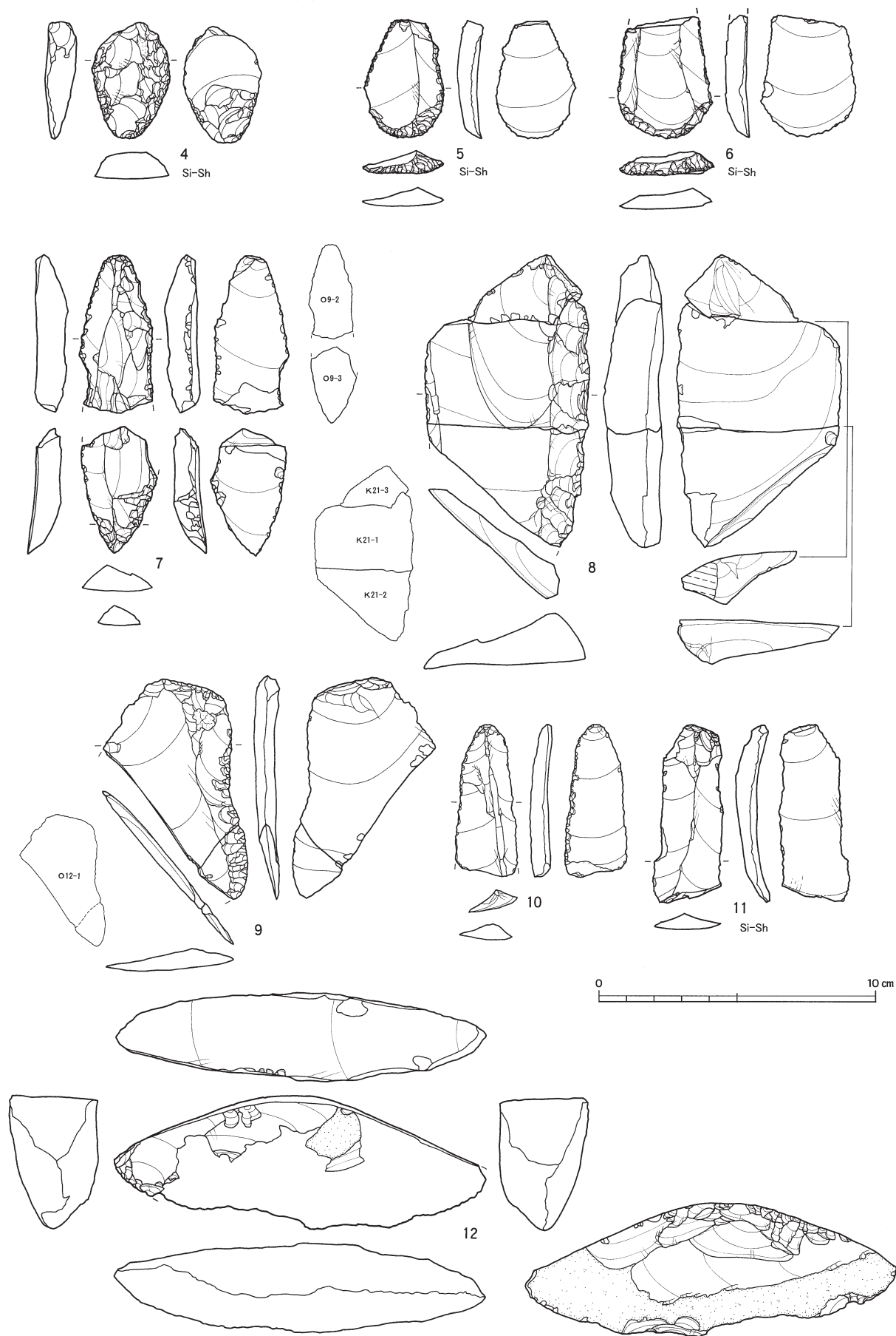
図Ⅲ-426 石器ブロック外の石器(2) 彫器・搔器・削器・二次加工ある剥片・石刃・舟底形石器
