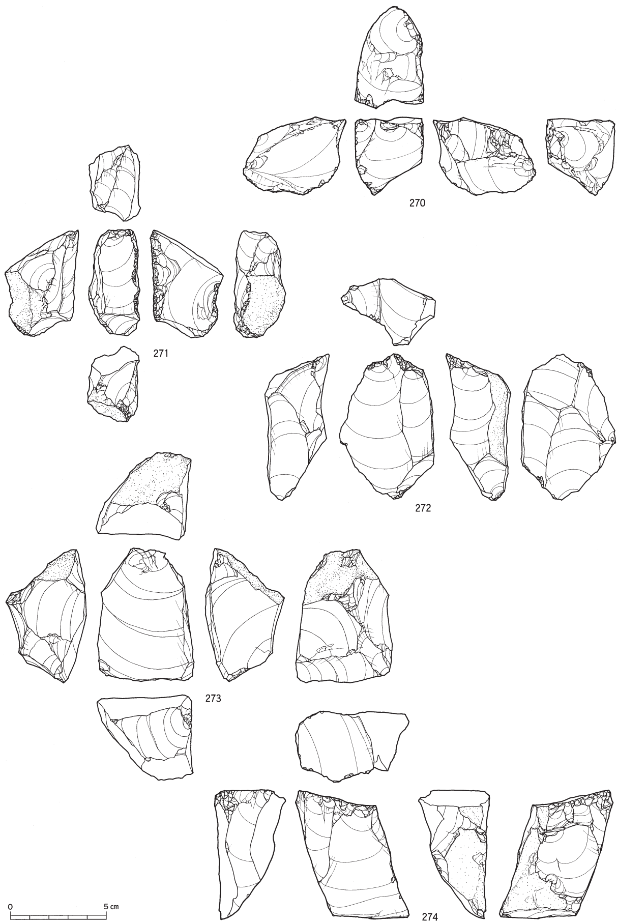
図IV-93 Sb-6~11の石器(16) 石核
