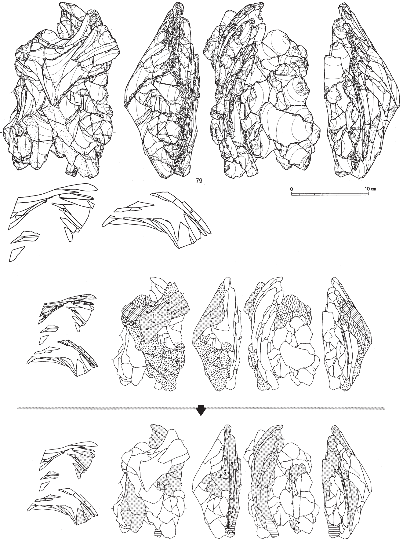
図IV-72 Sb-5の石器(49) 母岩34・接合118(1)
