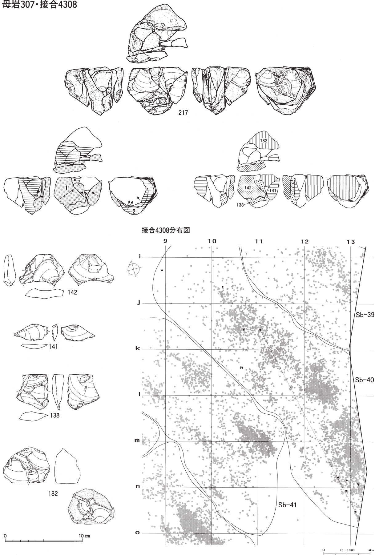
図Ⅲ-418 Sb-38~44の石器(49) 母岩307・接合4308
