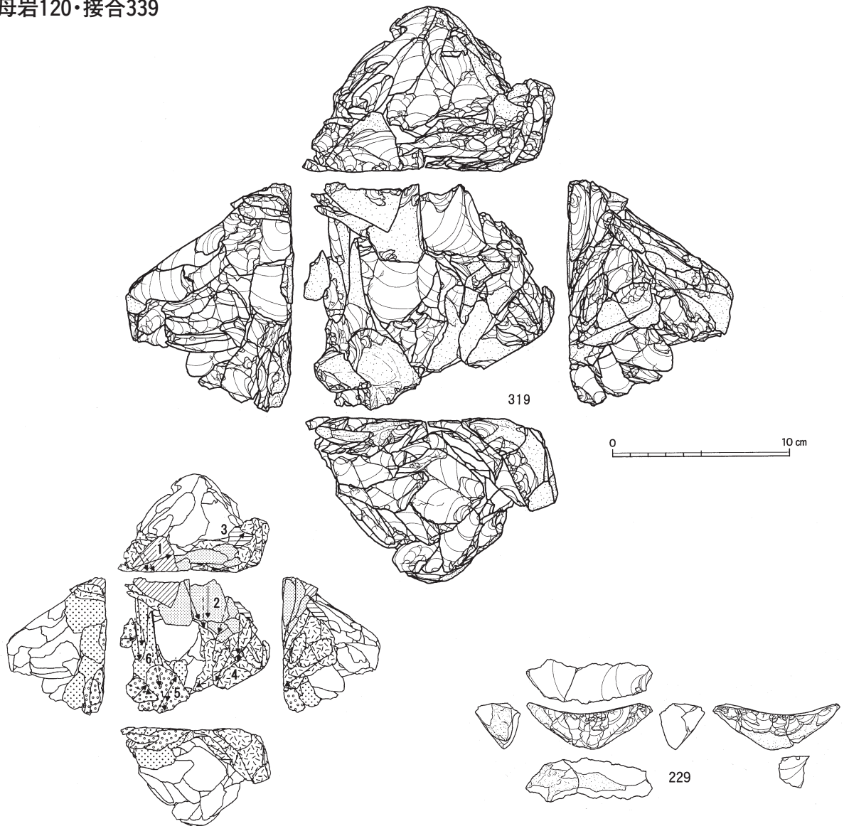
図IV-130 Sb-6~11の石器(39) 母岩170・接合592(2)、母岩120・接合339(1)
