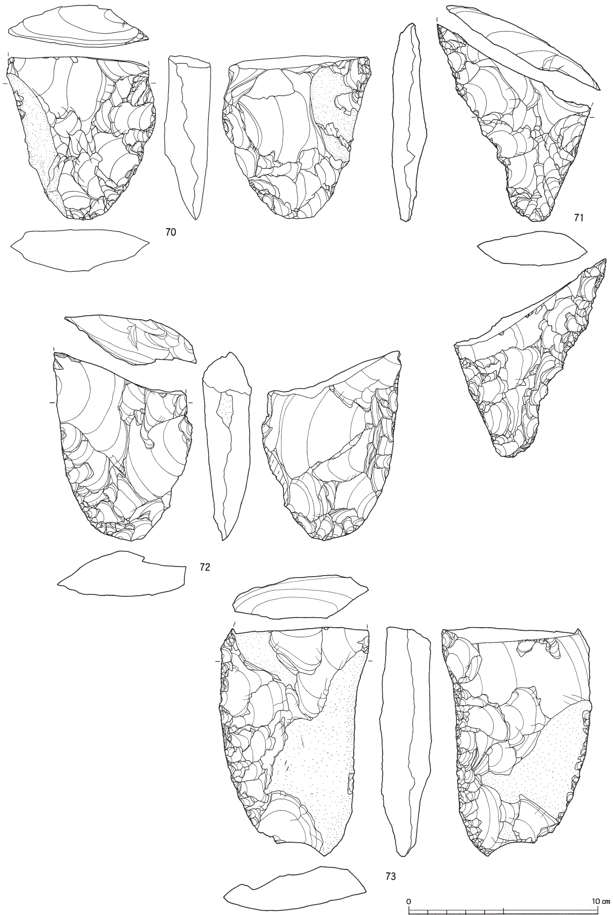
図Ⅲ-361 Sb-38~44の石器(13) 尖頭器
