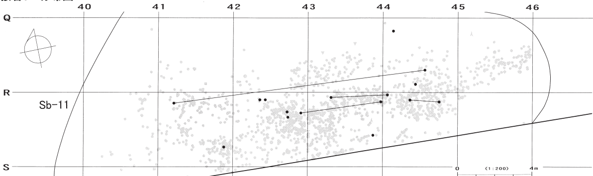
接合574分布図
