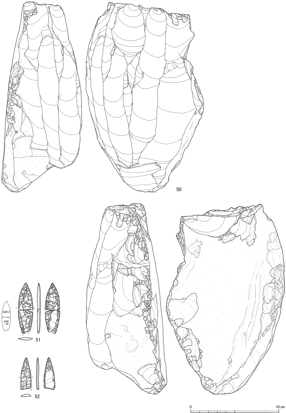
図Ⅲ-327 Sb-31~36の石器(6) 石刃核・石鏃
