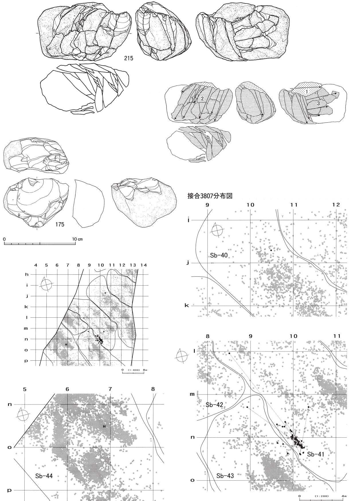
図Ⅲ-415 Sb-38~44の石器(46) 母岩393・接合3807
