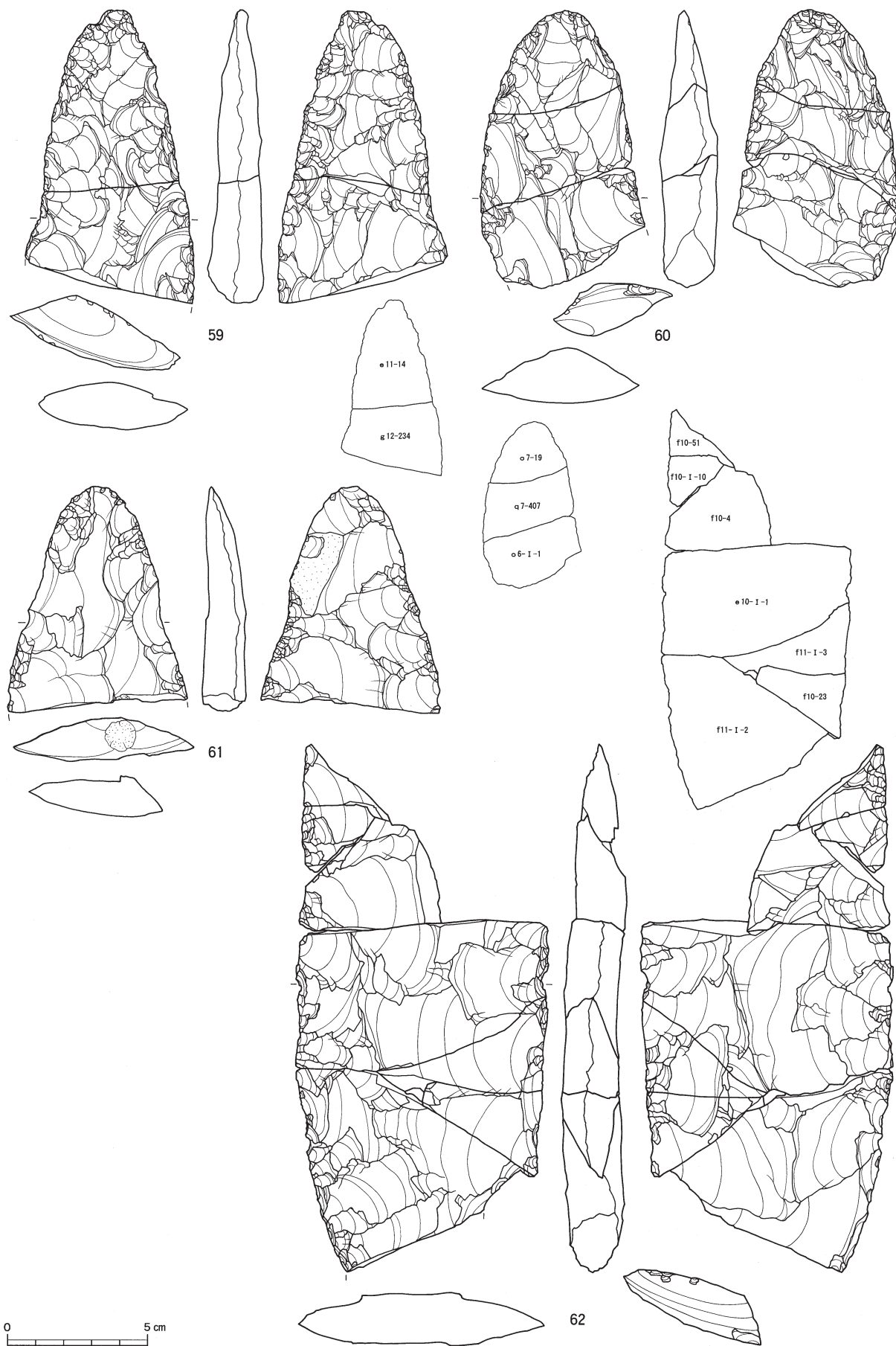
図Ⅲ-358 Sb-38~44の石器(10) 尖頭器
