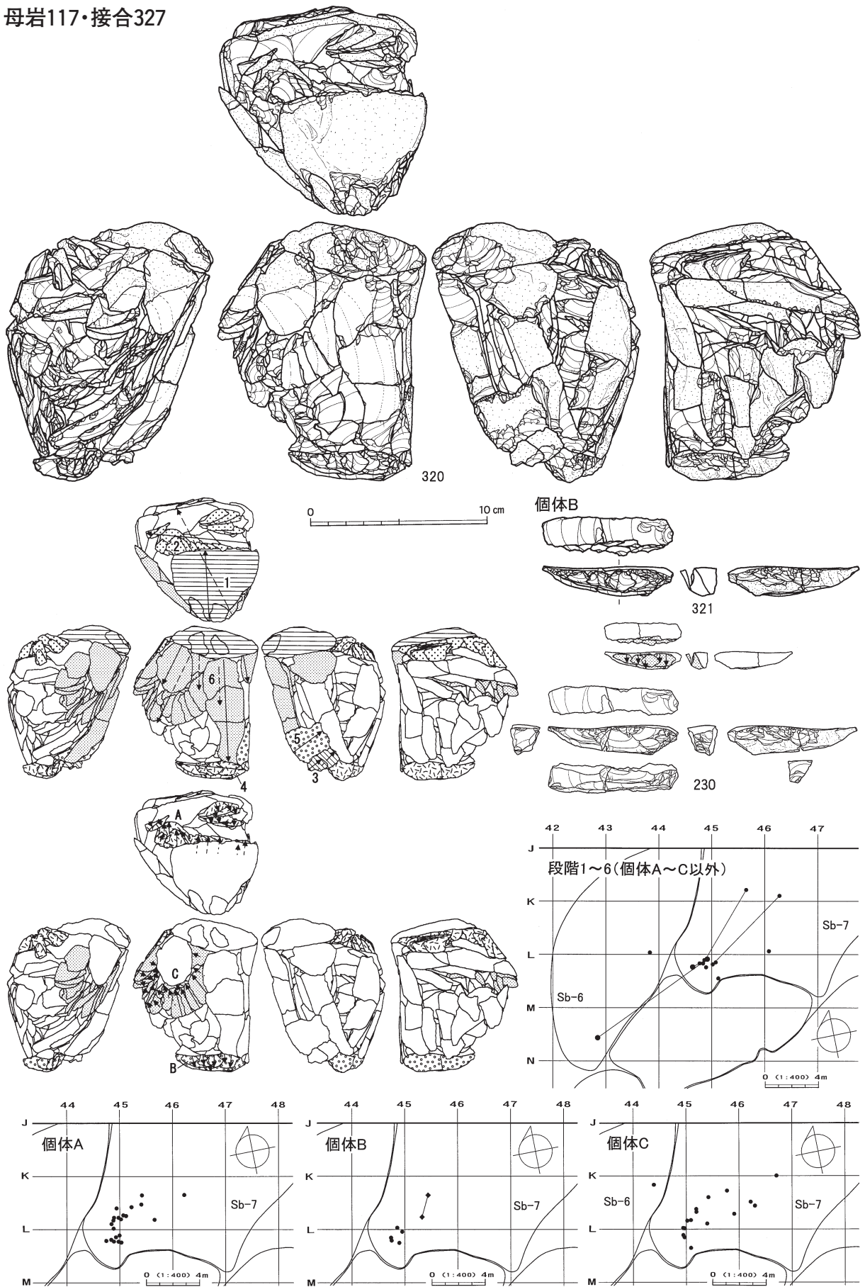
図IV-132 Sb-6~11の石器(41) 母岩117・接合327(1)
