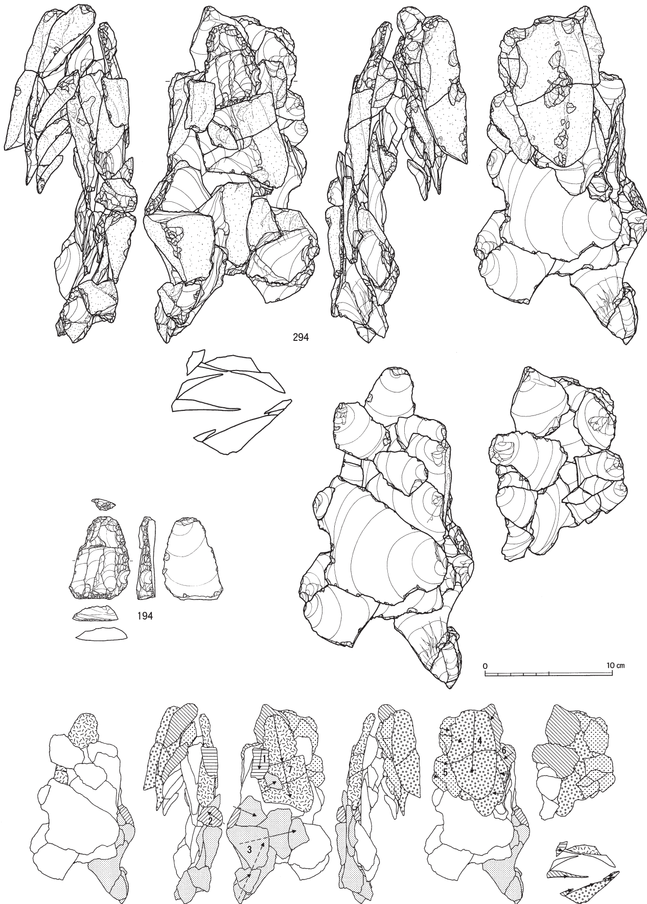
図Ⅳ-117 Sb-6~11の石器(26) 母岩137・接合439(1)
