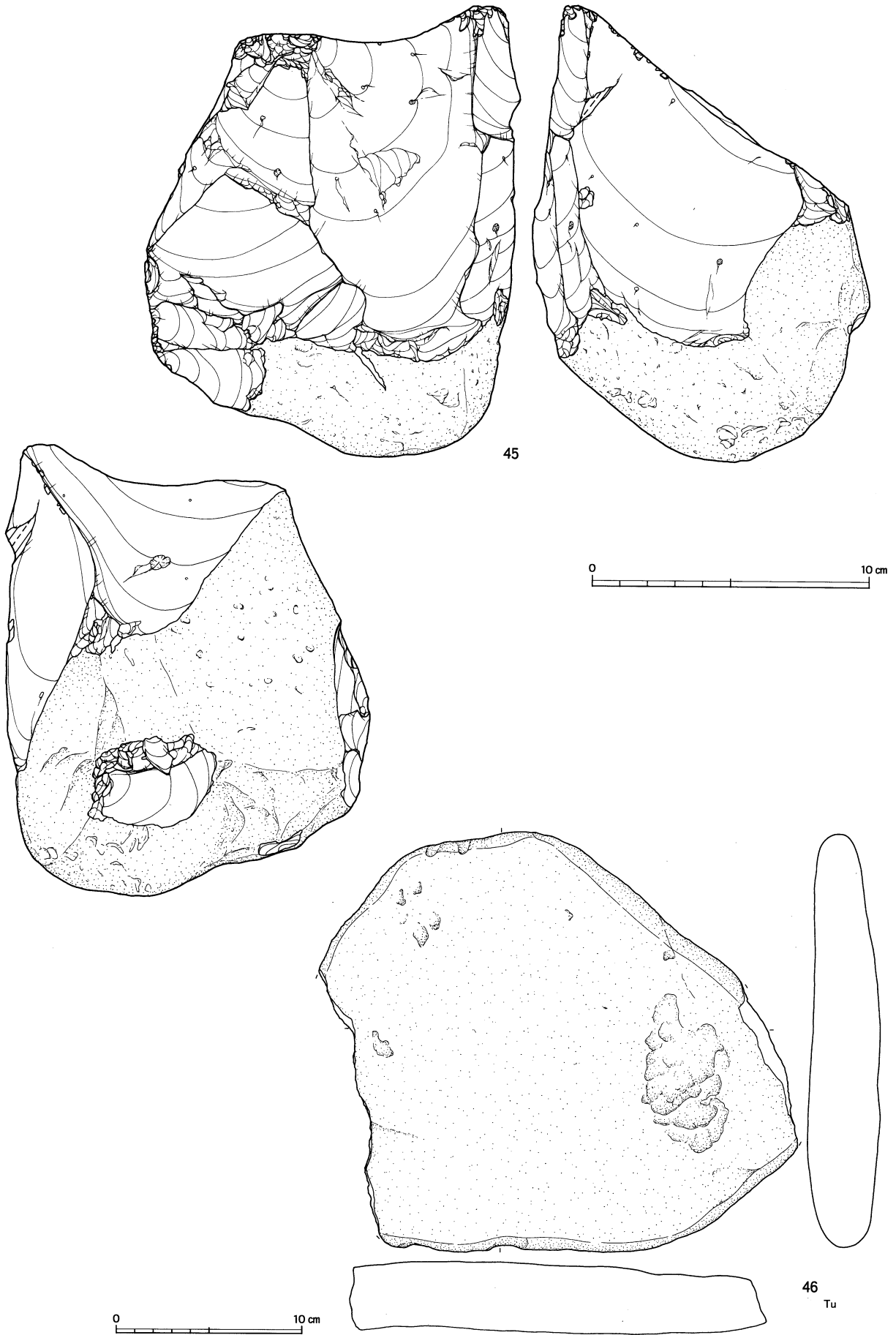
図V-13 Sb-5の石器(4)
