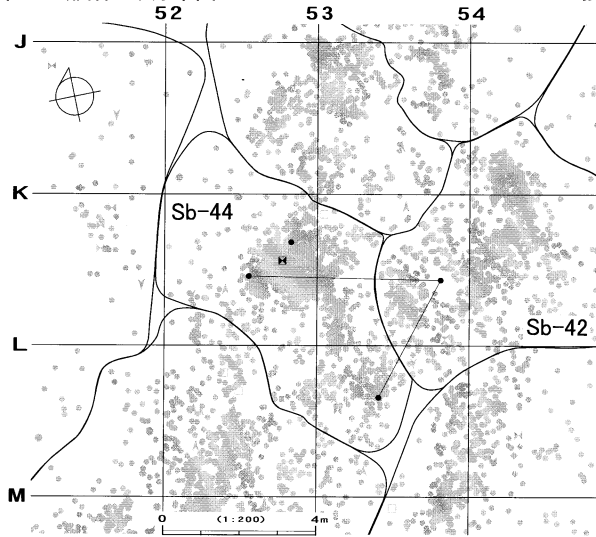
母岩346・接合1703
