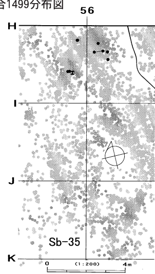
接合1499分布図
