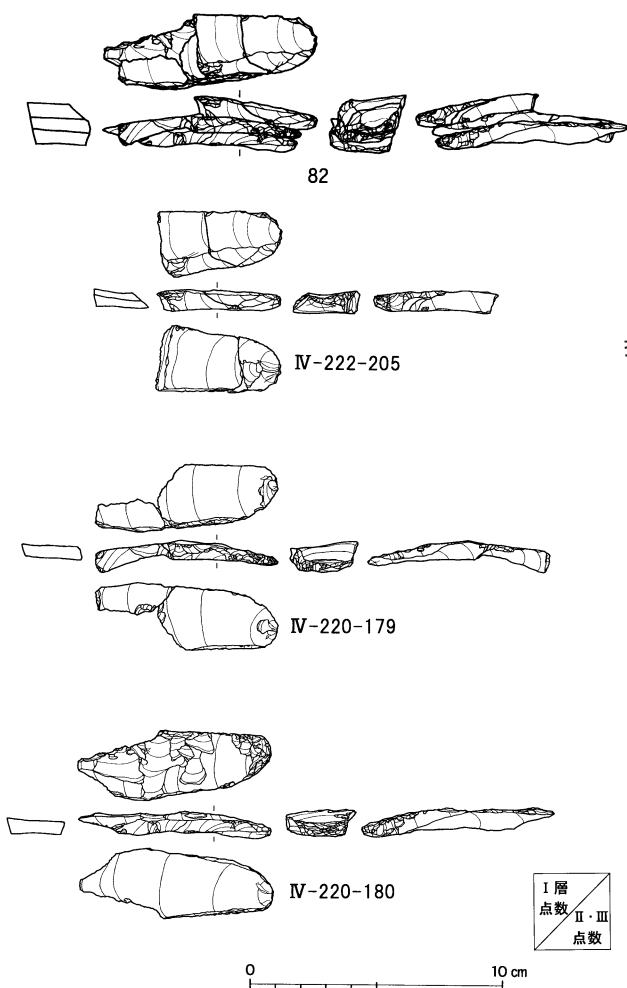
母岩259・接合1457
