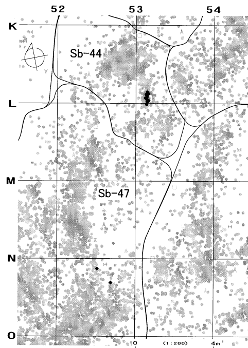
接合1579分布図
