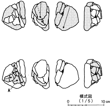
母岩359・接合1738
