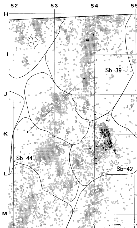
接合1573分布図
