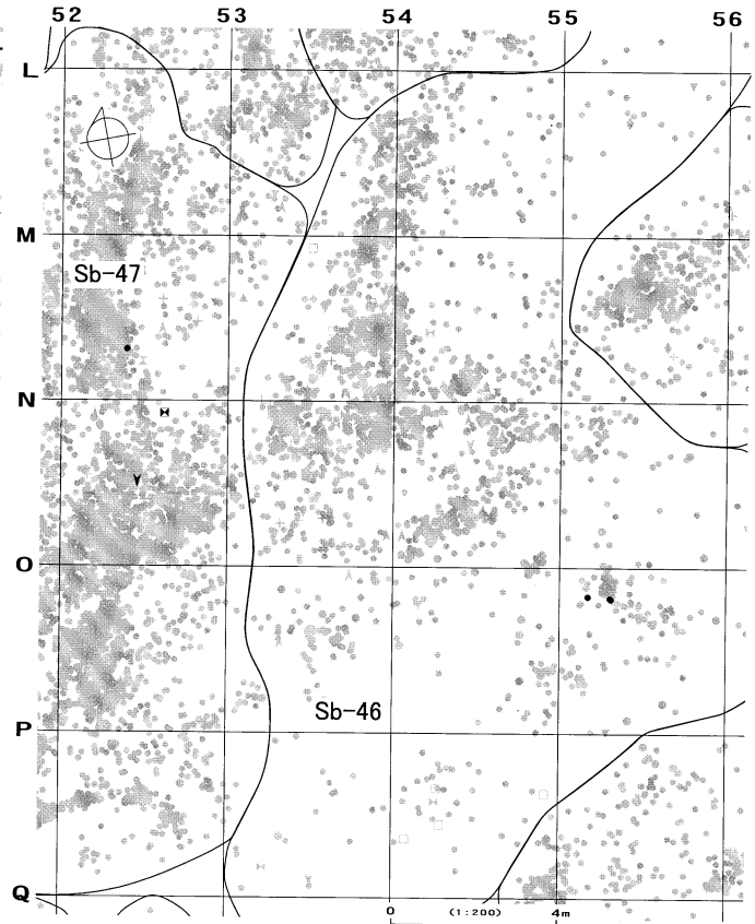
接合1738分布图
