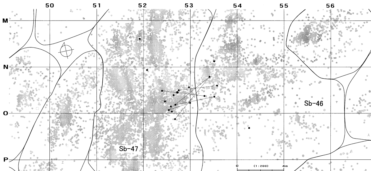
接合1699分布図
