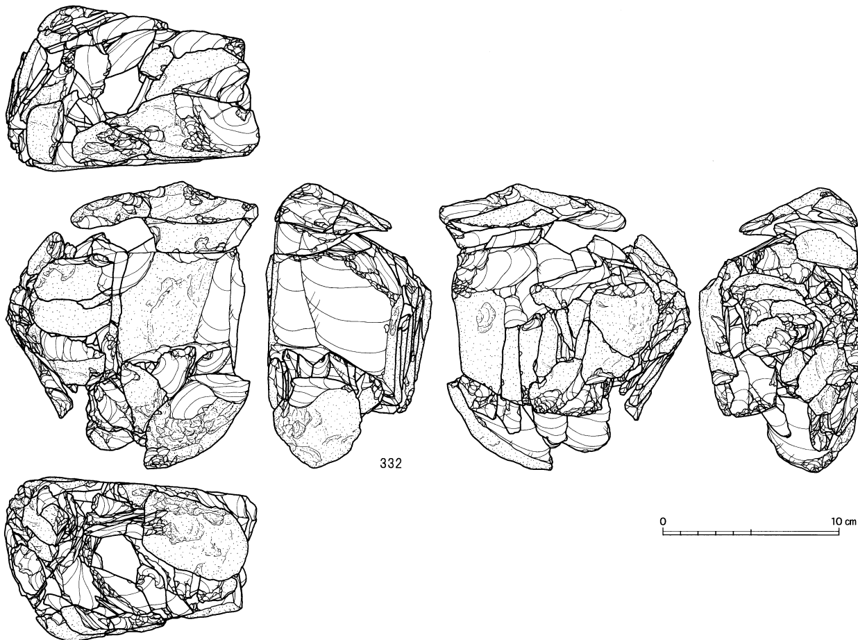
母岩366・接合1759
