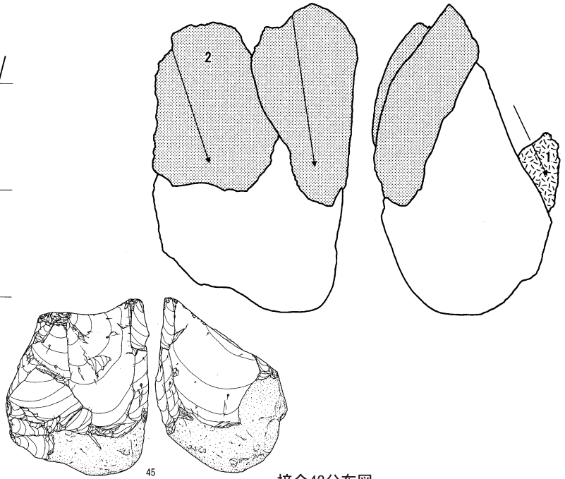
接合42分布図
