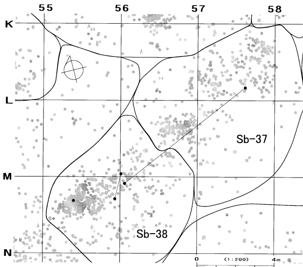
母岩338・接合1687
