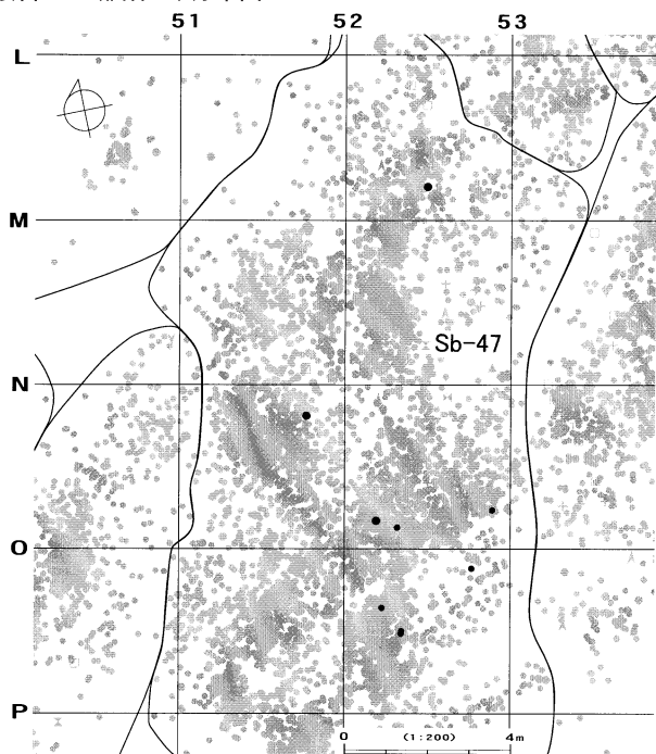
母岩268・接合1491
