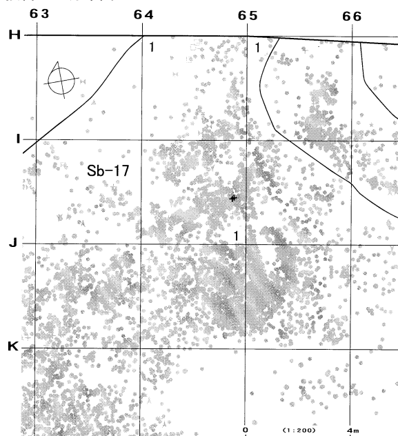
接合1457分布図
