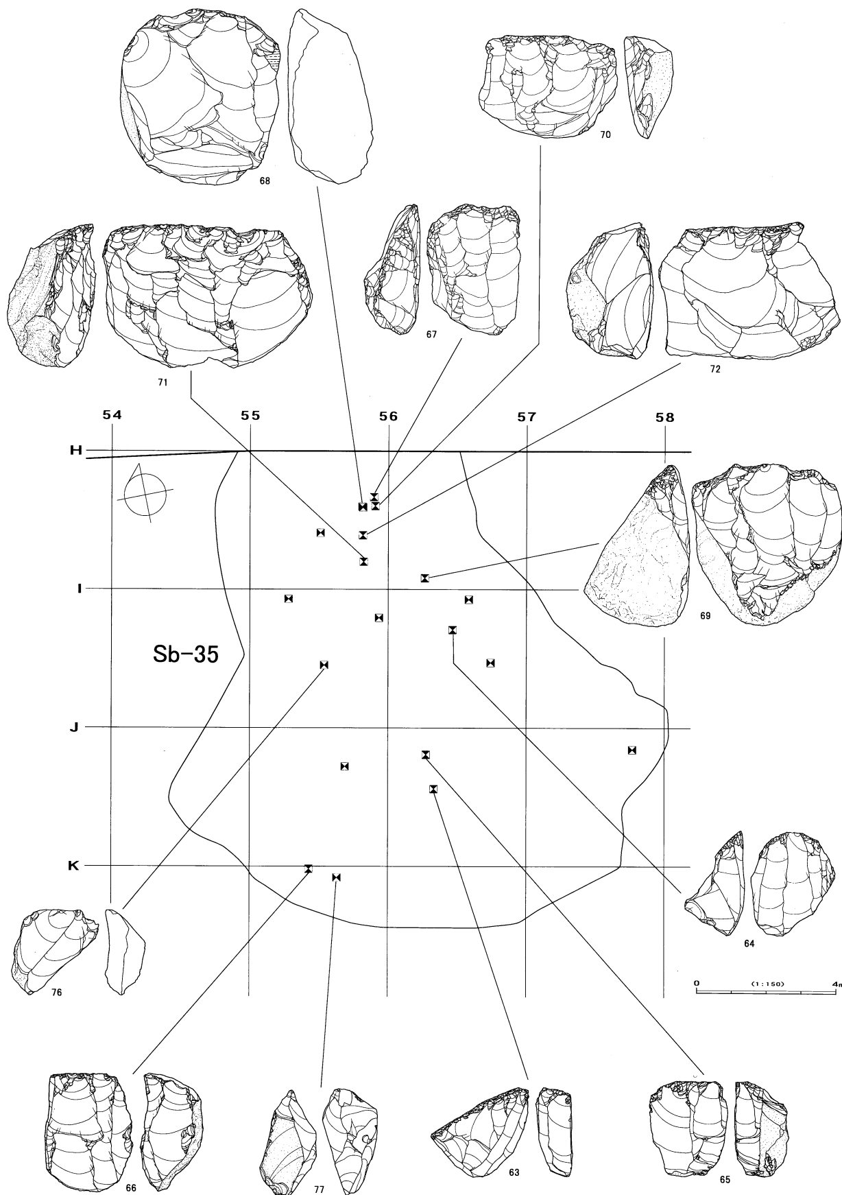
図IV-393 Sb-35の遺物(2)
