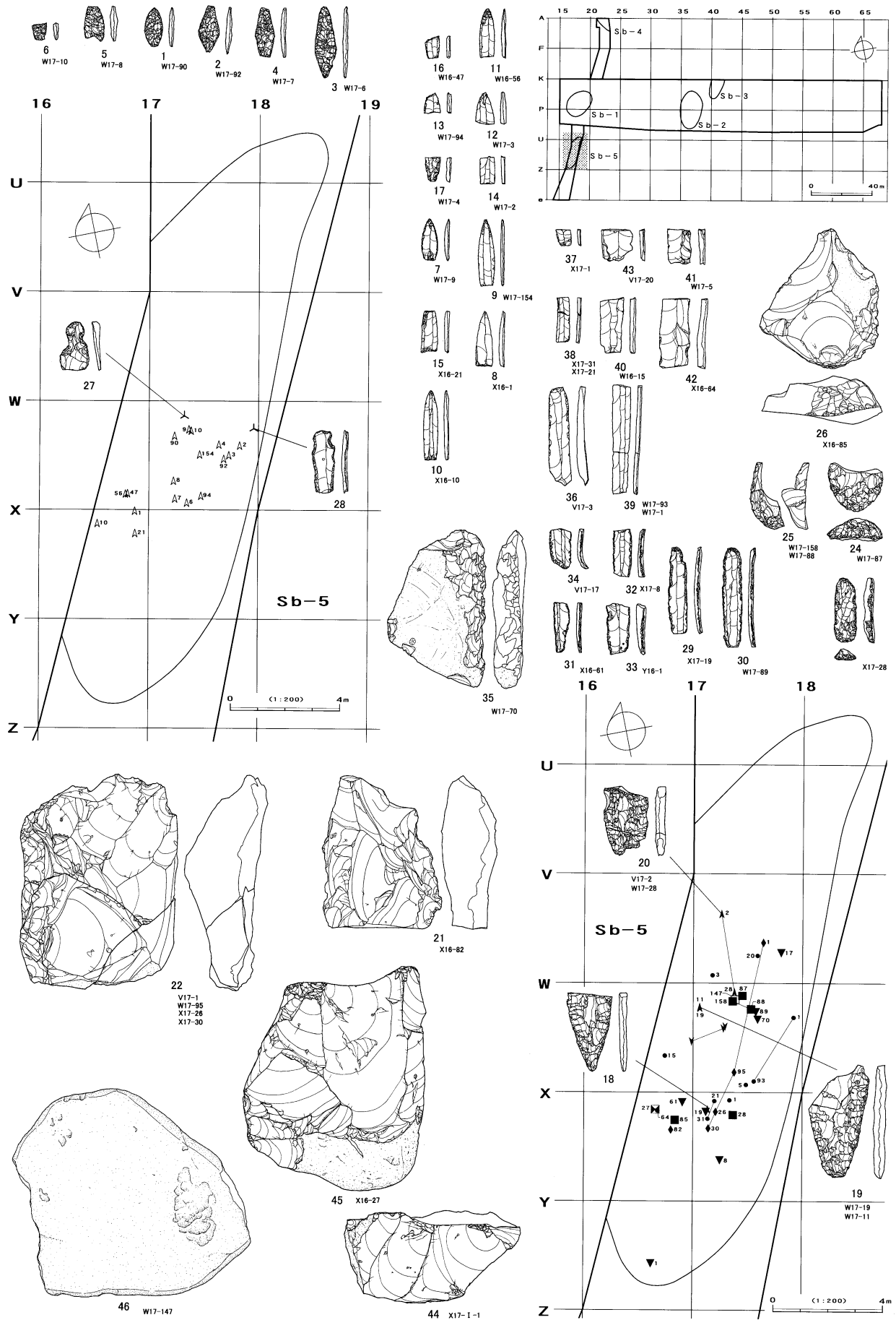
図V-15 Sb-5の遺物
