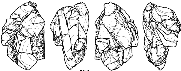
母岩338・接合1687
