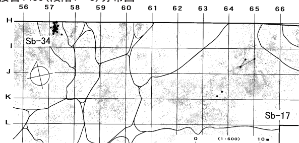
母岩259・接合1457
