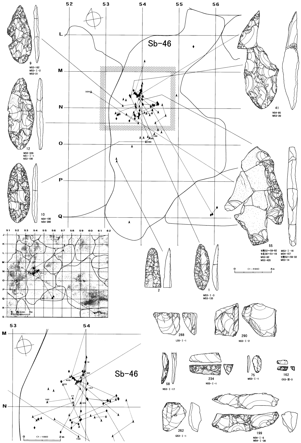
図IV-474 Sb-46の遺物(1)
