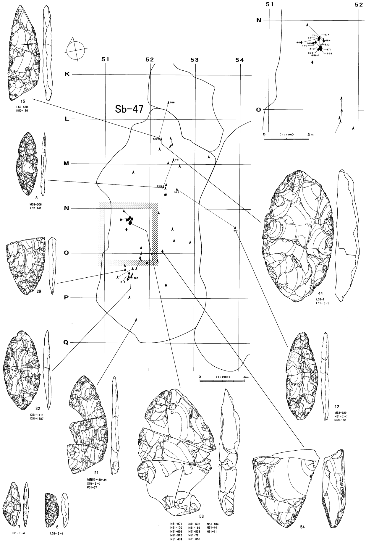
図IV-477 Sb-47の遺物(1)
