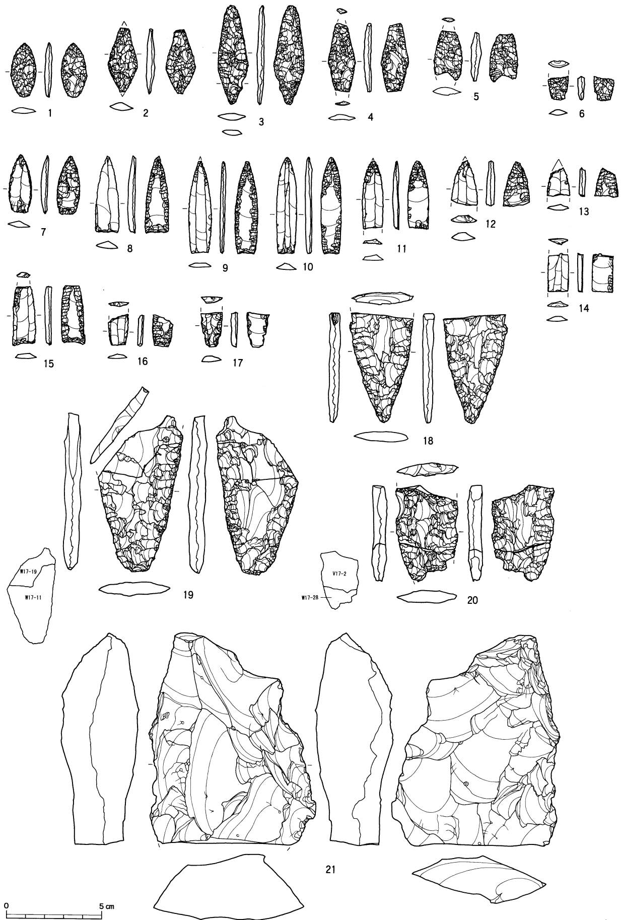
図V-10 Sb-5の石器(1)
