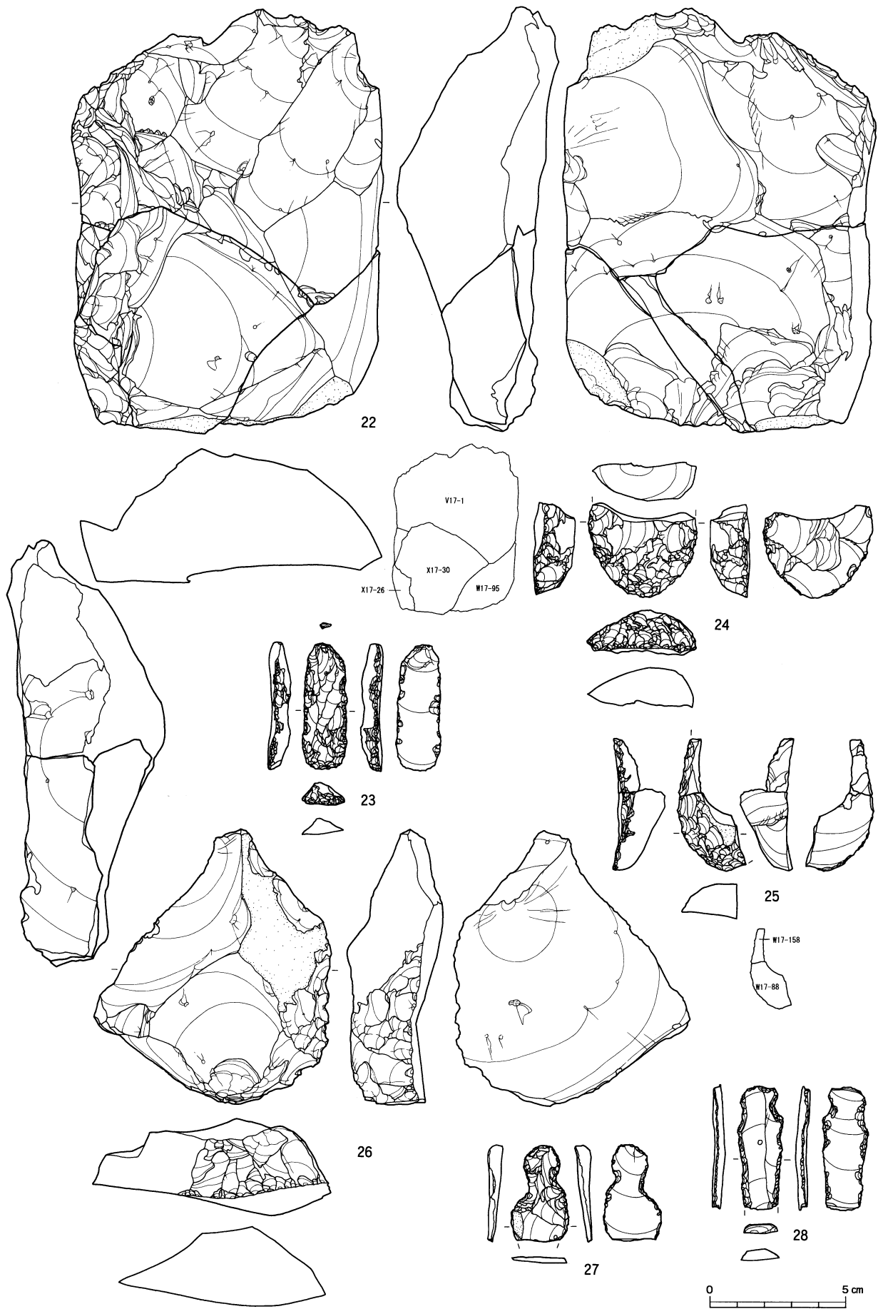
図V-11 Sb-5の石器(2)
