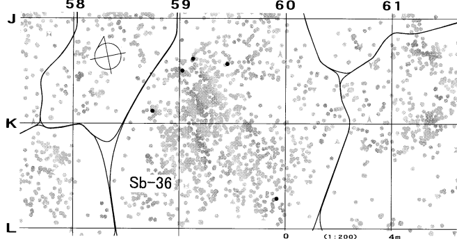
母岩342・接合1697
