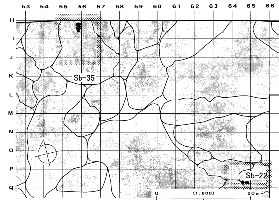
接合1257分布図
