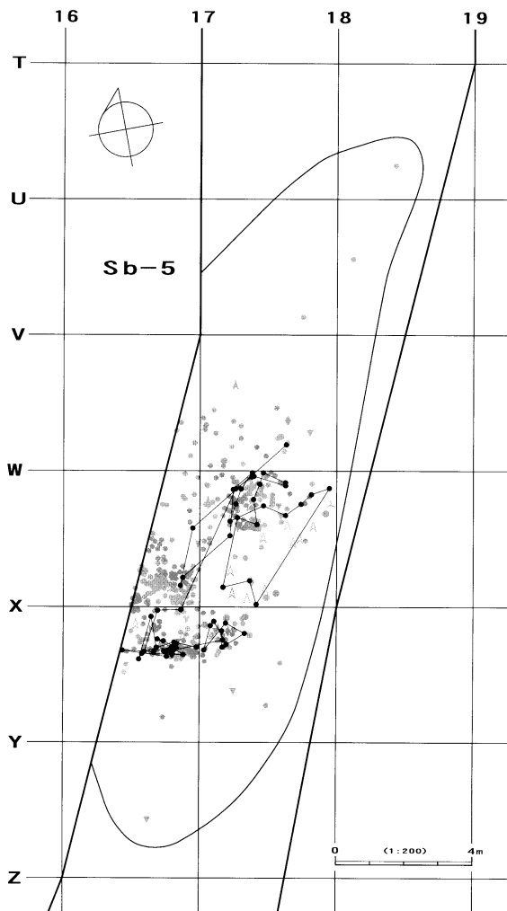
接合44分布図
