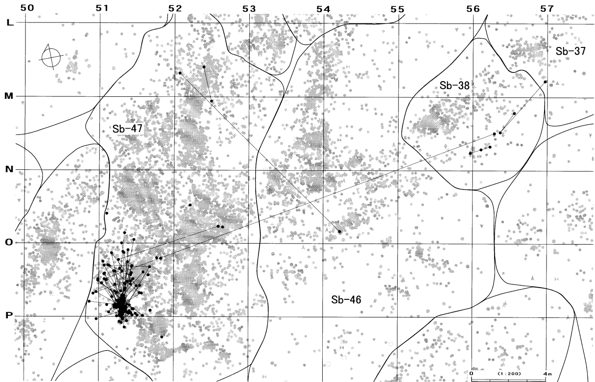
母岩345・接合1700
