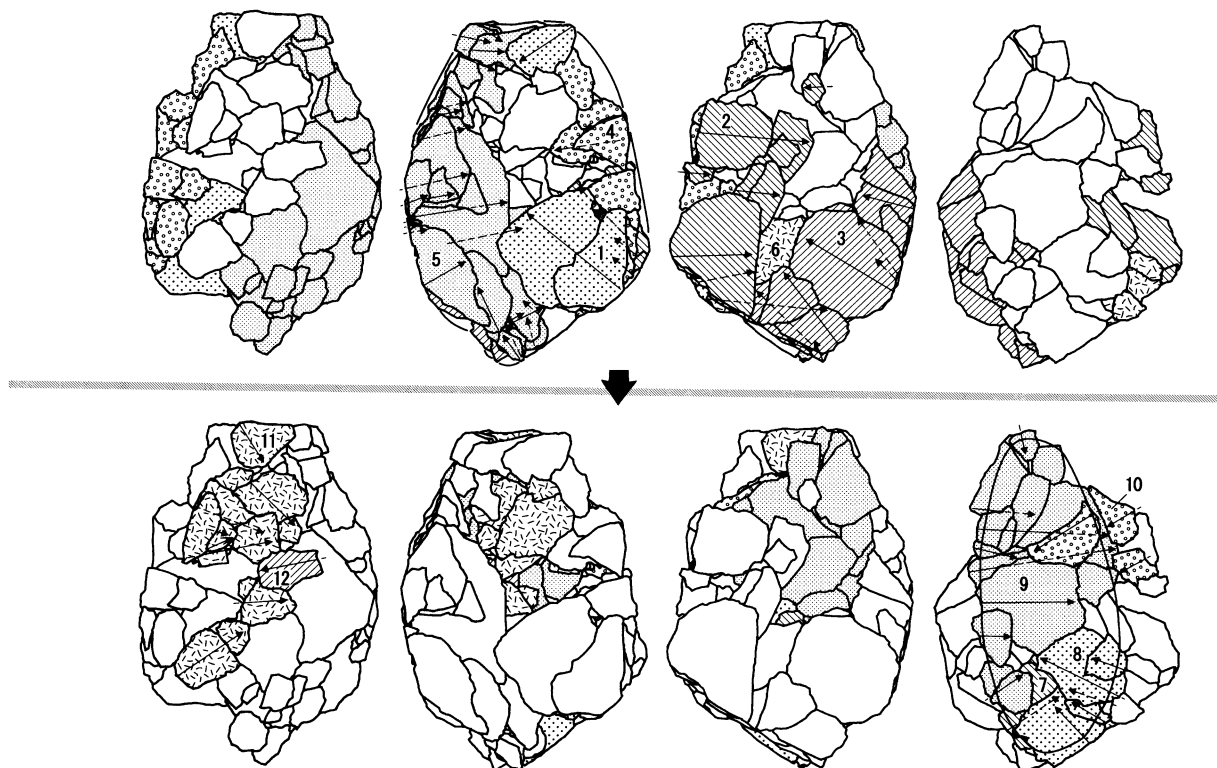
接合1488分布図
