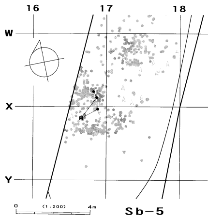
接合41分布図
