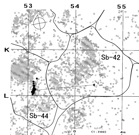
接合1577分布図
