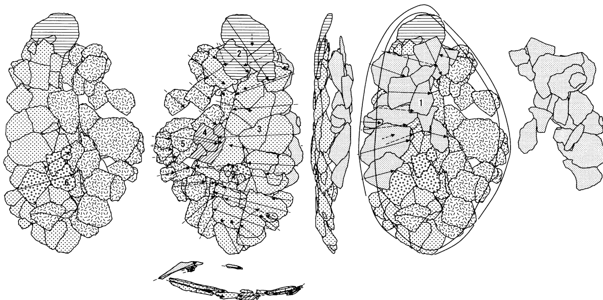
接合2029分布図
