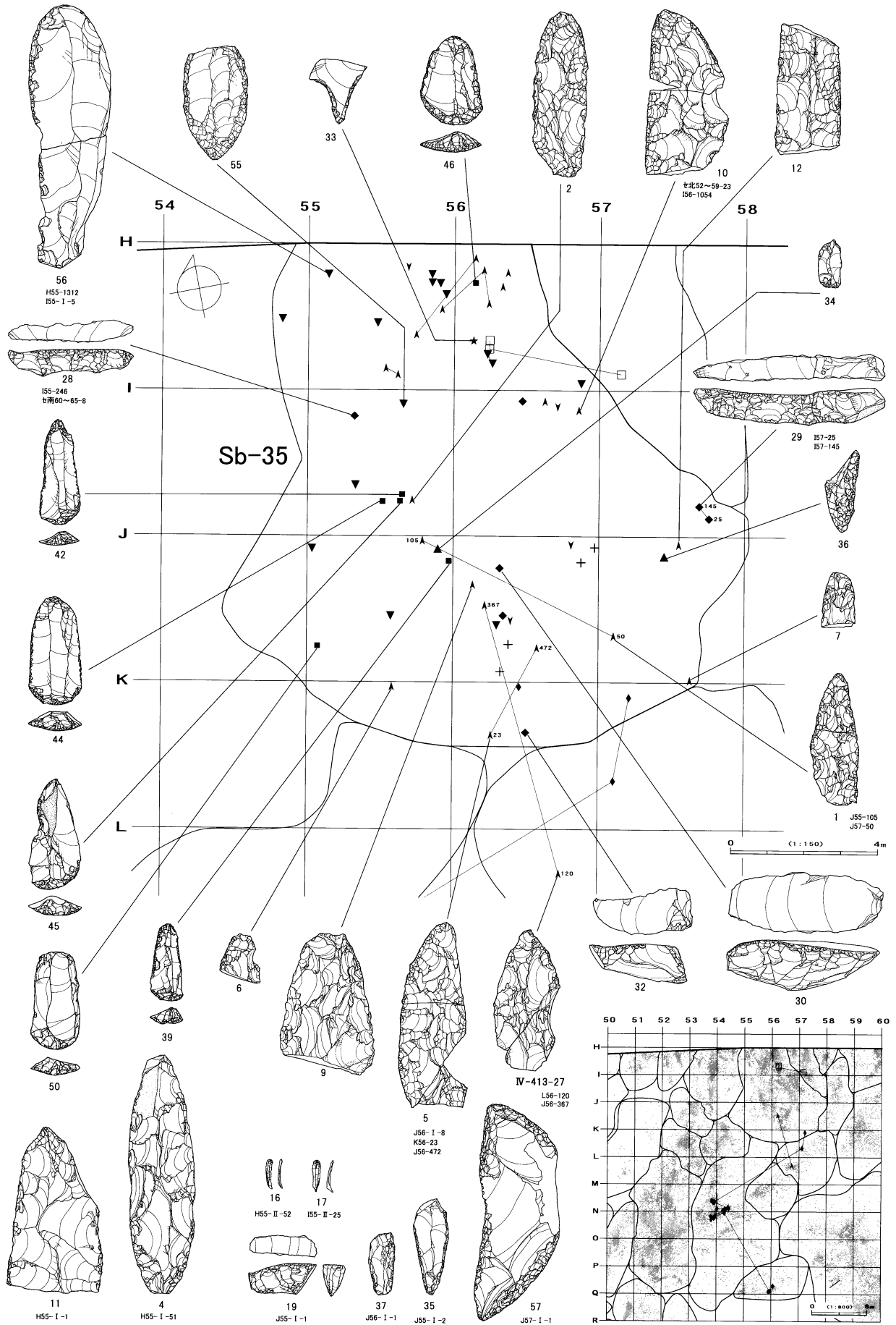
図IV-392 Sb-35の遺物(1)
