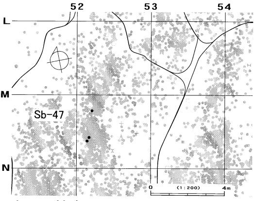
母岩359・接合1738
