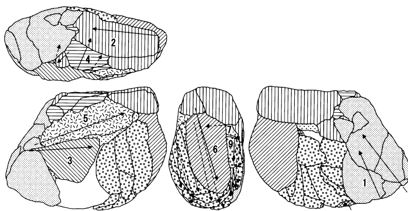
接合1715分布図 8
