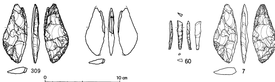
母岩2624
