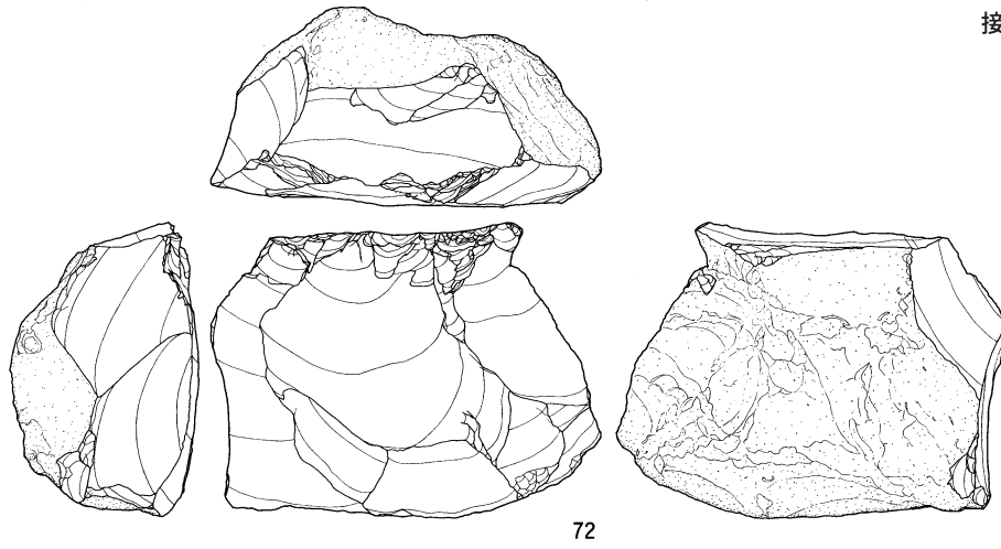
母岩343・接合1698
