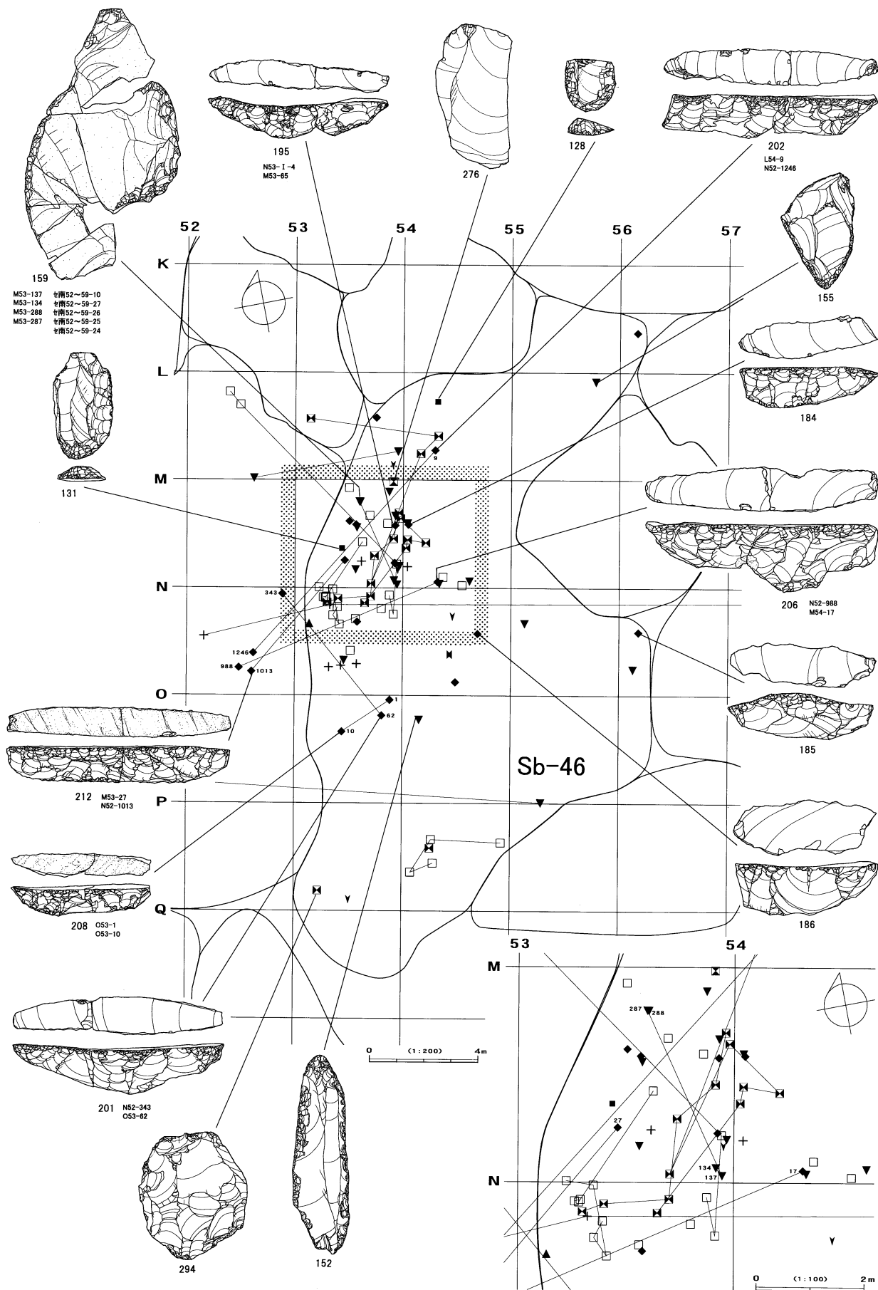
図IV-475 Sb-46の遺物(2)
