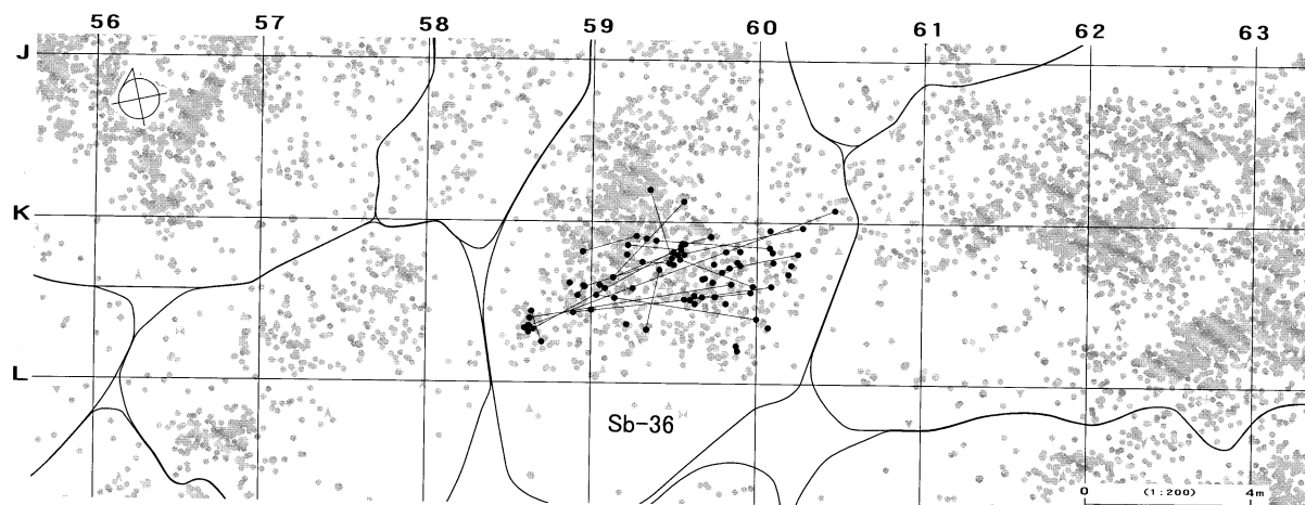
接合1577分布図
