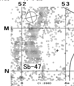
接合2624分布図
