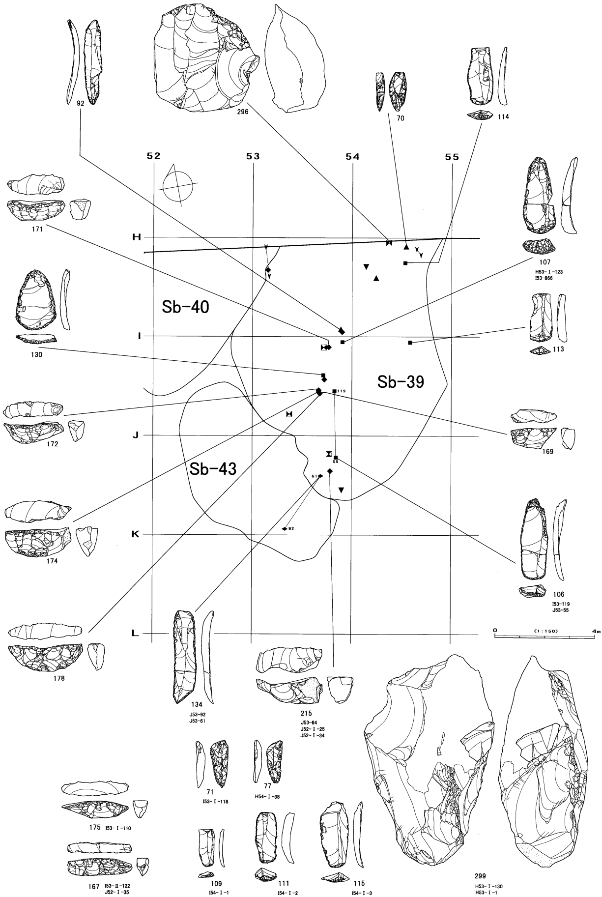
図IV-468 Sb-39の遺物
