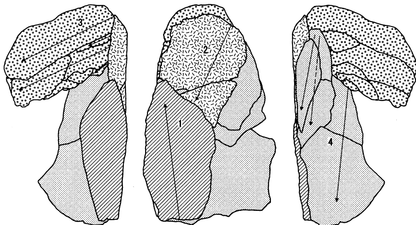
接合43分布図
