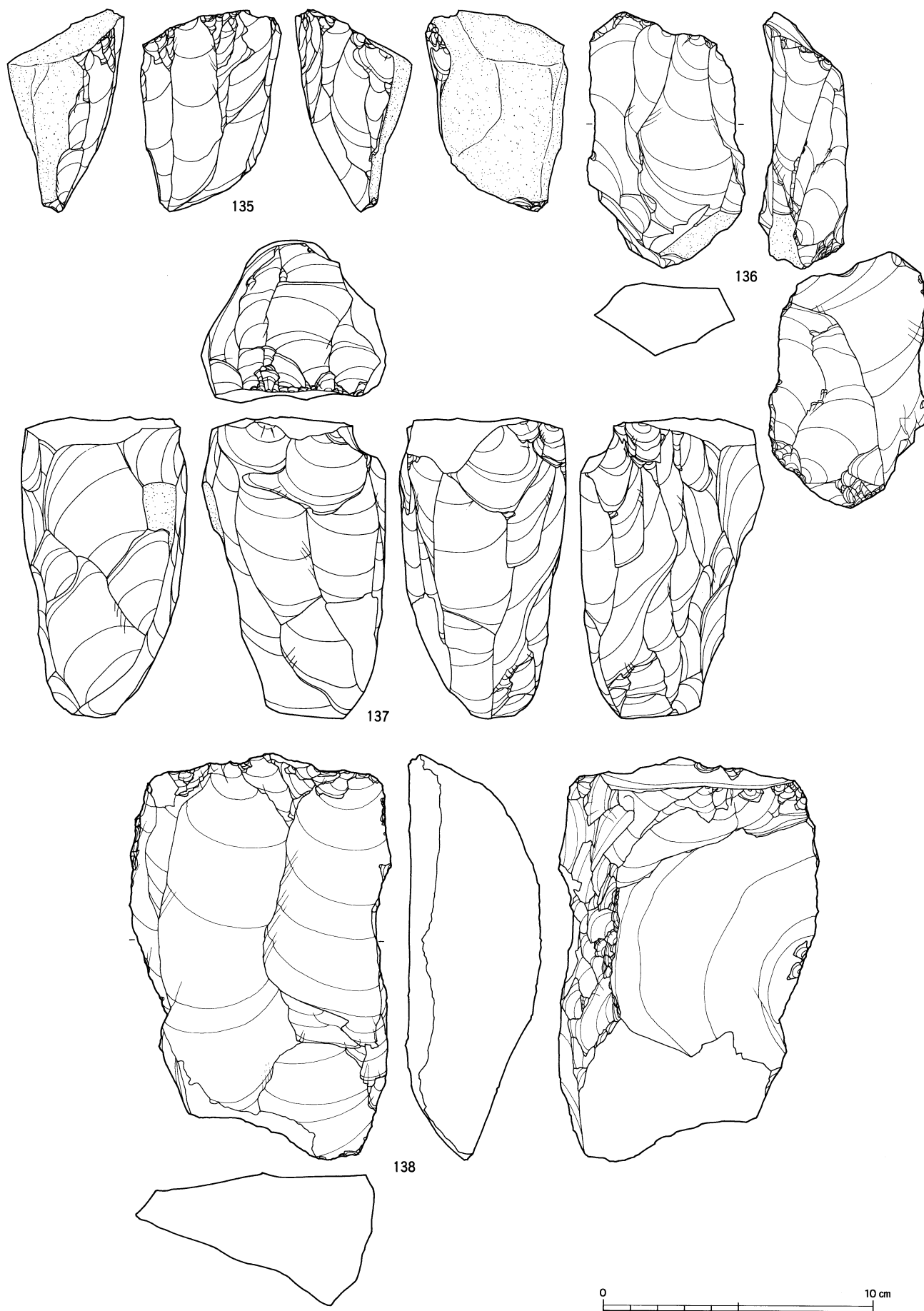
図IV-323 B区(Sb-20~29)の石器(33) 石刃核
