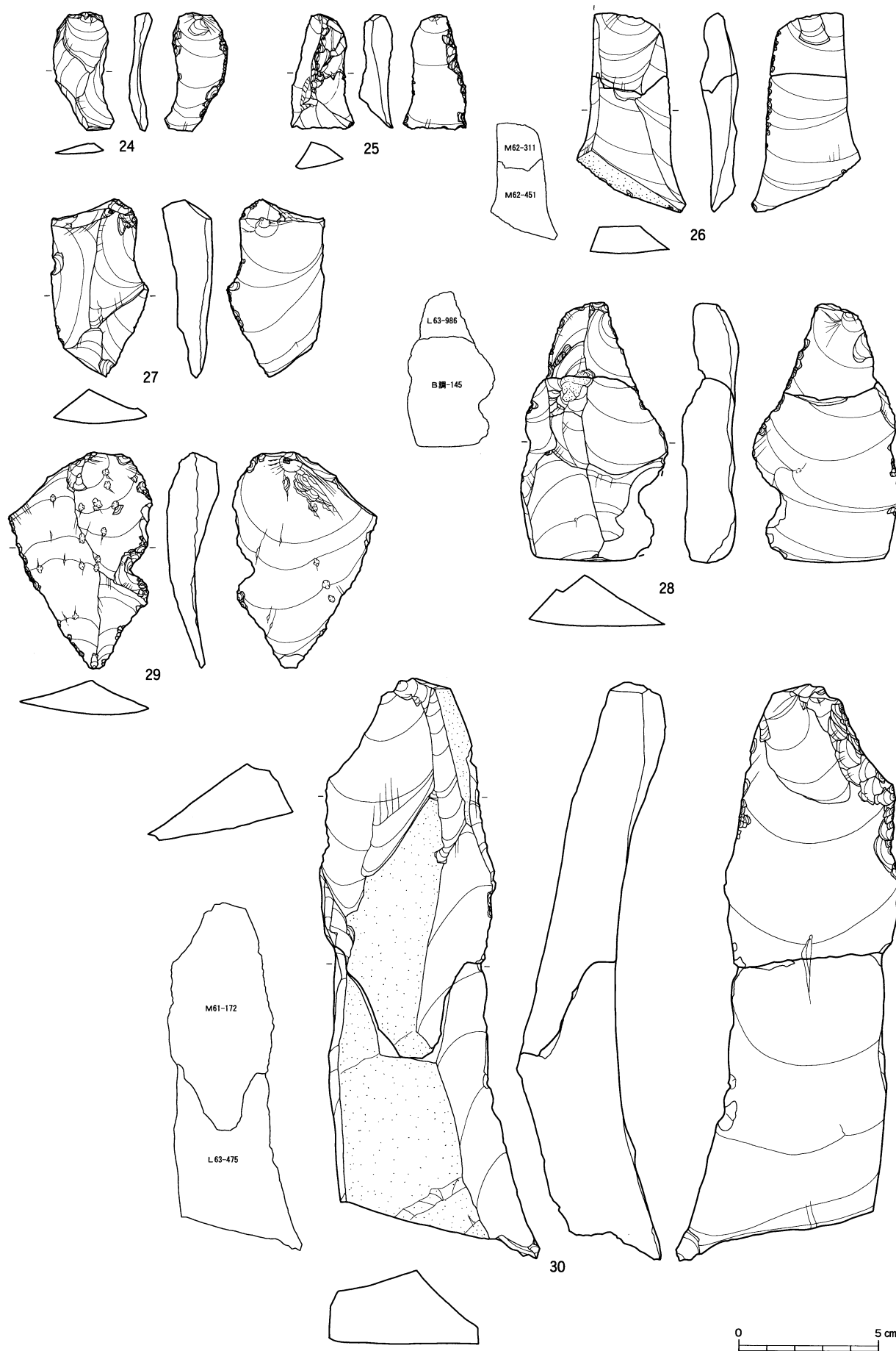
図IV-69 Sb-4~6の石器(2) 二次加工ある剥片
