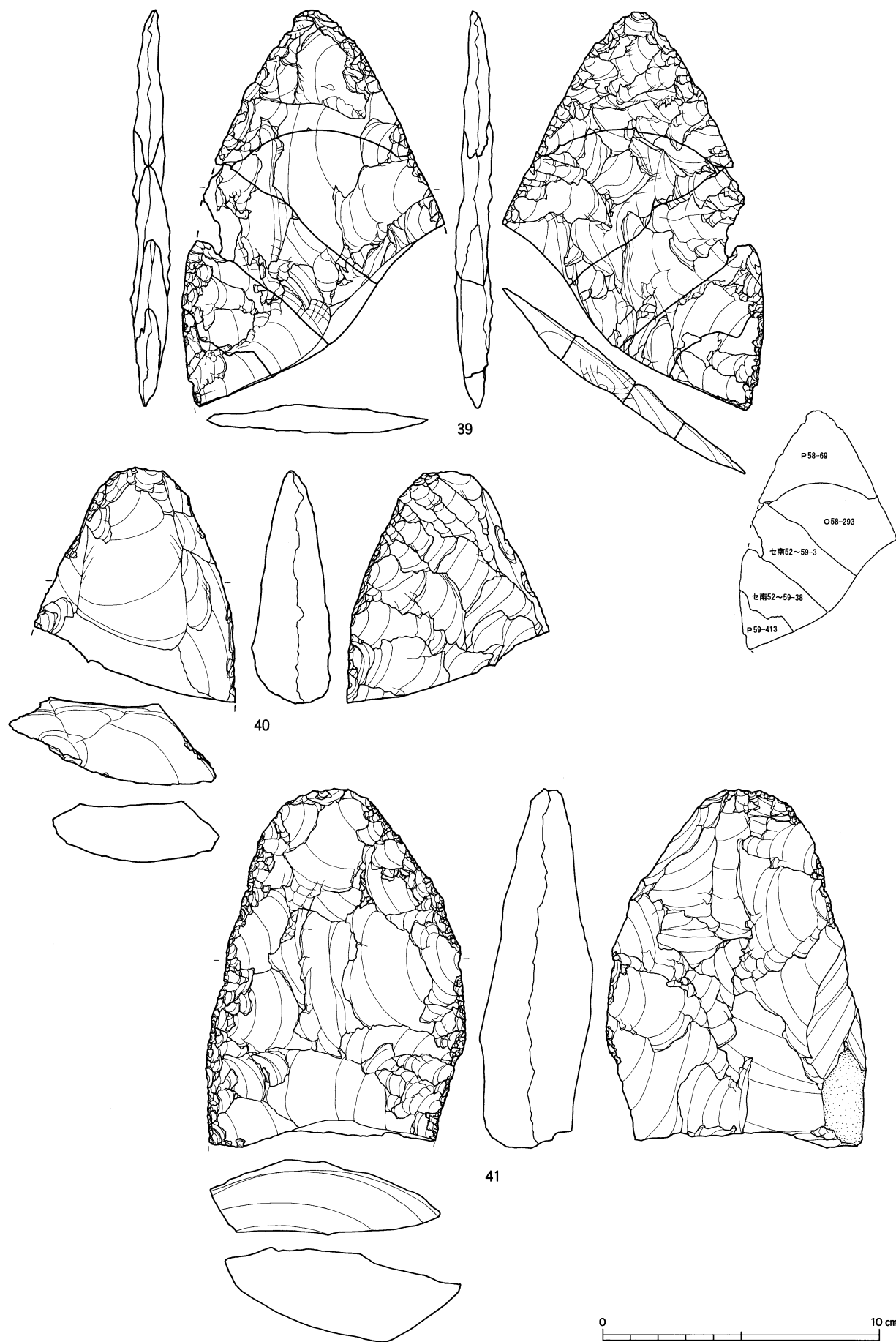
図IV-303 B区(Sb-20~29)の石器(13) 尖頭器
