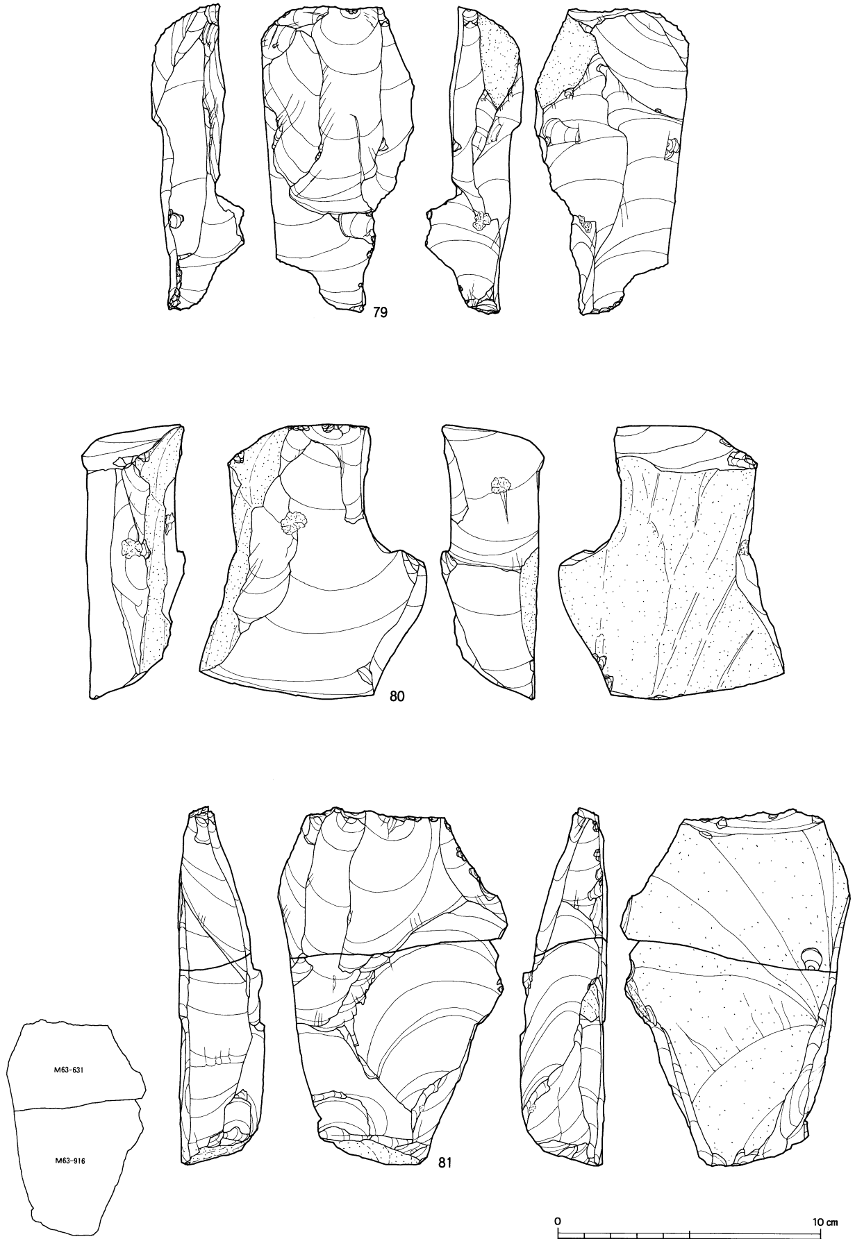
図IV-78 Sb-4~6の石器(11) 石核
