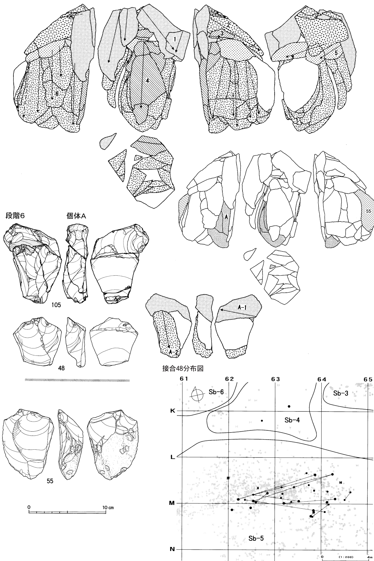
図IV-107 Sb-4~6の石器(29) 母岩22・接合48(2)
