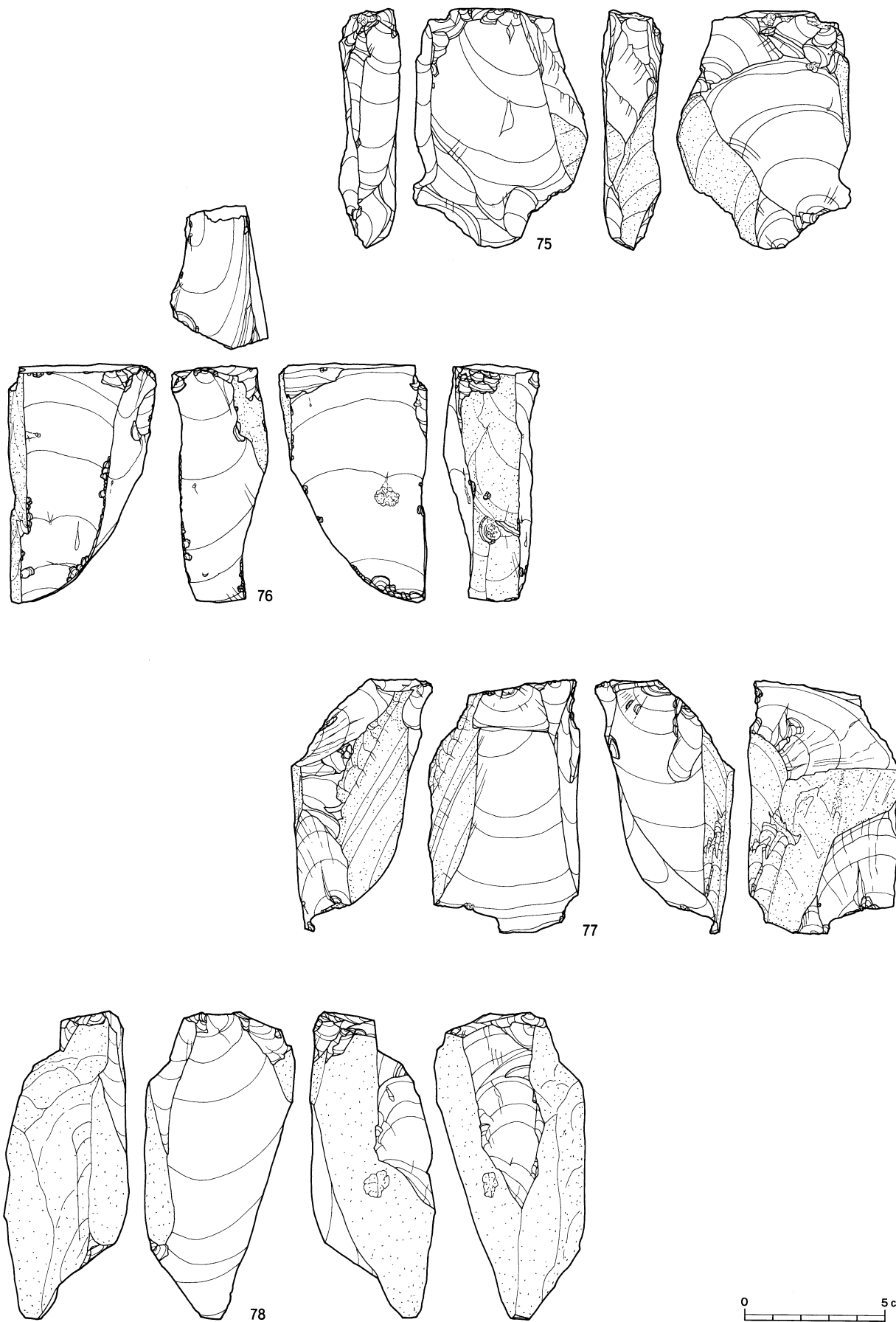
図IV-77 Sb-4~6の石器(10) 石核
