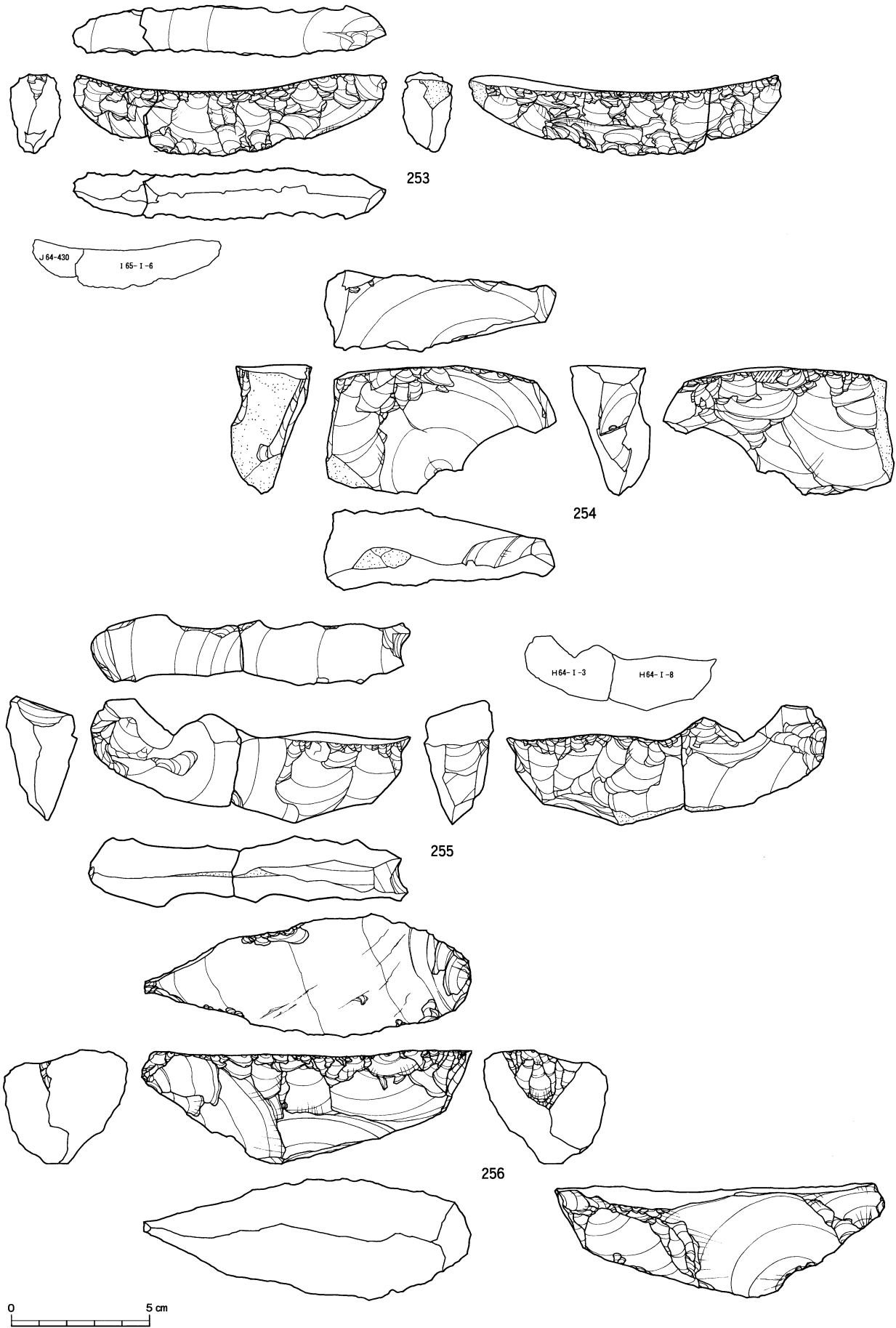
図IV-226 A区(Sb-14~19)の石器(18) 舟底形石器
