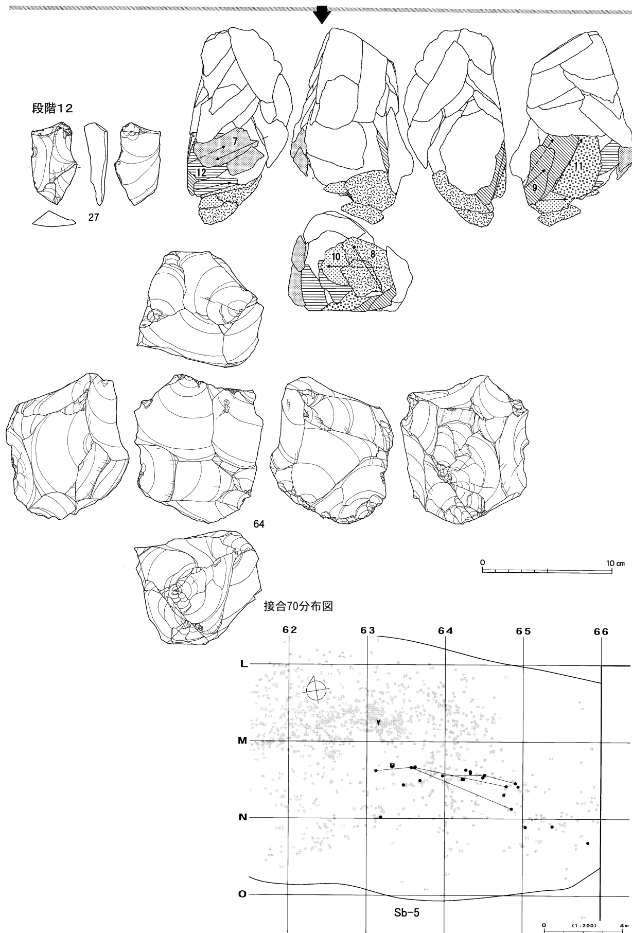
図IV-97 Sb-4~6の石器(19) 母岩32・接合70(2)
