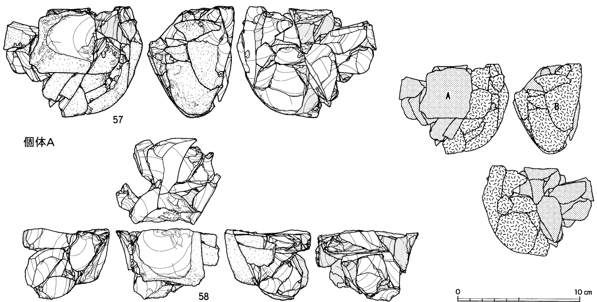
図IV-196 Sb-11~13の石器(6) 母岩459・接合278、母岩463・接合287(1)
