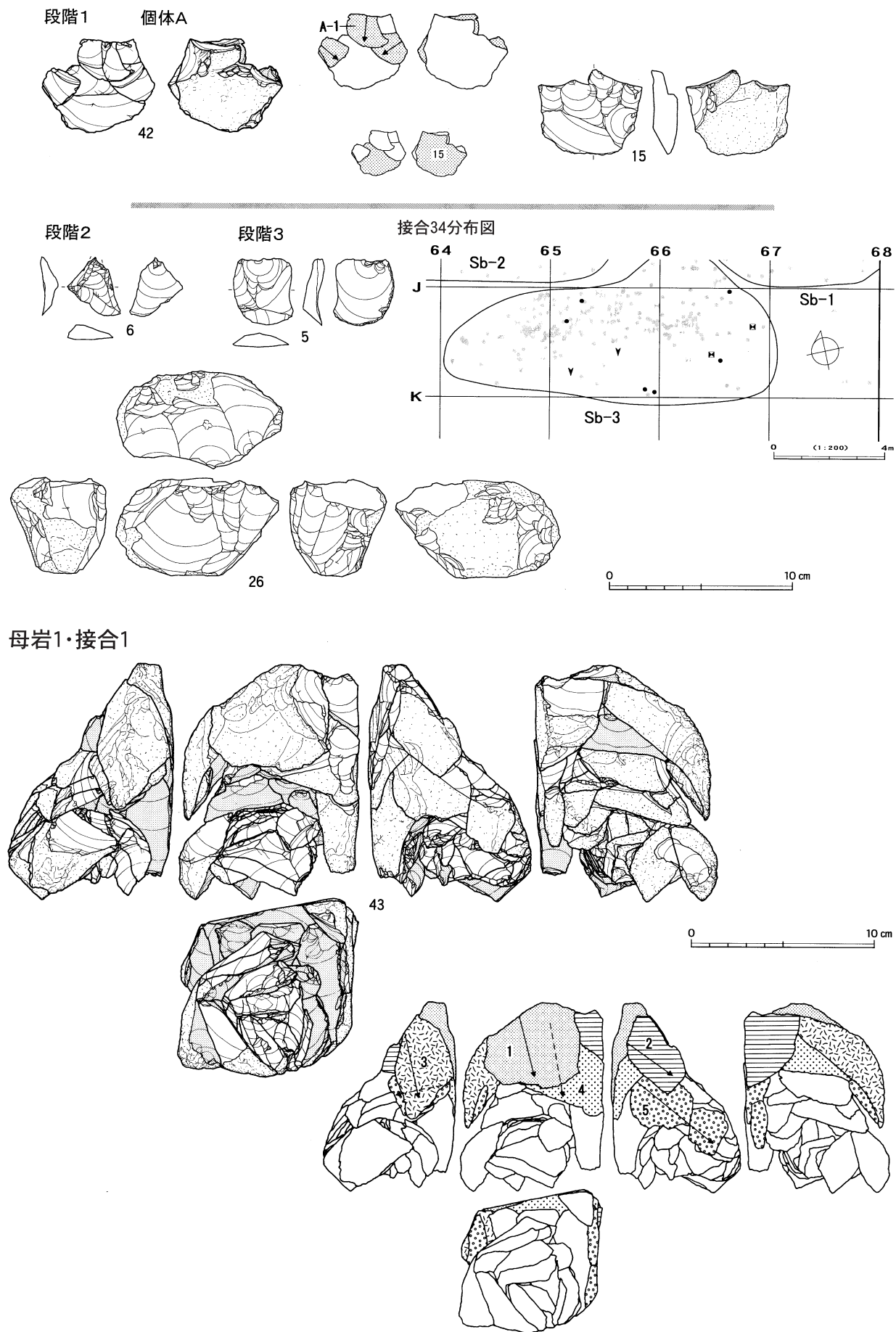
図IV-49 Sb-1~3の石器(9) 母岩17・接合34(2)、母岩1・接合1(1)
