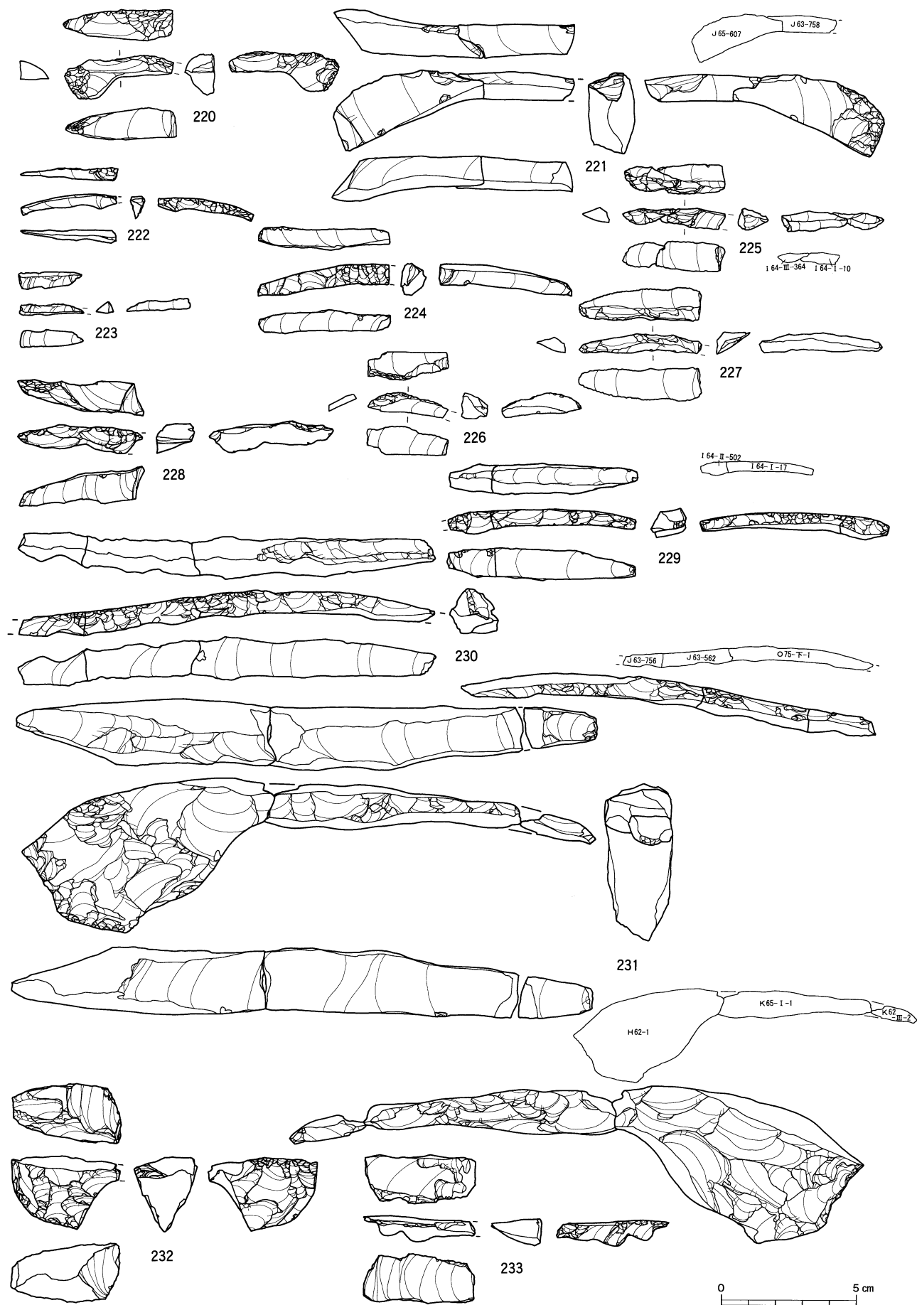
図IV-223 A区(Sb-14~19)の石器(15) 細石刃核削片
