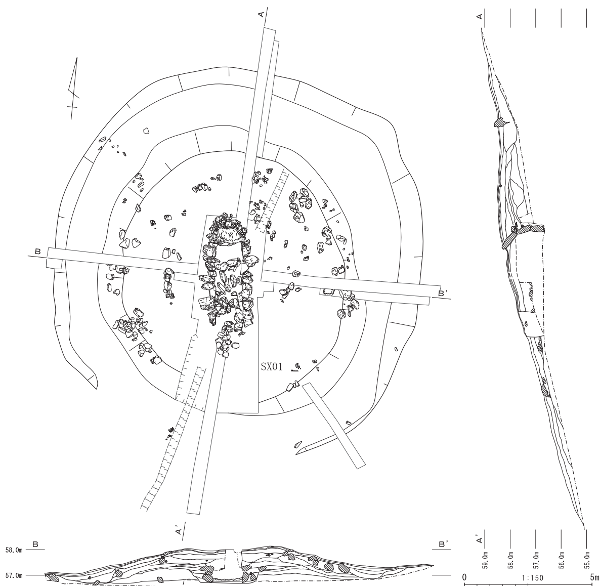
第7図 墳丘図
