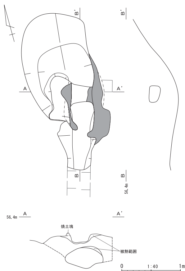
第12図 SX02実測図
