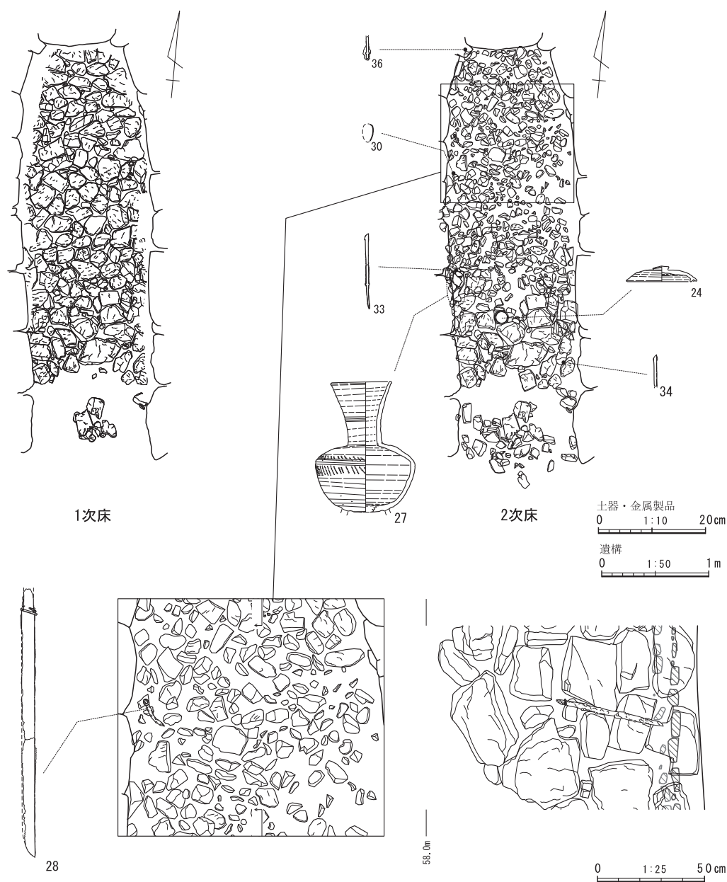
第15図 床面遺物出土状況図
