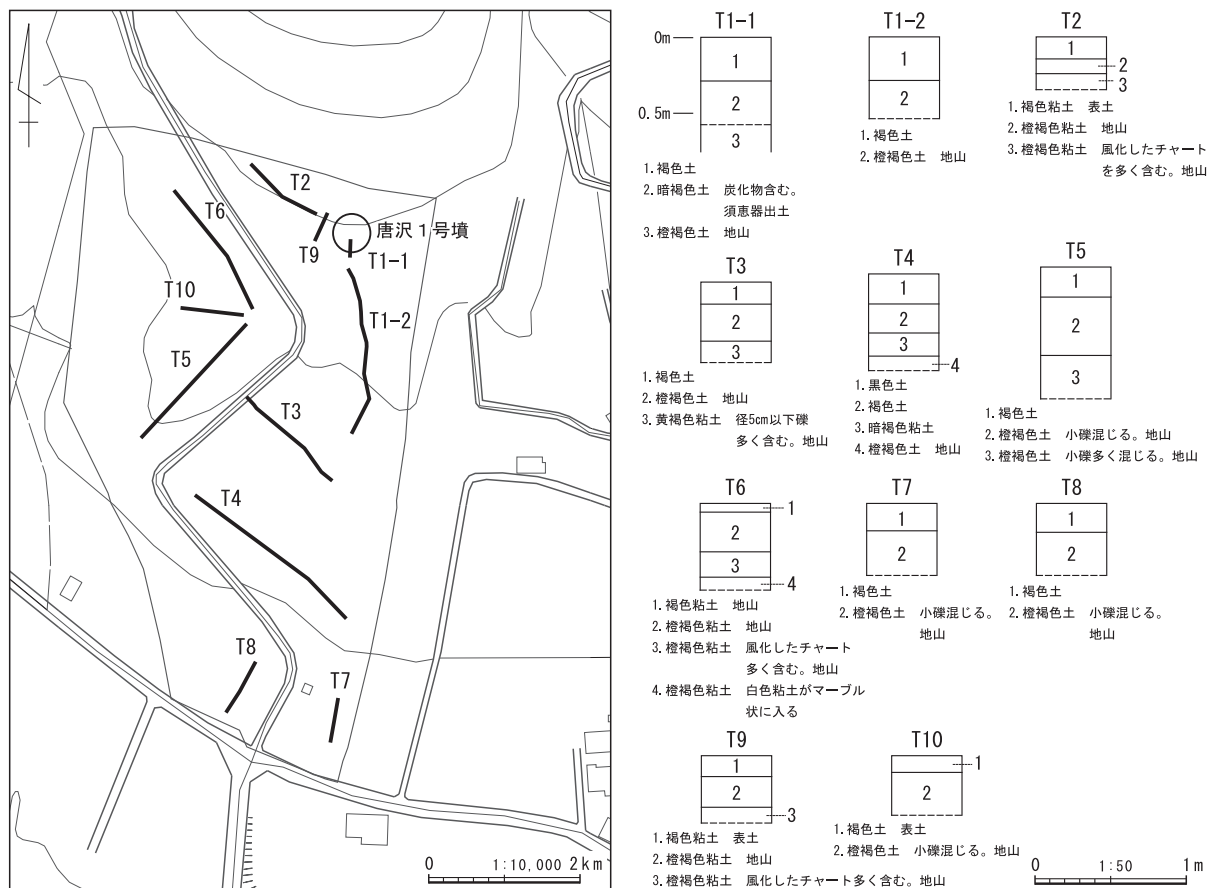
第4図 確認調査トレンチ配置図
