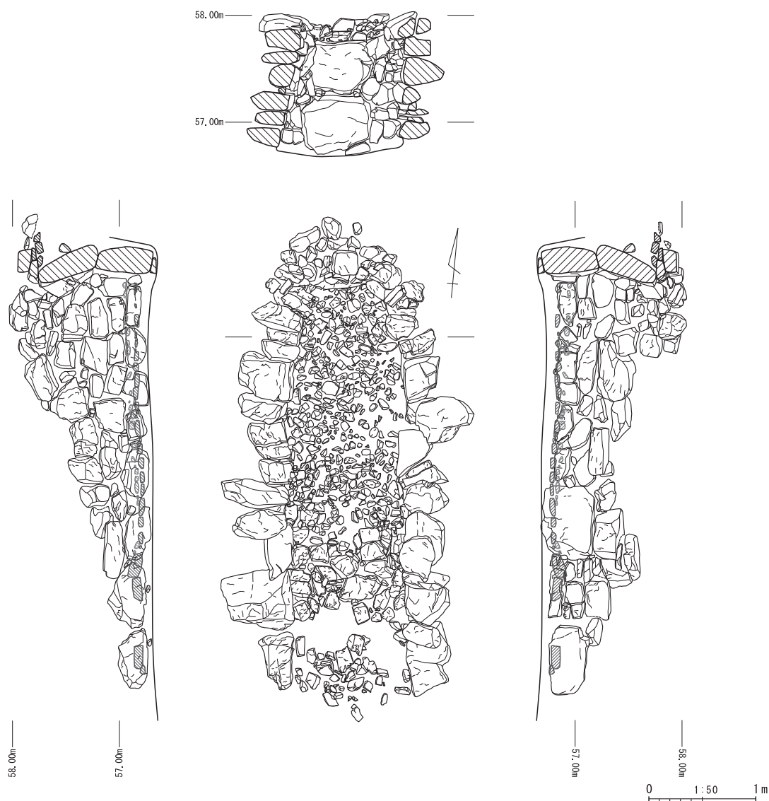
第13図 石室展開図
