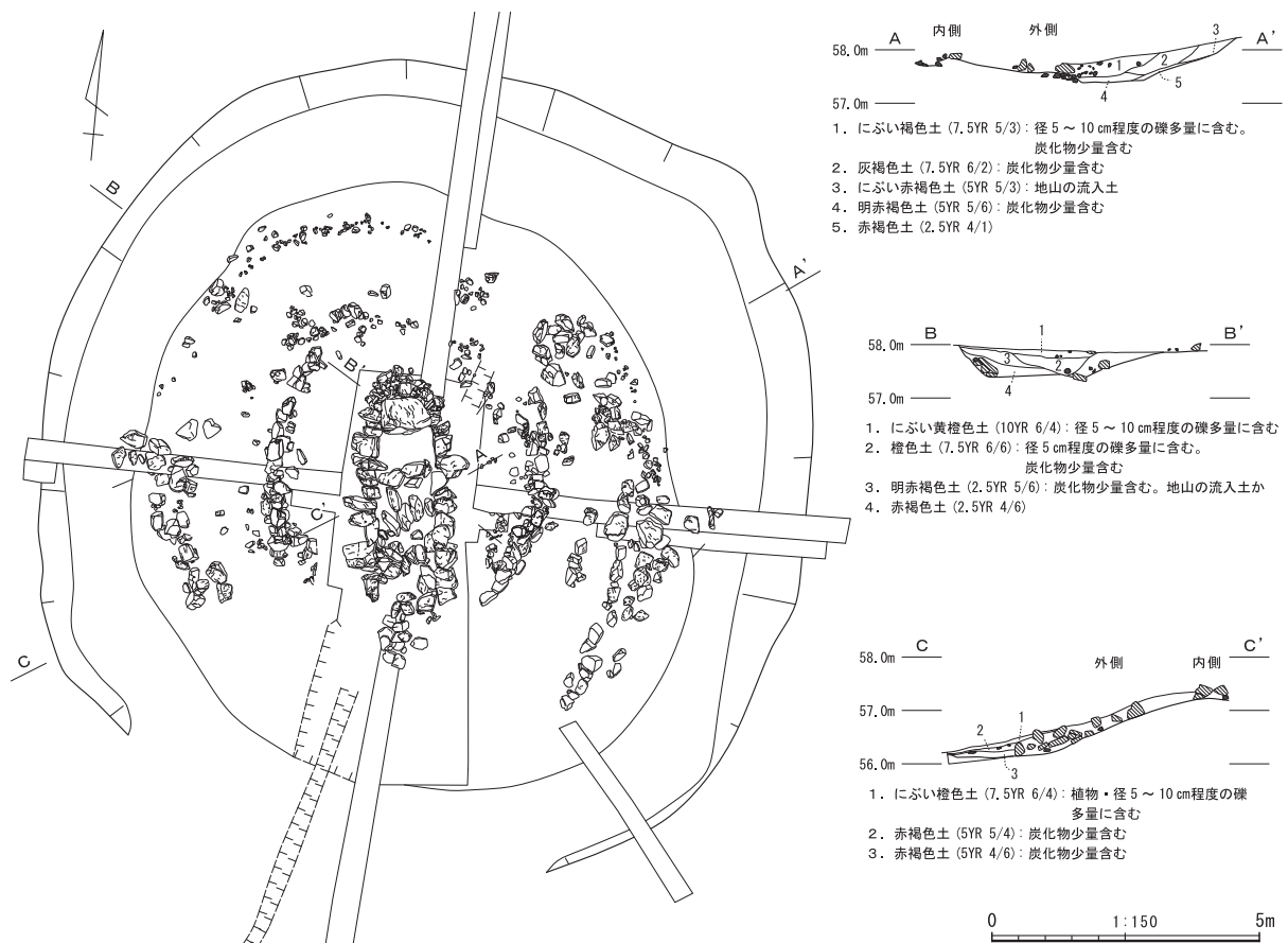
第10図 墳丘内石列検出状況図
