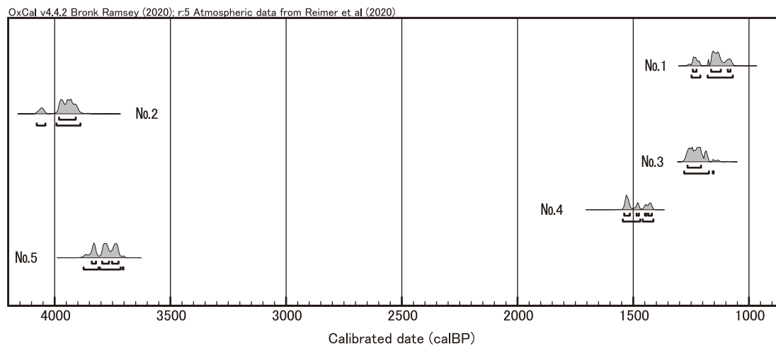
第21図 暦年較正結果
