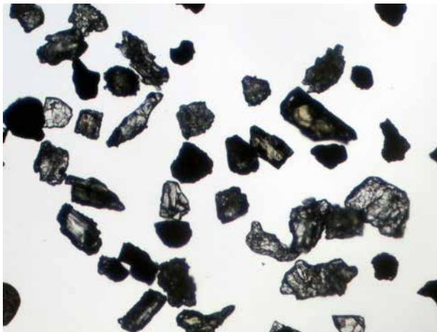
写真3 SK01 底面 SP 覆土・試料 1 (透過光) 右下：スポンジ状軽石型ガラス。 左上：繊維束状軽石型ガラス。 中央右上 (有色鉱物)：斜方輝石。
