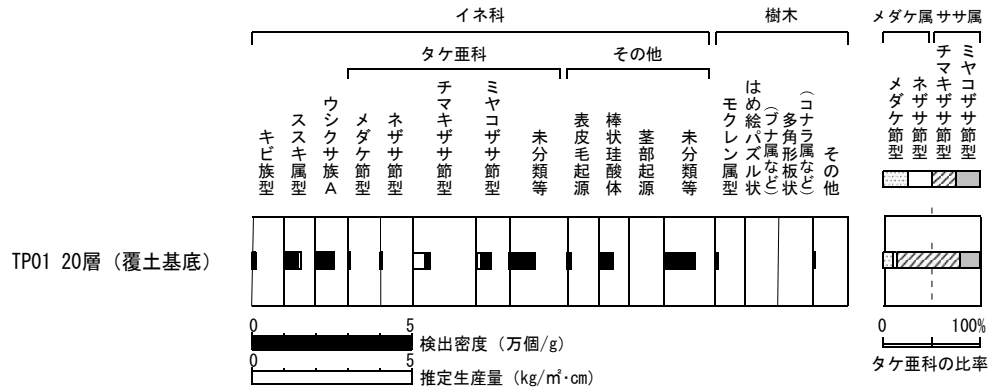
第E図 北玉川II遺跡調査区の植物珪酸体組成ダイアグラム
