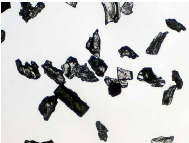
写真3 TP01・試料 25 (透過光) 上・右・右上：繊維束状軽石型ガラス. 左 (有色鉱物)：斜方輝石.
