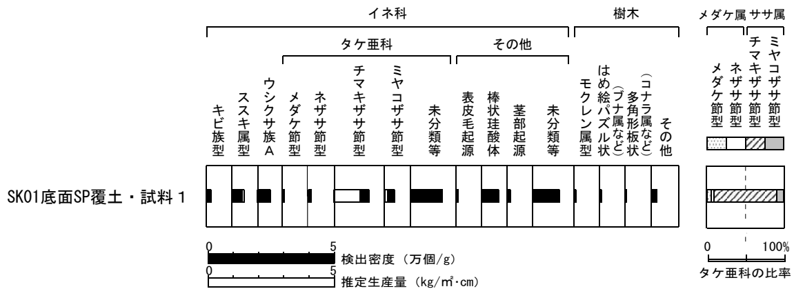
第D図 南玉川IV遺跡調査区におけるSK01底面SP覆土の植物珪酸体組成ダイアグラム
