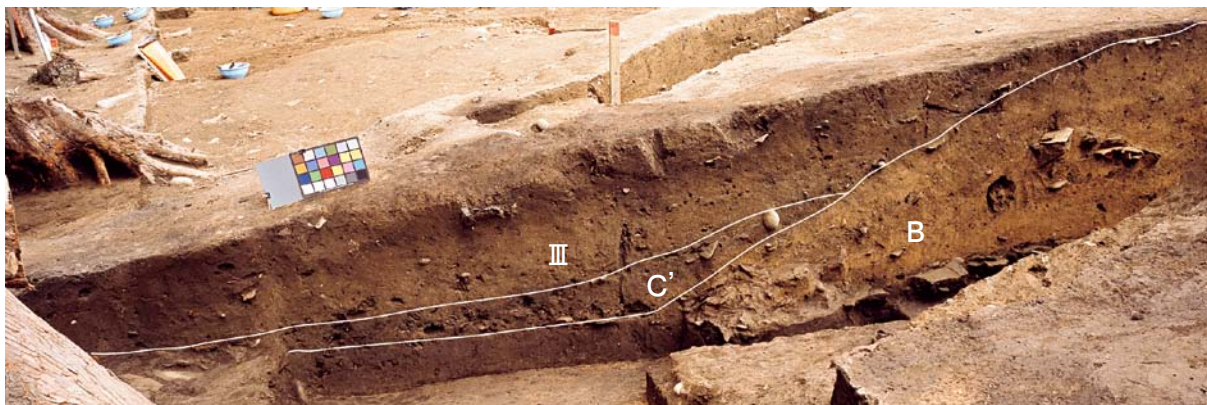
B、C' 盛土 土層断面 (G1,2区) 南東から
