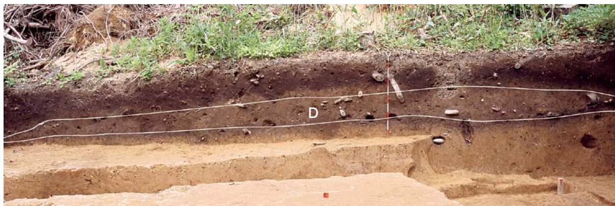
D盛土 土層断面 (C10,11区) 南東から
