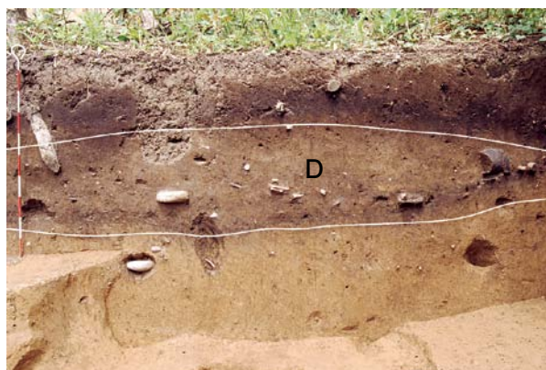
D盛土 土層断面 (C11区) 南東から
